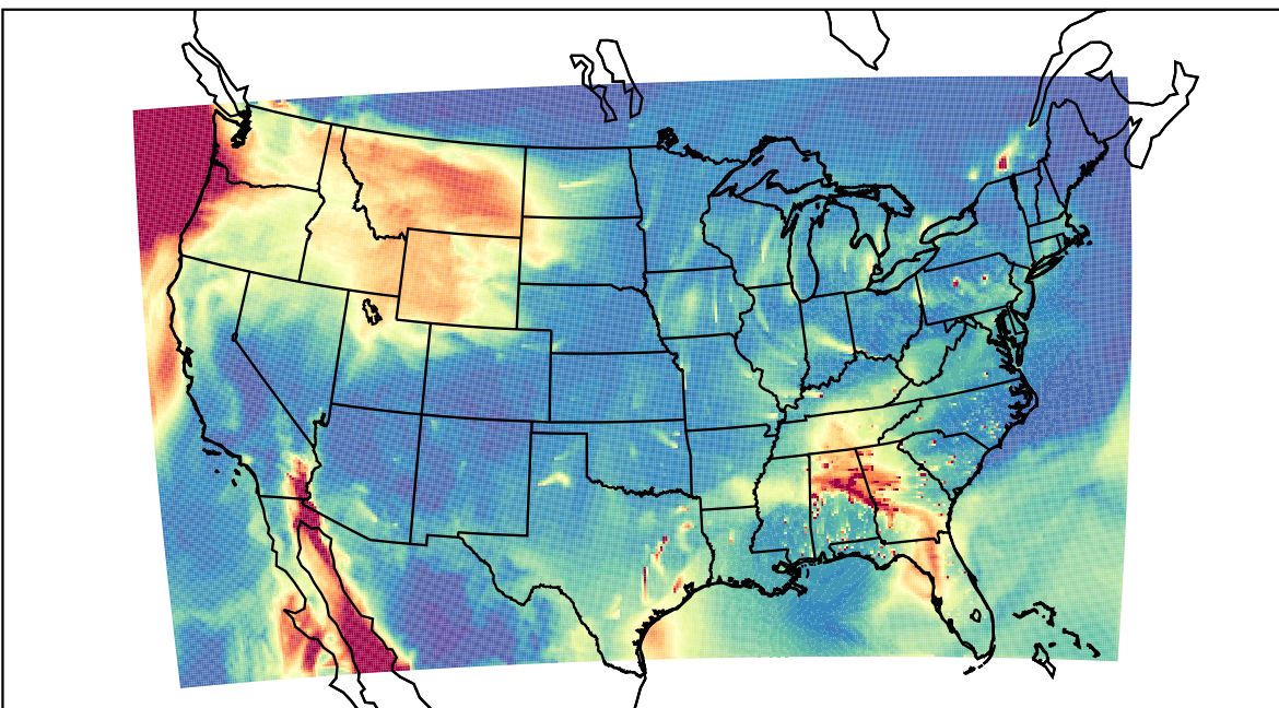
WRF 2021-02-26_17:00:00
