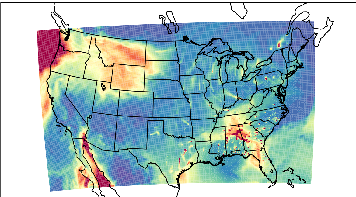
WRF 2021-02-26_18:00:00
