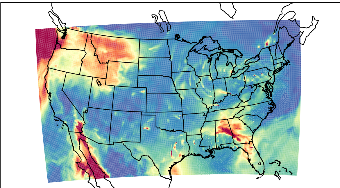
WRF 2021-02-26_15:00:00
