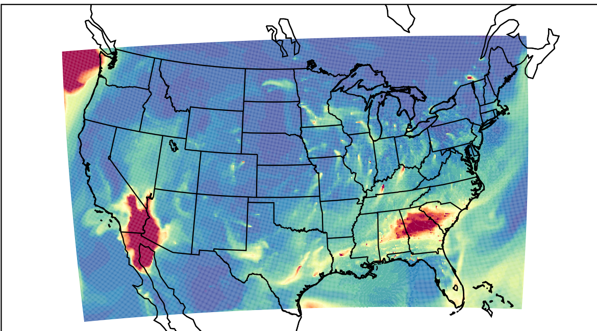
WRF 2021-02-25_13:00:00
