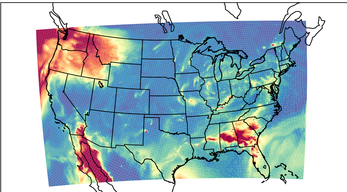
WRF 2021-02-26_10:00:00
