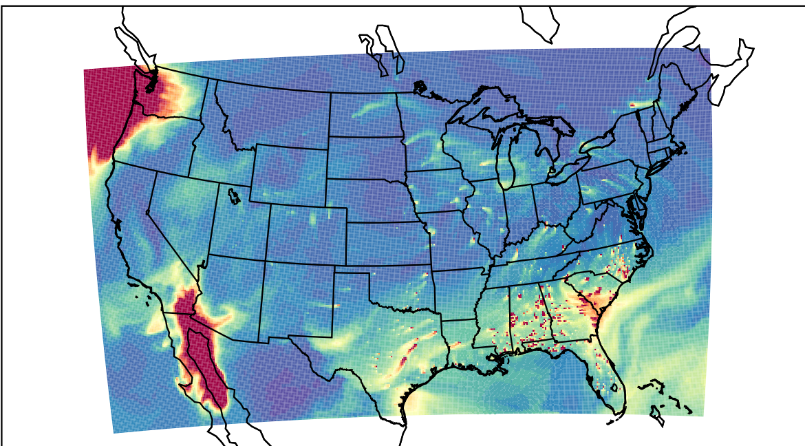
WRF 2021-02-25_20:00:00
