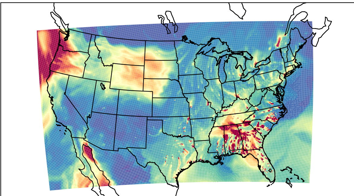
WRF 2021-02-26_23:00:00
