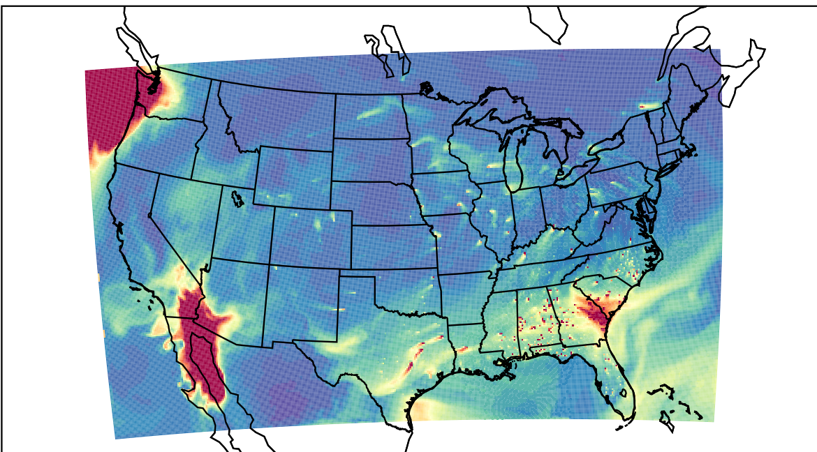
WRF 2021-02-25_18:00:00
