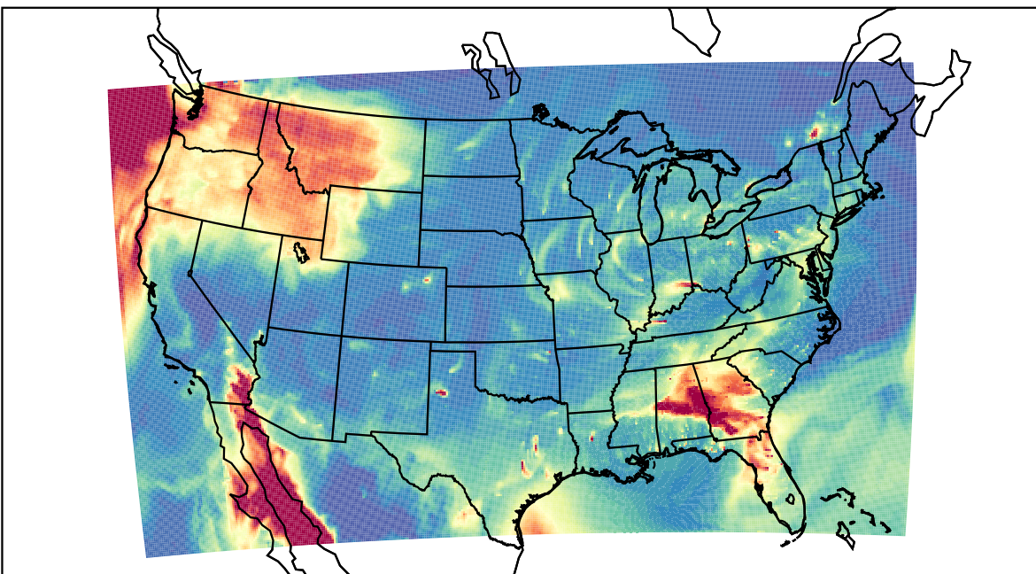
WRF 2021-02-26_13:00:00
