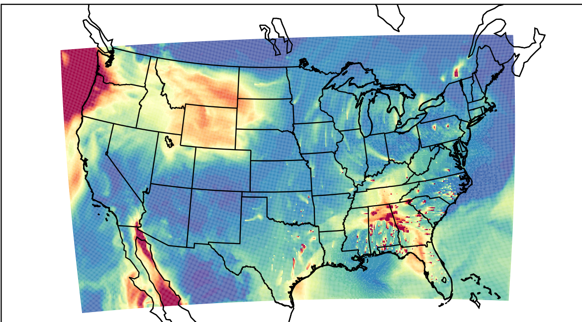
WRF 2021-02-26_19:00:00
