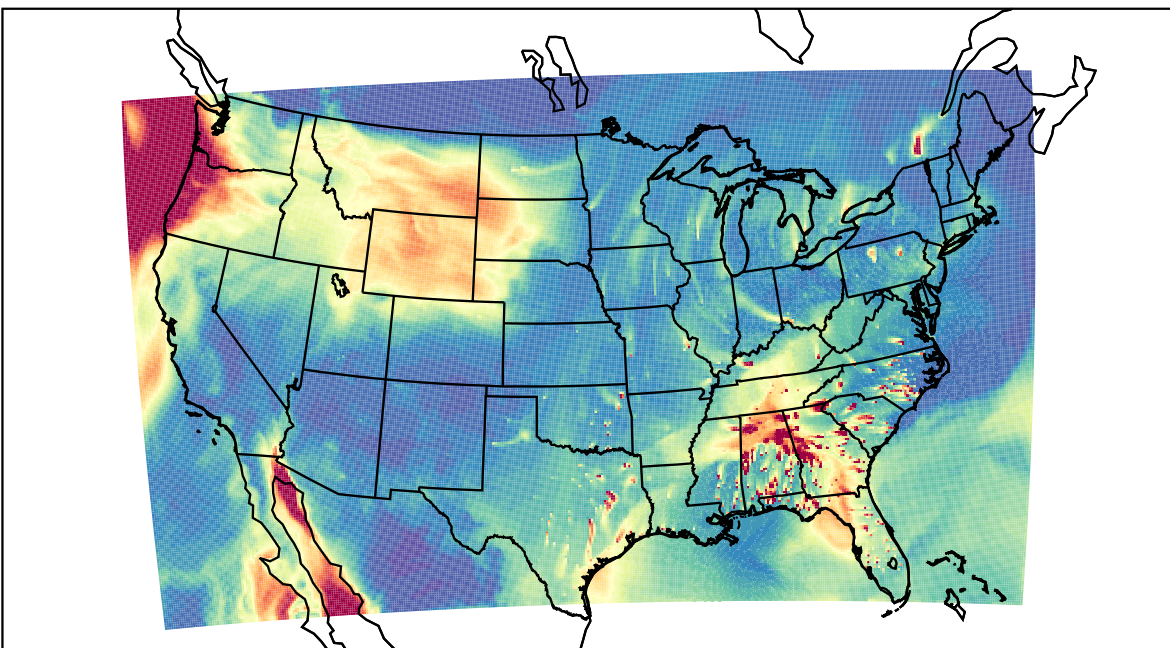
WRF 2021-02-26_20:00:00
