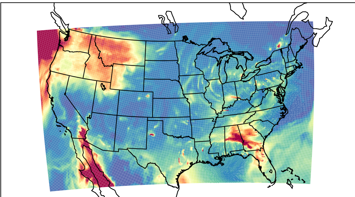
WRF 2021-02-26_14:00:00
