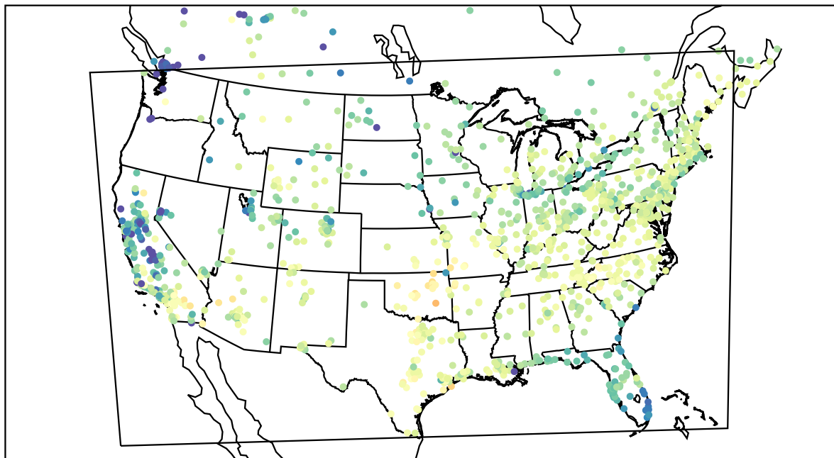
AirNOW (2021-03-03_18:00:00)
