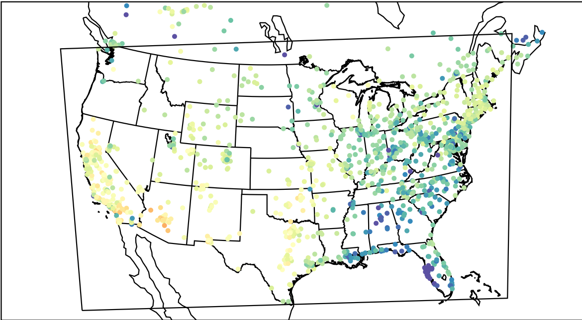
AirNOW (2021-03-02_23:00:00)
