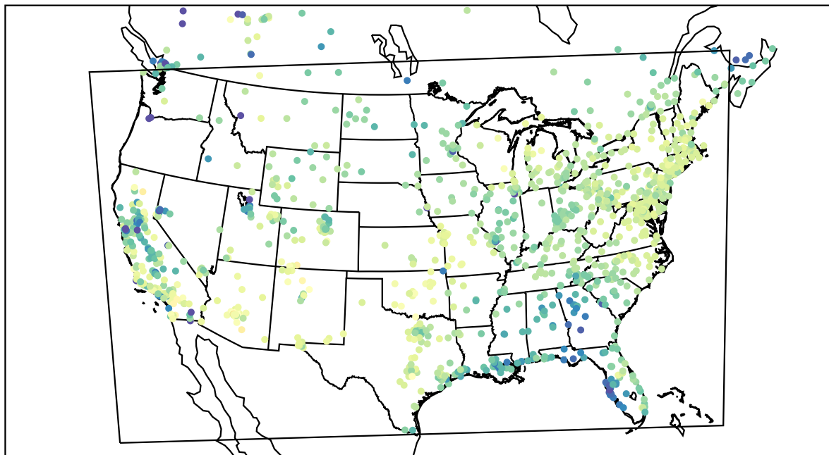
AirNOW (2021-03-02_18:00:00)
