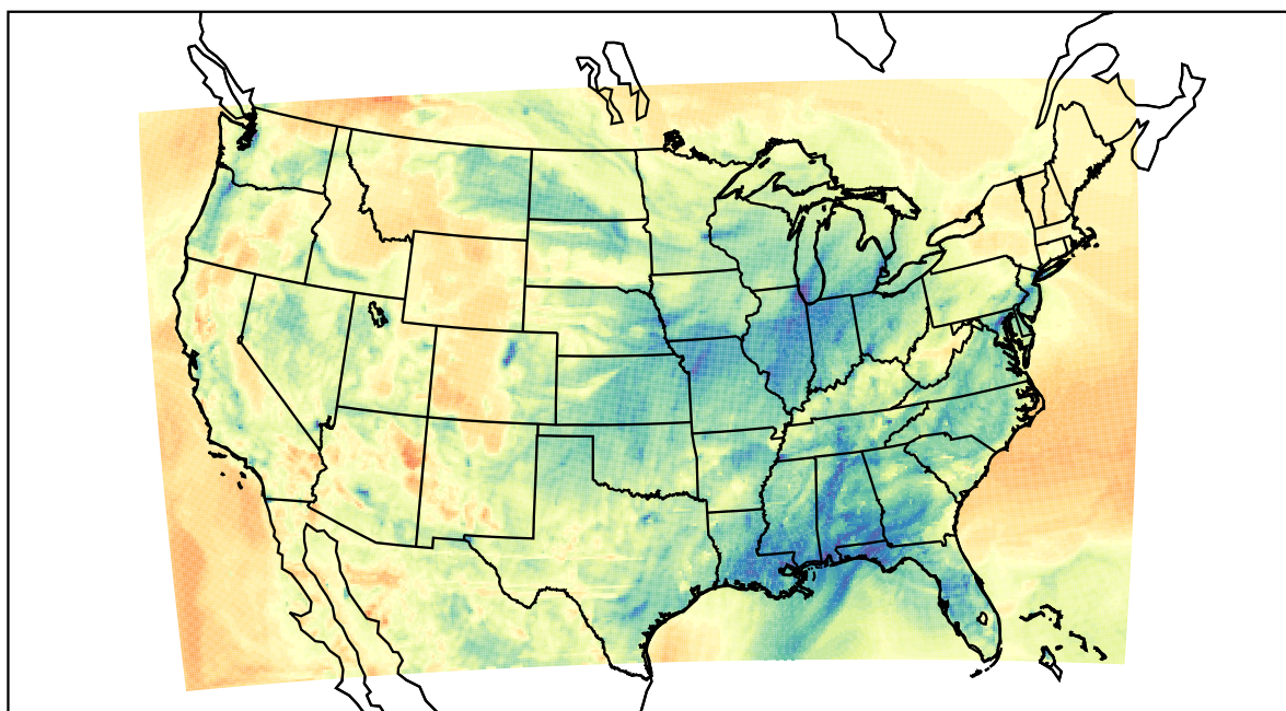
WRF (2021-03-03_03:00:00)
