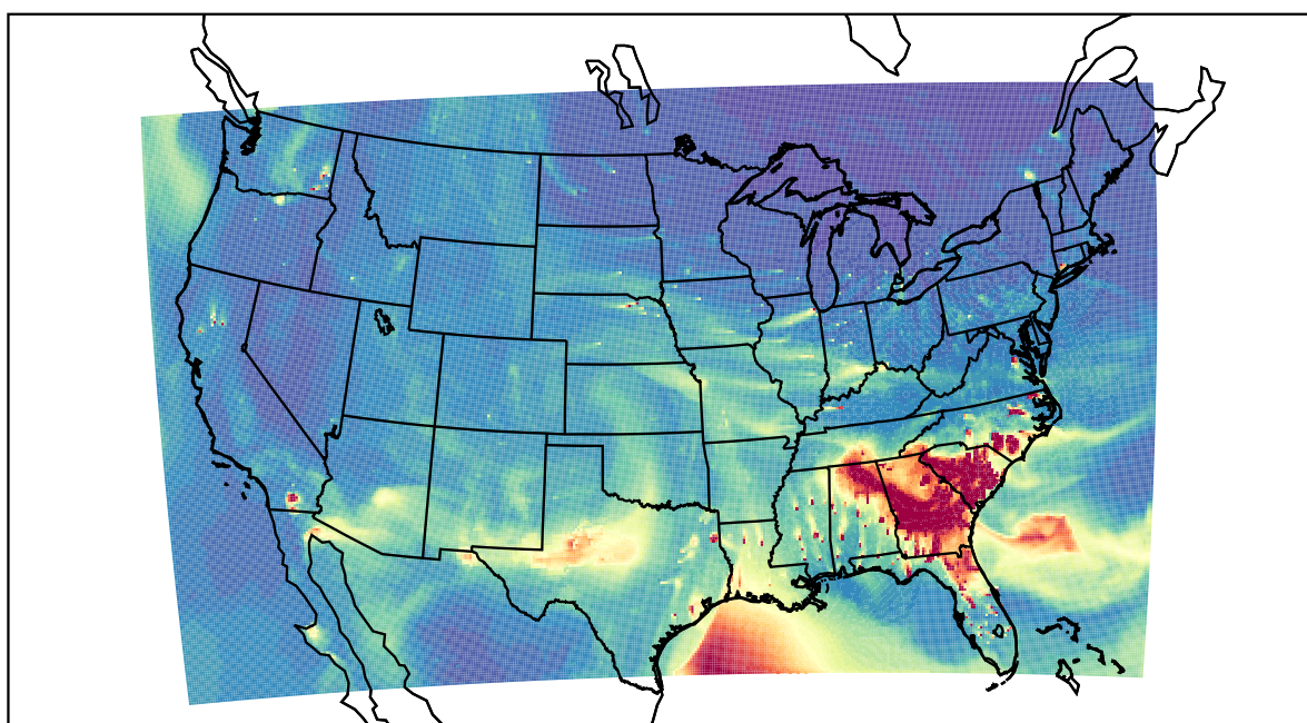
WRF 2021-03-14_23:00:00
