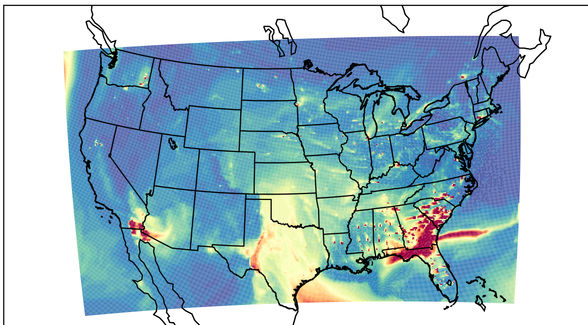
WRF 2021-03-13_23:00:00
