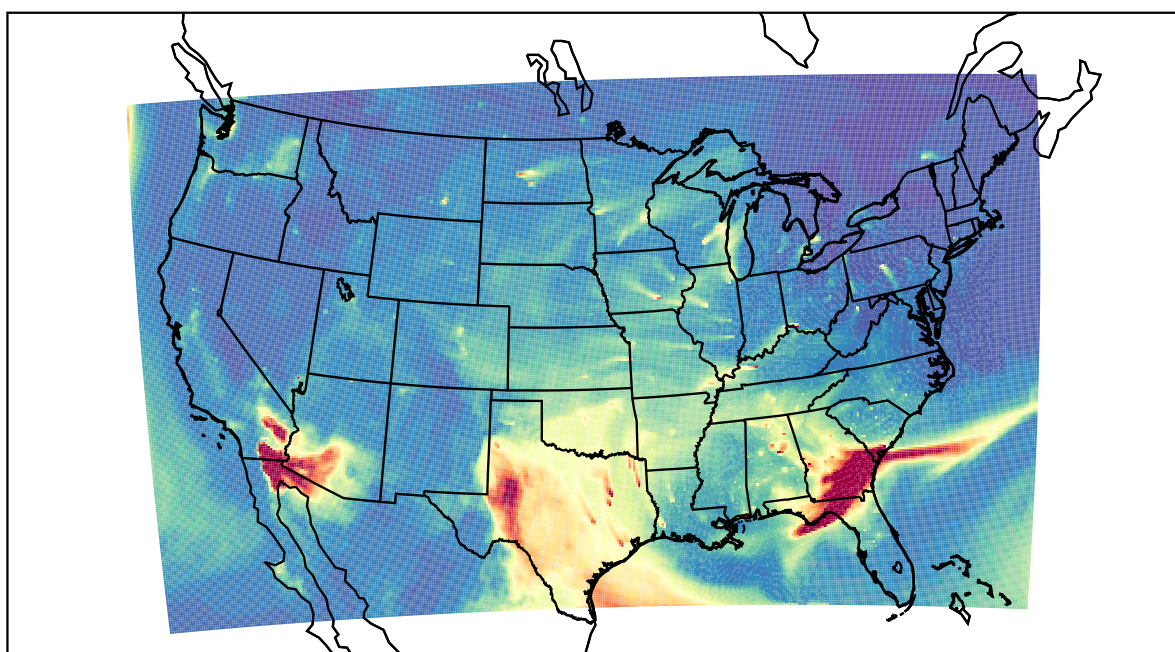
WRF 2021-03-13_16:00:00
