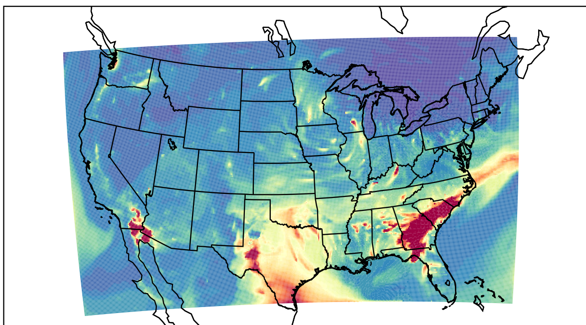
WRF 2021-03-13_06:00:00
