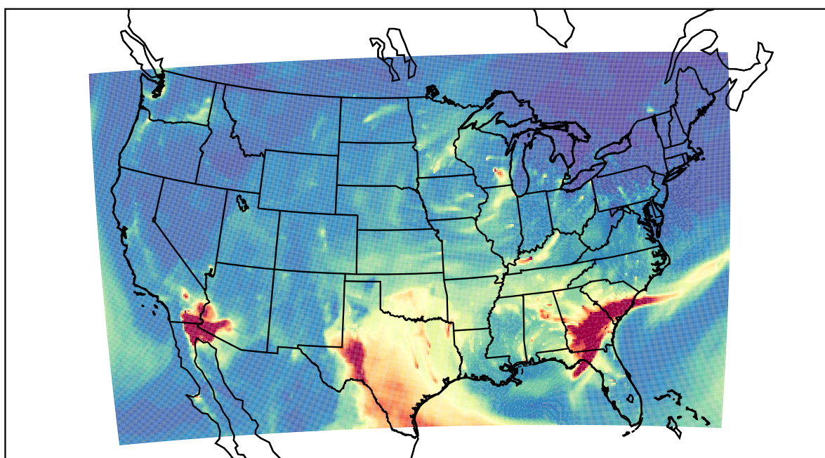
WRF 2021-03-13_11:00:00
