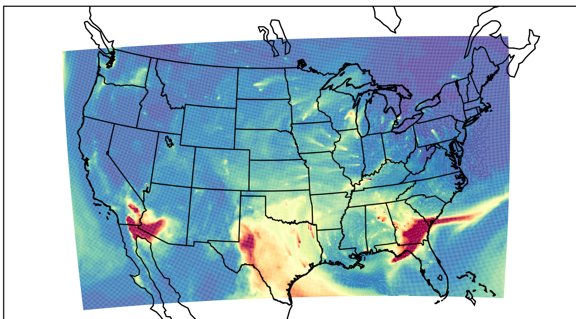
WRF 2021-03-13_15:00:00
