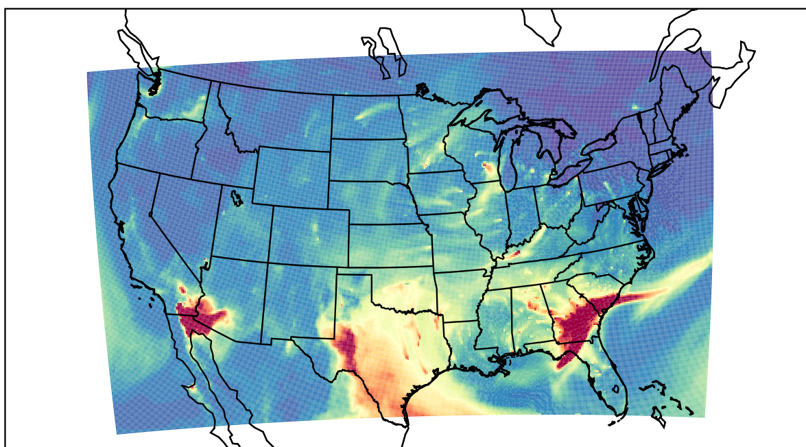
WRF 2021-03-13_12:00:00
