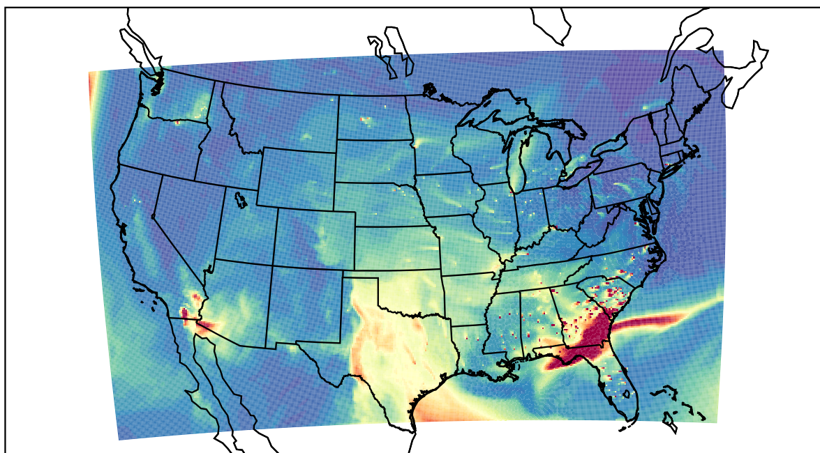
WRF 2021-03-13_20:00:00
