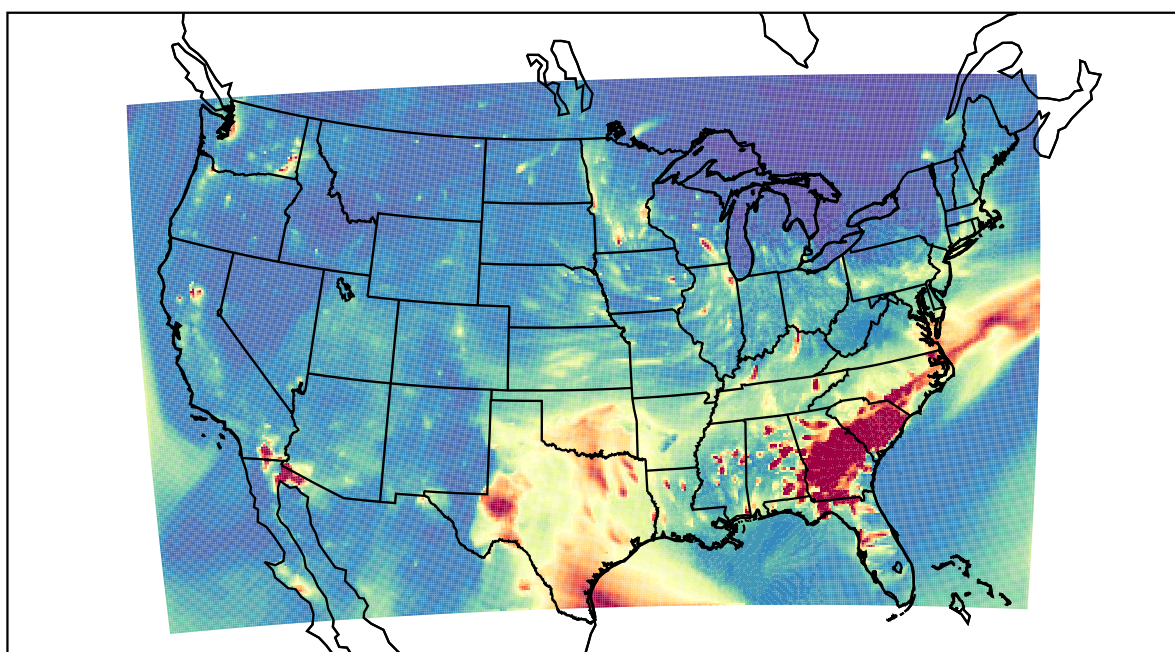
WRF 2021-03-13_03:00:00
