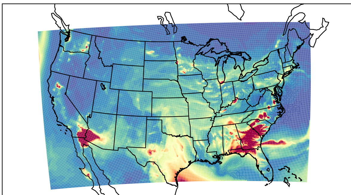
WRF 2021-03-14_04:00:00
