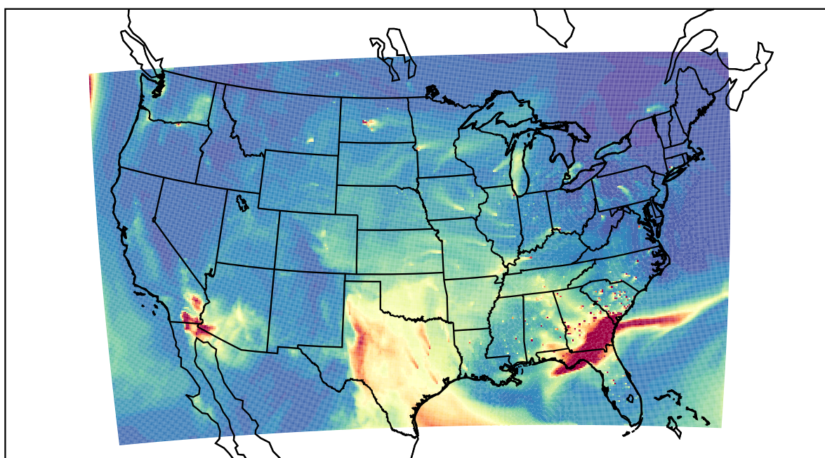
WRF 2021-03-13_18:00:00
