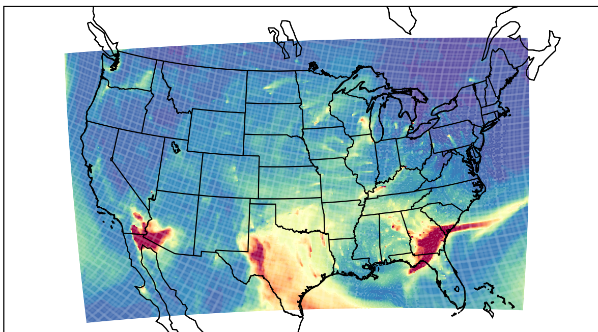
WRF 2021-03-13_14:00:00
