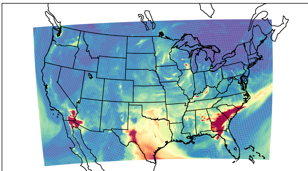
WRF 2021-03-13_08:00:00
