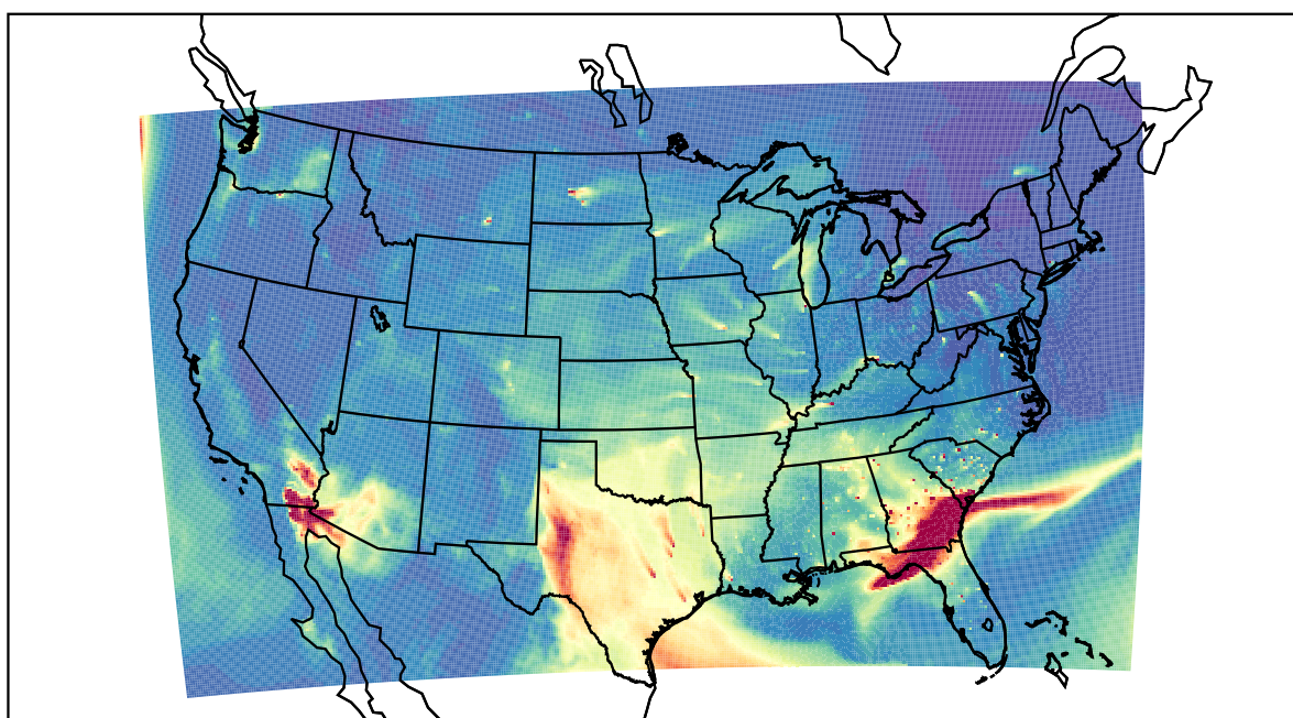
WRF 2021-03-13_17:00:00
