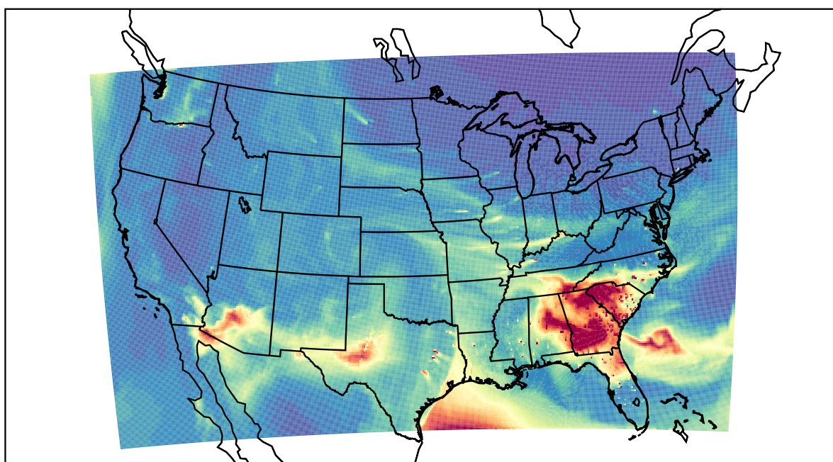
WRF 2021-03-14_18:00:00
