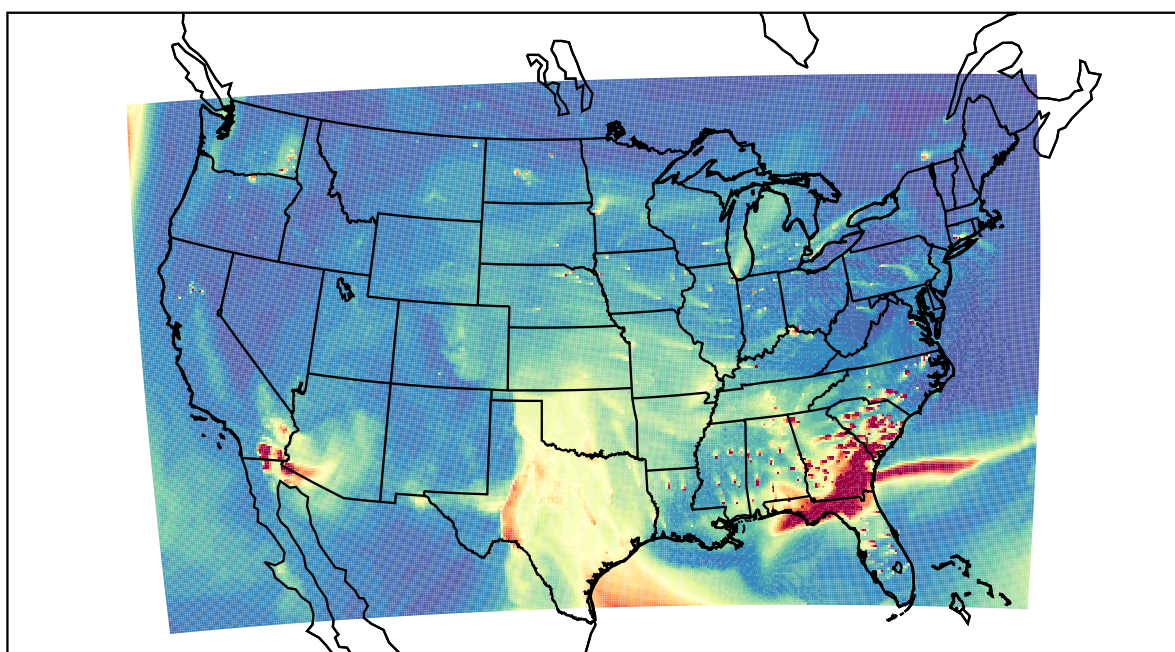
WRF 2021-03-13_22:00:00
