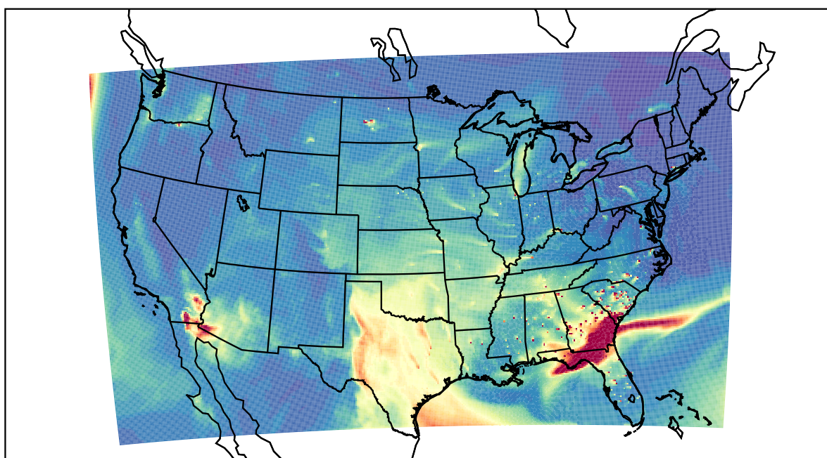
WRF 2021-03-13_19:00:00
