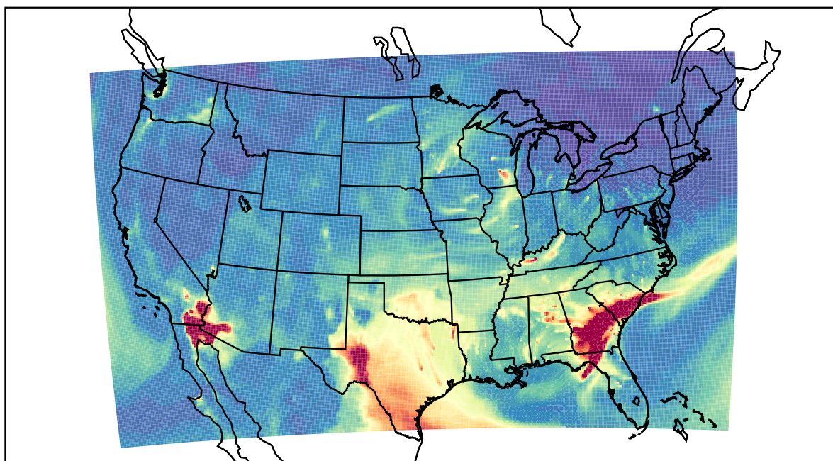
WRF 2021-03-13_10:00:00
