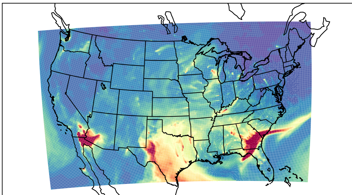
WRF 2021-03-13_13:00:00
