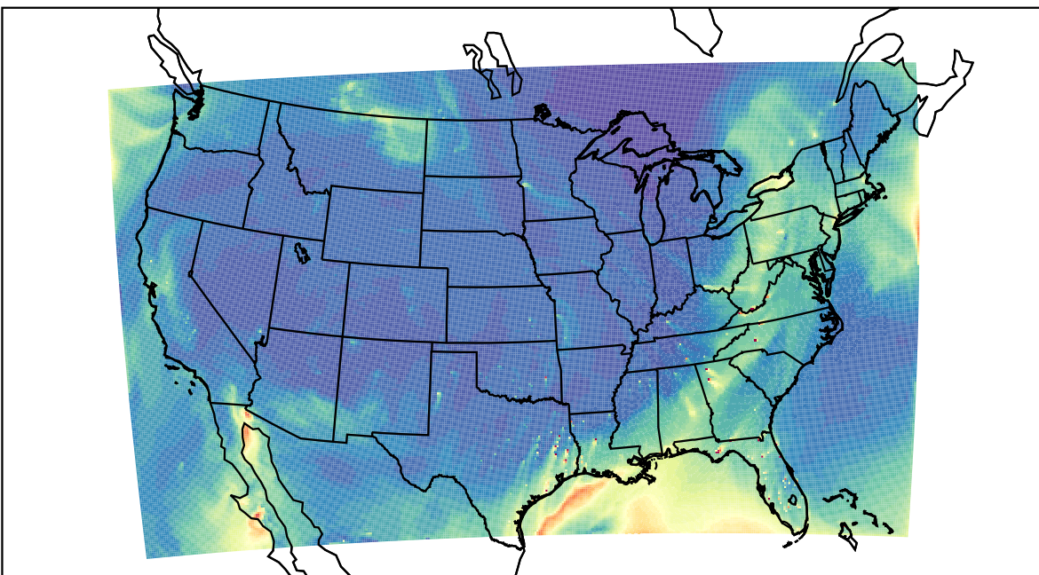
WRF 2021-03-28_20:00:00
