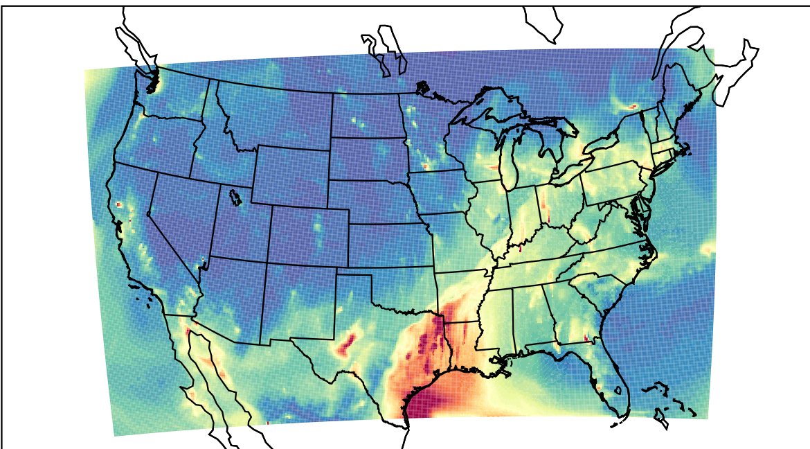
WRF 2021-03-28_04:00:00
