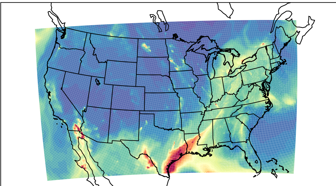
WRF 2021-03-28_11:00:00
