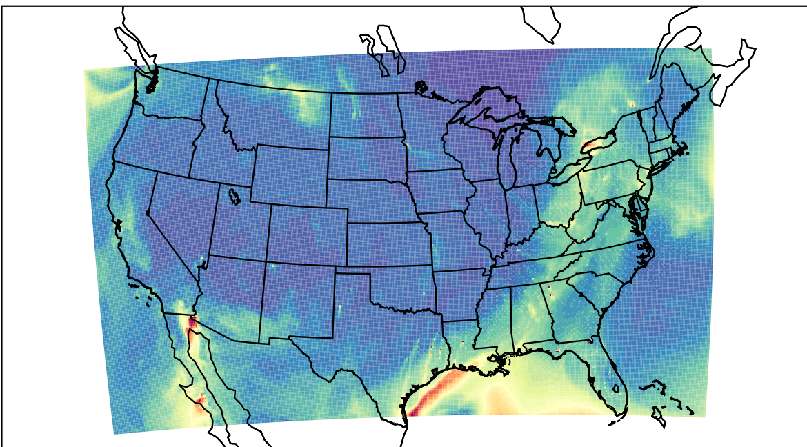
WRF 2021-03-28_18:00:00
