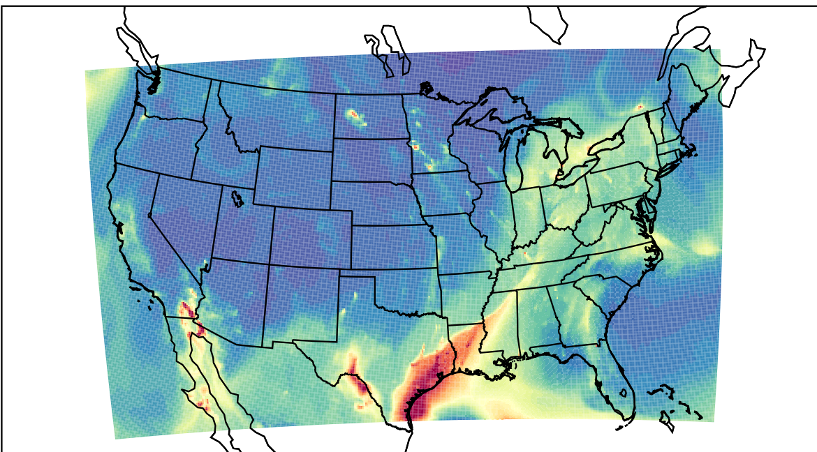
WRF 2021-03-28_10:00:00
