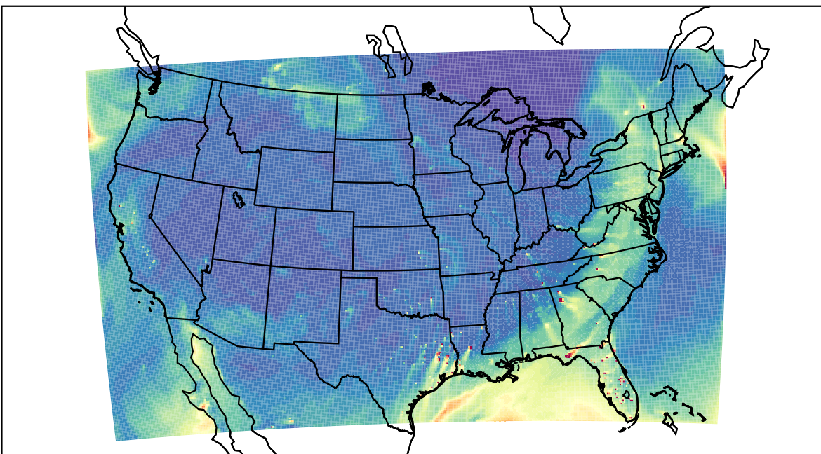
WRF 2021-03-28_23:00:00
