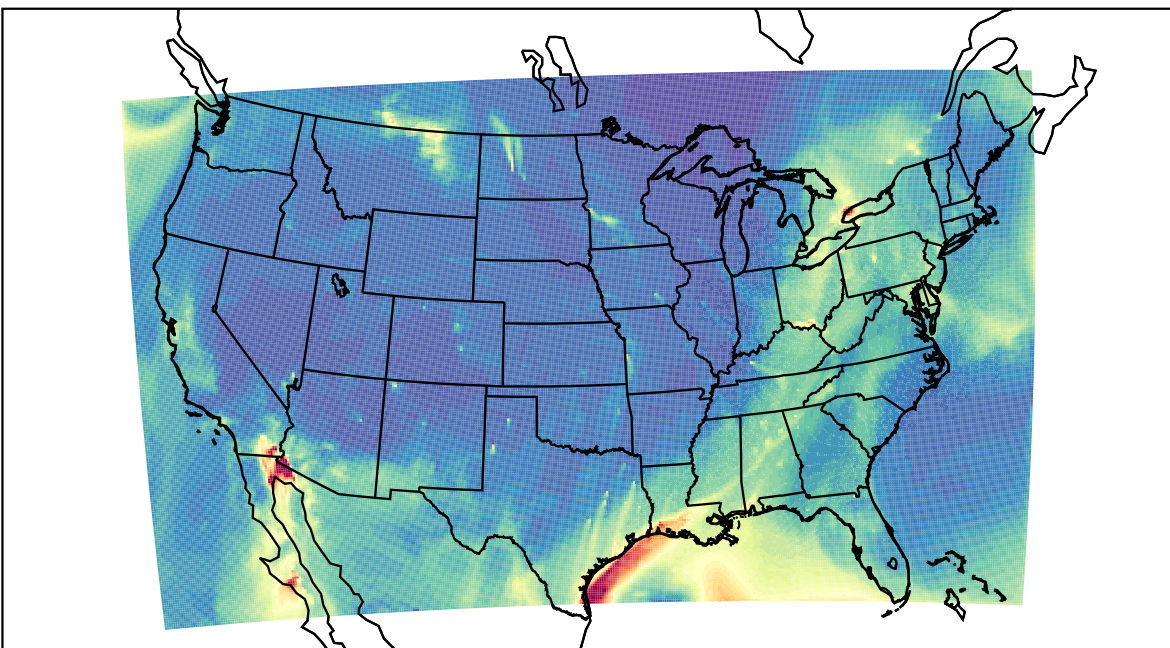
WRF 2021-03-28_16:00:00
