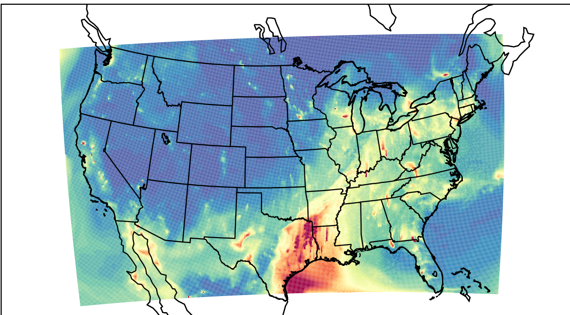
WRF 2021-03-28_03:00:00
