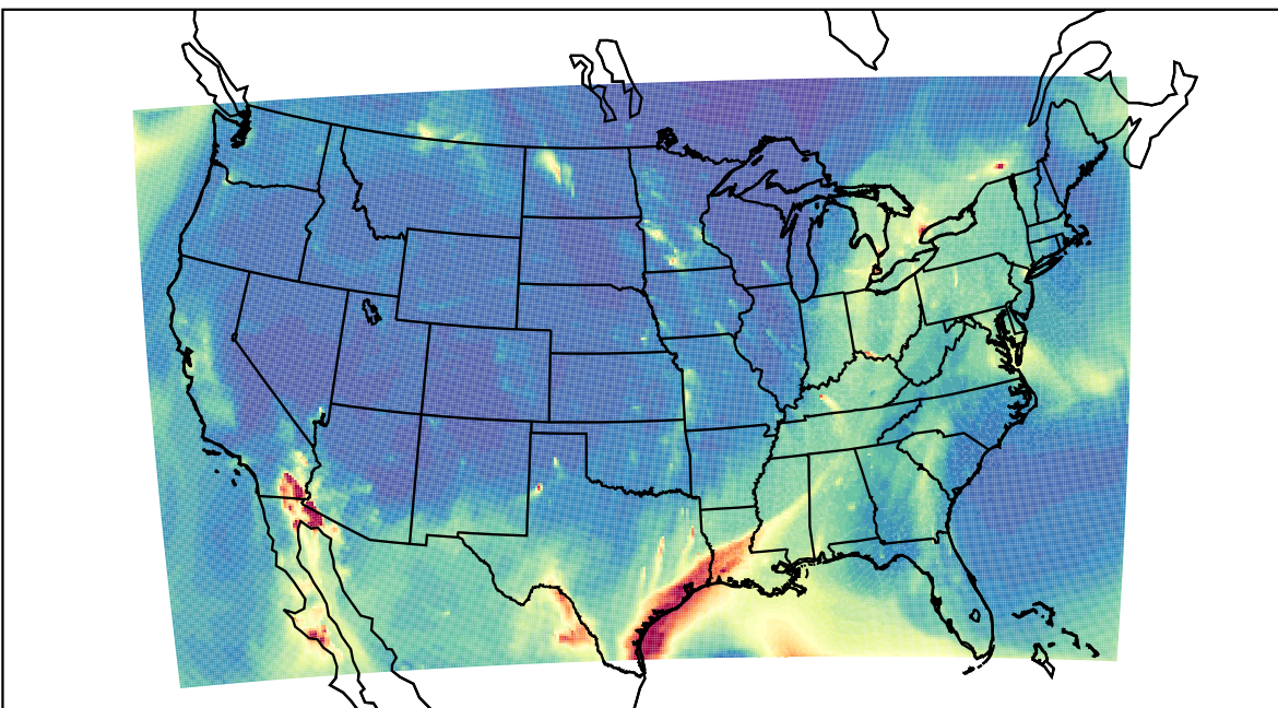
WRF 2021-03-28_13:00:00
