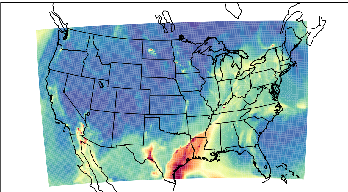
WRF 2021-03-28_08:00:00
