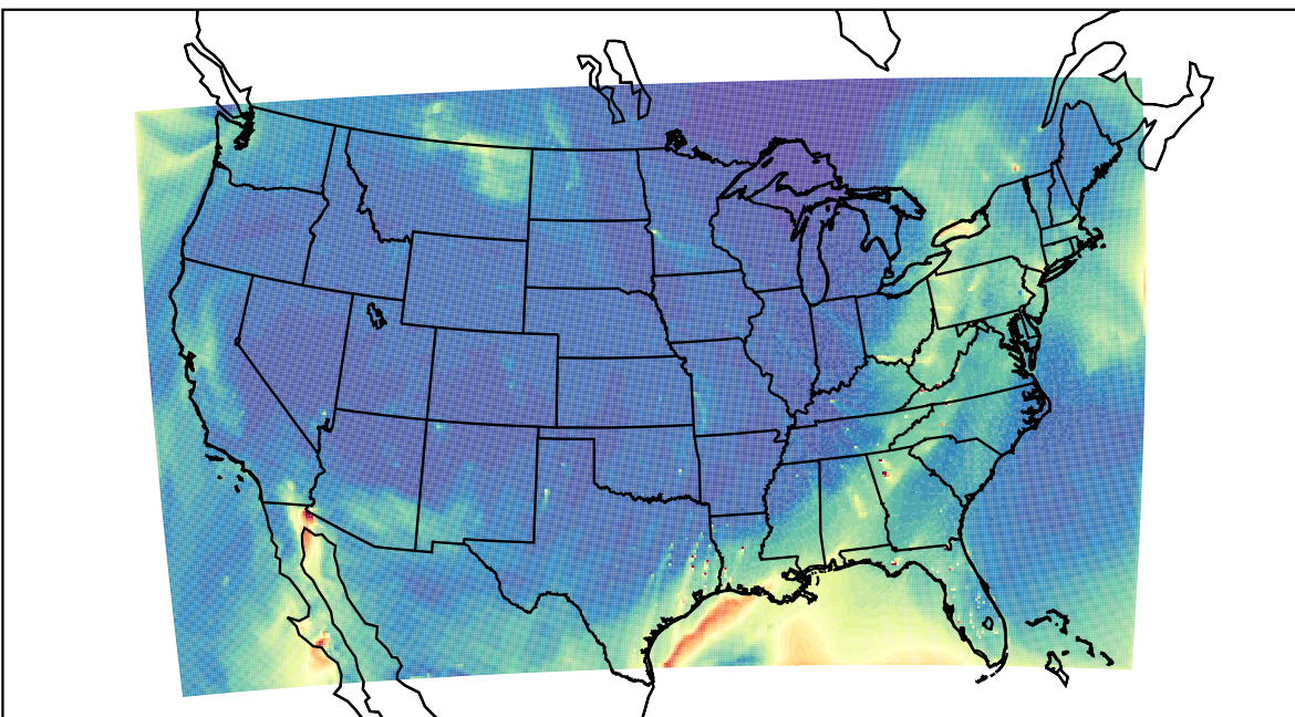
WRF 2021-03-28_19:00:00
