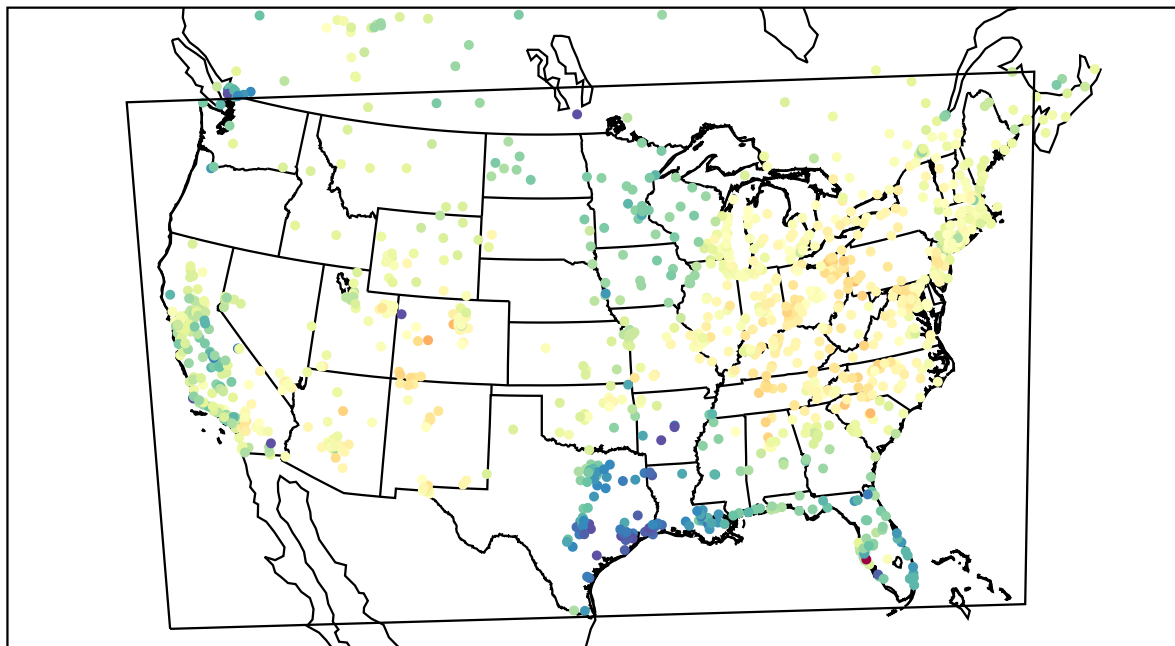
AirNOW (2021-03-30_18:00:00)
