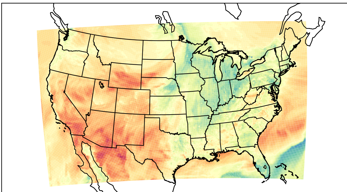
WRF (2021-03-30_00:00:00)
