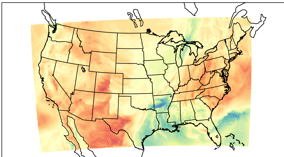
WRF (2021-03-30_20:00:00)
