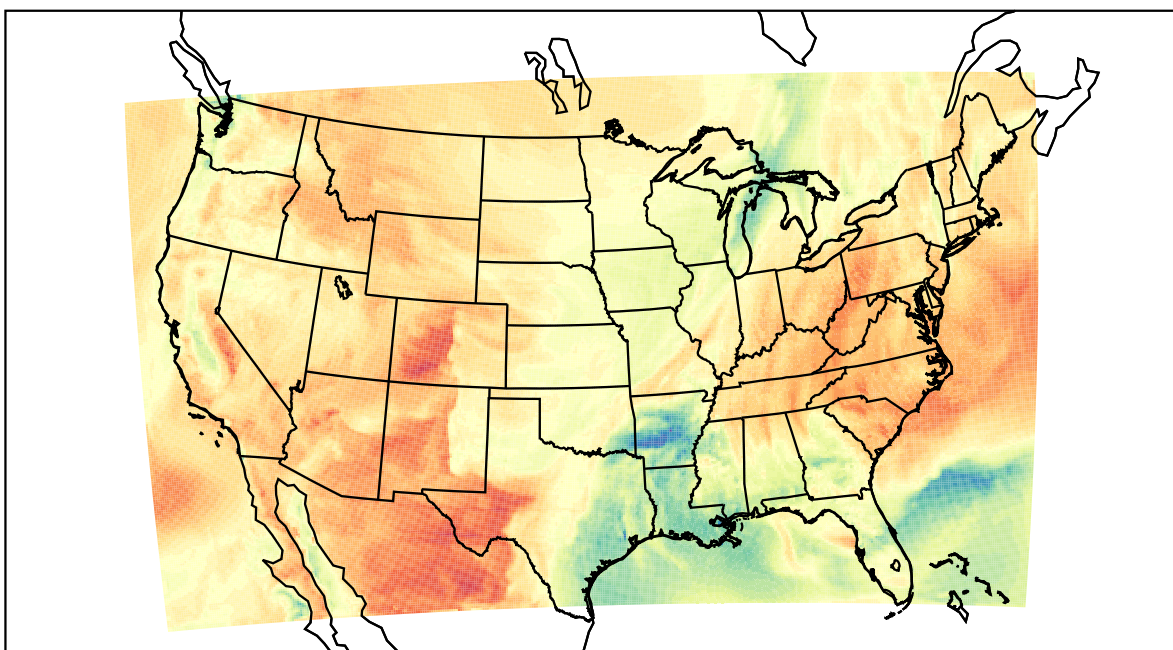
WRF (2021-03-30_19:00:00)
