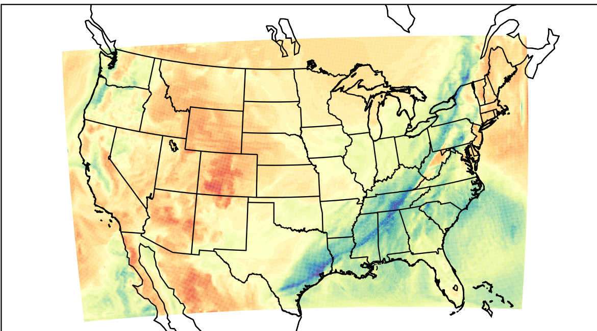
WRF (2021-03-31_18:00:00)
