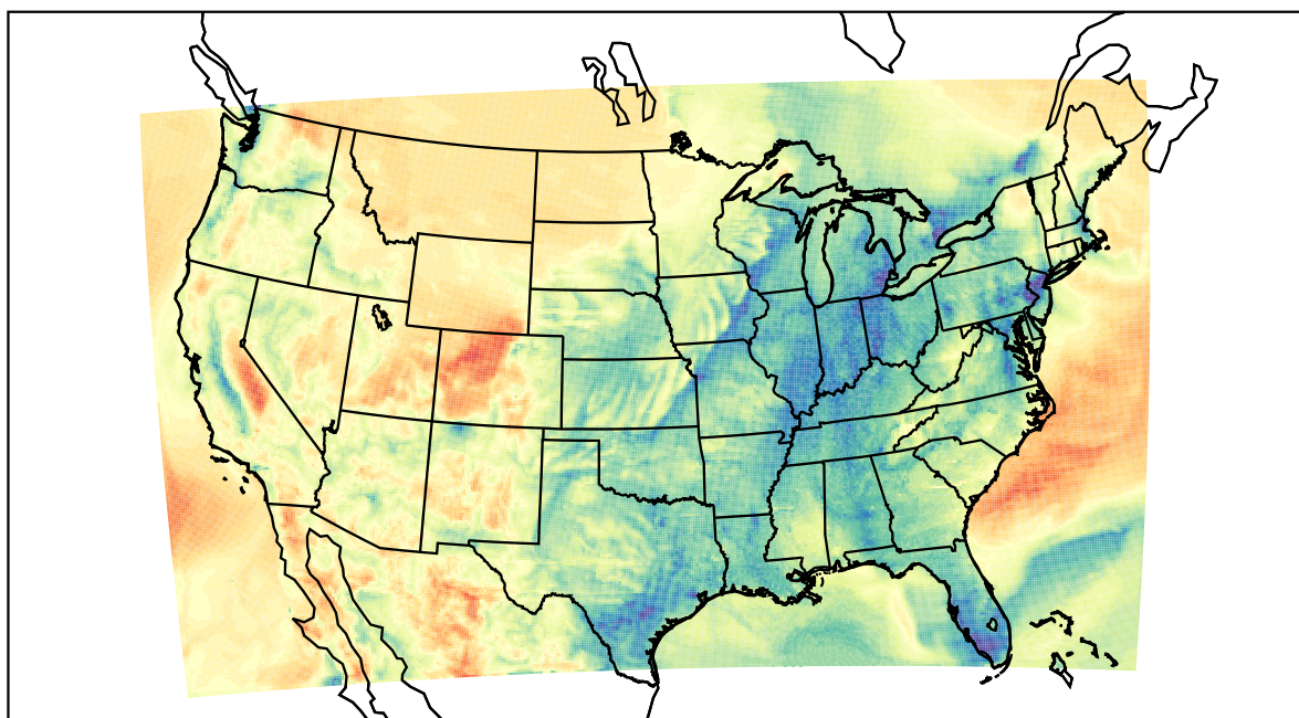
WRF (2021-03-30_11:00:00)
