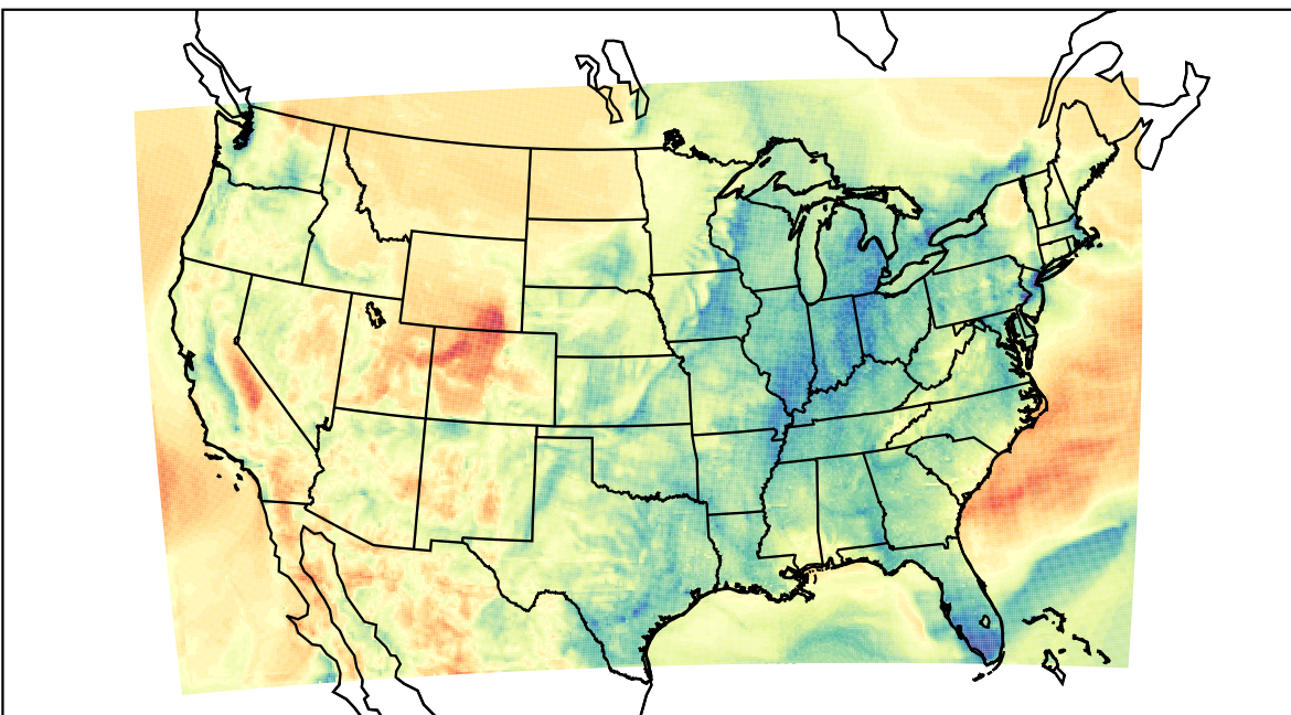
WRF (2021-03-30_08:00:00)
