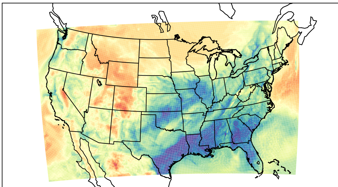
WRF (2021-03-31_13:00:00)
