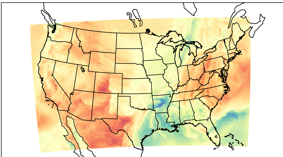
WRF (2021-03-30_21:00:00)
