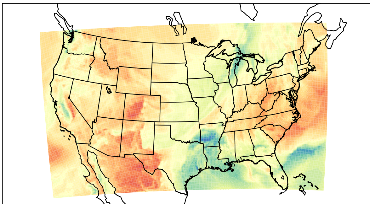
WRF (2021-03-30_18:00:00)
