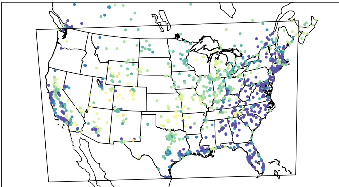
AirNOW (2021-03-30_10:00:00)
