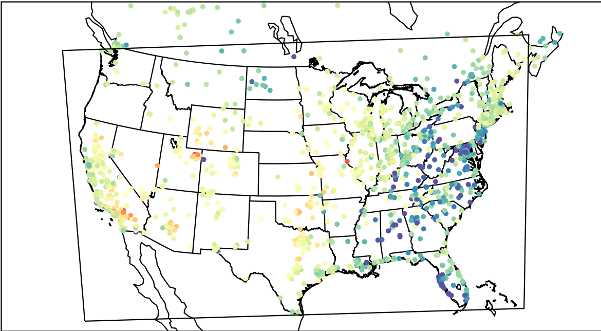
AirNOW (2021-03-30_01:00:00)
