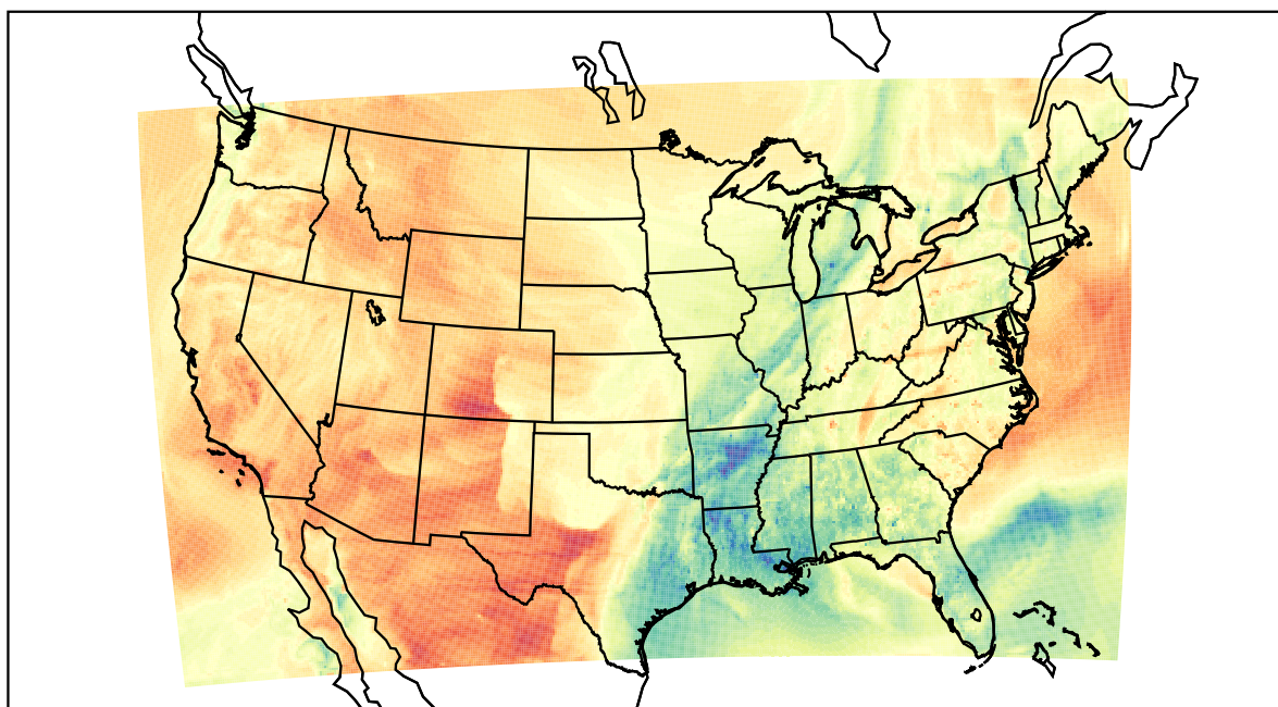
WRF (2021-03-30_23:00:00)
