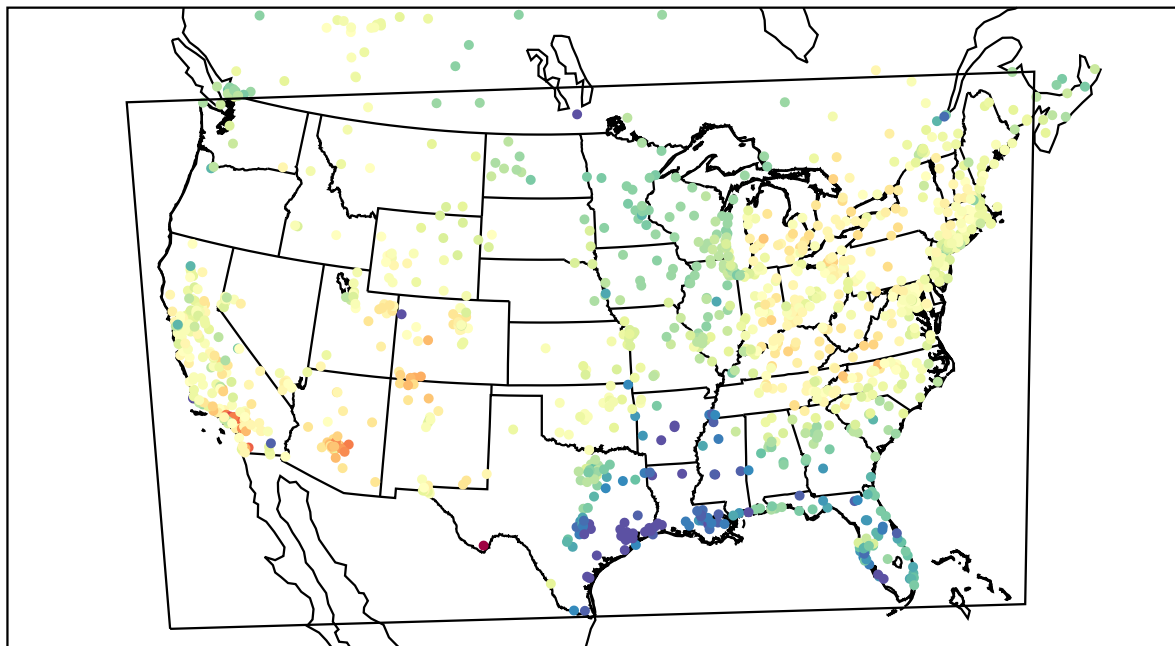
AirNOW (2021-03-30_23:00:00)
