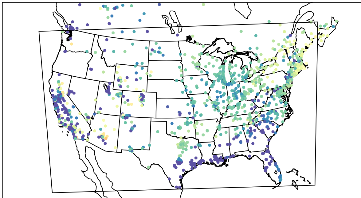
AirNOW (2021-03-31_13:00:00)
