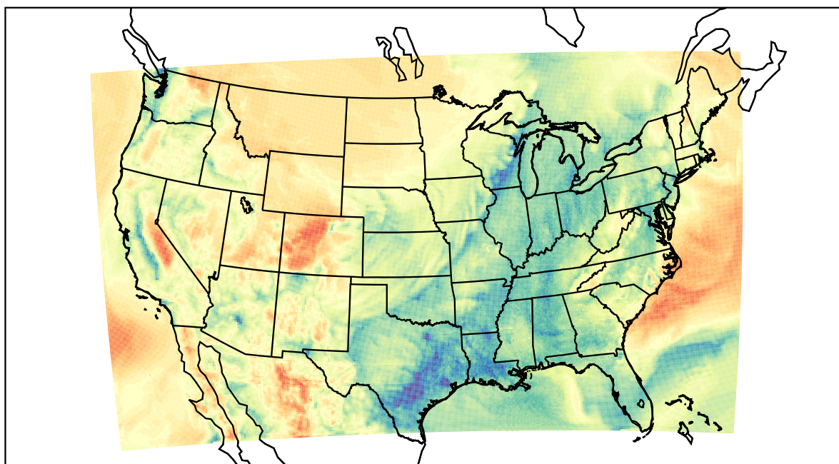
WRF (2021-03-30_14:00:00)
