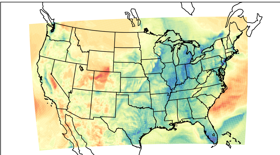
WRF (2021-03-30_09:00:00)
