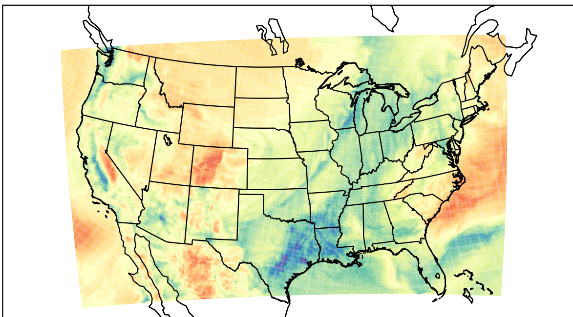
WRF (2021-03-30_15:00:00)
