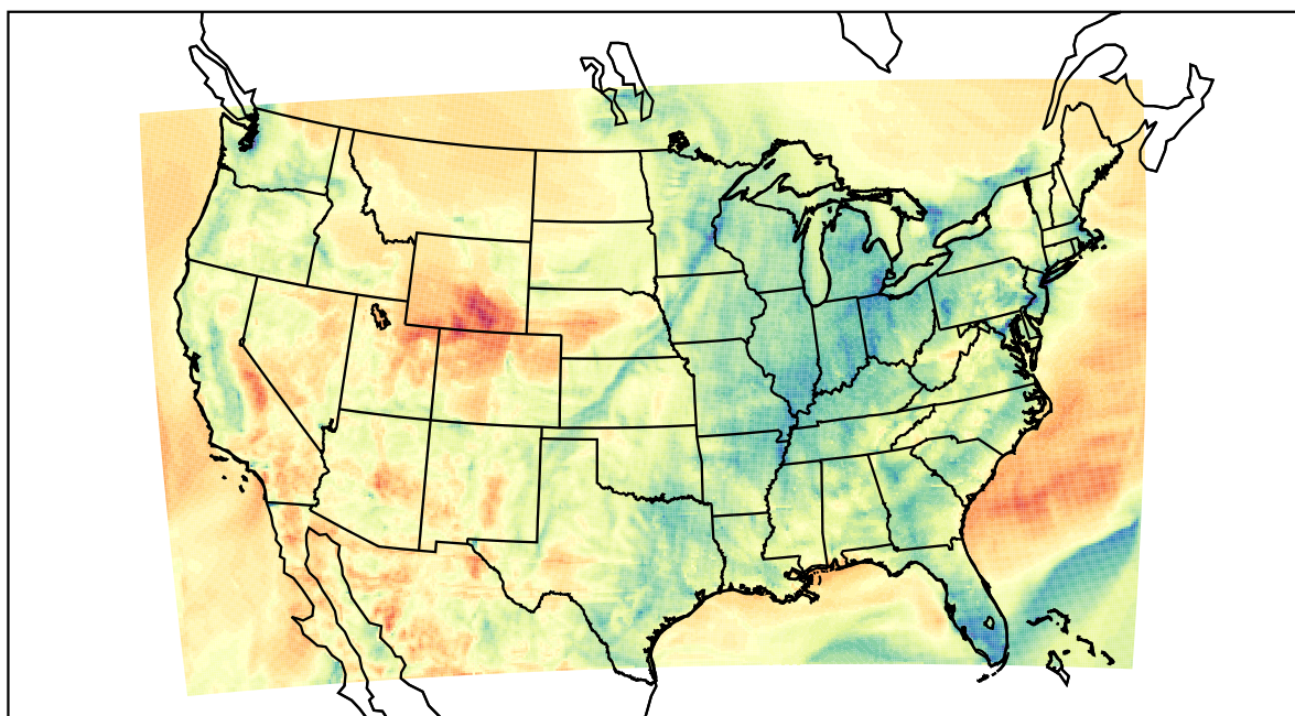
WRF (2021-03-30_04:00:00)
