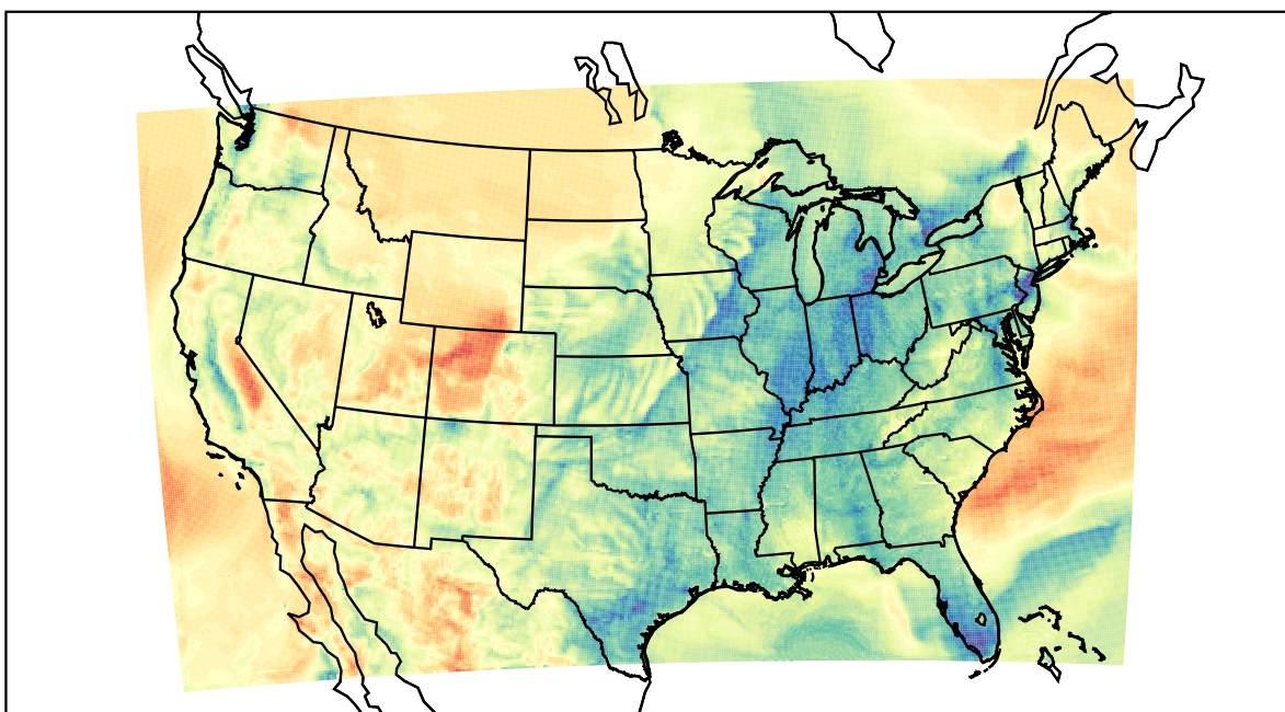
WRF (2021-03-30_10:00:00)
