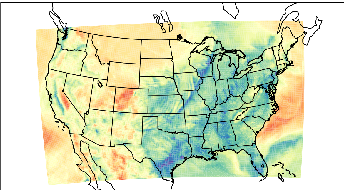
WRF (2021-03-30_13:00:00)
