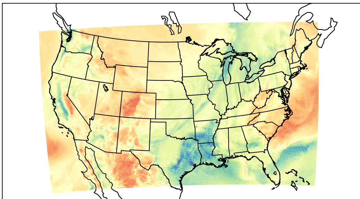
WRF (2021-03-30_16:00:00)
