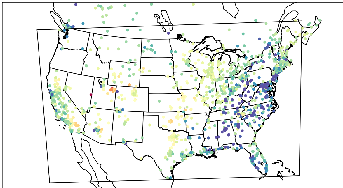
AirNOW (2021-03-30_03:00:00)
