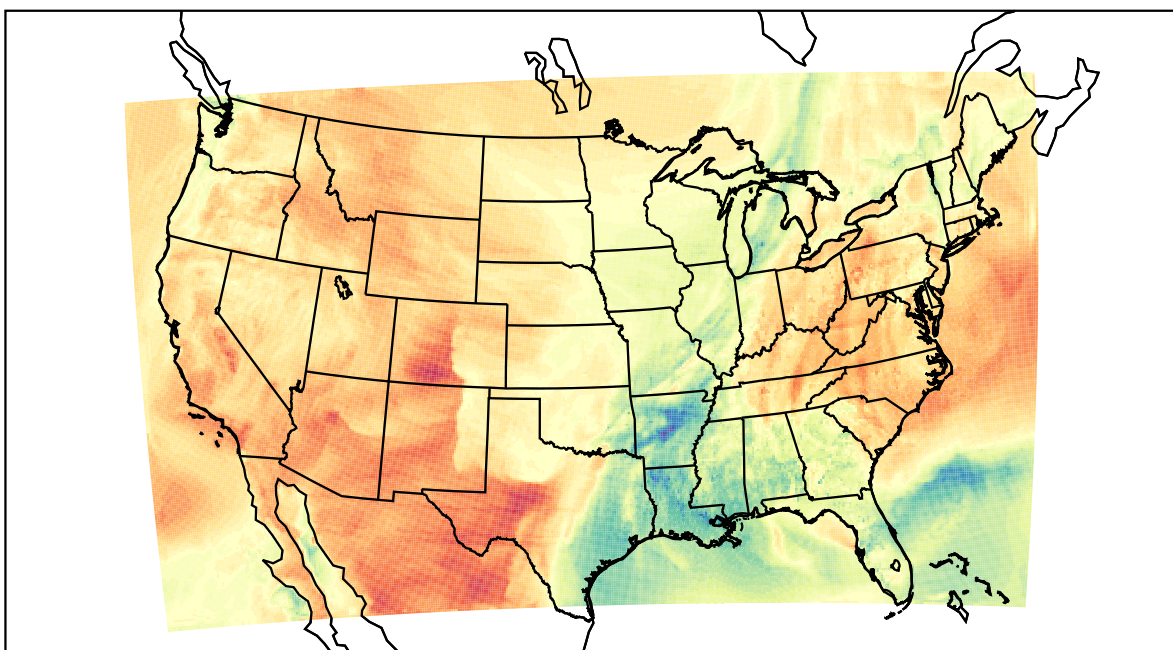
WRF (2021-03-30_22:00:00)
