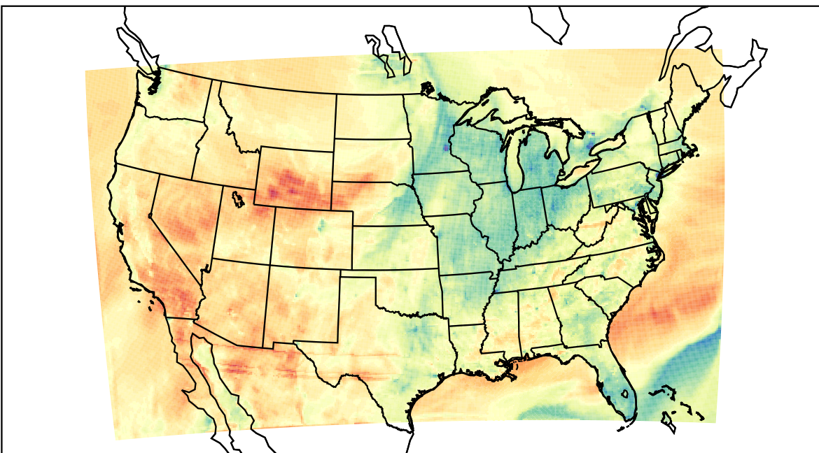
WRF (2021-03-30_01:00:00)
