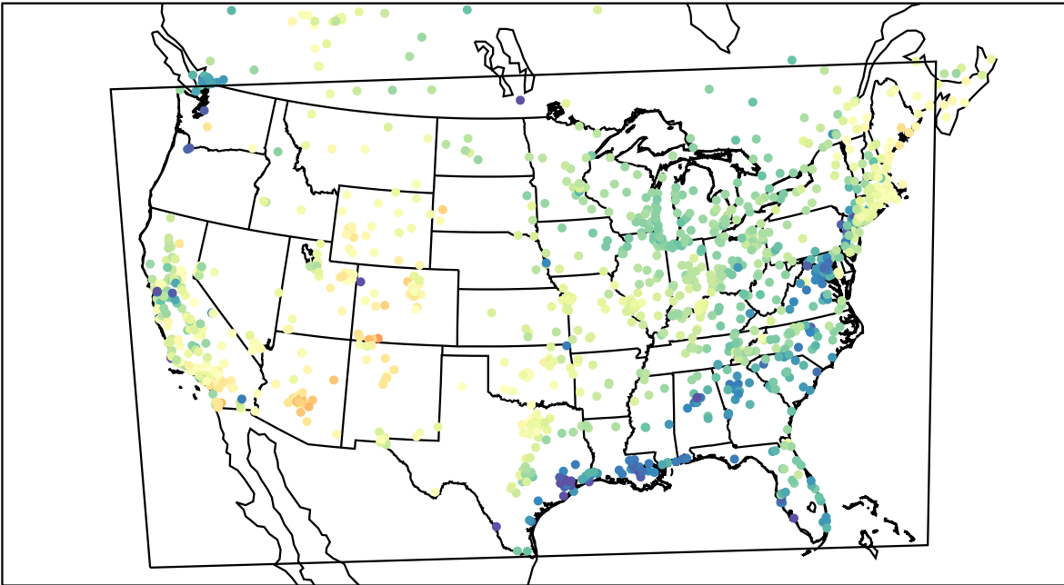
AirNOW (2021-03-31_18:00:00)
