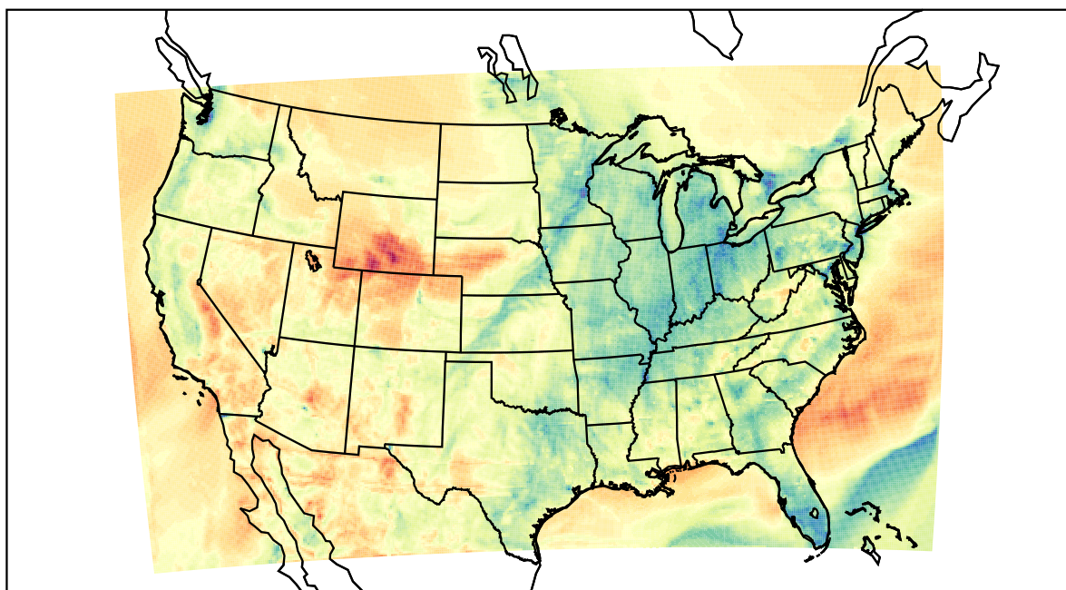
WRF (2021-03-30_03:00:00)
