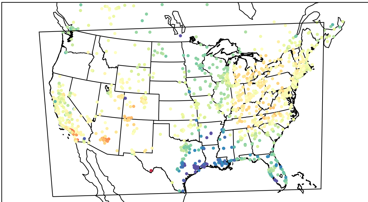
AirNOW (2021-03-30_22:00:00)
