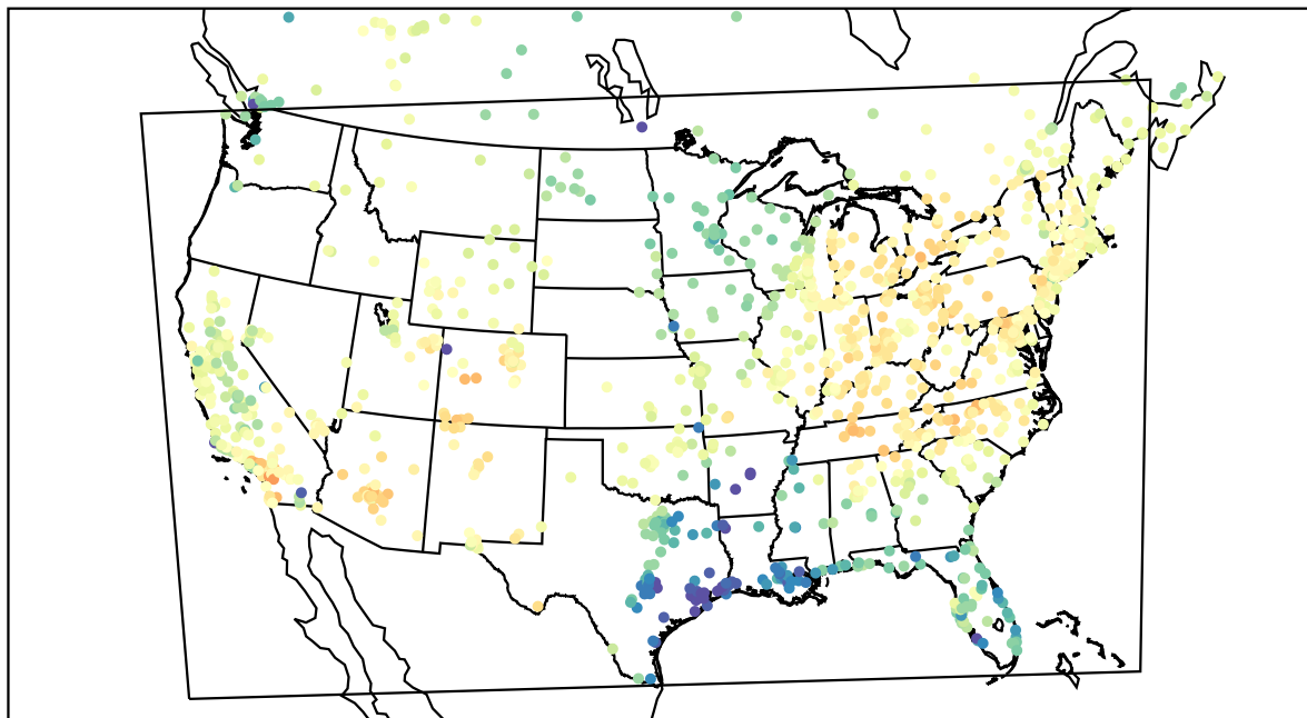
AirNOW (2021-03-30_20:00:00)
