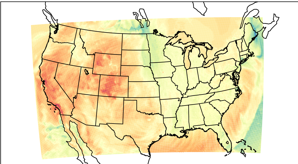
WRF (2021-04-01_23:00:00)
