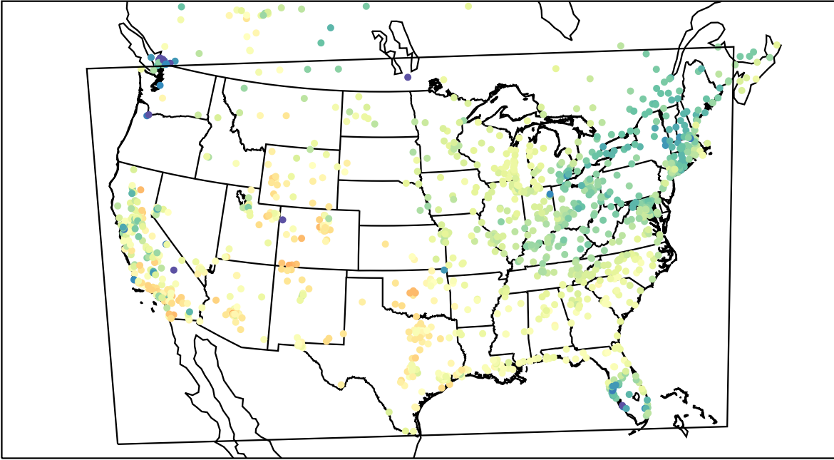
AirNOW (2021-04-01_18:00:00)
