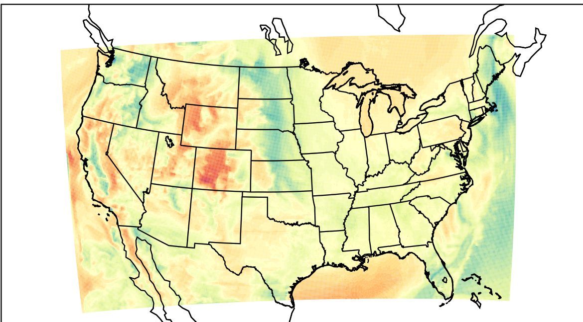
WRF (2021-04-01_17:00:00)
