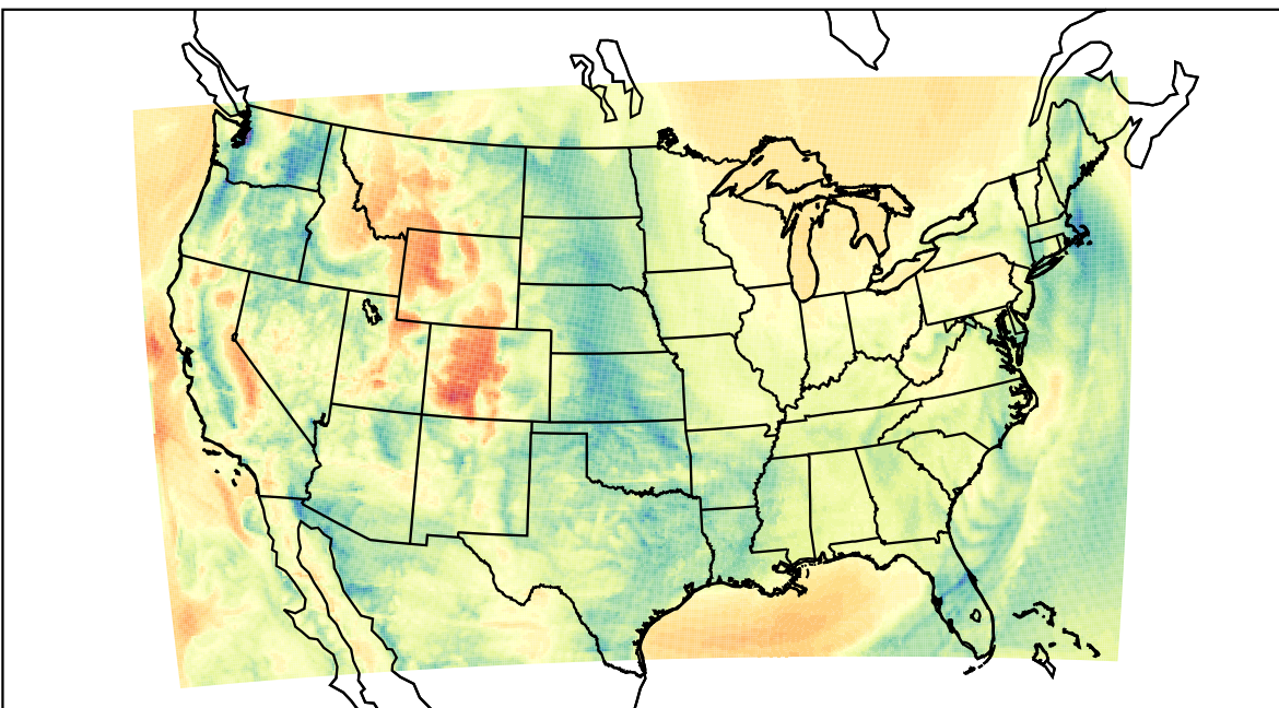
WRF (2021-04-01_15:00:00)
