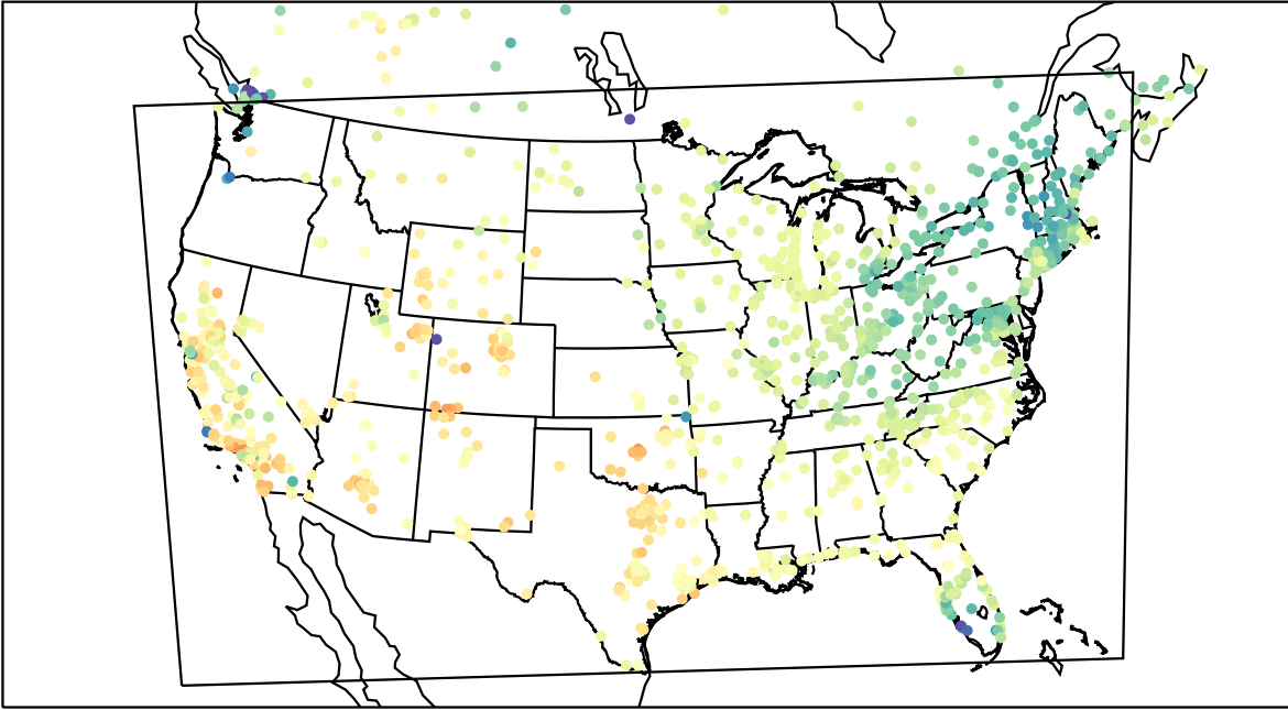
AirNOW (2021-04-01_19:00:00)
