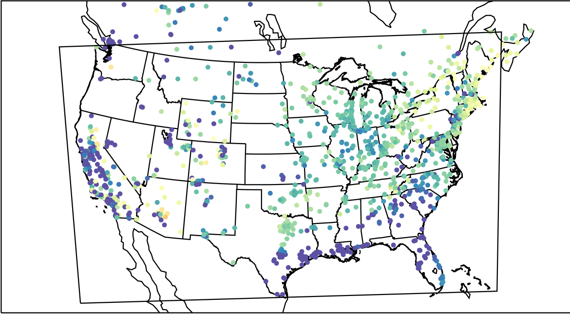
AirNOW (2021-03-31_13:00:00)
