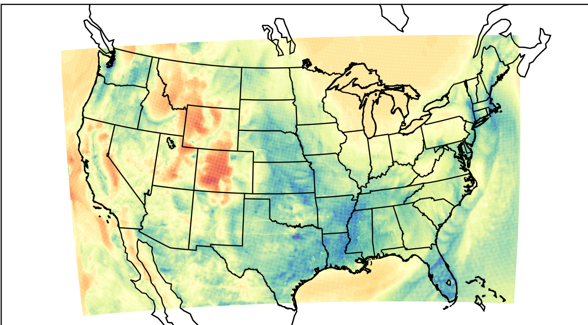
WRF (2021-04-01_13:00:00)
