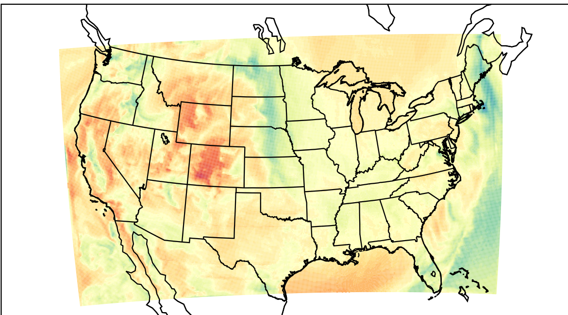
WRF (2021-04-01_18:00:00)
