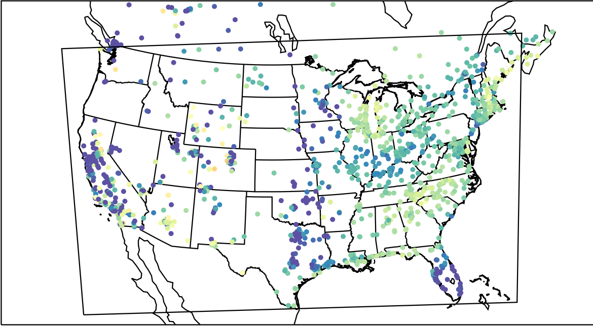
AirNOW (2021-04-01_13:00:00)
