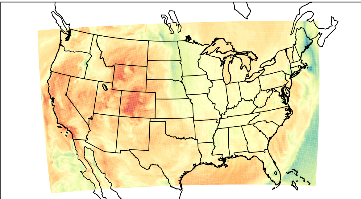
WRF (2021-04-01_20:00:00)
