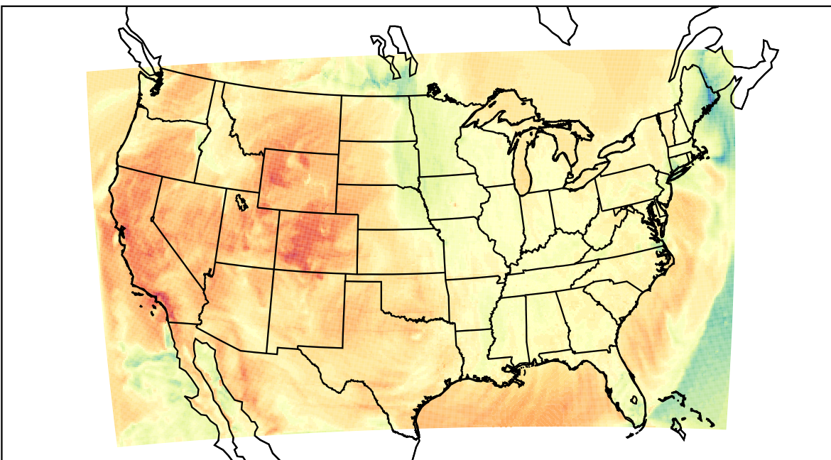
WRF (2021-04-01_22:00:00)
