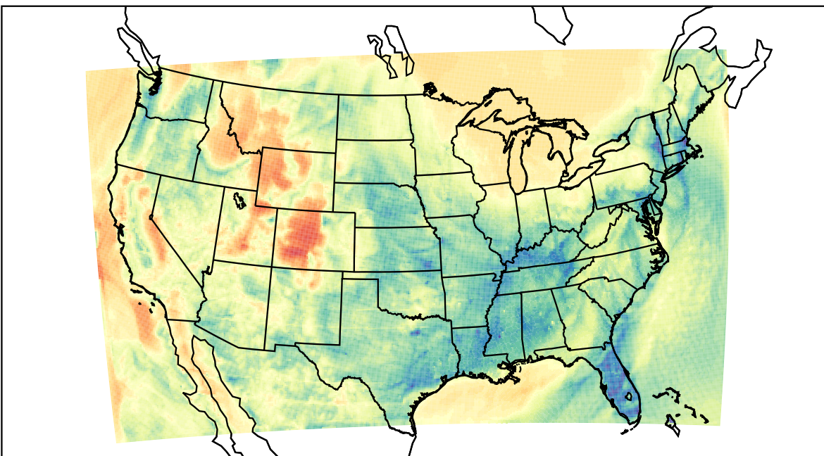
WRF (2021-04-01_11:00:00)
