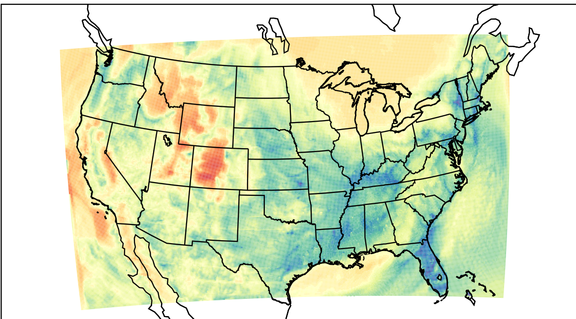
WRF (2021-04-01_10:00:00)
