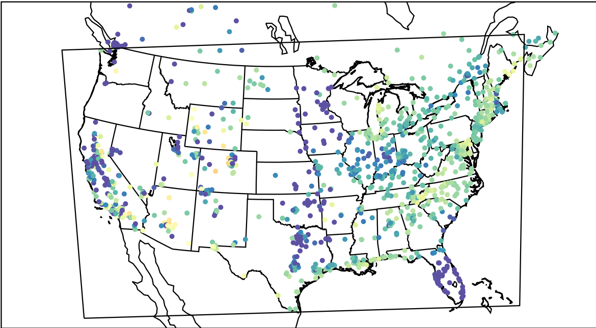
AirNOW (2021-04-01_10:00:00)
