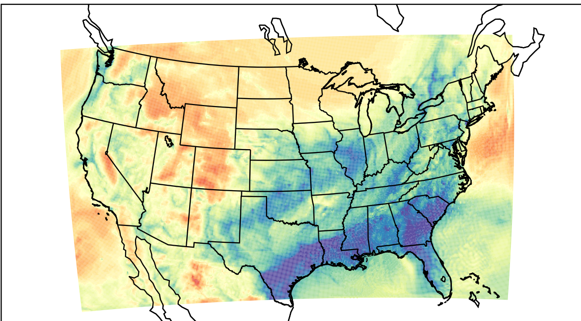
WRF (2021-03-31_13:00:00)
