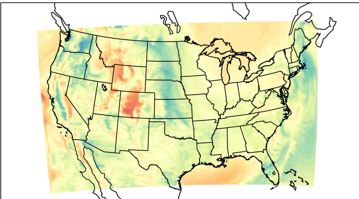
WRF (2021-04-01_16:00:00)
