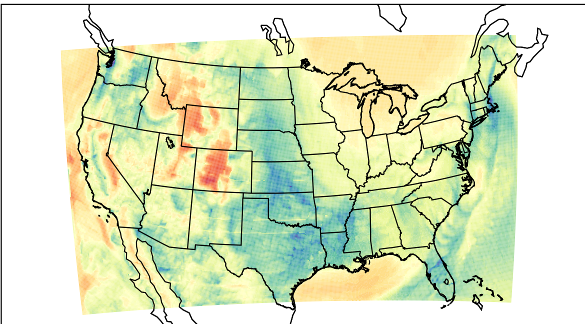
WRF (2021-04-01_14:00:00)
