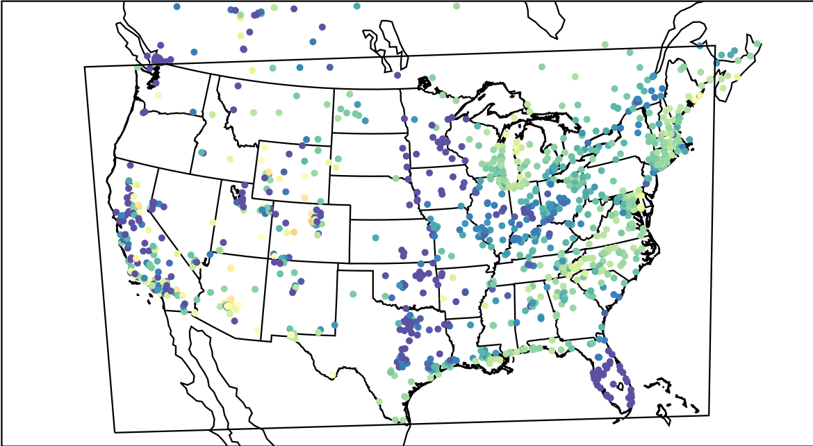
AirNOW (2021-04-01_11:00:00)
