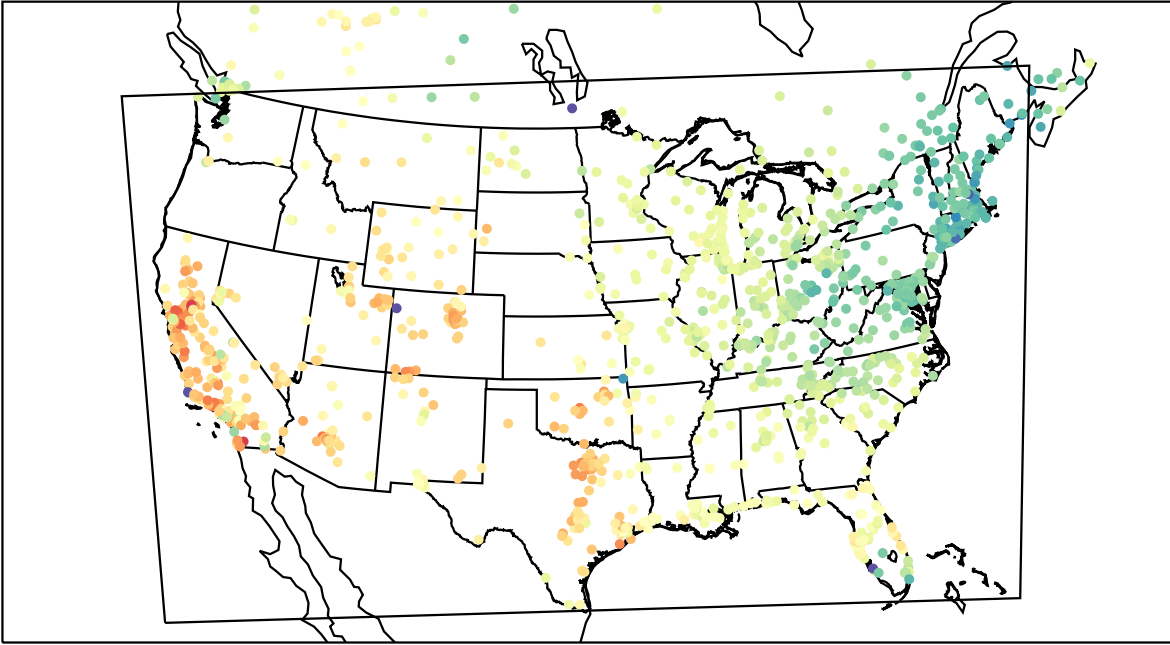
AirNOW (2021-04-01_23:00:00)
