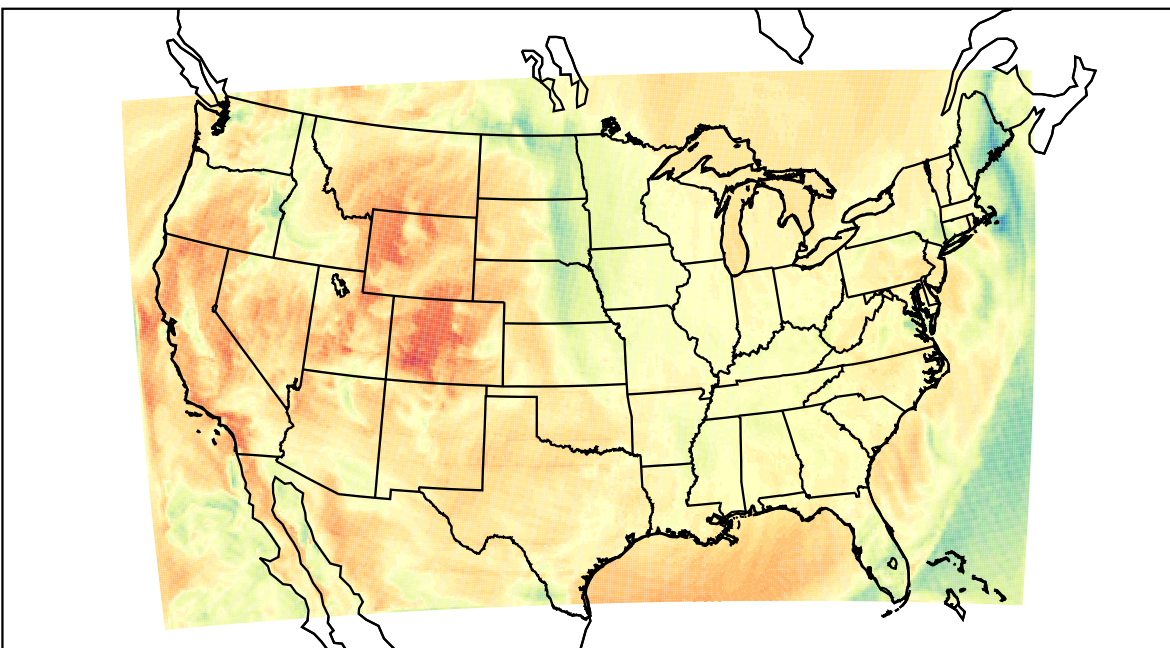
WRF (2021-04-01_19:00:00)
