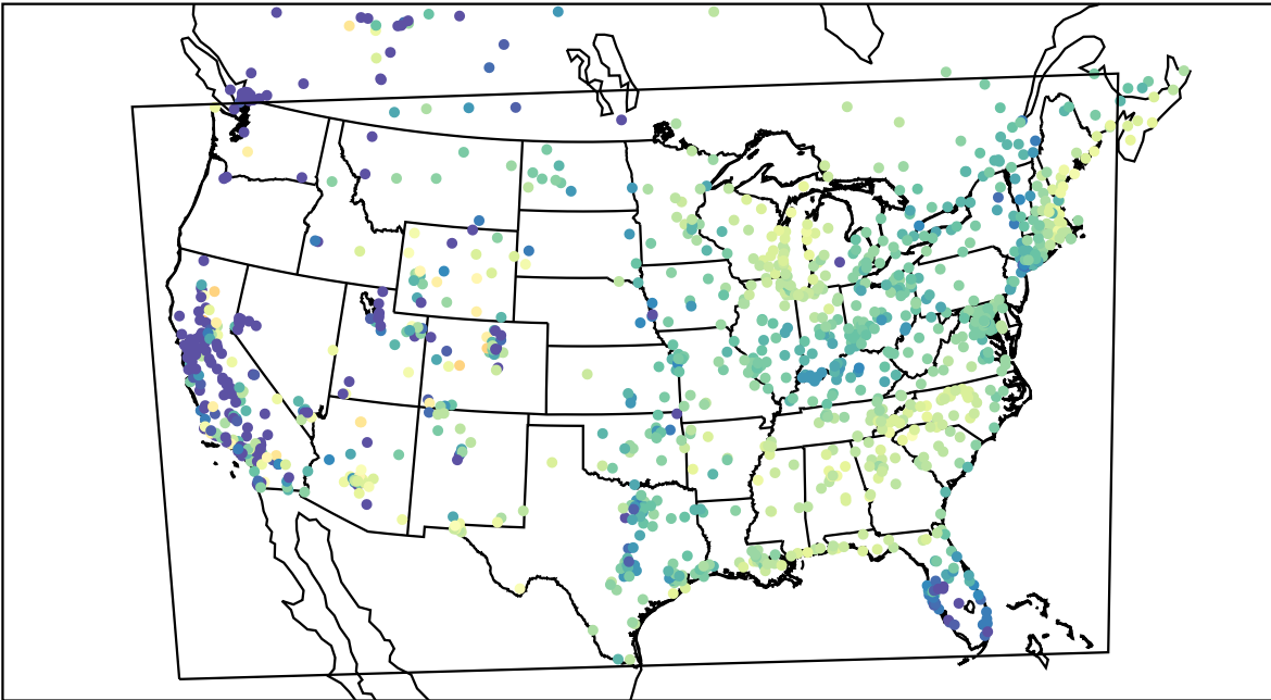
AirNOW (2021-04-01_14:00:00)
