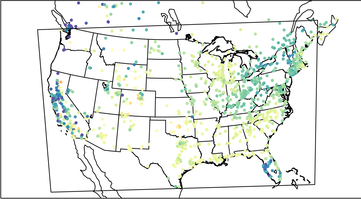
AirNOW (2021-04-01_16:00:00)
