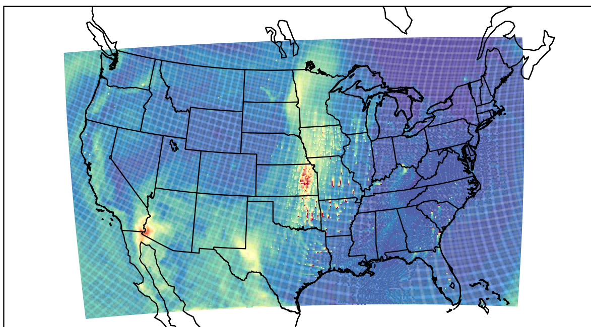
WRF 2021-04-02_20:00:00
