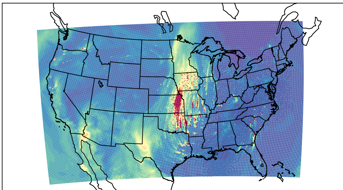
WRF 2021-04-02_23:00:00
