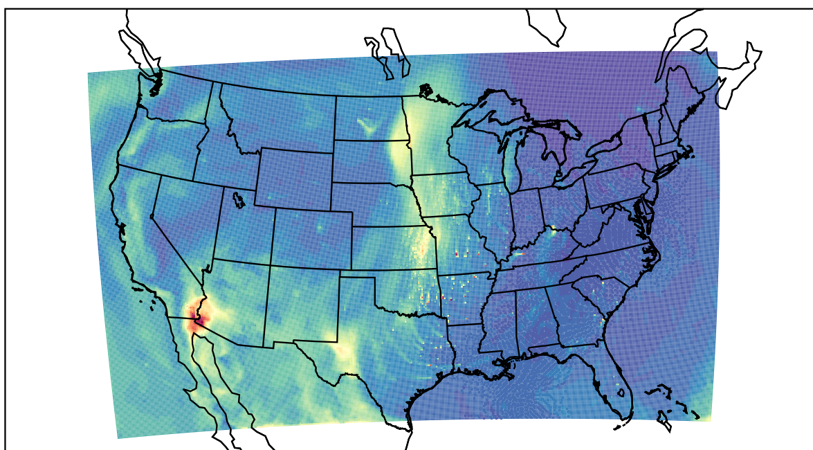
WRF 2021-04-02_18:00:00
