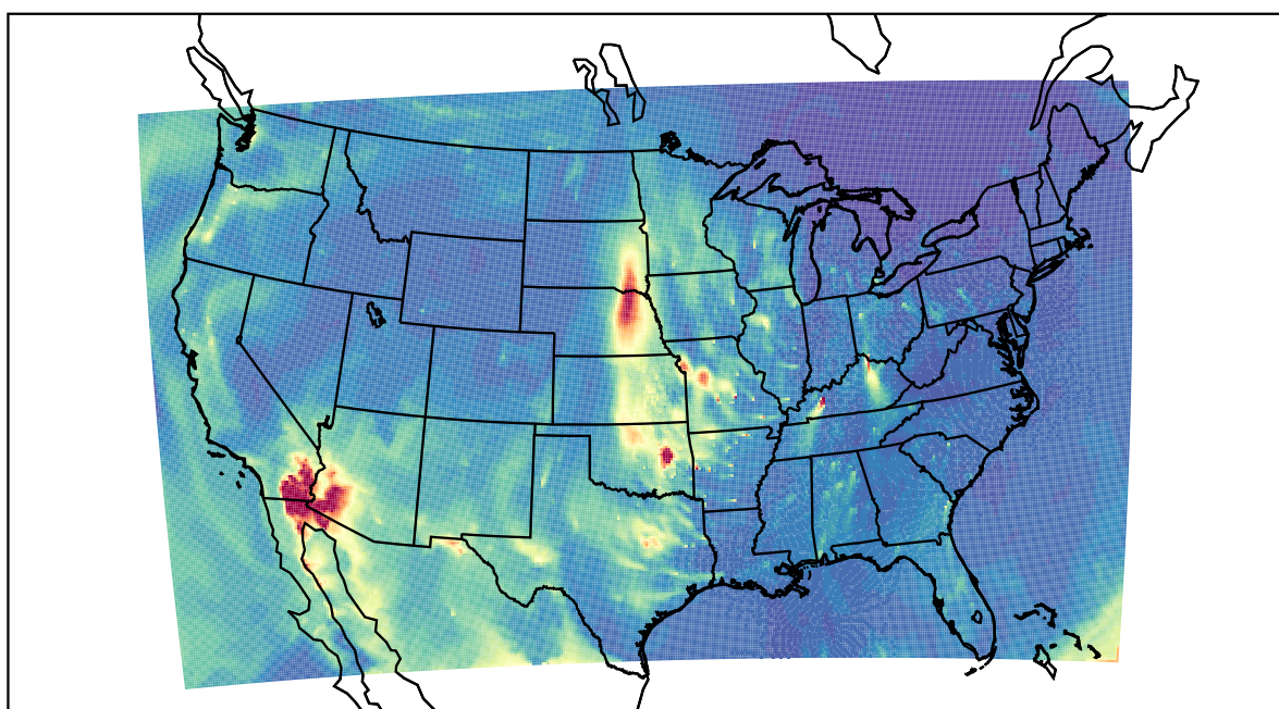
WRF 2021-04-02_11:00:00
