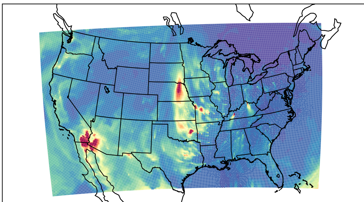
WRF 2021-04-02_10:00:00
