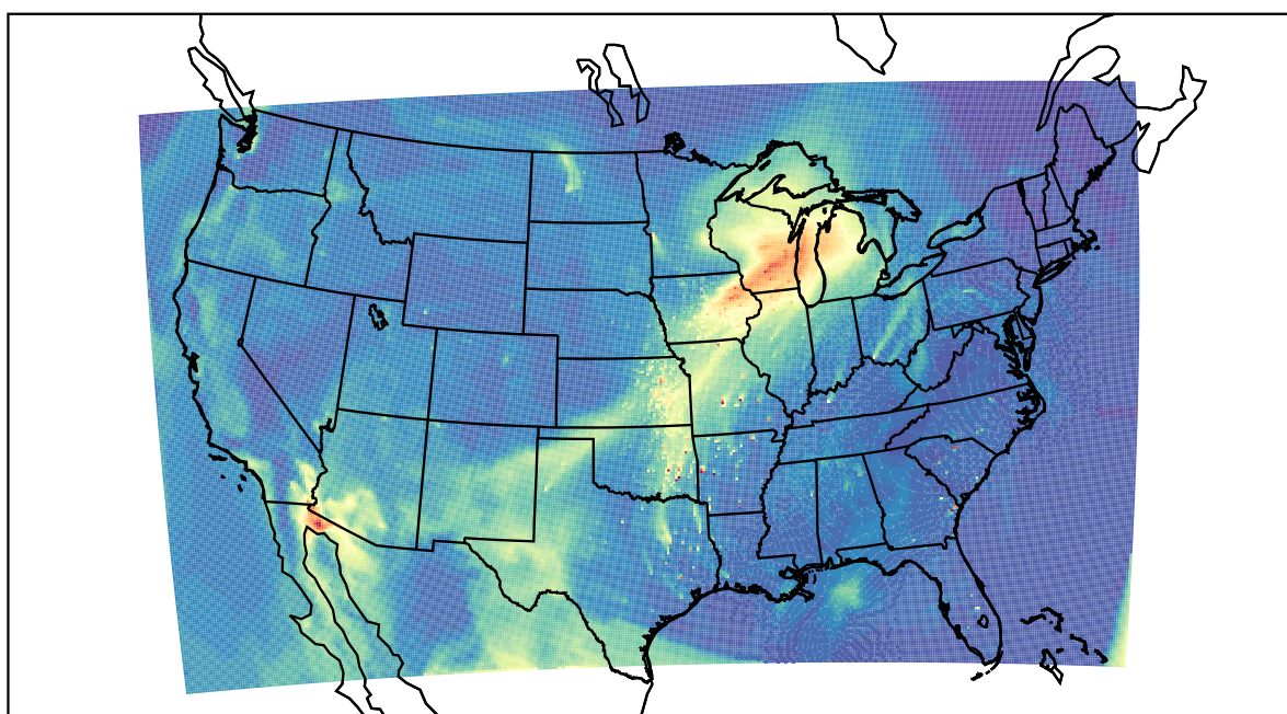
WRF 2021-04-03_18:00:00
