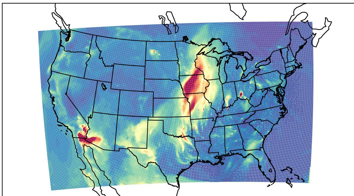
WRF 2021-04-03_10:00:00
