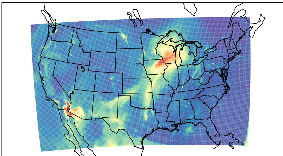
WRF 2021-04-03_16:00:00
