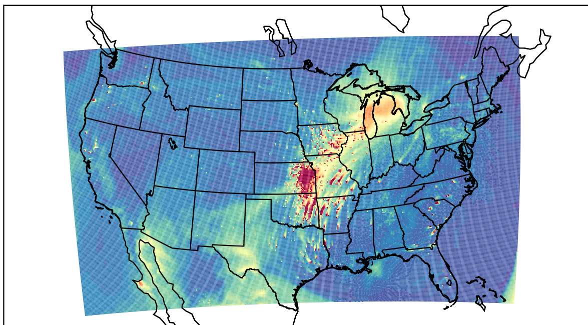
WRF 2021-04-03_23:00:00
