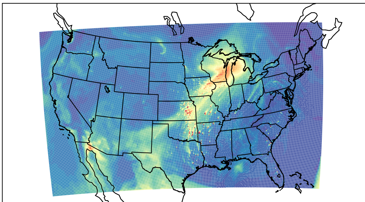
WRF 2021-04-03_19:00:00
