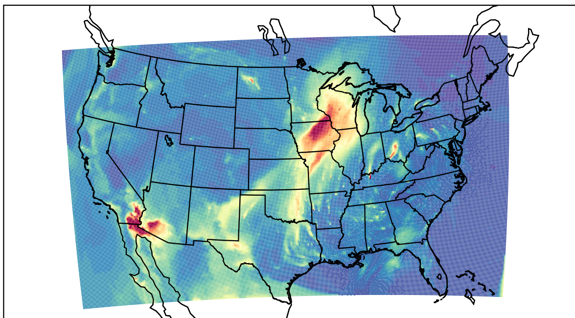
WRF 2021-04-03_13:00:00
