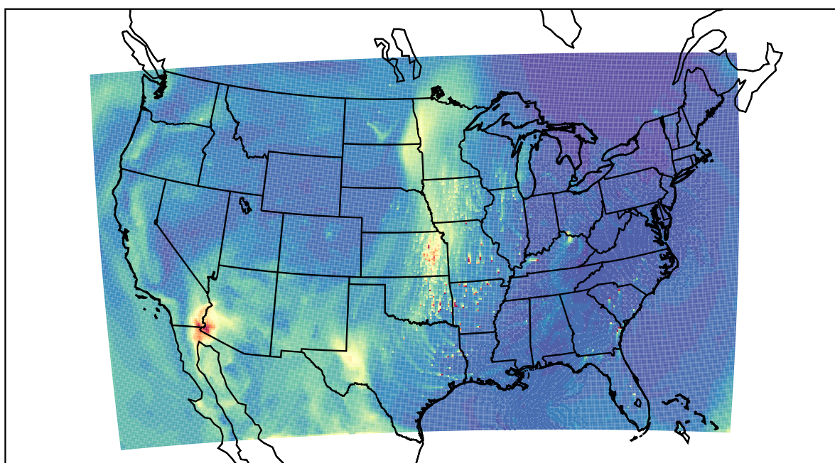
WRF 2021-04-02_19:00:00
