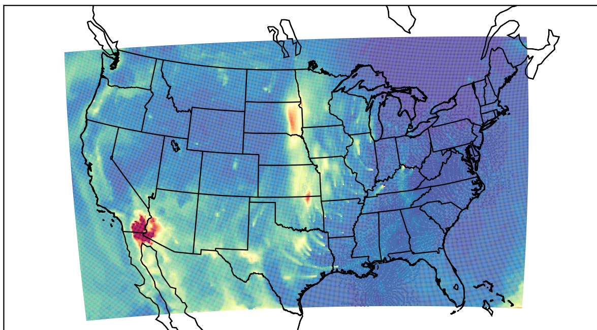
WRF 2021-04-02_14:00:00
