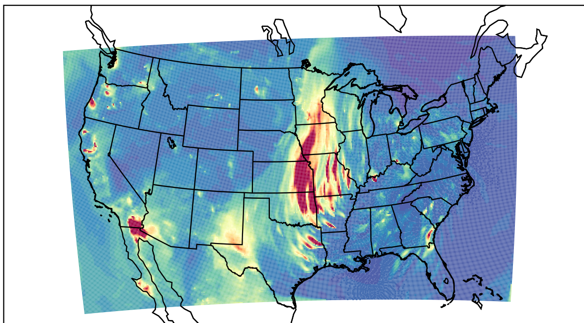
WRF 2021-04-03_04:00:00
