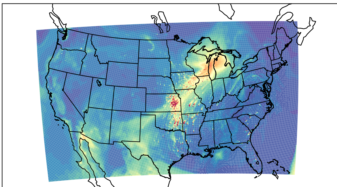
WRF 2021-04-03_20:00:00
