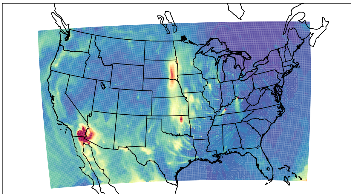
WRF 2021-04-02_13:00:00
