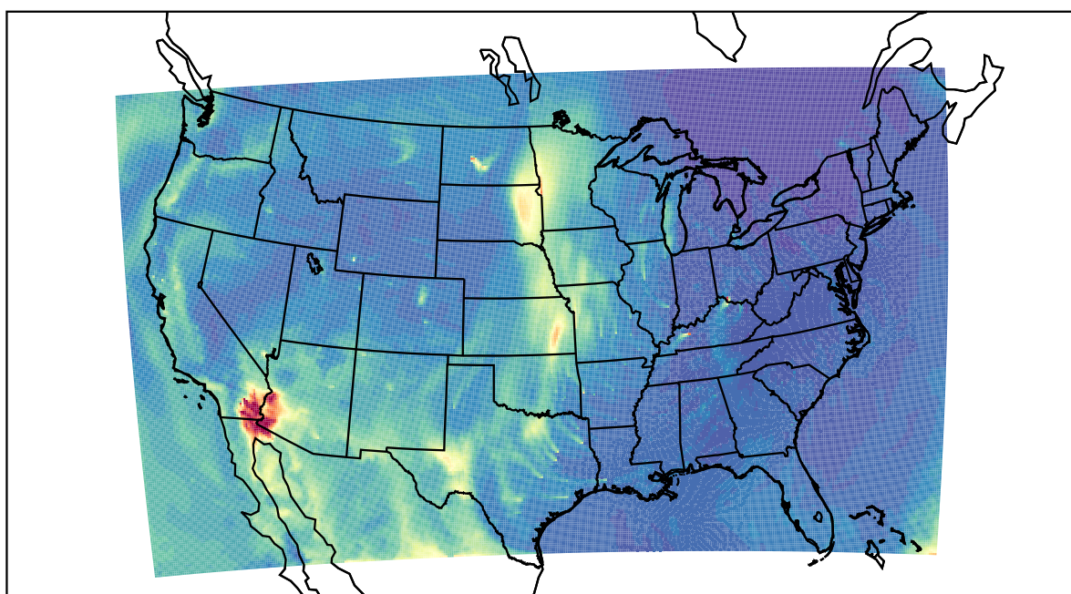
WRF 2021-04-02_16:00:00
