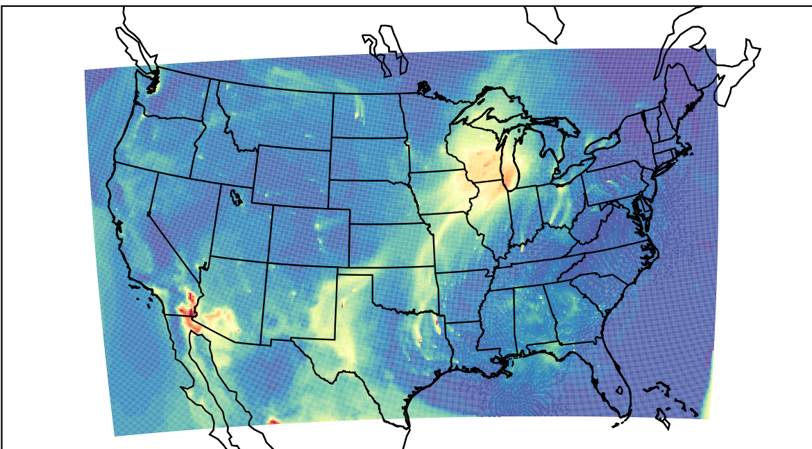
WRF 2021-04-03_16:00:00
