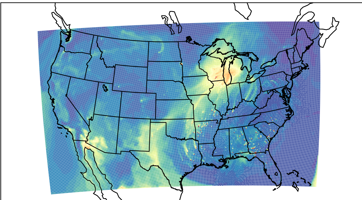
WRF 2021-04-03_18:00:00
