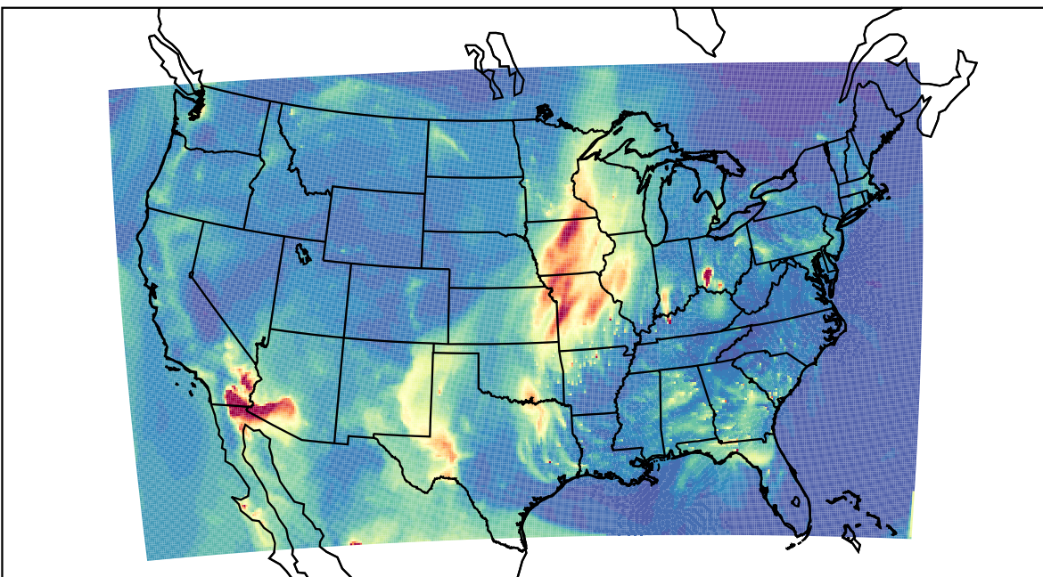
WRF 2021-04-03_10:00:00
