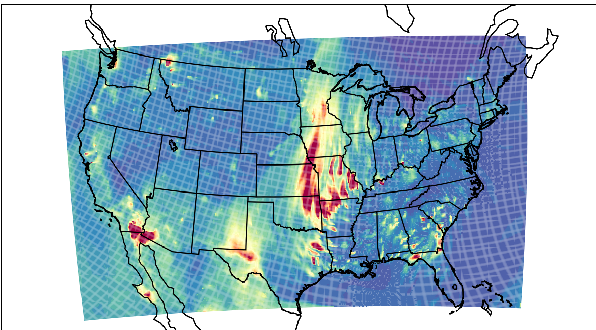
WRF 2021-04-03_04:00:00
