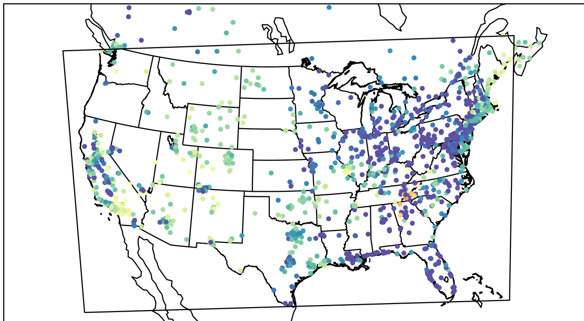
AirNOW (2021-04-13_10:00:00)
