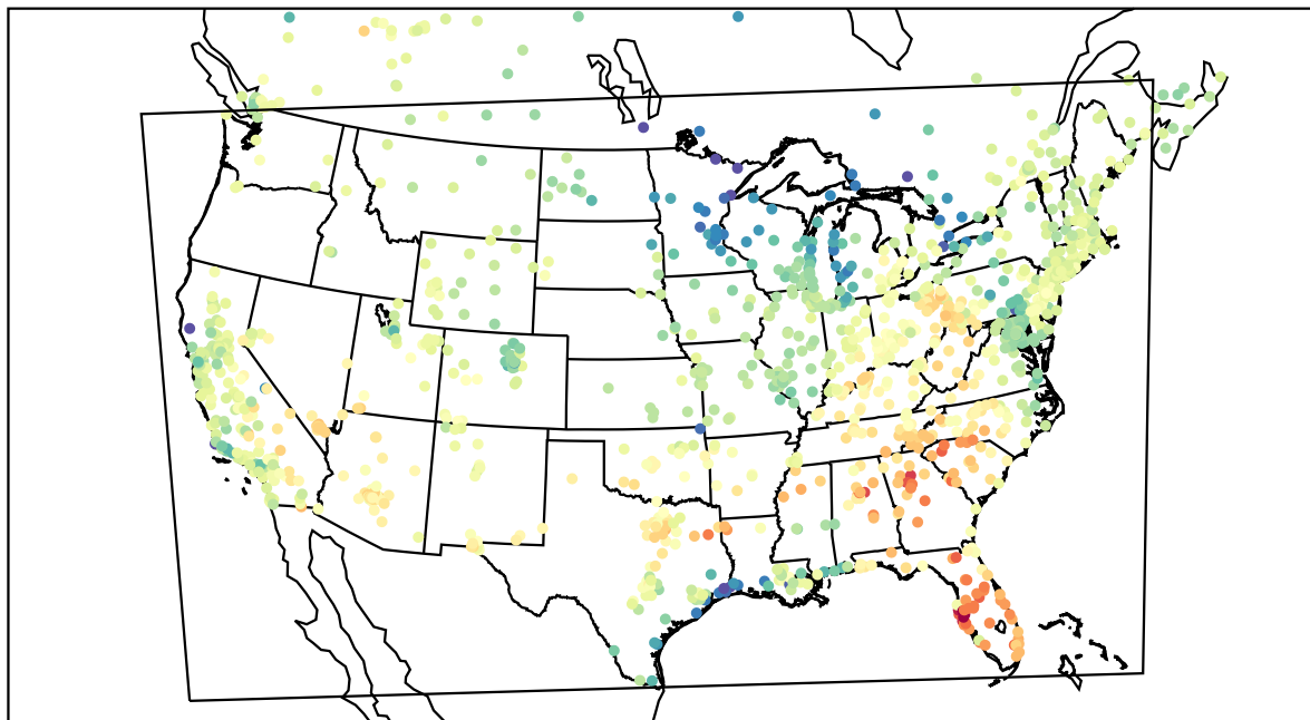
AirNOW (2021-04-13_19:00:00)
