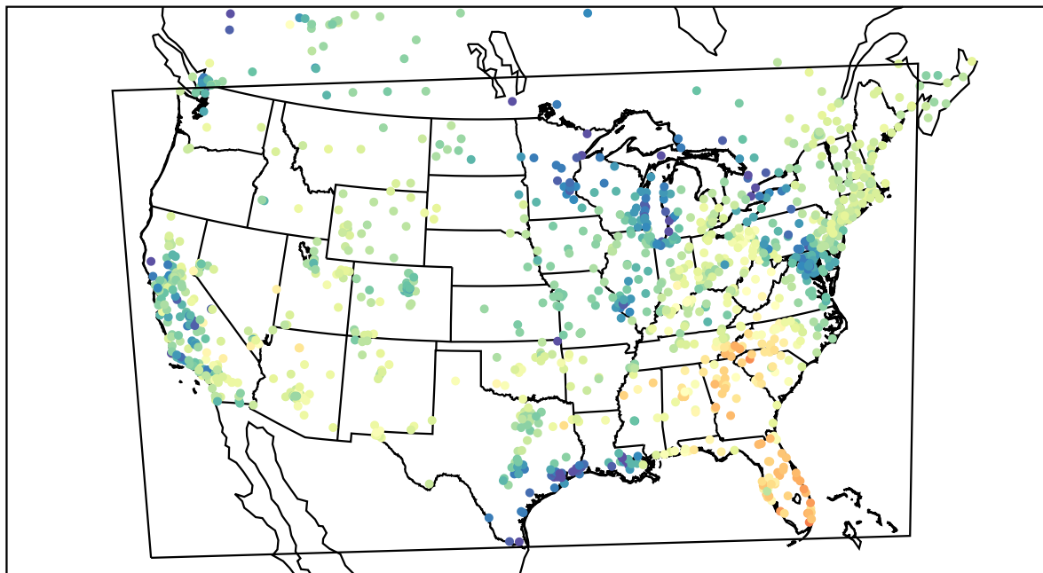
AirNOW (2021-04-13_16:00:00)
