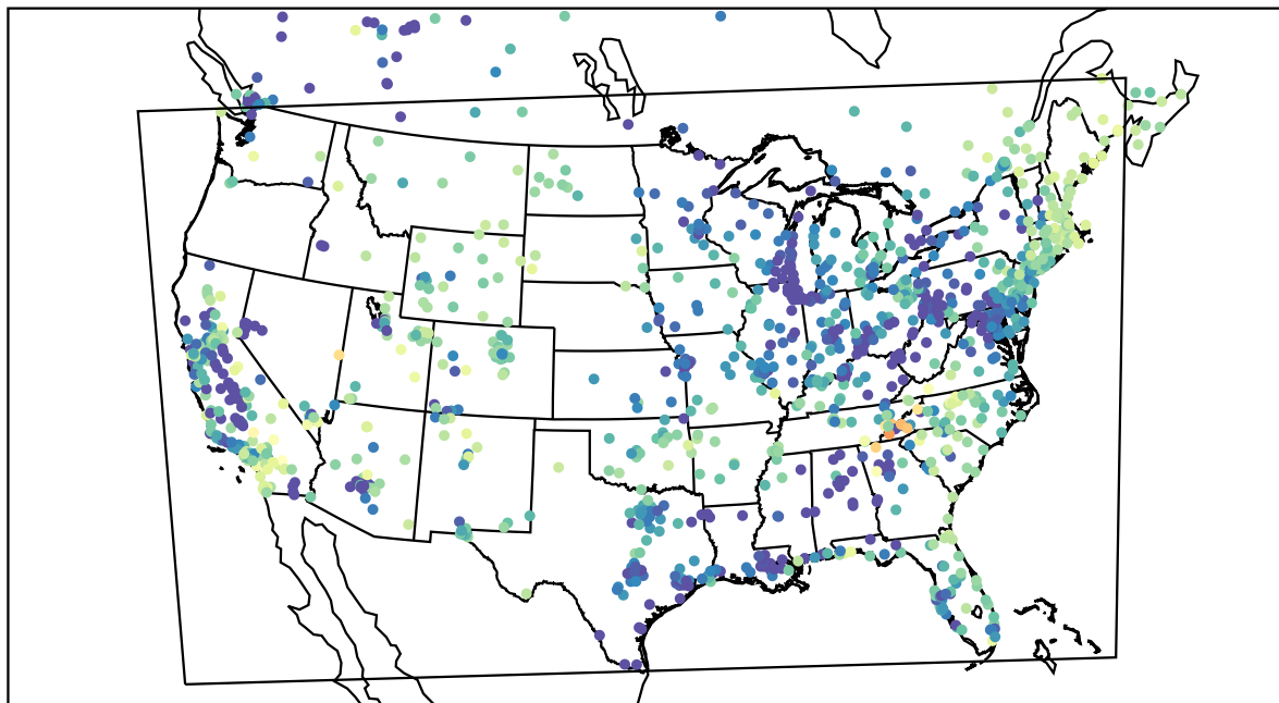
AirNOW (2021-04-13_13:00:00)
