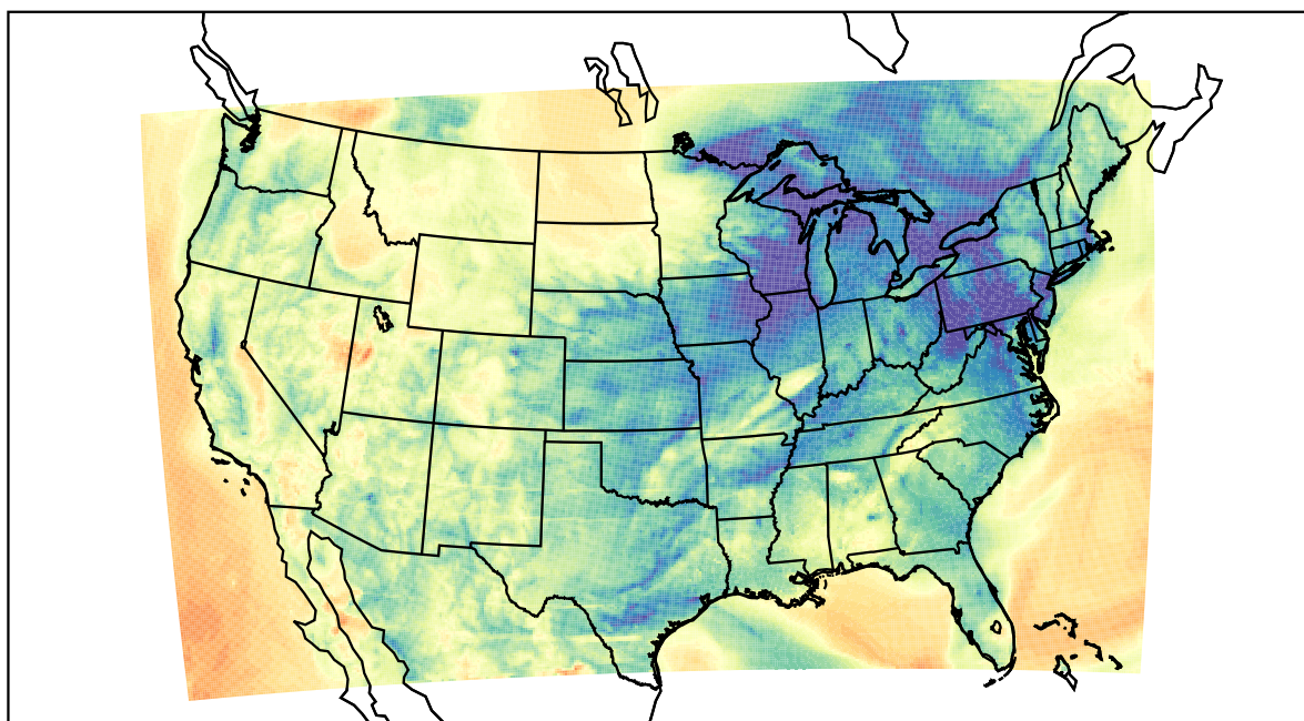
WRF (2021-04-13_10:00:00)
