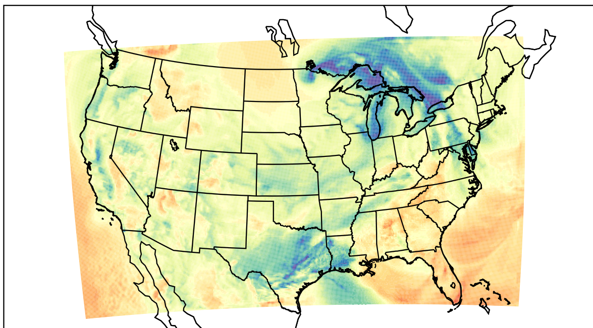
WRF (2021-04-13_16:00:00)
