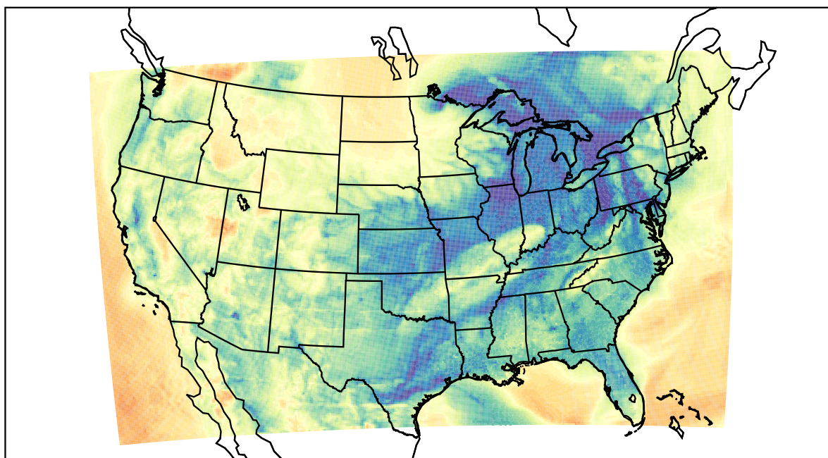
WRF (2021-04-13_13:00:00)
