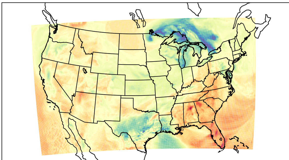
WRF (2021-04-13_18:00:00)
