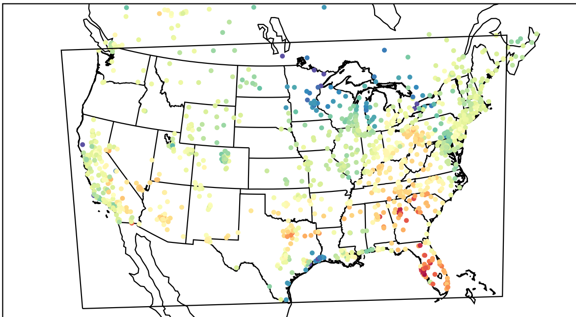
AirNOW (2021-04-13_20:00:00)
