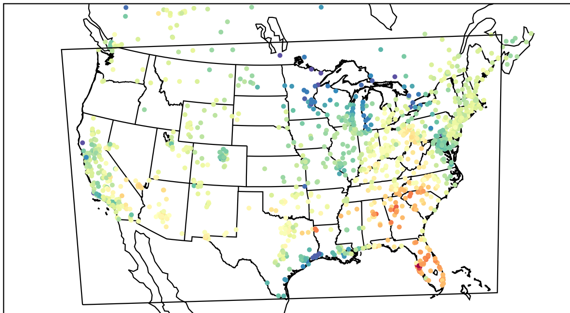
AirNOW (2021-04-13_18:00:00)
