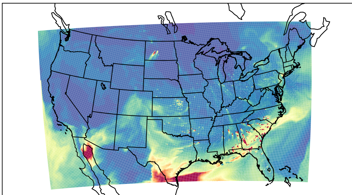
WRF 2021-04-15_20:00:00
