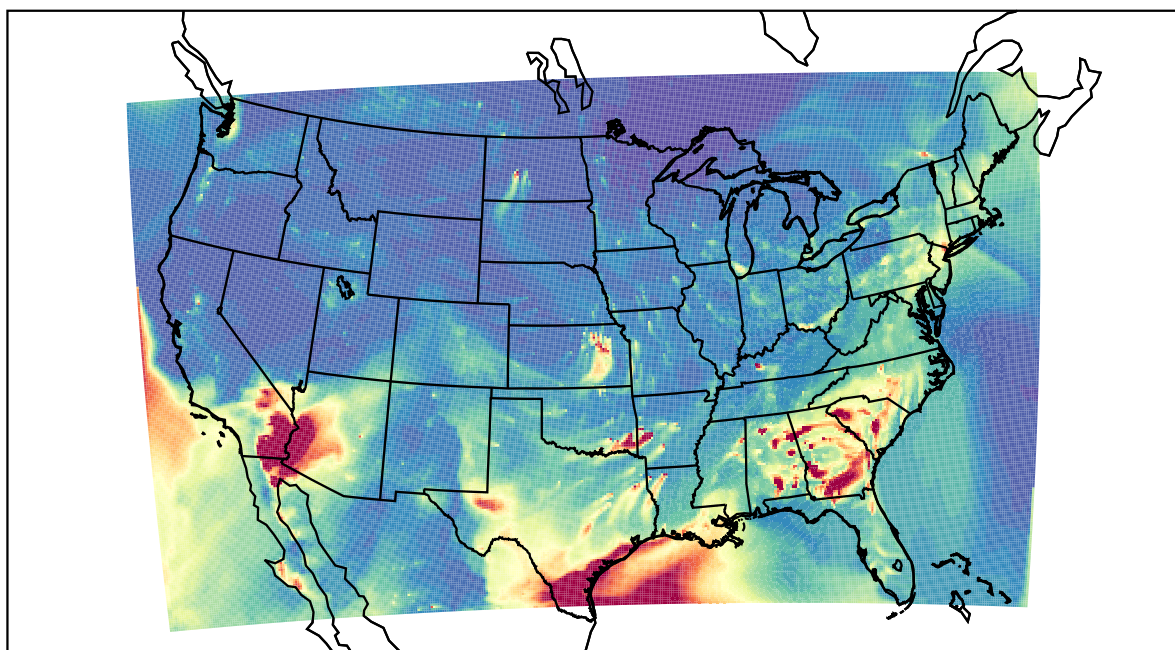
WRF 2021-04-15_03:00:00
