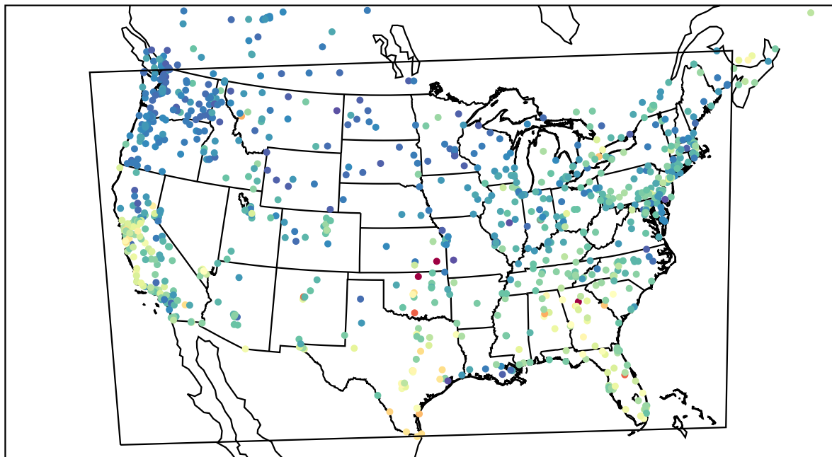
AirNOW
