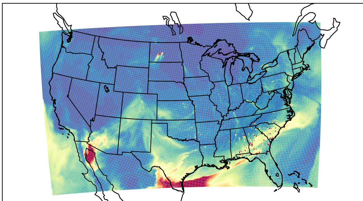
WRF 2021-04-15_18:00:00
