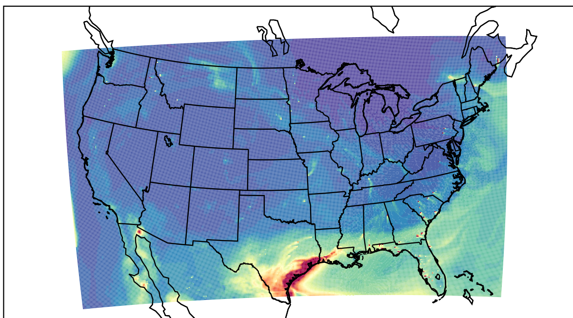
WRF 2021-04-30_20:00:00
