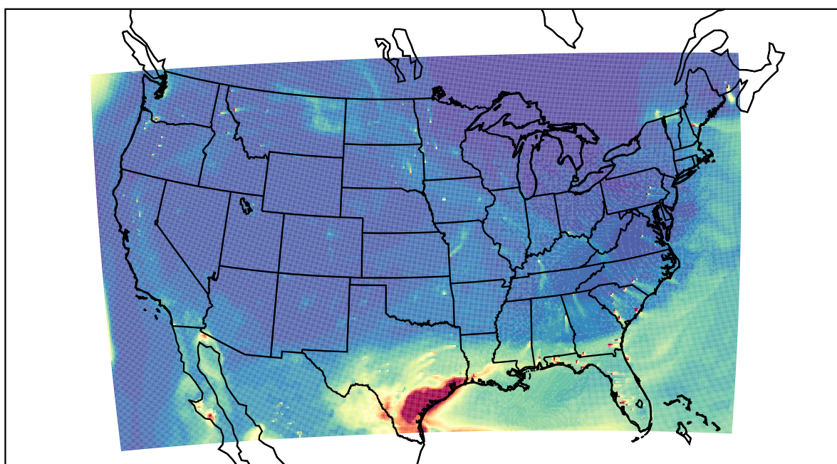
WRF 2021-04-30_22:00:00
