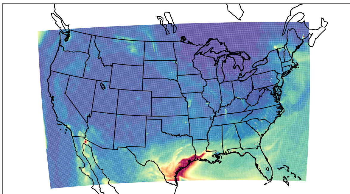
WRF 2021-04-30_18:00:00
