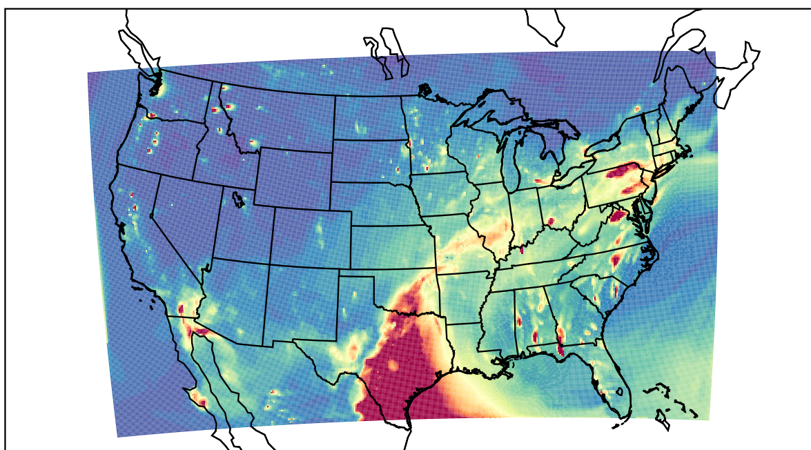
WRF 2021-04-29_03:00:00
