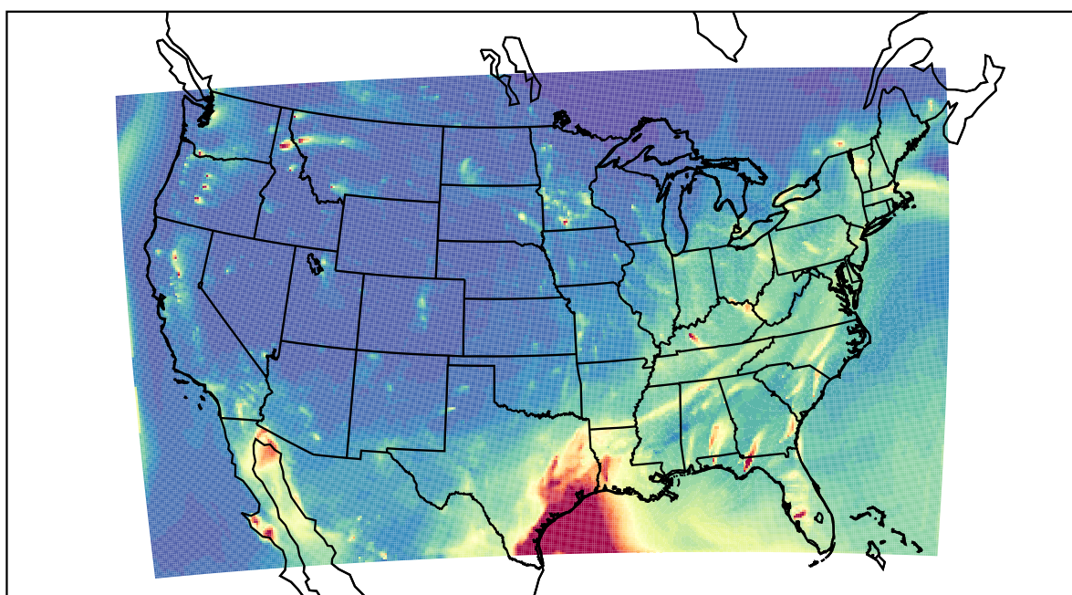
WRF 2021-04-30_04:00:00
