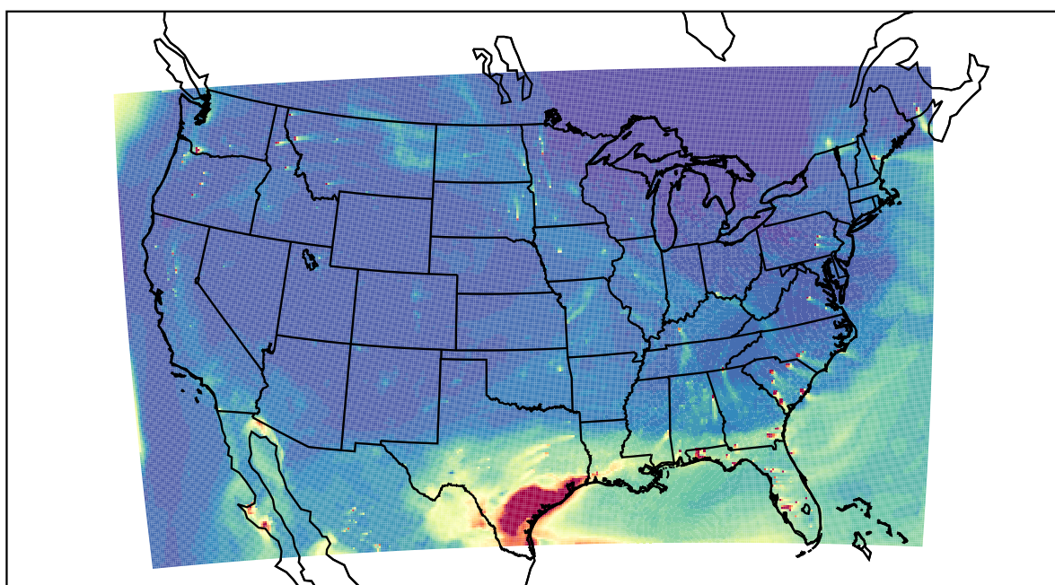
WRF 2021-04-30_23:00:00
