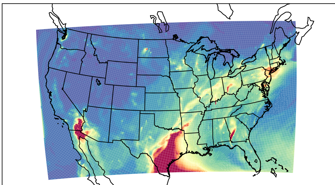
WRF 2021-04-29_10:00:00
