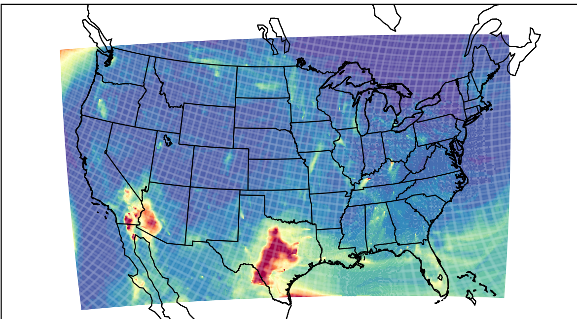
WRF 2021-05-01_07:00:00
