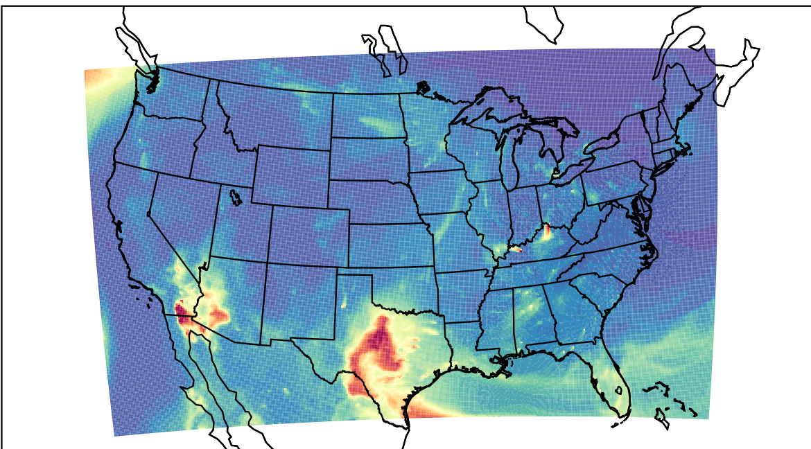
WRF 2021-05-01_11:00:00
