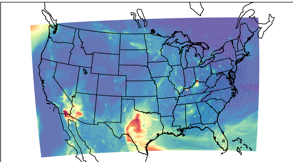
WRF 2021-05-01_12:00:00
