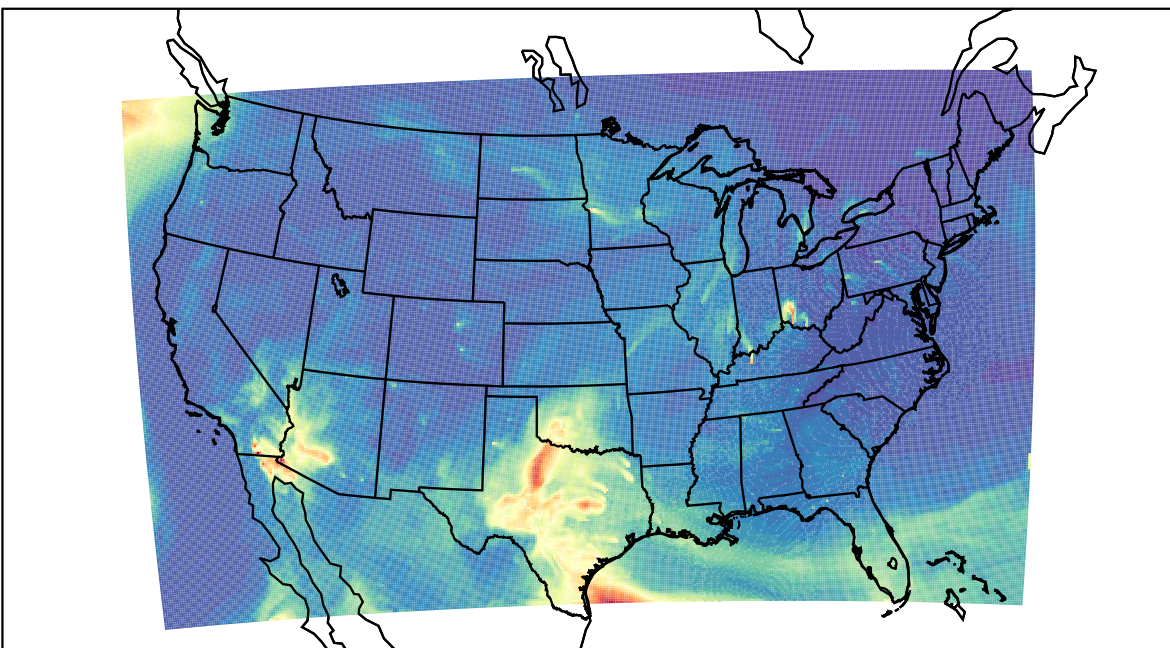
WRF 2021-05-01_16:00:00
