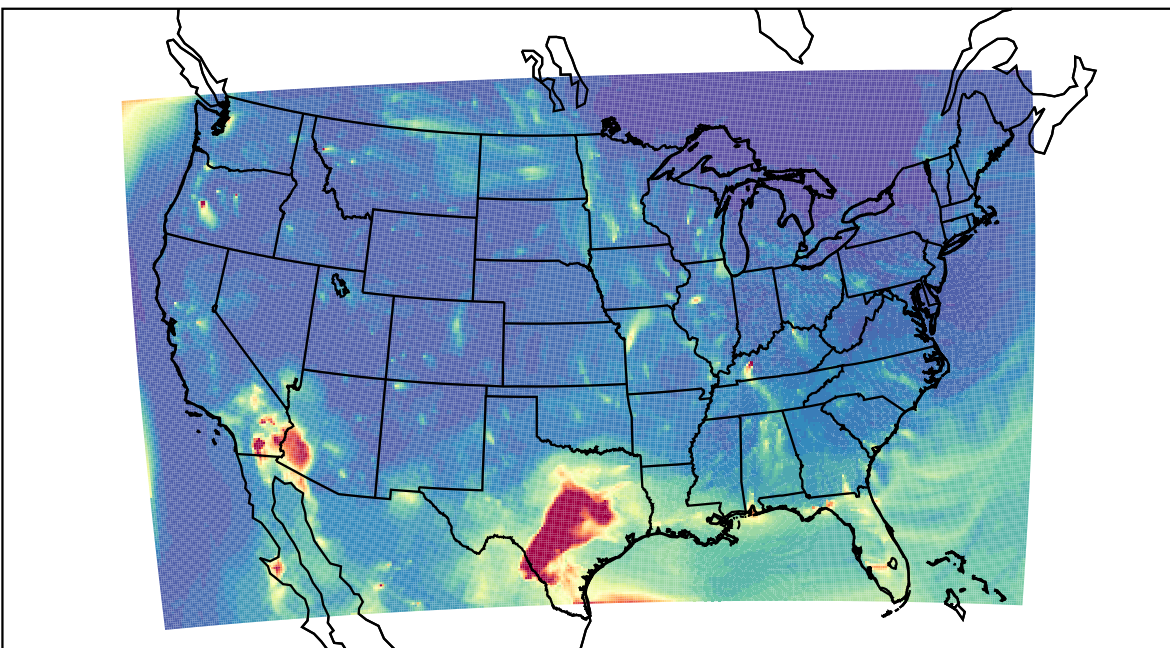
WRF 2021-05-01_04:00:00
