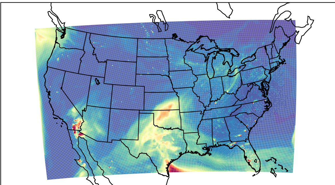
WRF 2021-05-01_23:00:00
