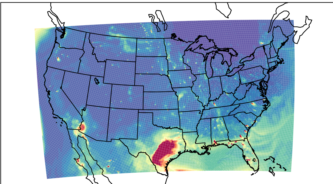
WRF 2021-05-01_01:00:00
