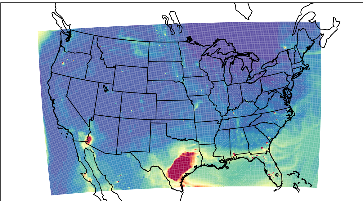
WRF 2021-04-30_23:00:00
