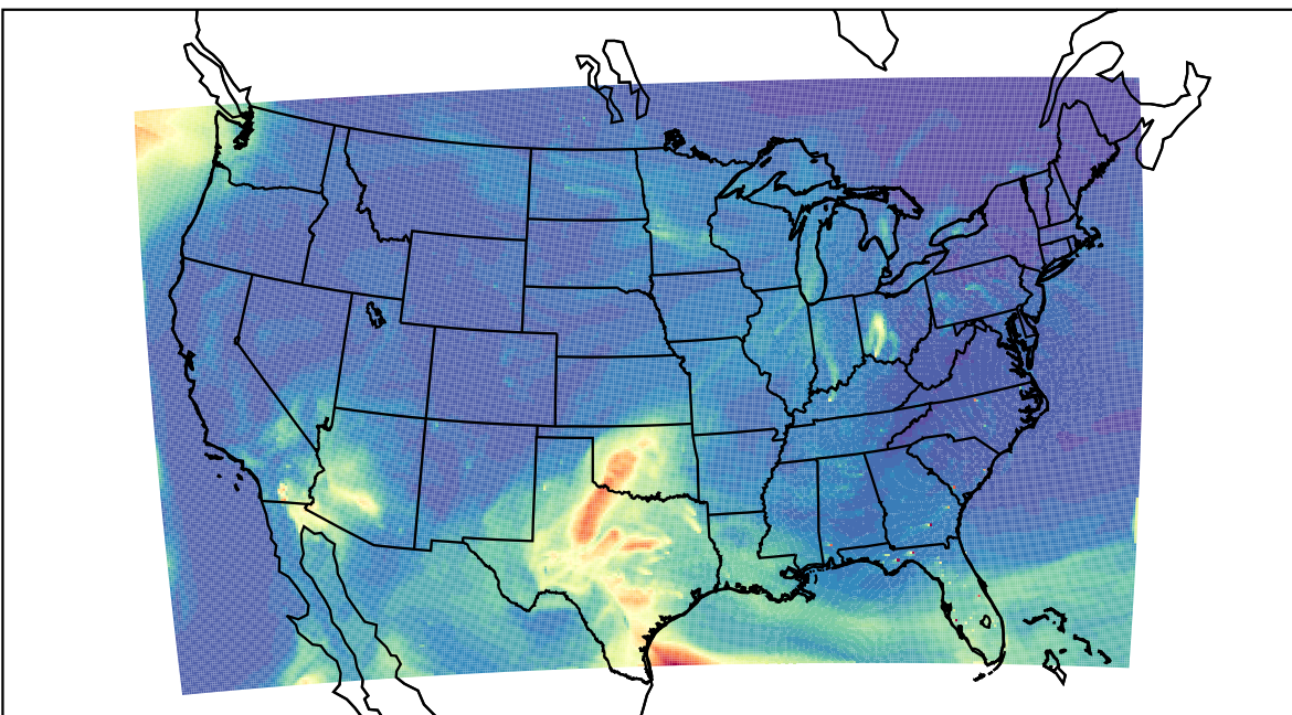
WRF 2021-05-01_18:00:00
