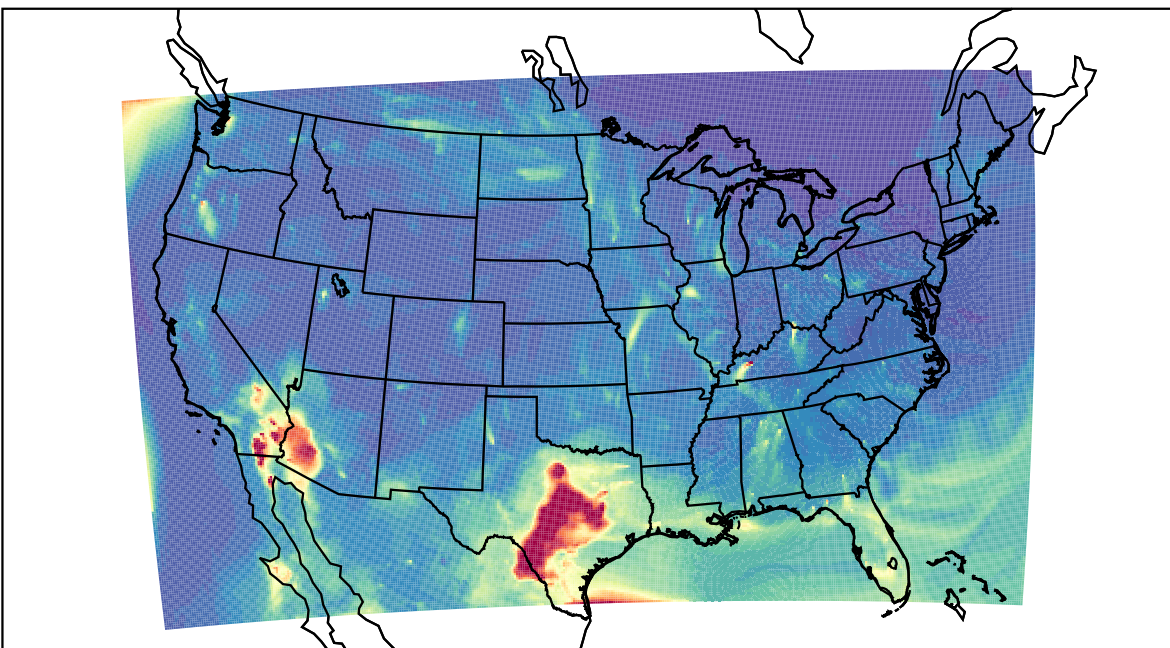
WRF 2021-05-01_06:00:00
