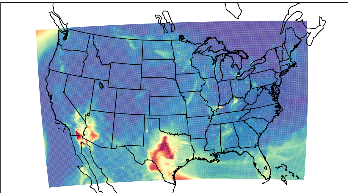
WRF 2021-05-01_10:00:00
