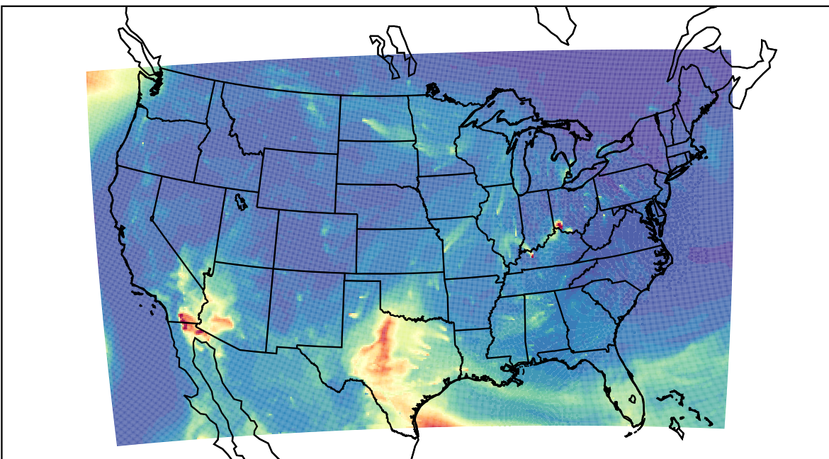
WRF 2021-05-01_14:00:00
