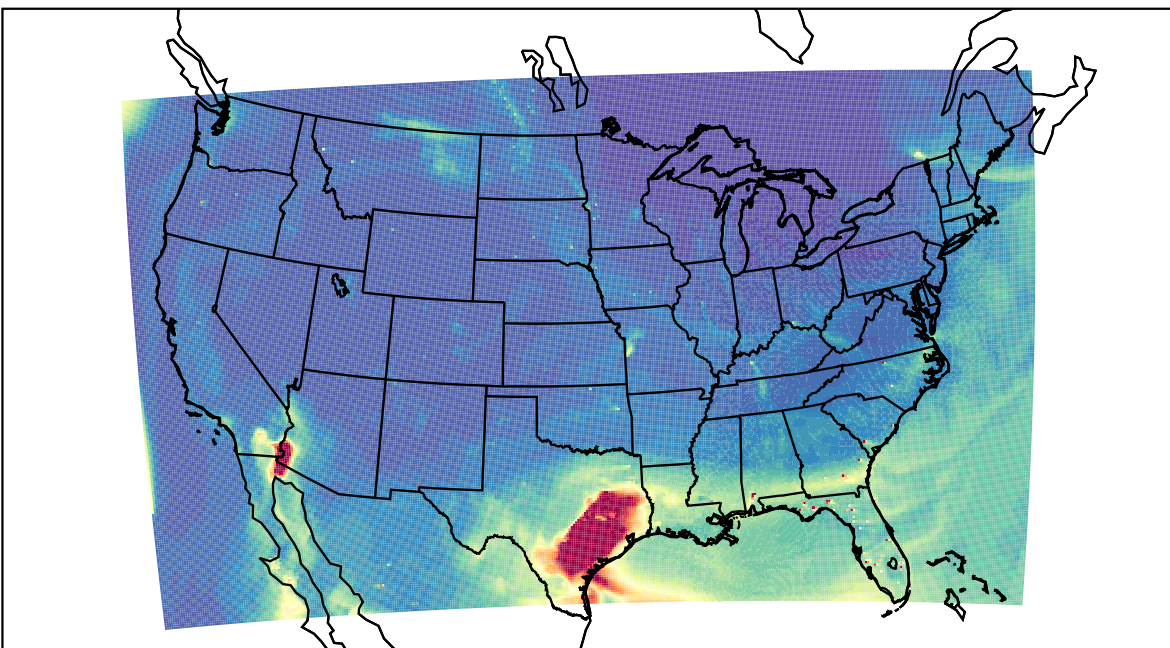
WRF 2021-04-30_20:00:00
