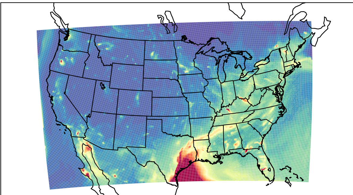
WRF 2021-04-30_04:00:00
