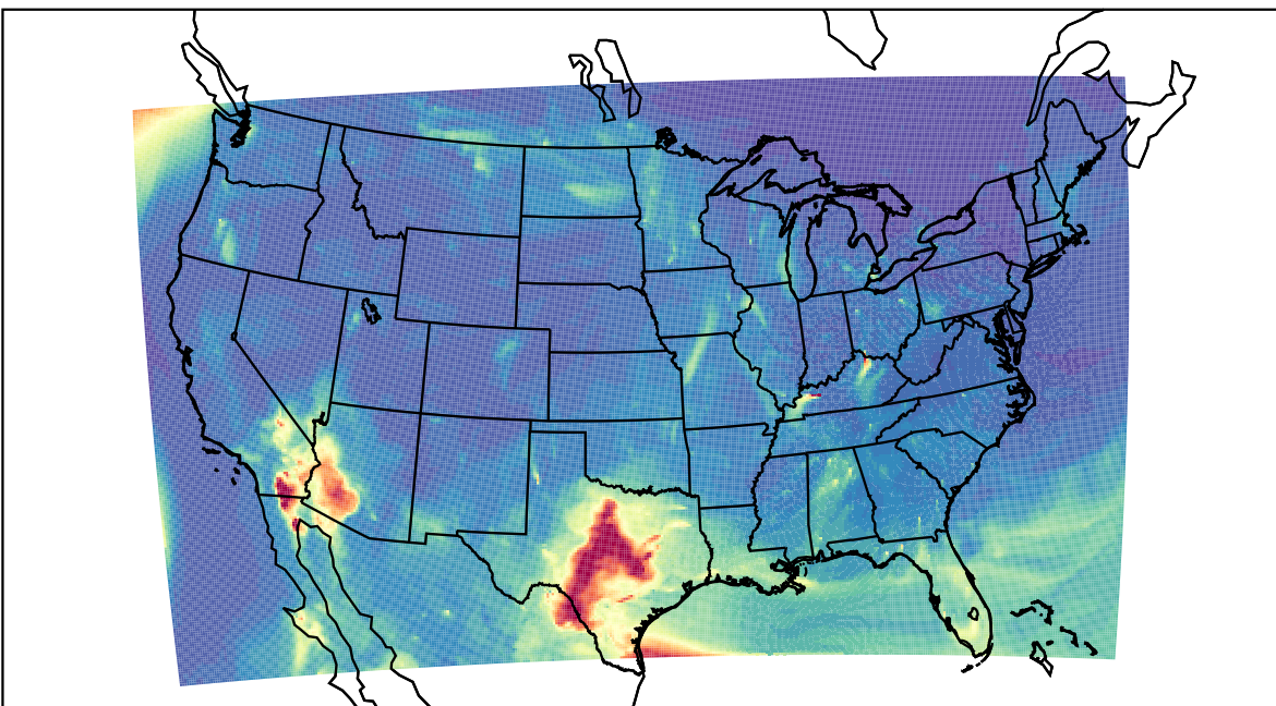
WRF 2021-05-01_08:00:00
