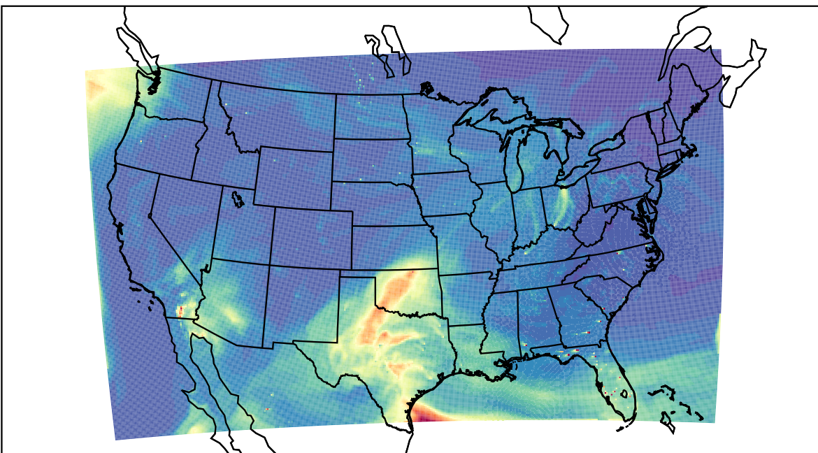
WRF 2021-05-01_20:00:00
