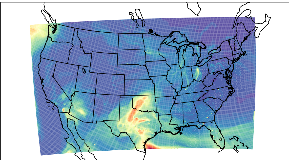
WRF 2021-05-01_19:00:00
