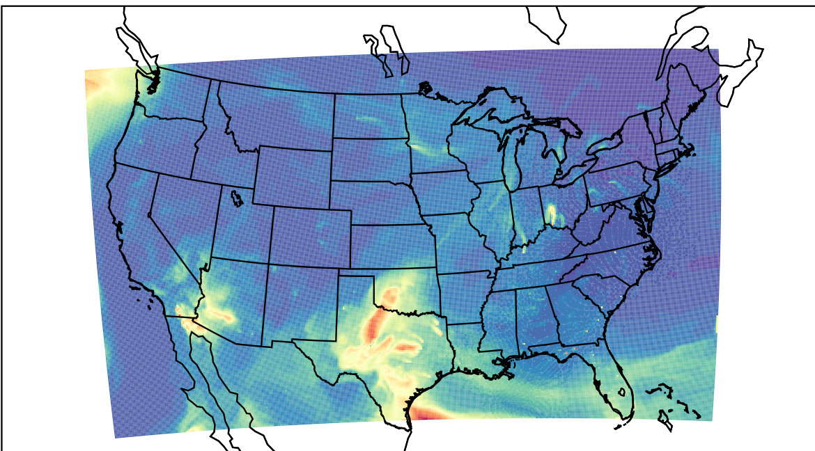
WRF 2021-05-01_17:00:00
