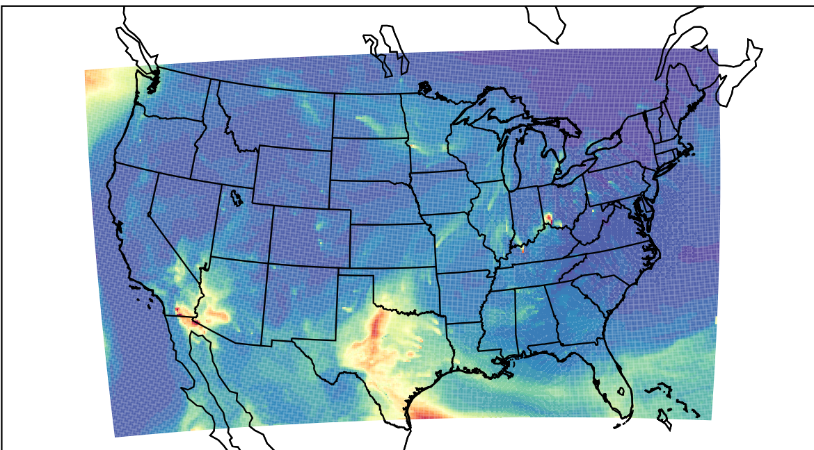
WRF 2021-05-01_15:00:00
