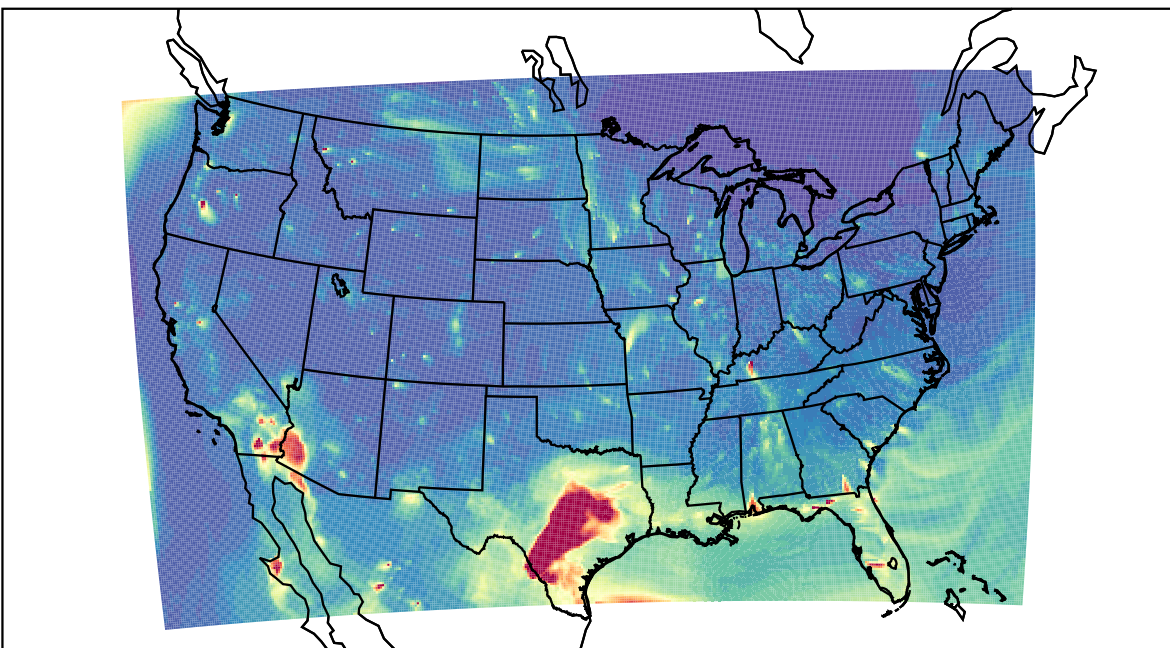
WRF 2021-05-01_03:00:00
