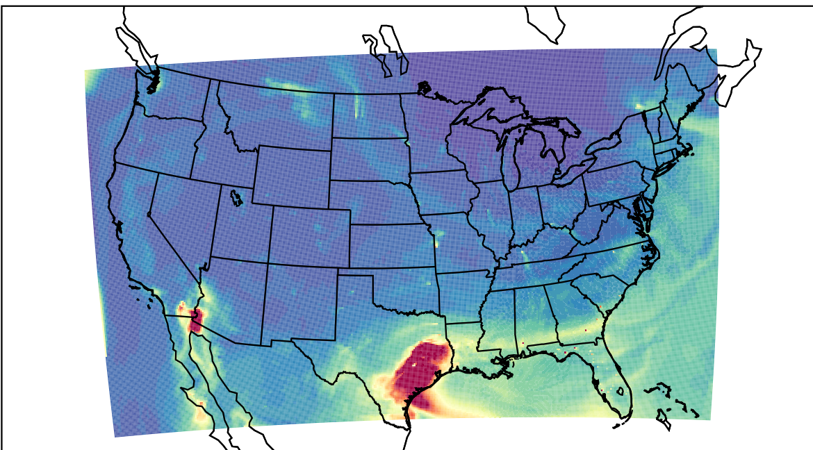
WRF 2021-04-30_18:00:00
