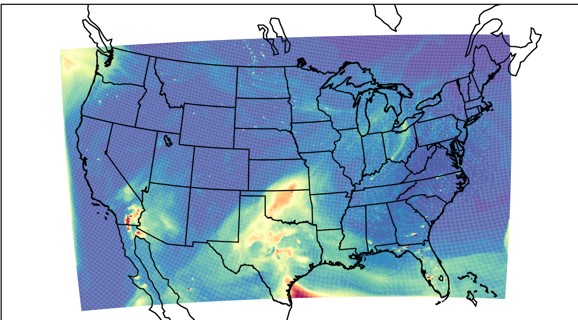
WRF 2021-05-01_22:00:00
