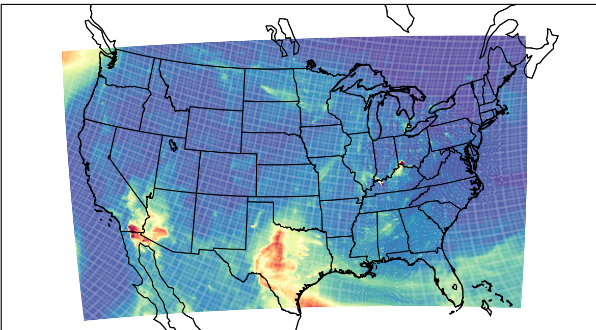
WRF 2021-05-01_13:00:00
