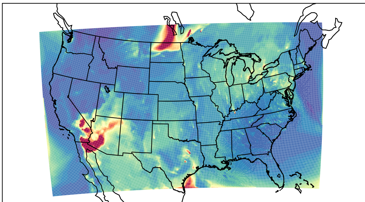
WRF 2021-05-20_13:00:00
