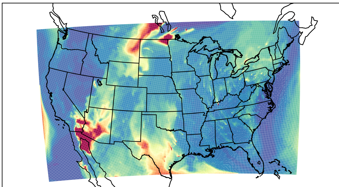
WRF 2021-05-21_13:00:00
