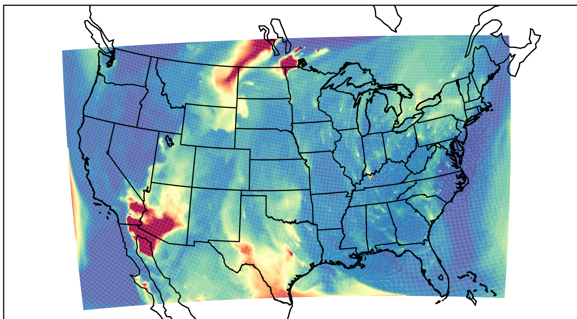
WRF 2021-05-21_11:00:00
