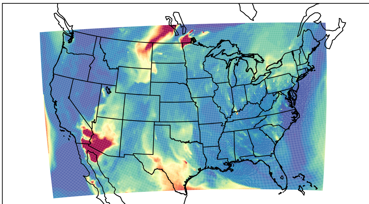
WRF 2021-05-21_10:00:00
