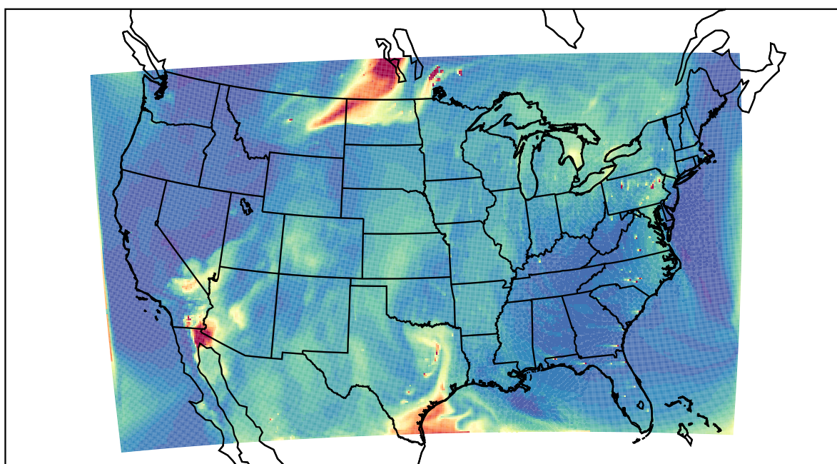
WRF 2021-05-20_20:00:00
