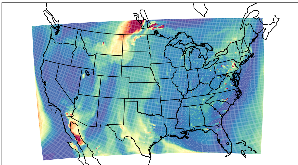
WRF 2021-05-21_23:00:00
