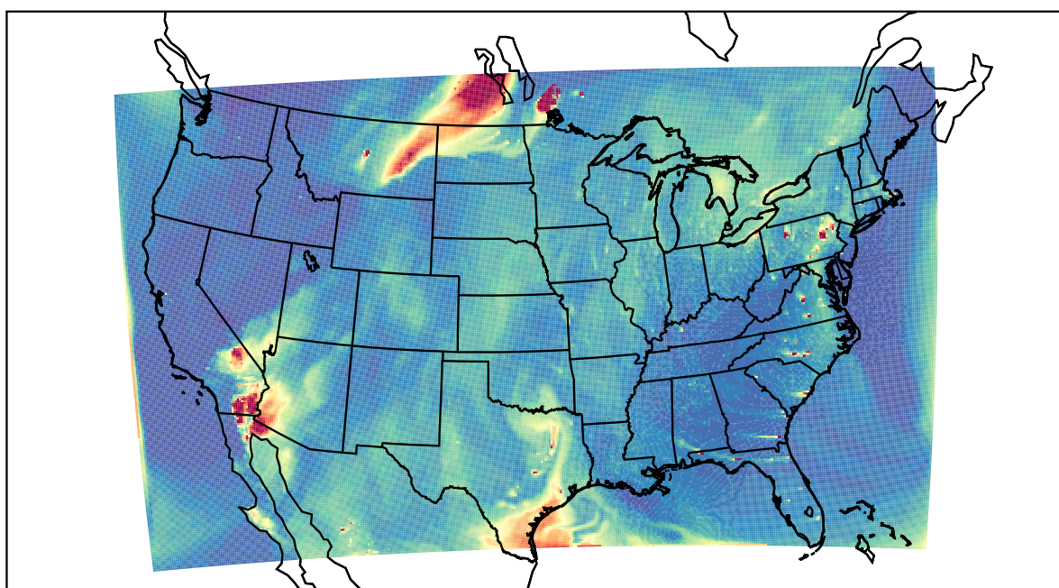
WRF 2021-05-20_23:00:00
