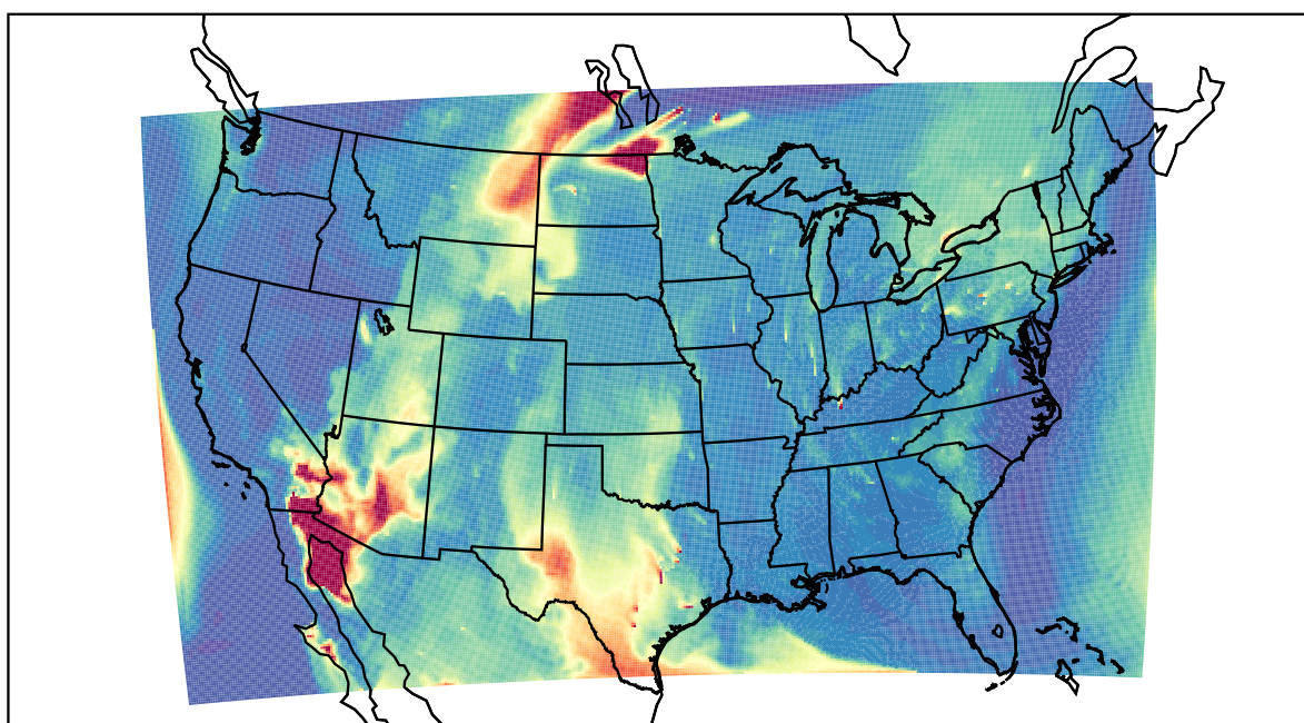
WRF 2021-05-21_14:00:00
