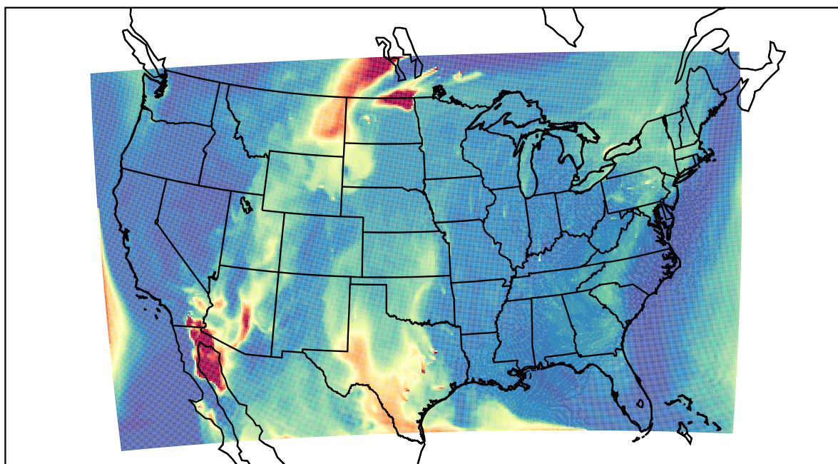
WRF 2021-05-21_16:00:00
