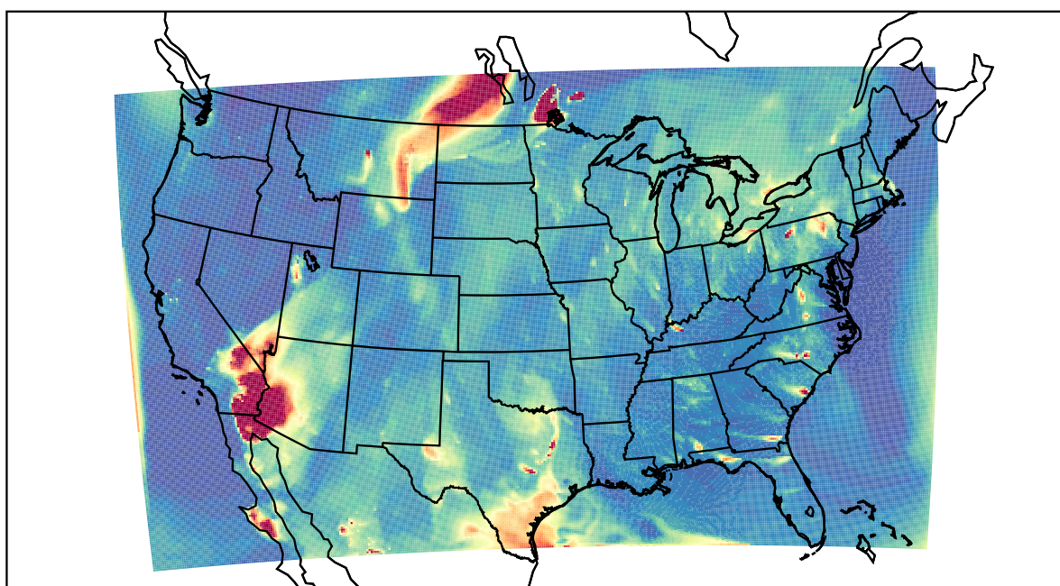
WRF 2021-05-21_03:00:00
