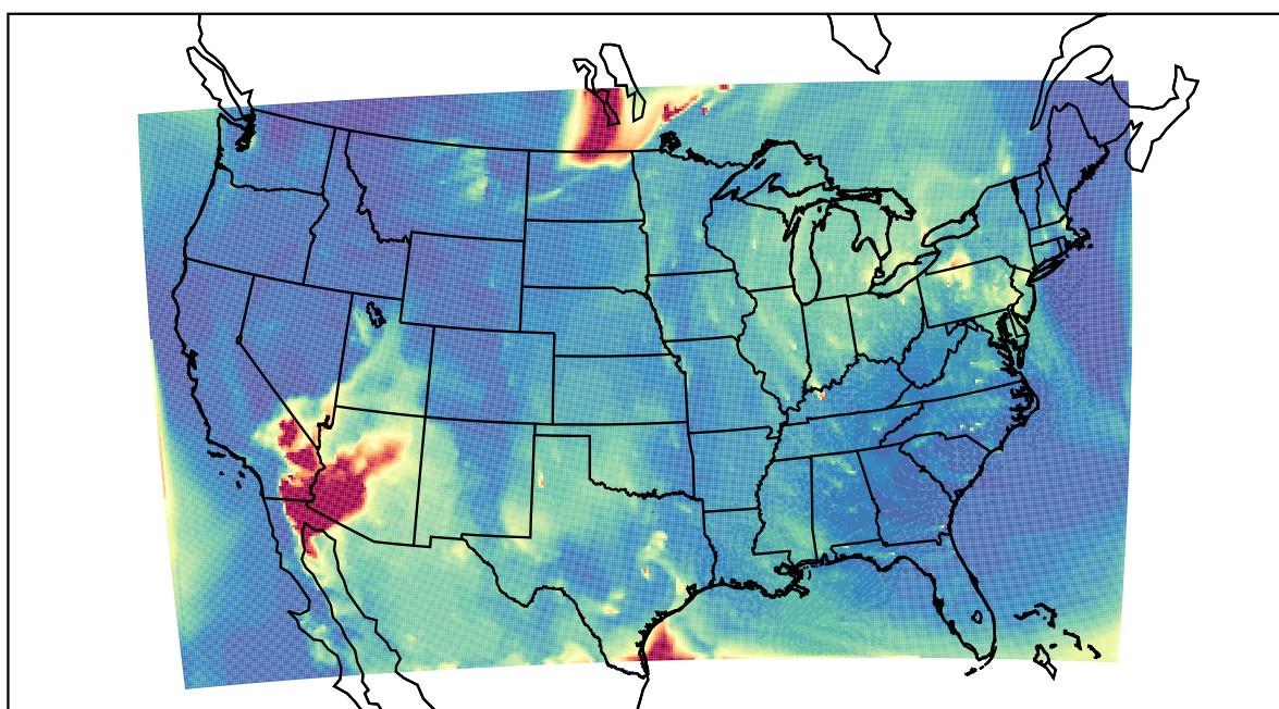
WRF 2021-05-20_10:00:00
