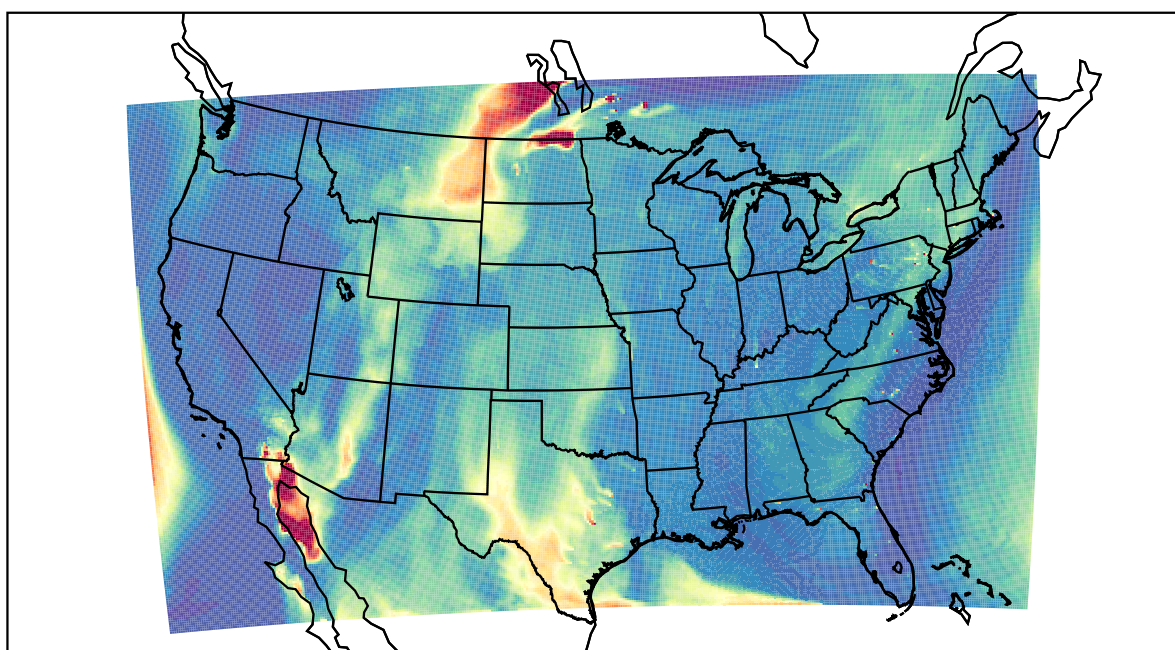
WRF 2021-05-21_18:00:00
