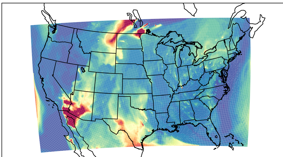
WRF 2021-05-21_12:00:00
