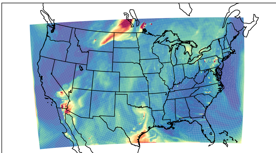
WRF 2021-05-20_22:00:00
