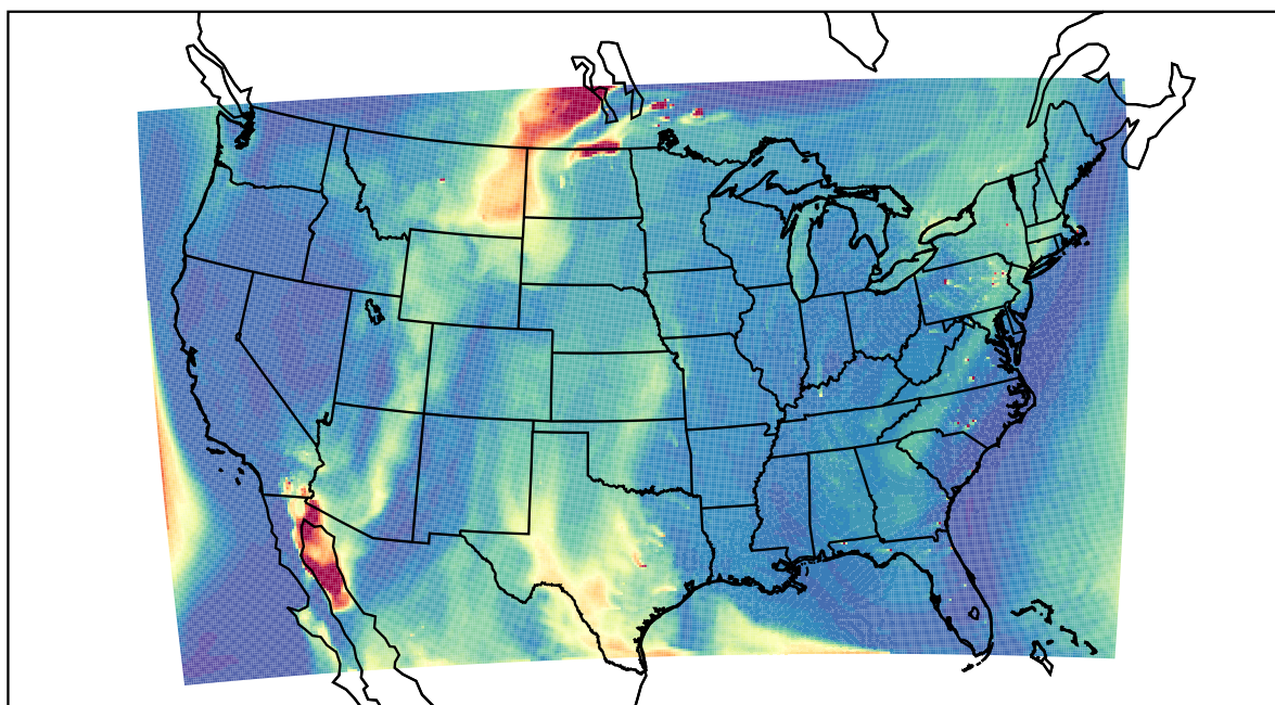
WRF 2021-05-21_19:00:00
