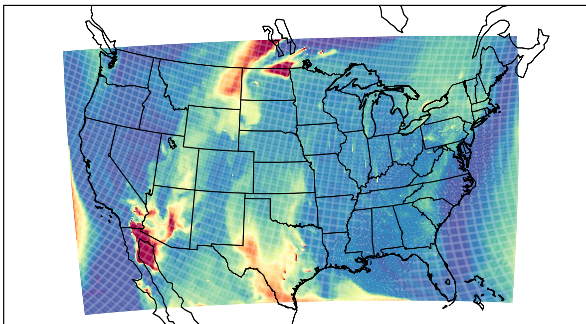
WRF 2021-05-21_15:00:00
