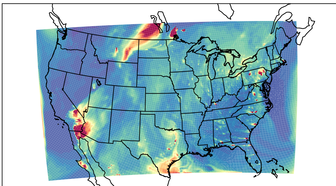
WRF 2021-05-21_01:00:00
