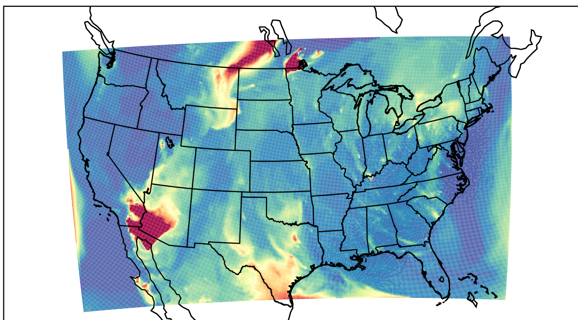
WRF 2021-05-21_08:00:00
