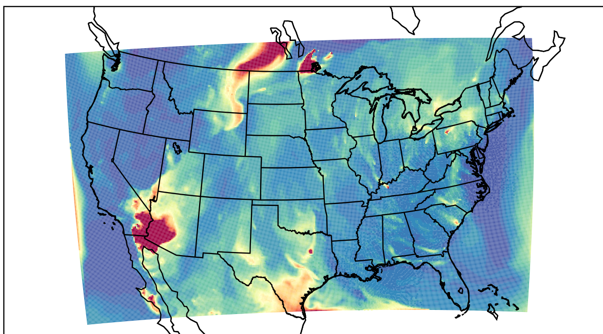
WRF 2021-05-21_06:00:00
