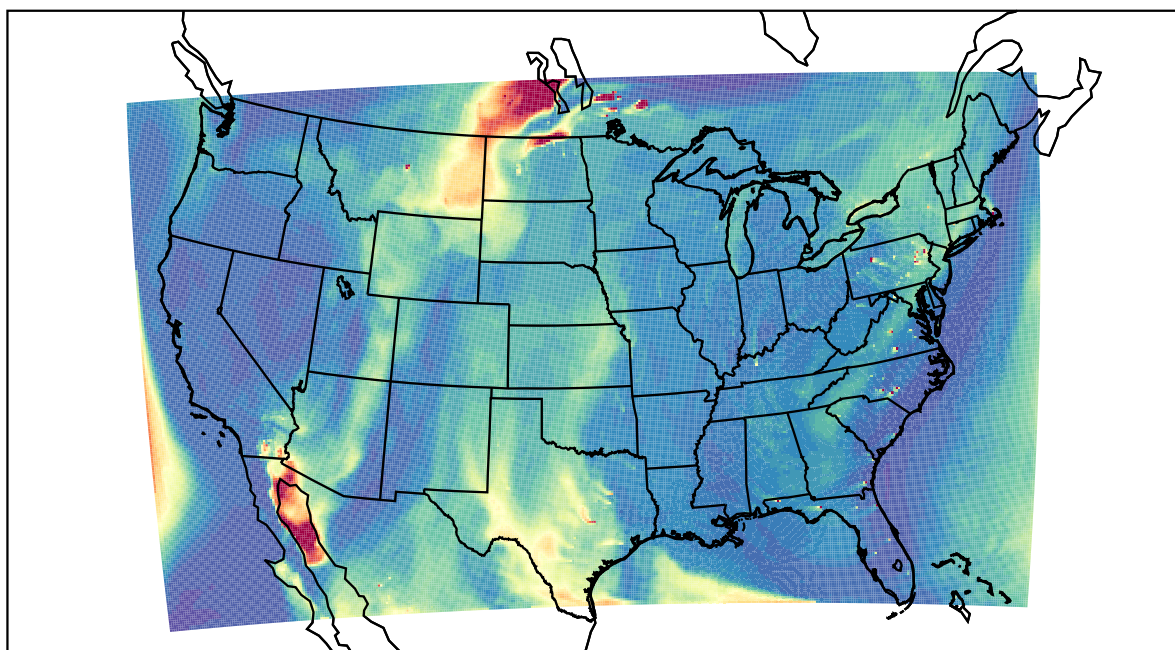
WRF 2021-05-21_20:00:00
