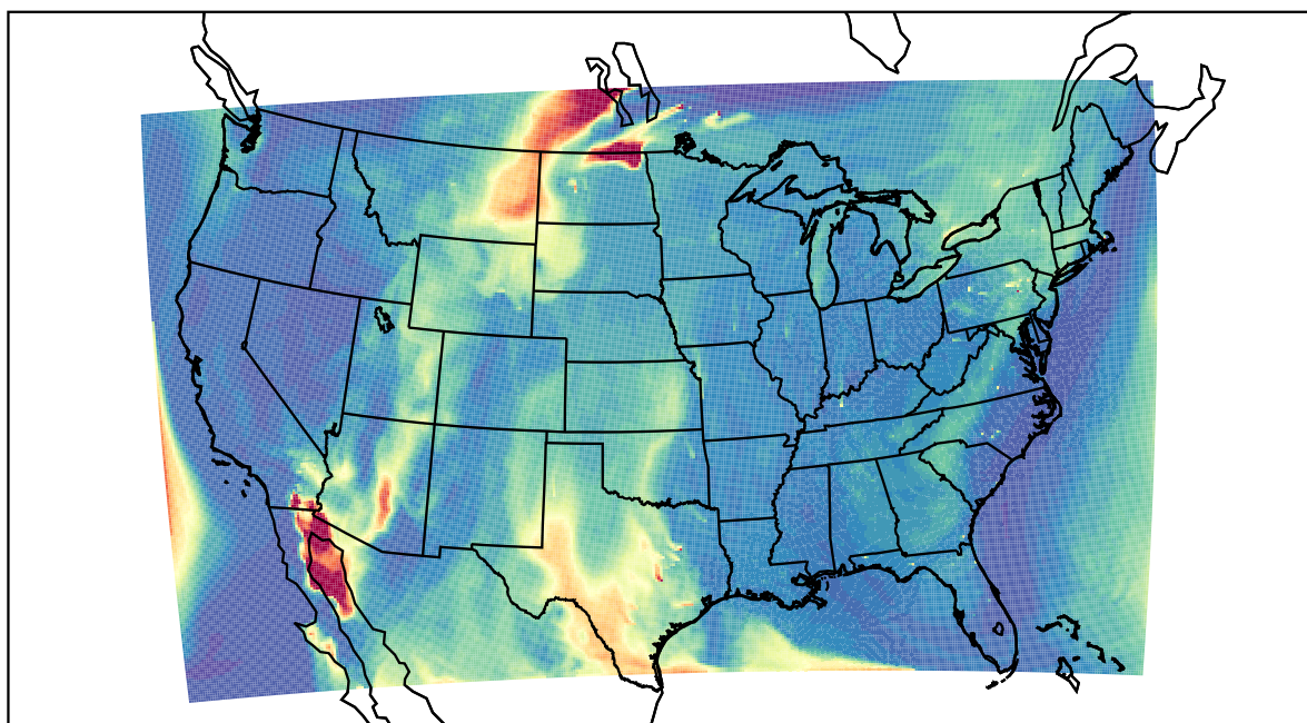
WRF 2021-05-21_17:00:00
