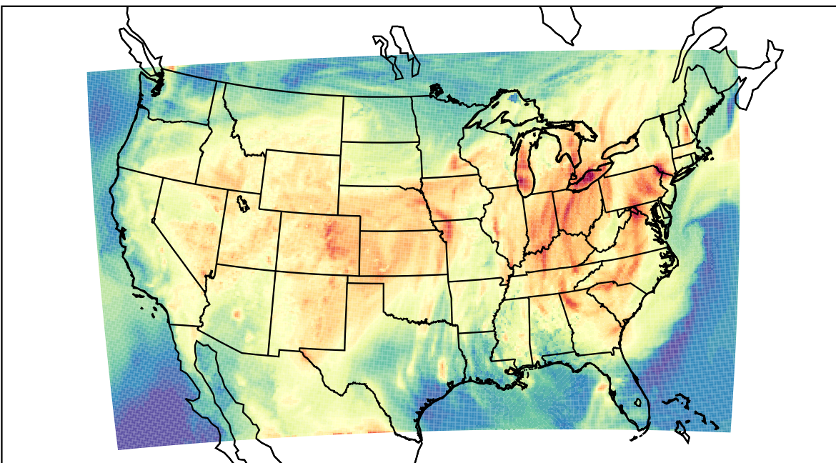
WRF (2021-06-24_20:00:00)
