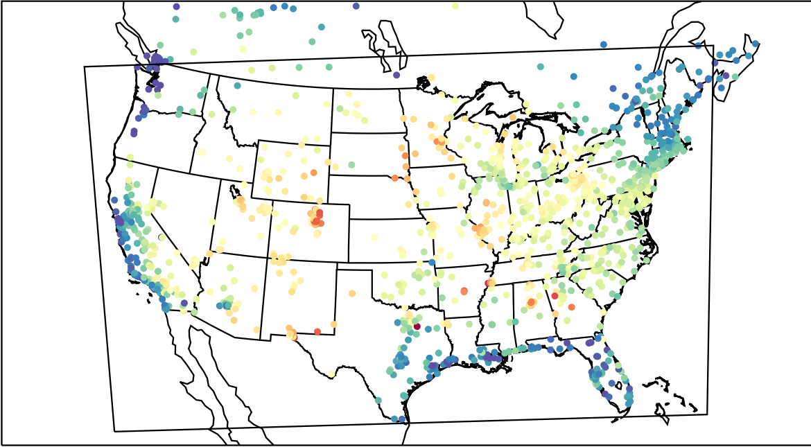
AirNOW (2021-06-23_18:00:00)
