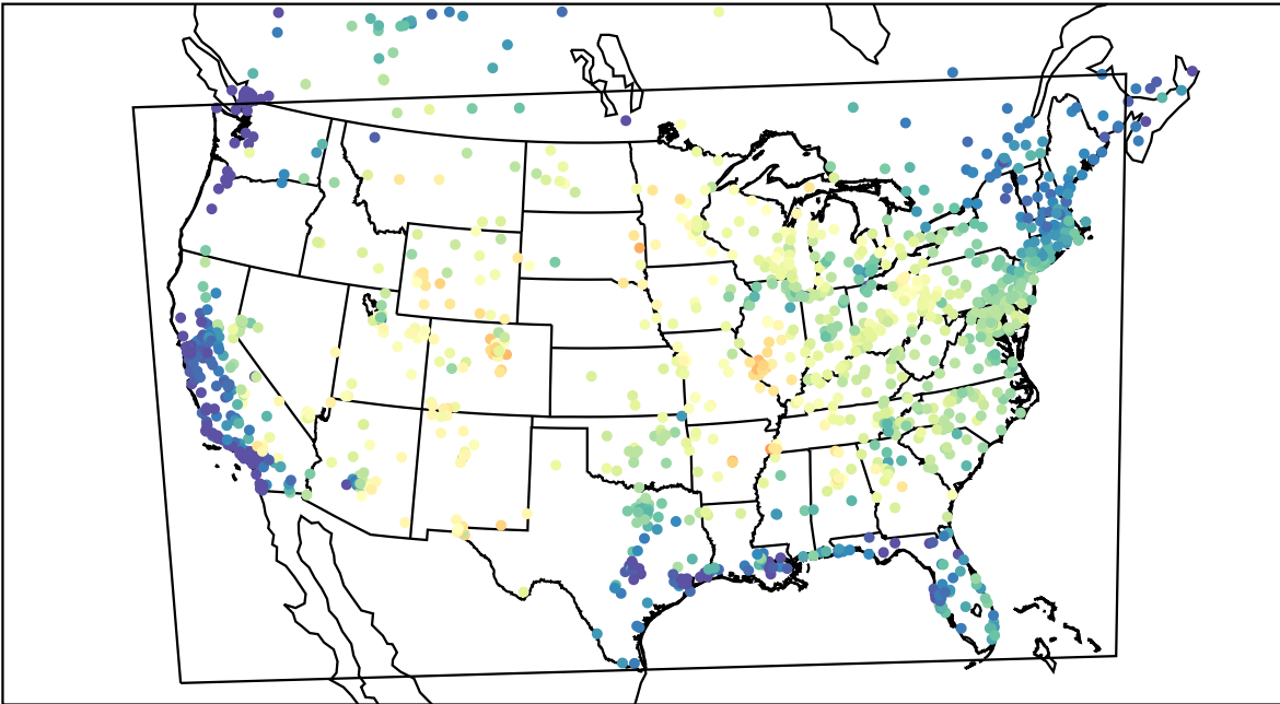
AirNOW (2021-06-23_16:00:00)
