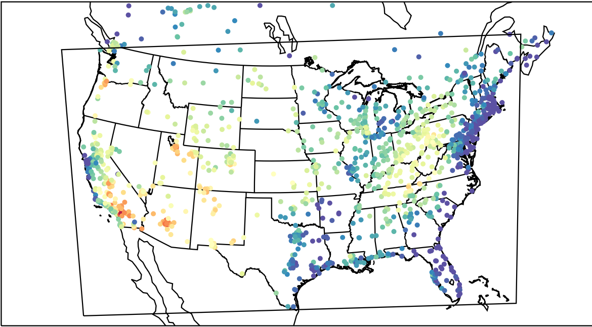
AirNOW (2021-06-26_18:00:00)
