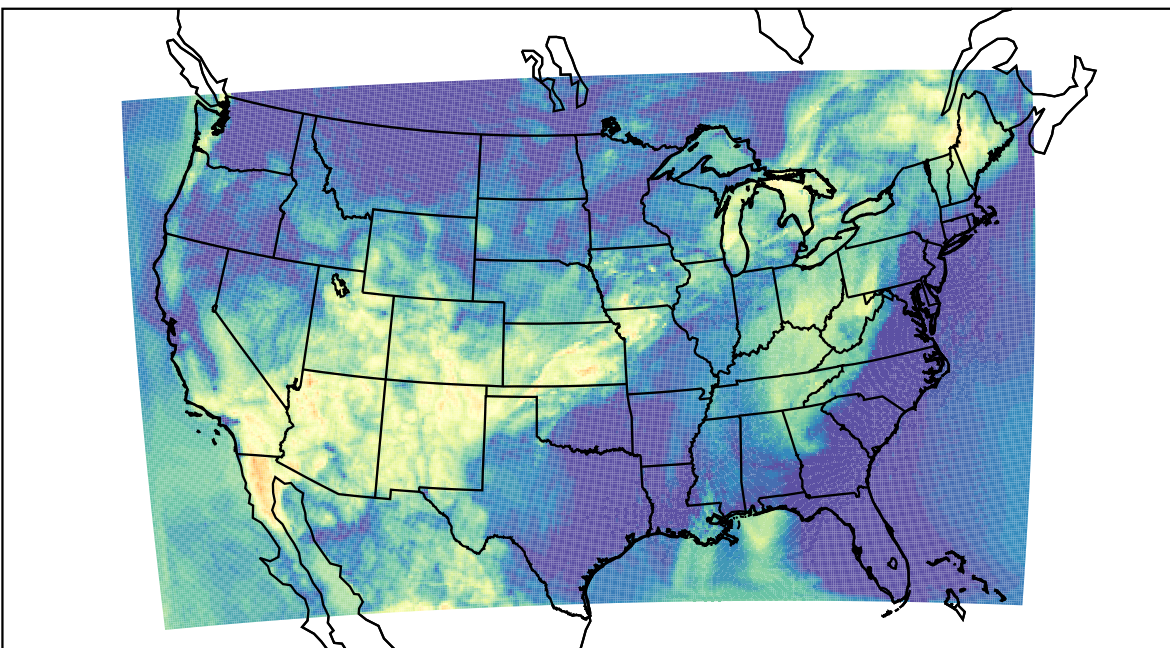
WRF (2021-06-26_13:00:00)
