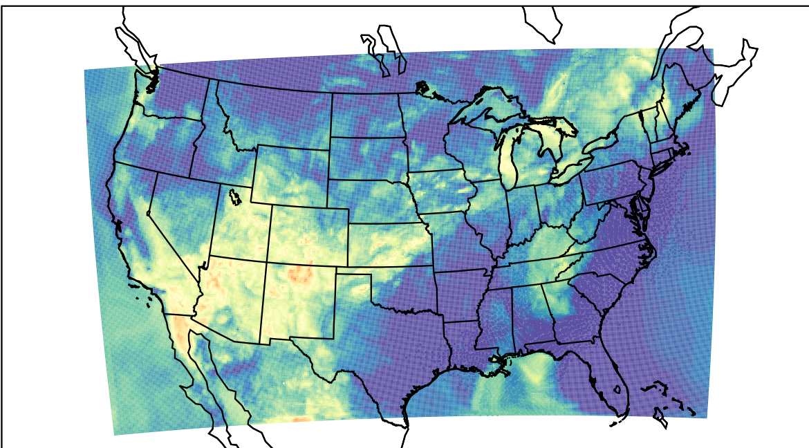
WRF (2021-06-26_10:00:00)
