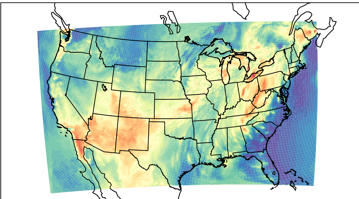
WRF (2021-06-26_18:00:00)
