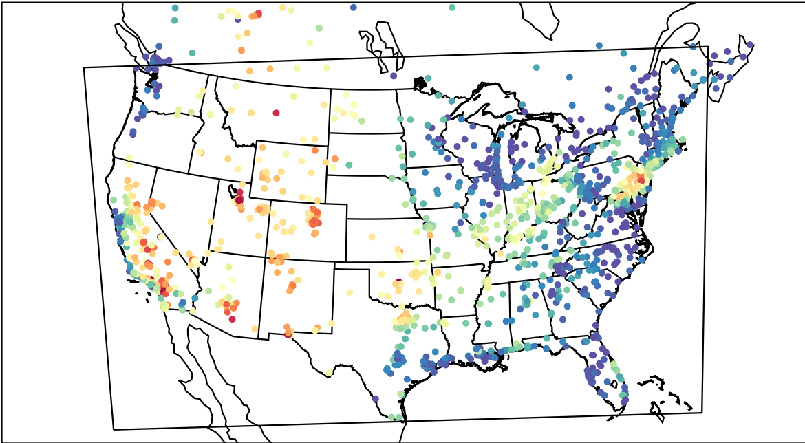
AirNOW (2021-07-08_18:00:00)
