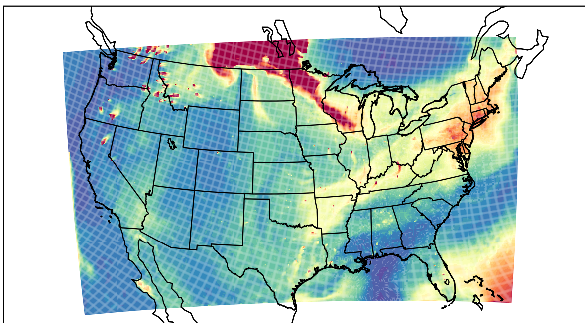
WRF 2021-07-21_00:00:00
