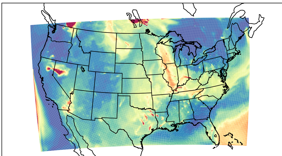
WRF 2021-07-22_12:00:00
