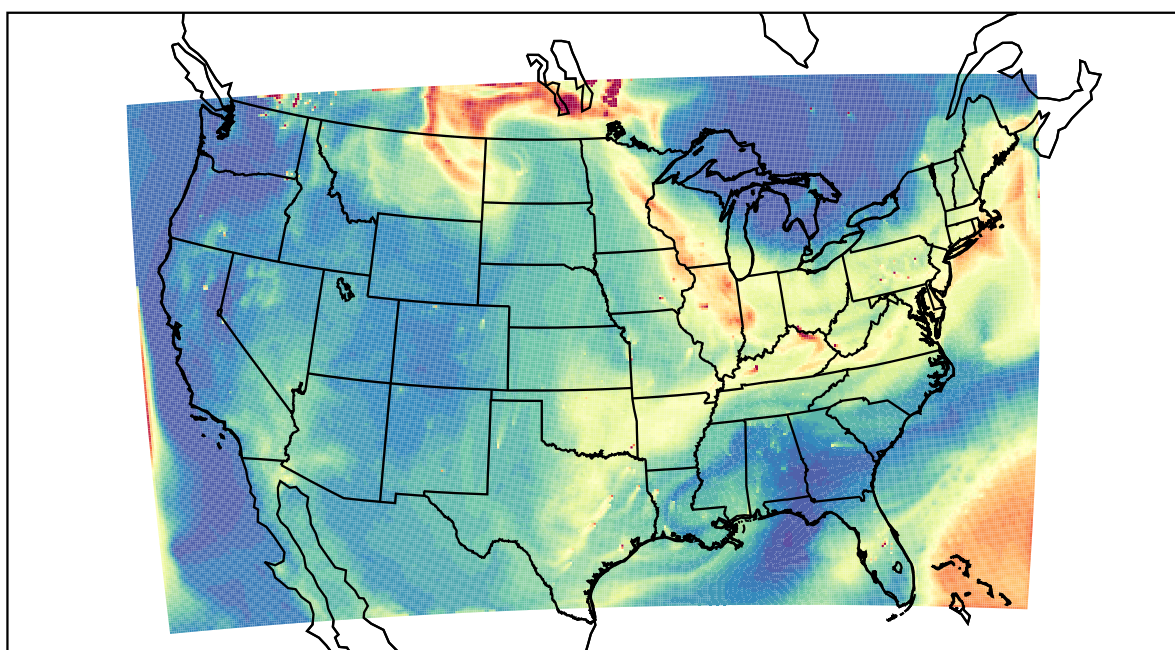
WRF 2021-07-21_19:00:00
