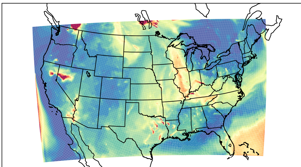
WRF 2021-07-22_13:00:00
