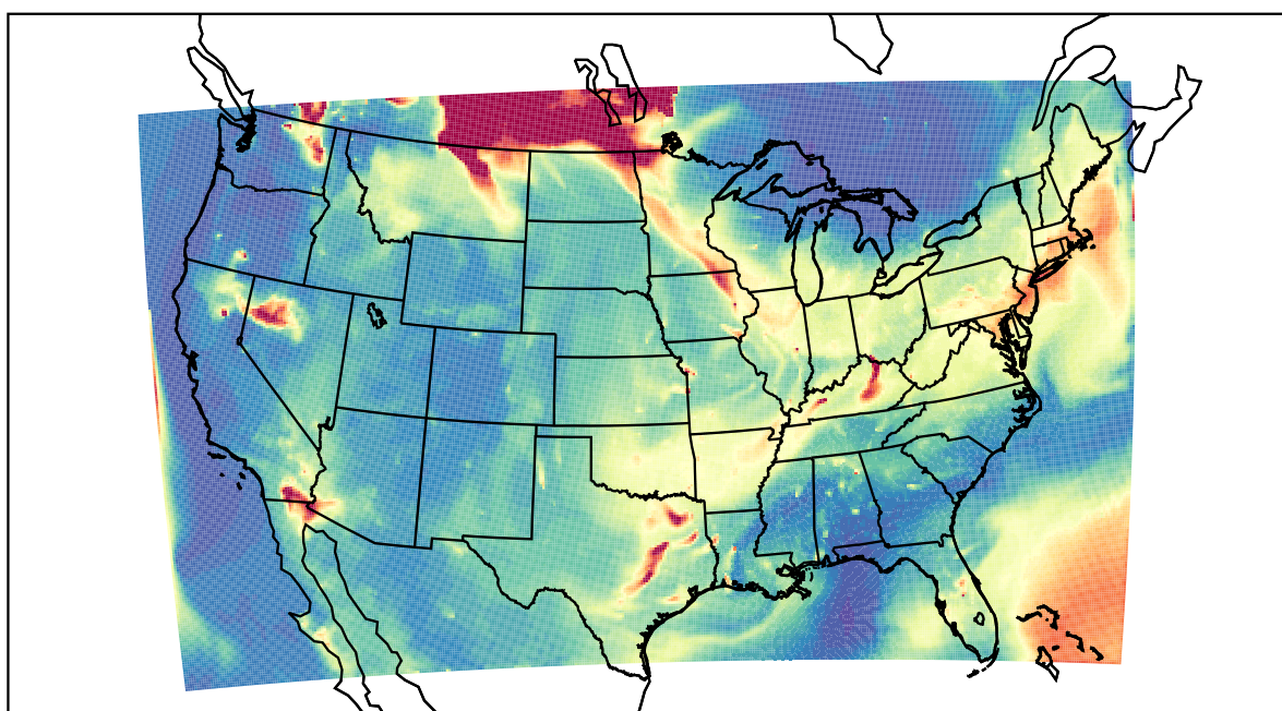
WRF 2021-07-21_12:00:00
