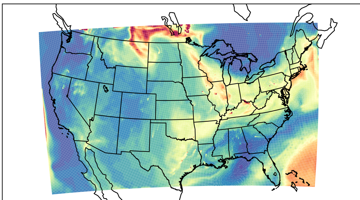
WRF 2021-07-21_18:00:00
