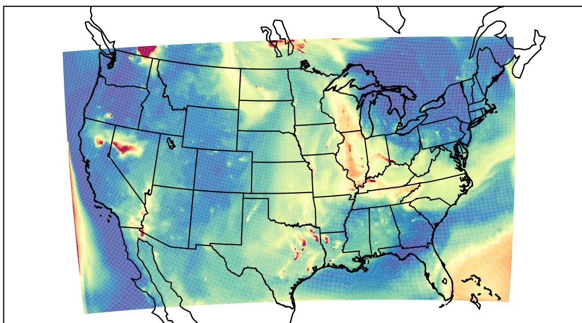
WRF 2021-07-22_14:00:00
