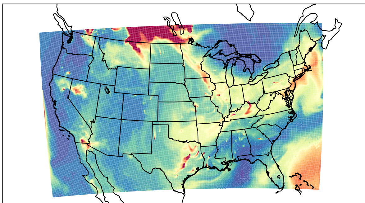
WRF 2021-07-21_14:00:00
