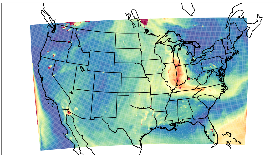
WRF 2021-07-22_22:00:00
