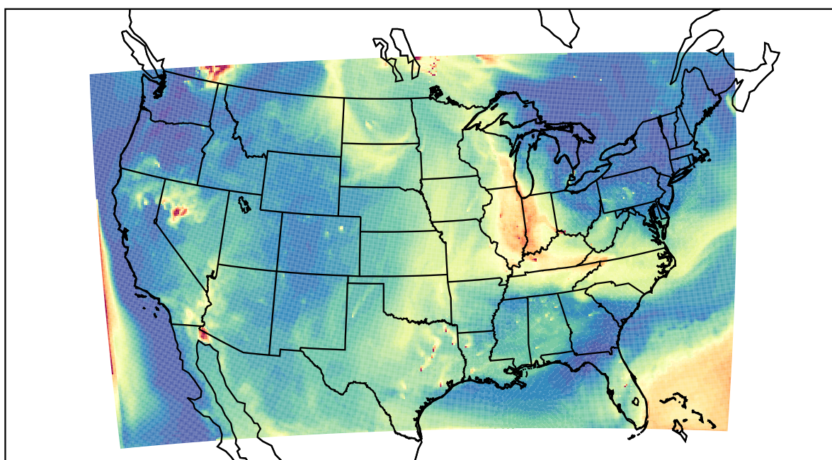
WRF 2021-07-22_17:00:00
