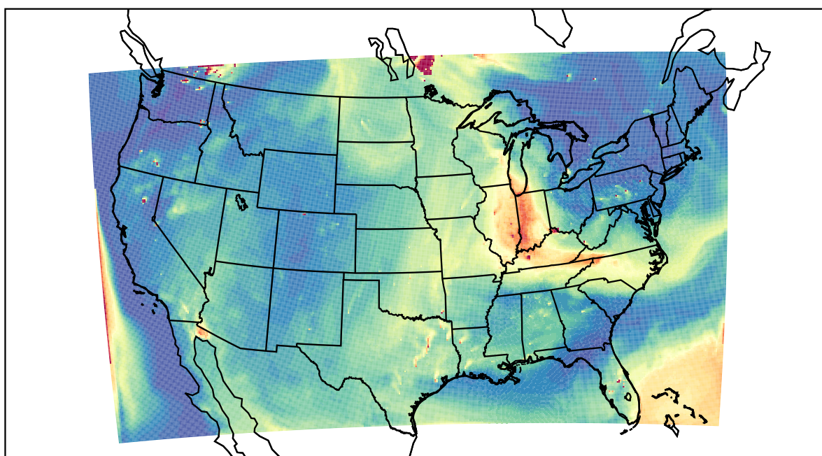
WRF 2021-07-22_20:00:00
