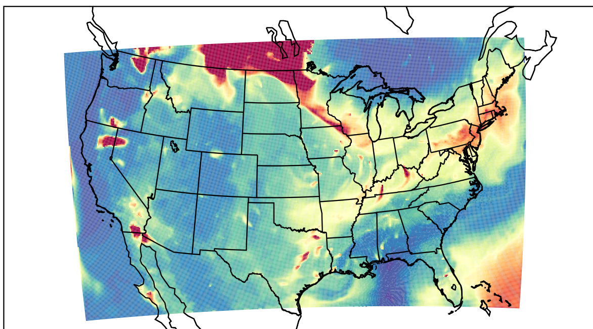
WRF 2021-07-21_06:00:00
