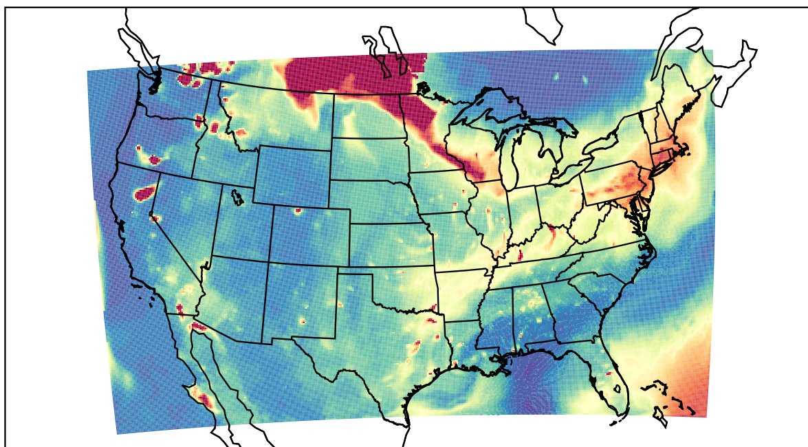
WRF 2021-07-21_03:00:00
