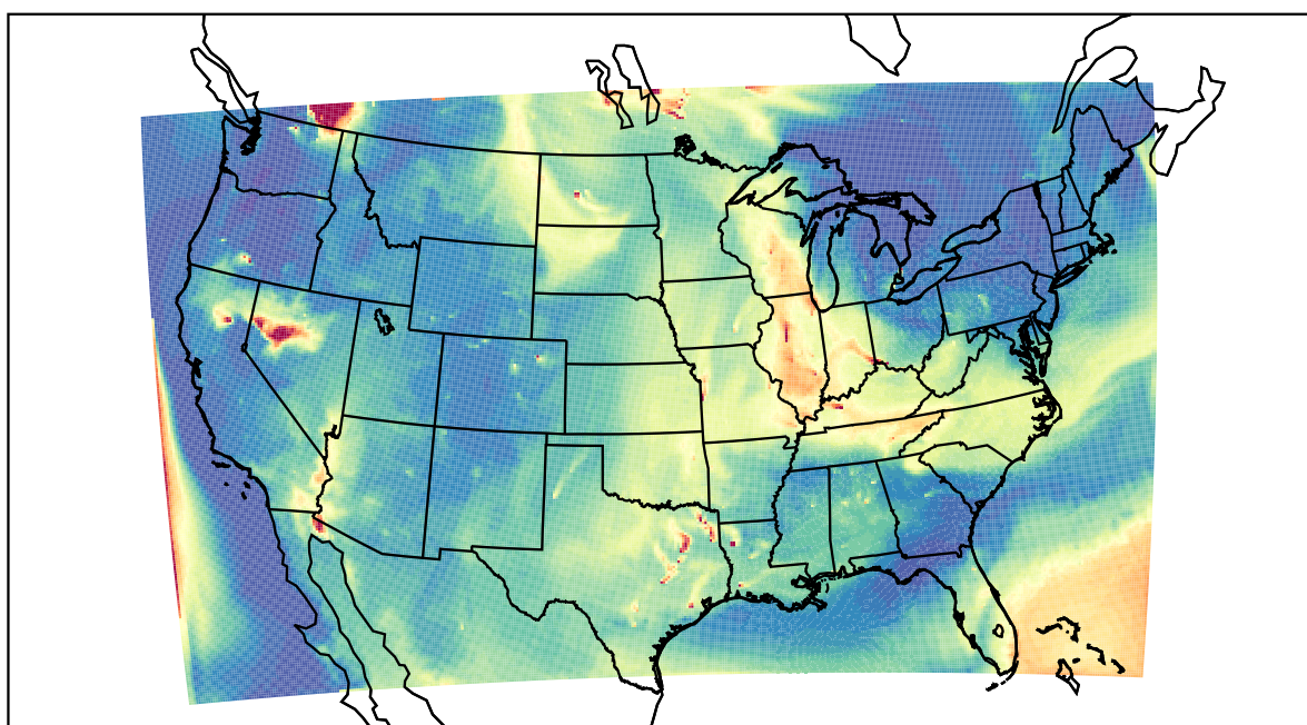
WRF 2021-07-22_15:00:00
