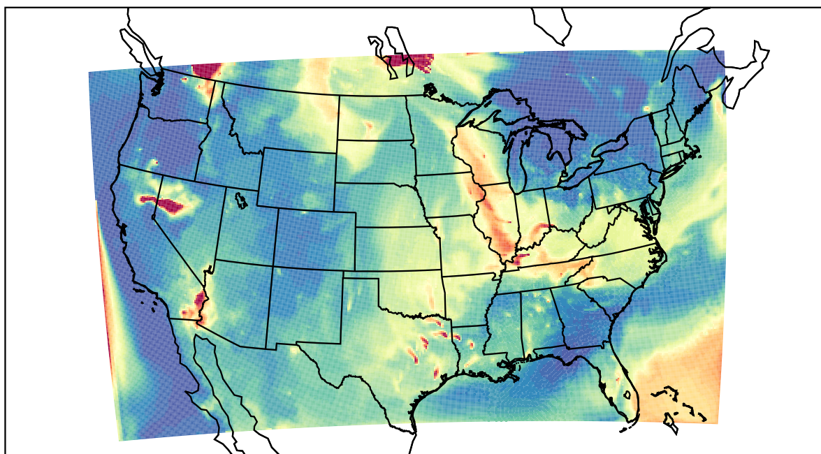
WRF 2021-07-22_10:00:00
