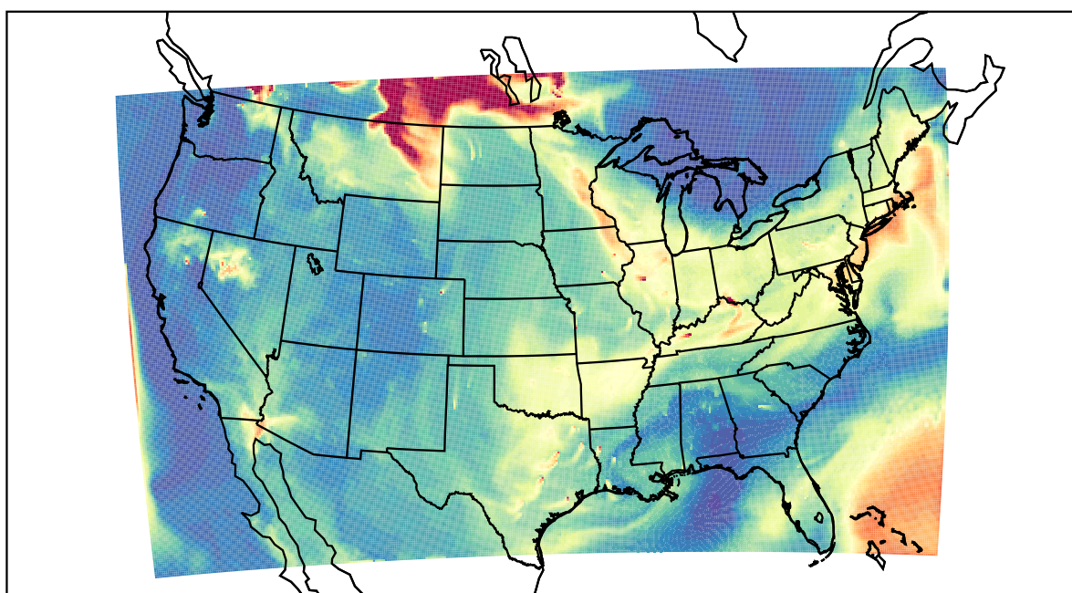
WRF 2021-07-21_16:00:00
