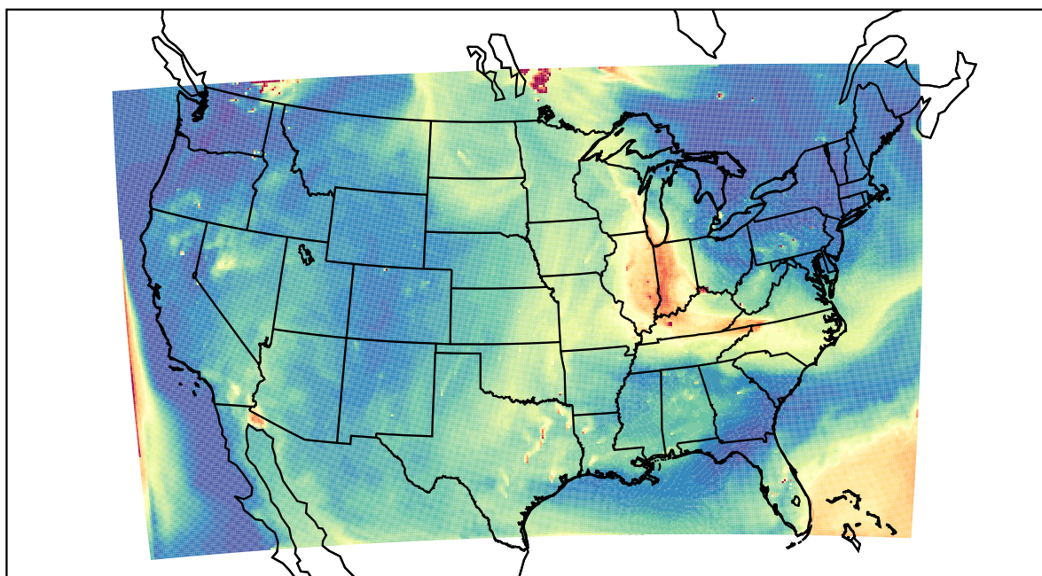
WRF 2021-07-22_19:00:00
