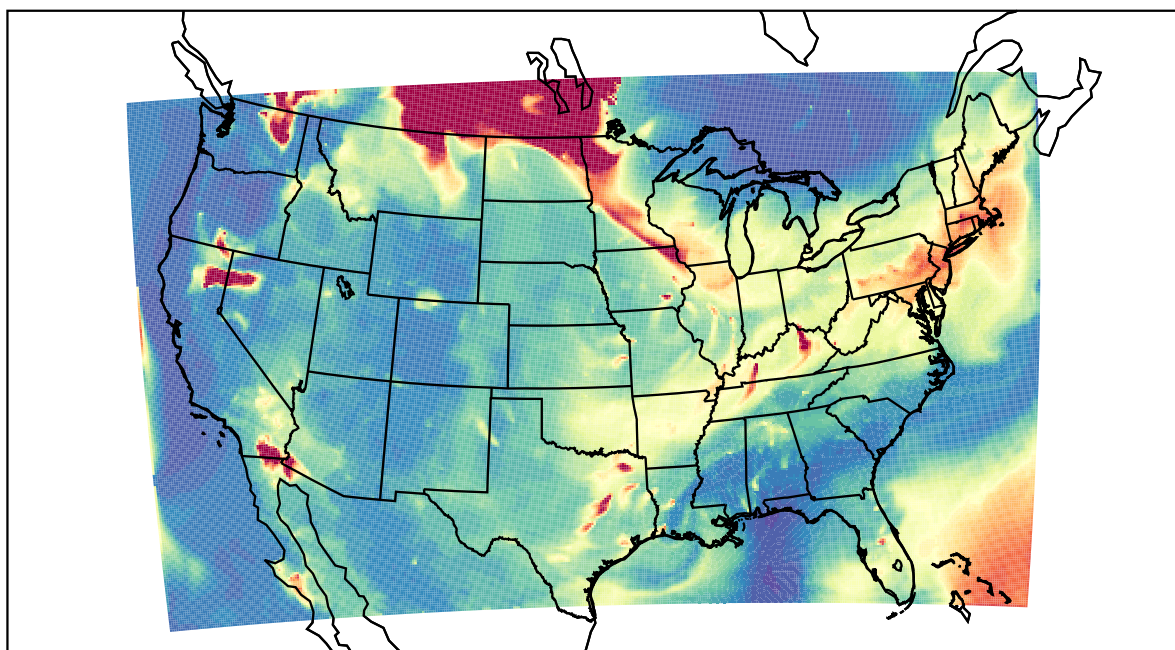
WRF 2021-07-21_07:00:00
