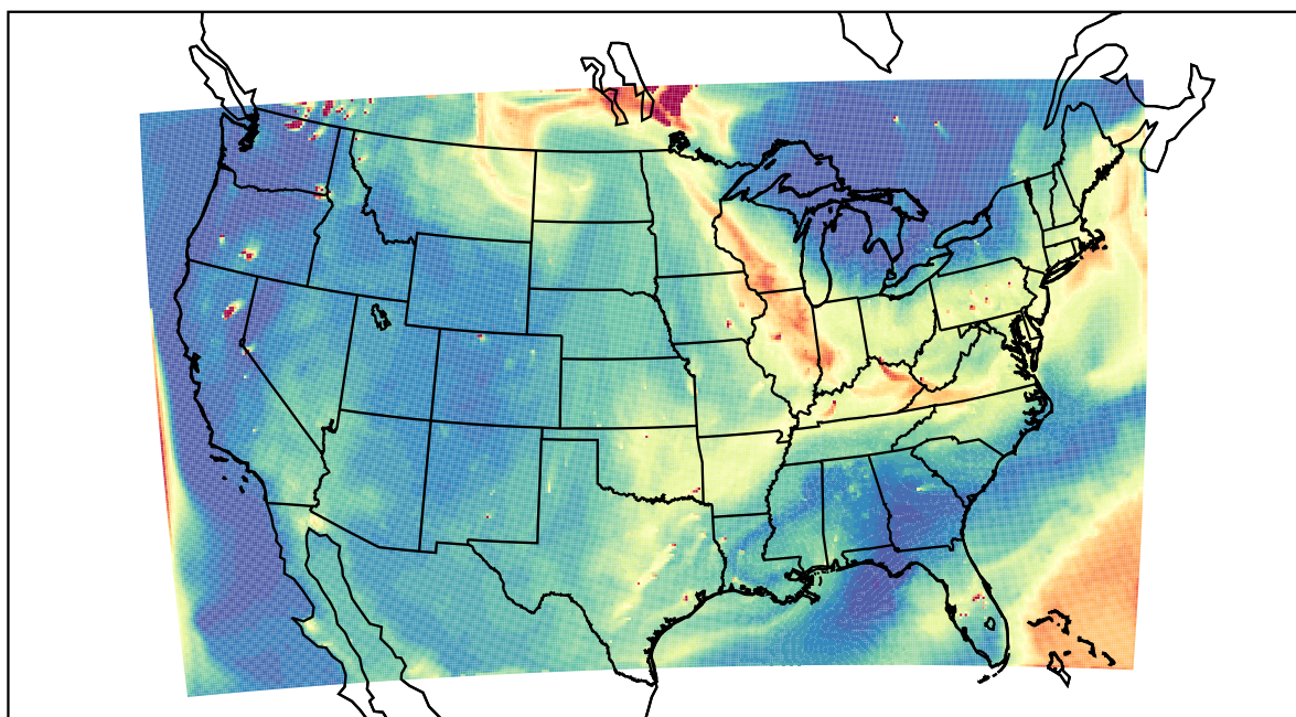
WRF 2021-07-21_22:00:00
