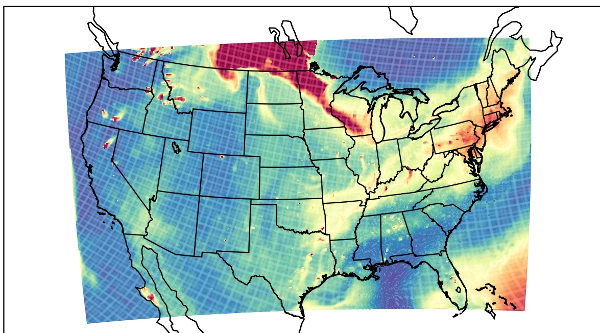
WRF 2021-07-21_01:00:00
