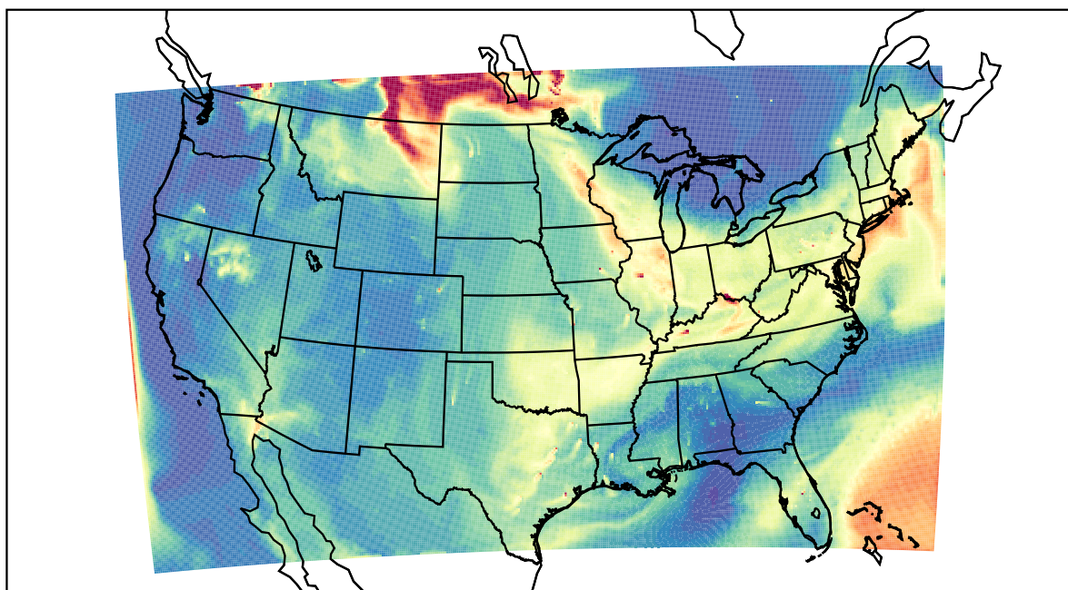
WRF 2021-07-21_17:00:00
