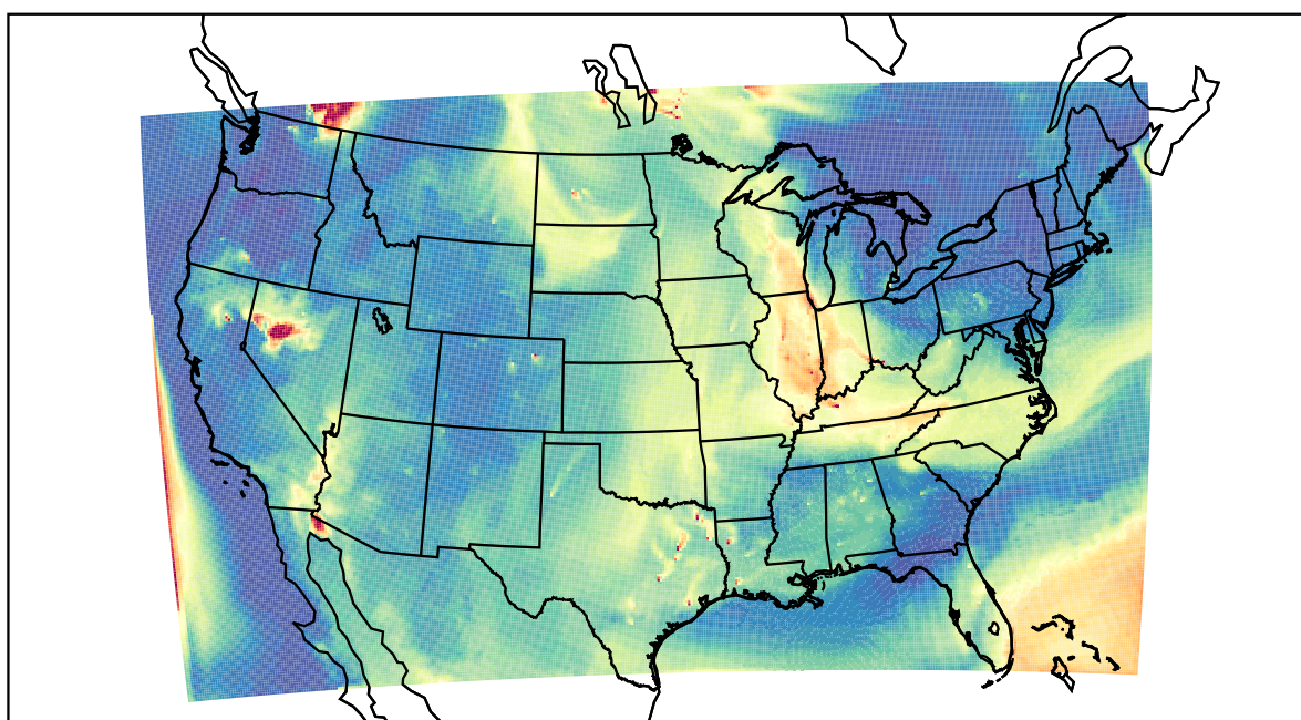
WRF 2021-07-22_16:00:00
