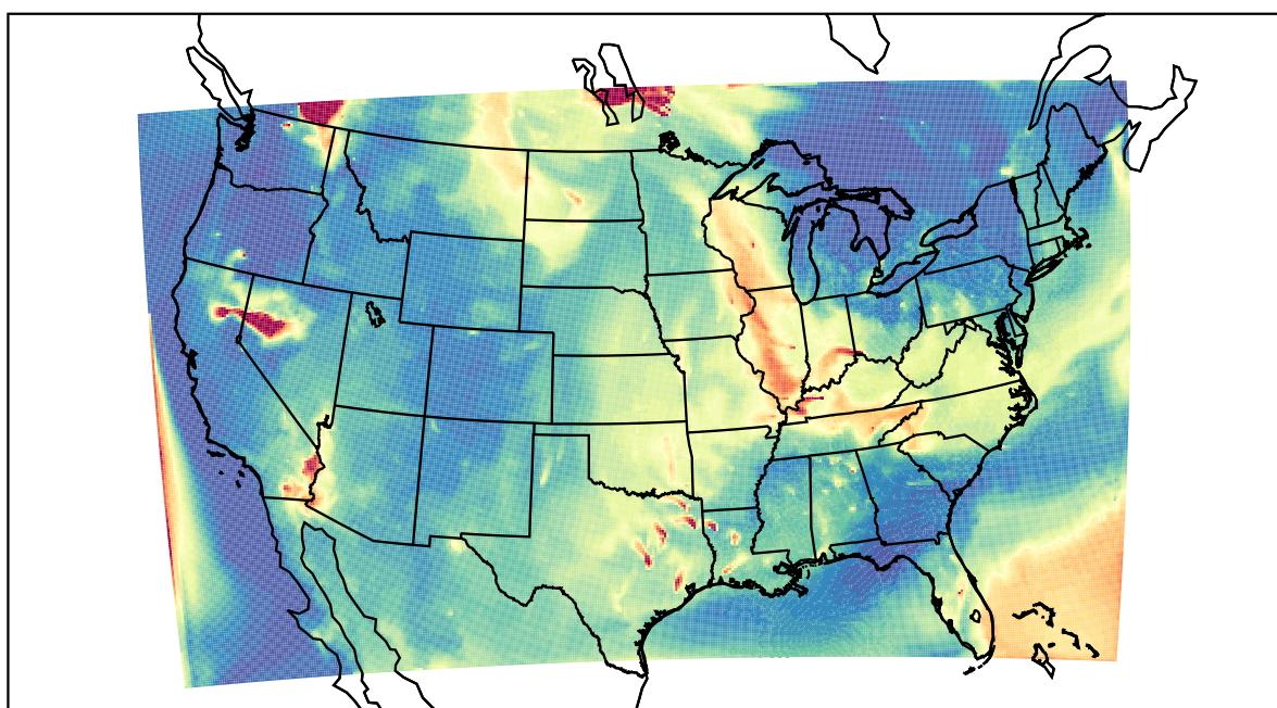
WRF 2021-07-22_11:00:00
