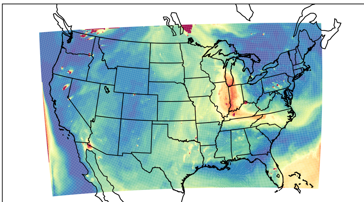
WRF 2021-07-22_23:00:00
