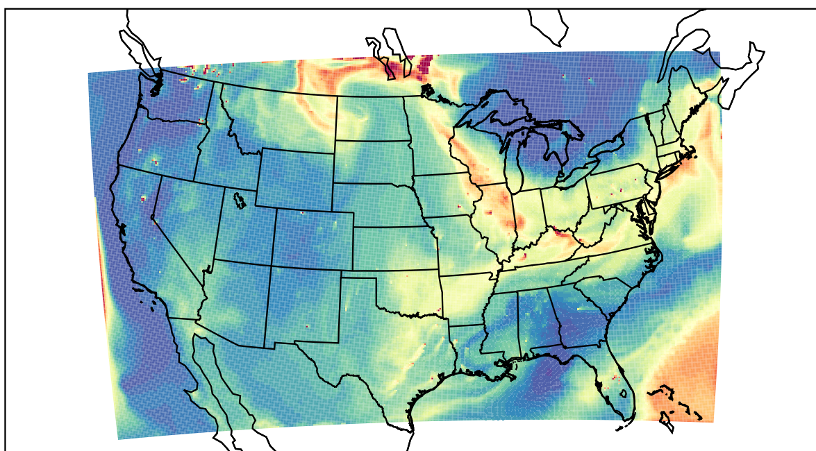
WRF 2021-07-21_20:00:00
