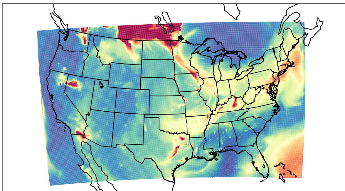
WRF 2021-07-21_11:00:00
