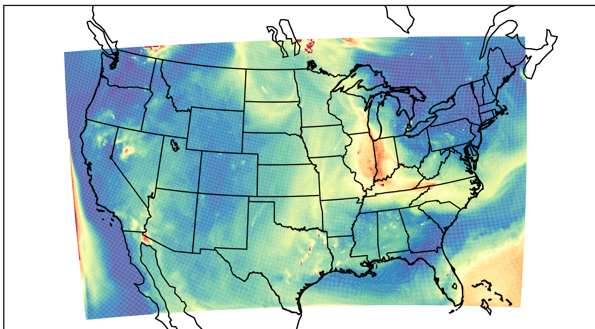
WRF 2021-07-22_18:00:00
