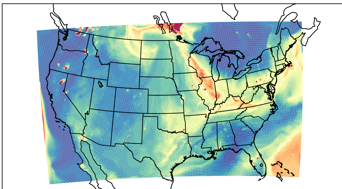
WRF 2021-07-21_23:00:00
