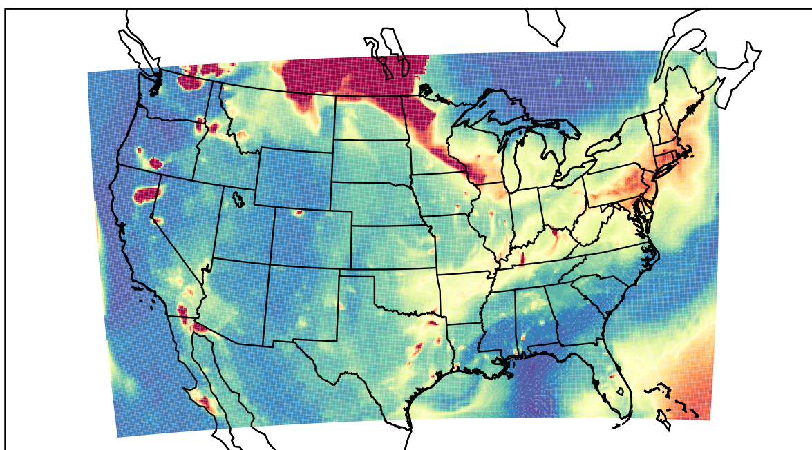
WRF 2021-07-21_04:00:00
