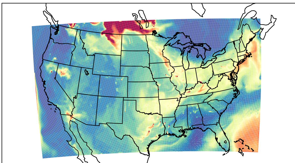
WRF 2021-07-21_15:00:00
