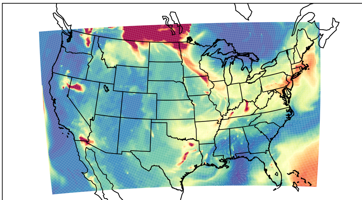
WRF 2021-07-21_10:00:00
