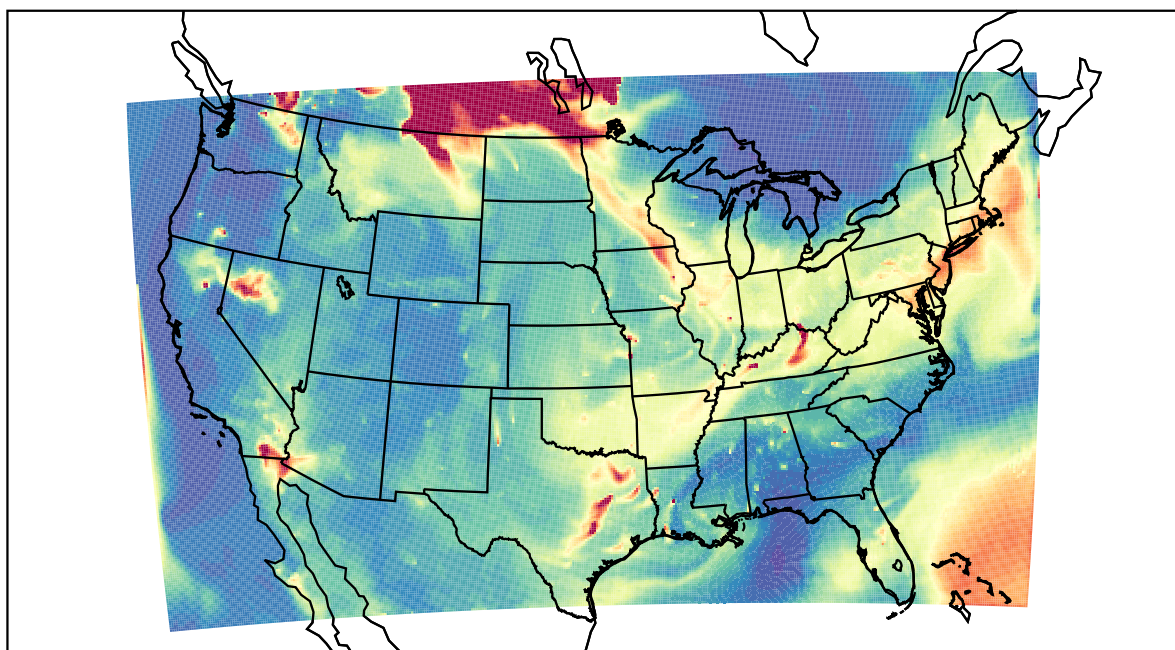
WRF 2021-07-21_13:00:00
