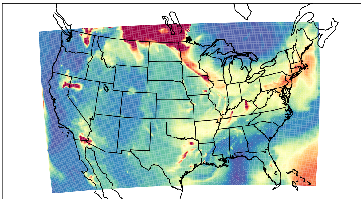
WRF 2021-07-21_08:00:00
