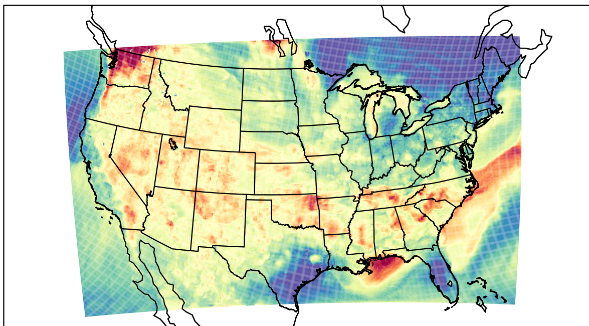
WRF (2021-08-01_03:00:00)
