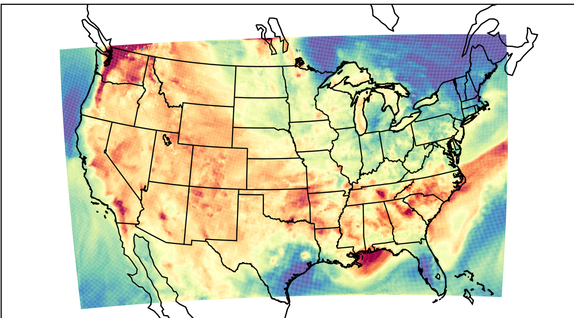
WRF (2021-08-01_01:00:00)
