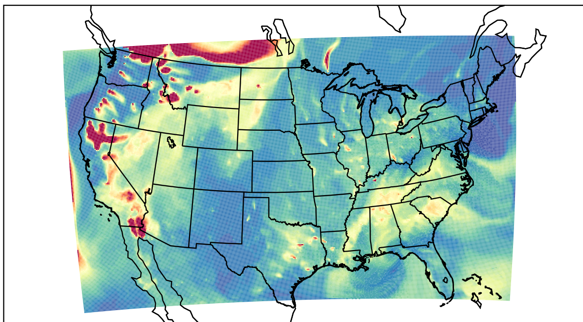
WRF 2021-08-17_04:00:00
