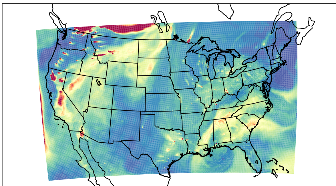
WRF 2021-08-17_00:00:00
