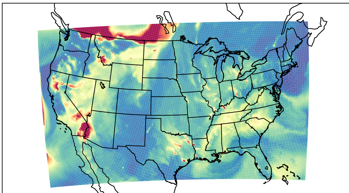
WRF 2021-08-17_08:00:00
