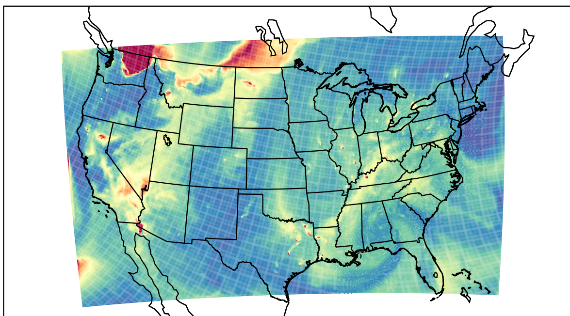
WRF 2021-08-17_16:00:00
