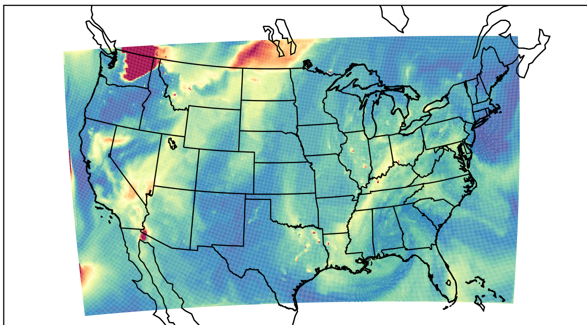
WRF 2021-08-17_18:00:00
