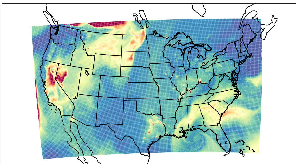
WRF 2021-08-16_18:00:00
