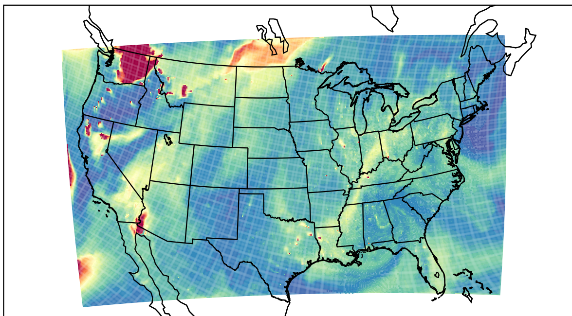
WRF 2021-08-17_23:00:00
