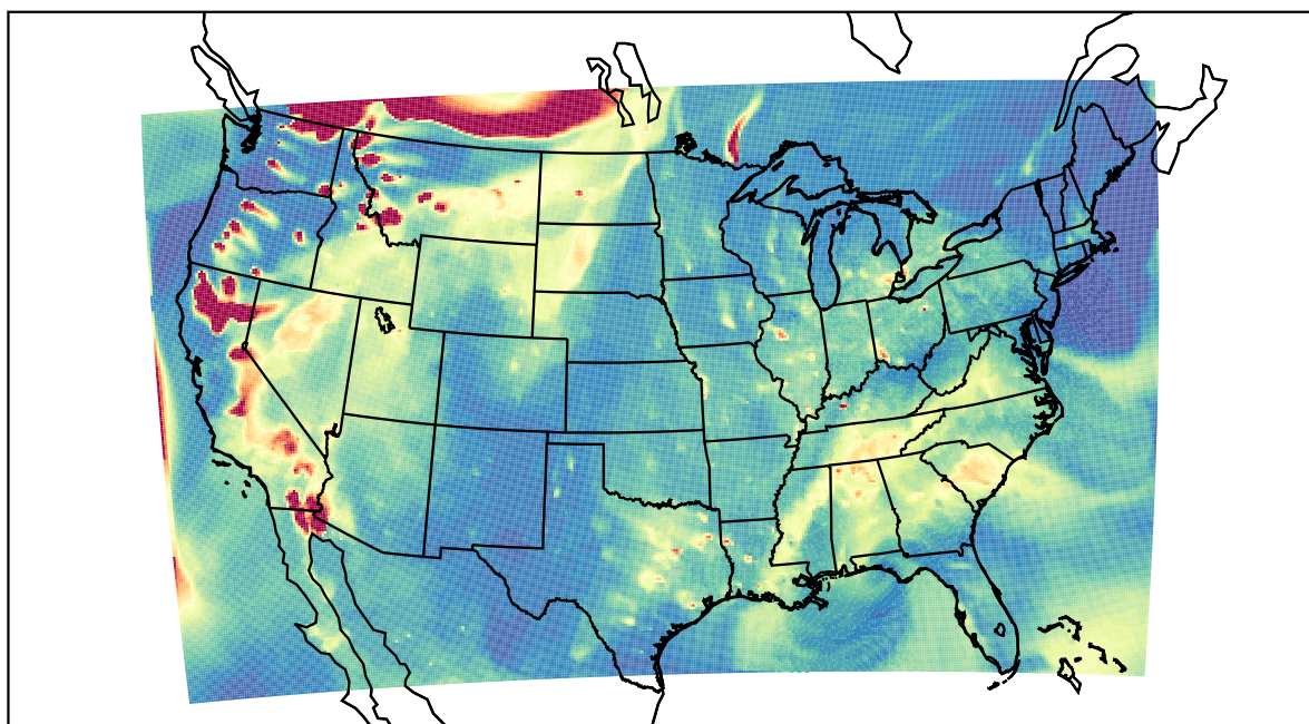
WRF 2021-08-17_03:00:00
