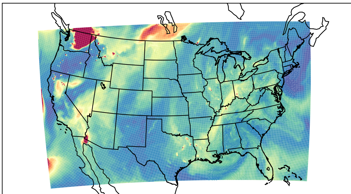
WRF 2021-08-17_20:00:00
