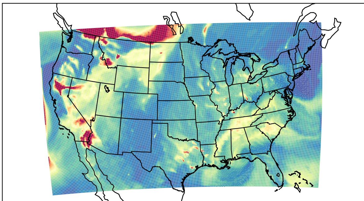
WRF 2021-08-17_06:00:00
