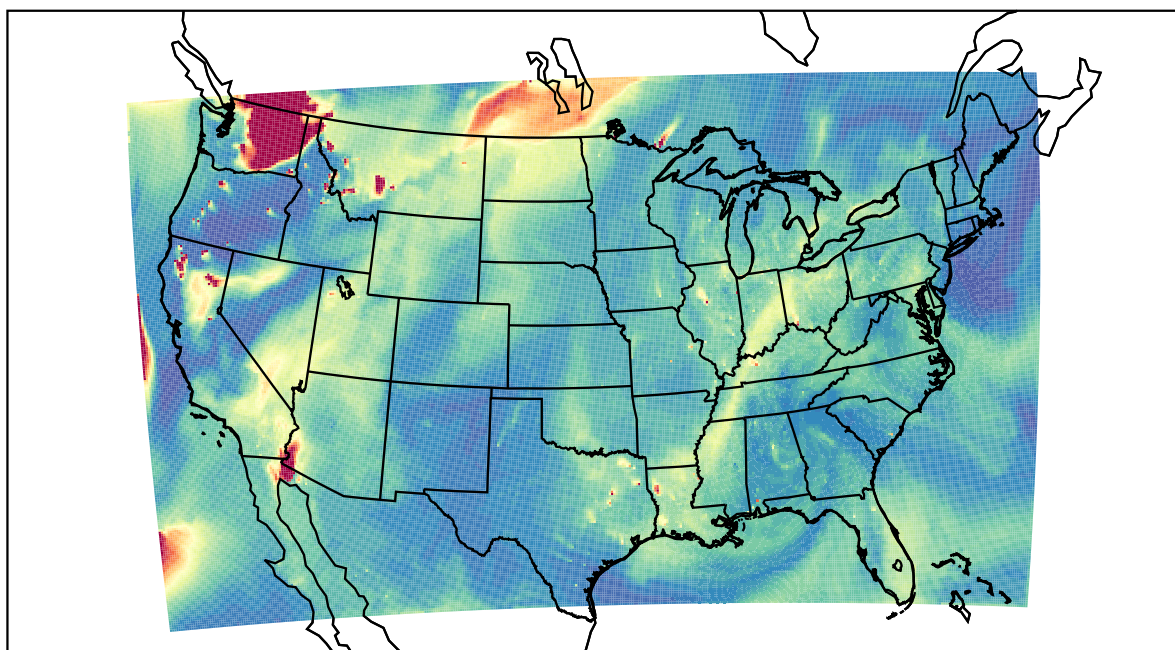
WRF 2021-08-17_22:00:00
