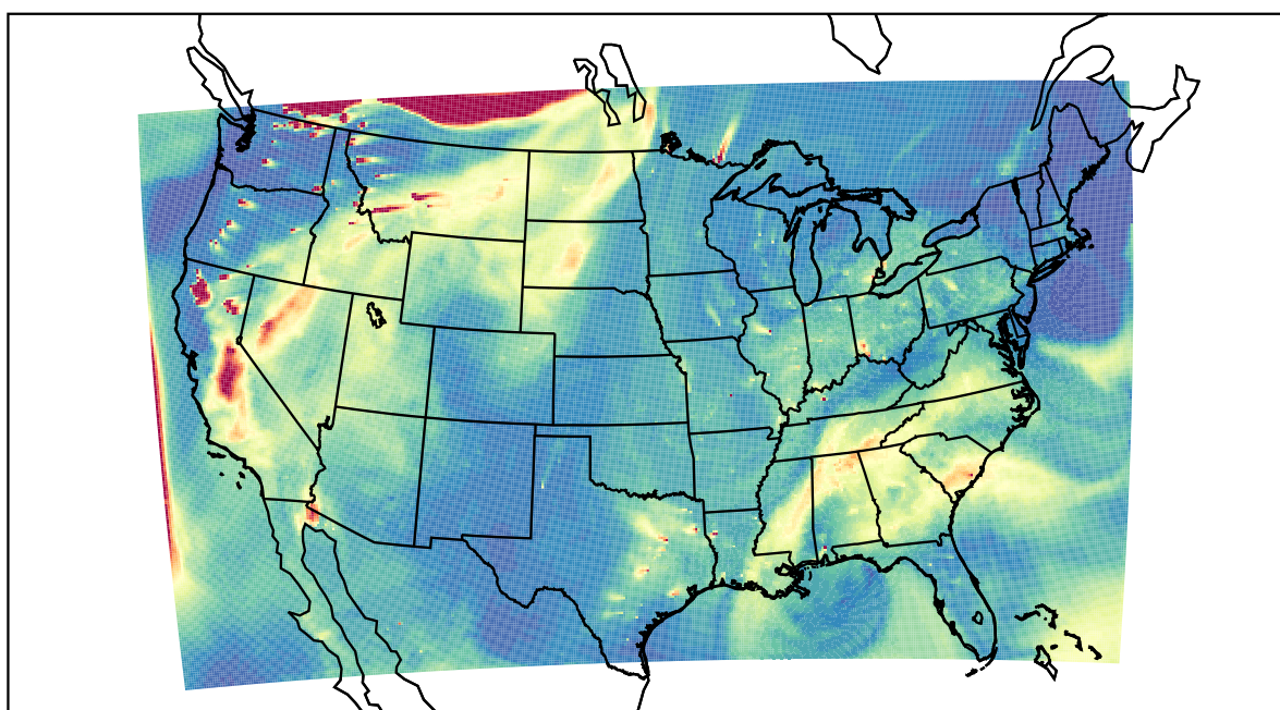
WRF 2021-08-16_23:00:00
