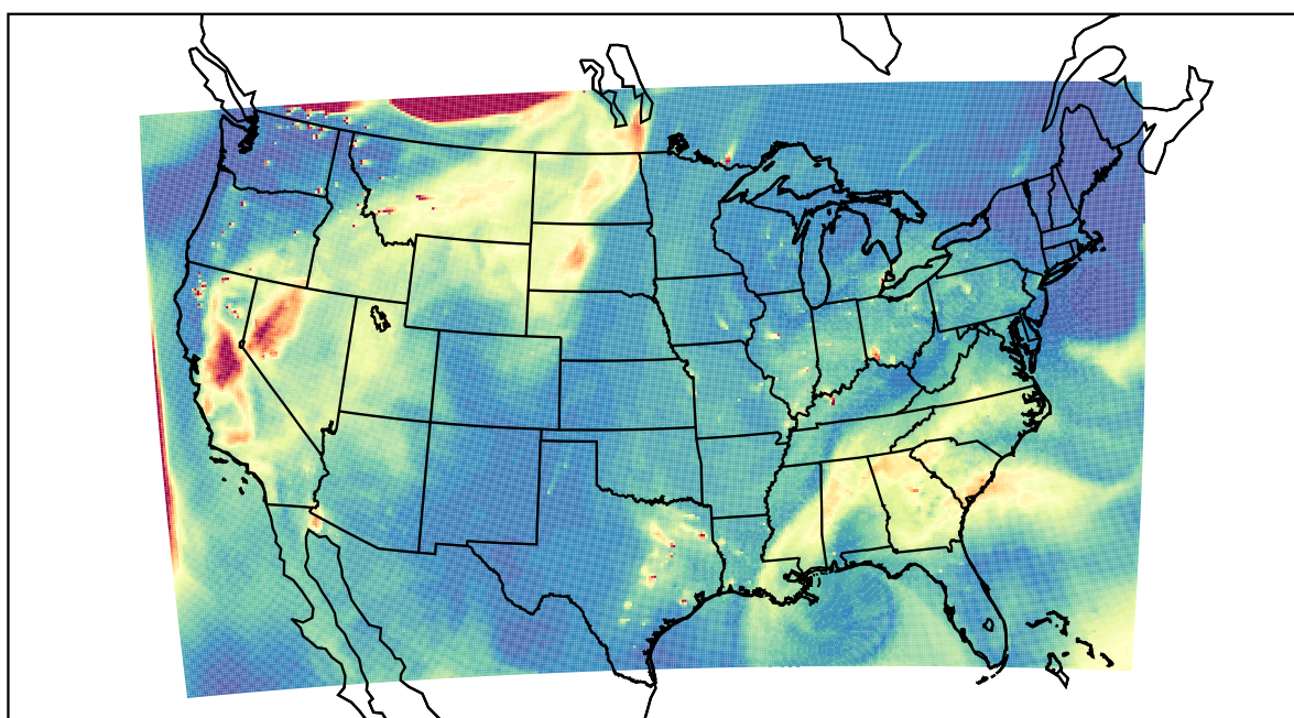
WRF 2021-08-16_20:00:00
