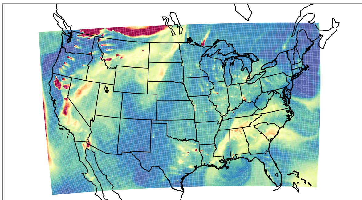
WRF 2021-08-17_01:00:00
