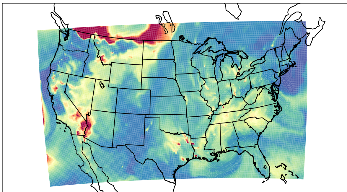
WRF 2021-08-17_10:00:00
