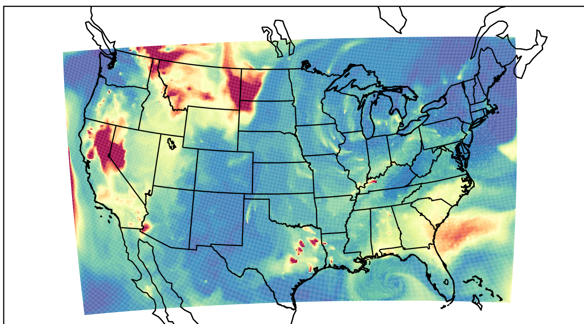
WRF 2021-08-16_10:00:00
