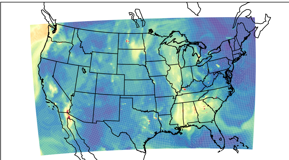
WRF 2021-10-01_17:00:00
