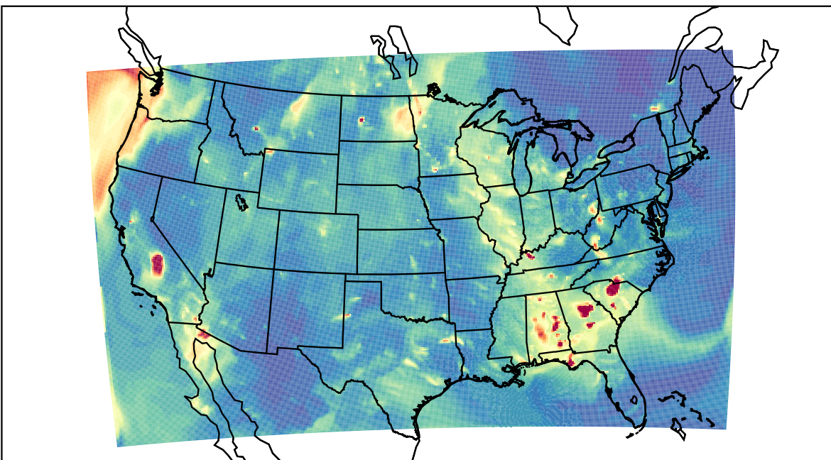
WRF 2021-10-01_04:00:00
