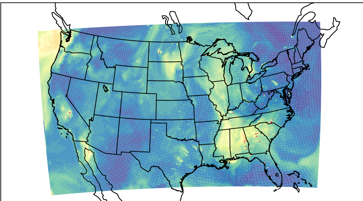
WRF 2021-10-01_20:00:00
