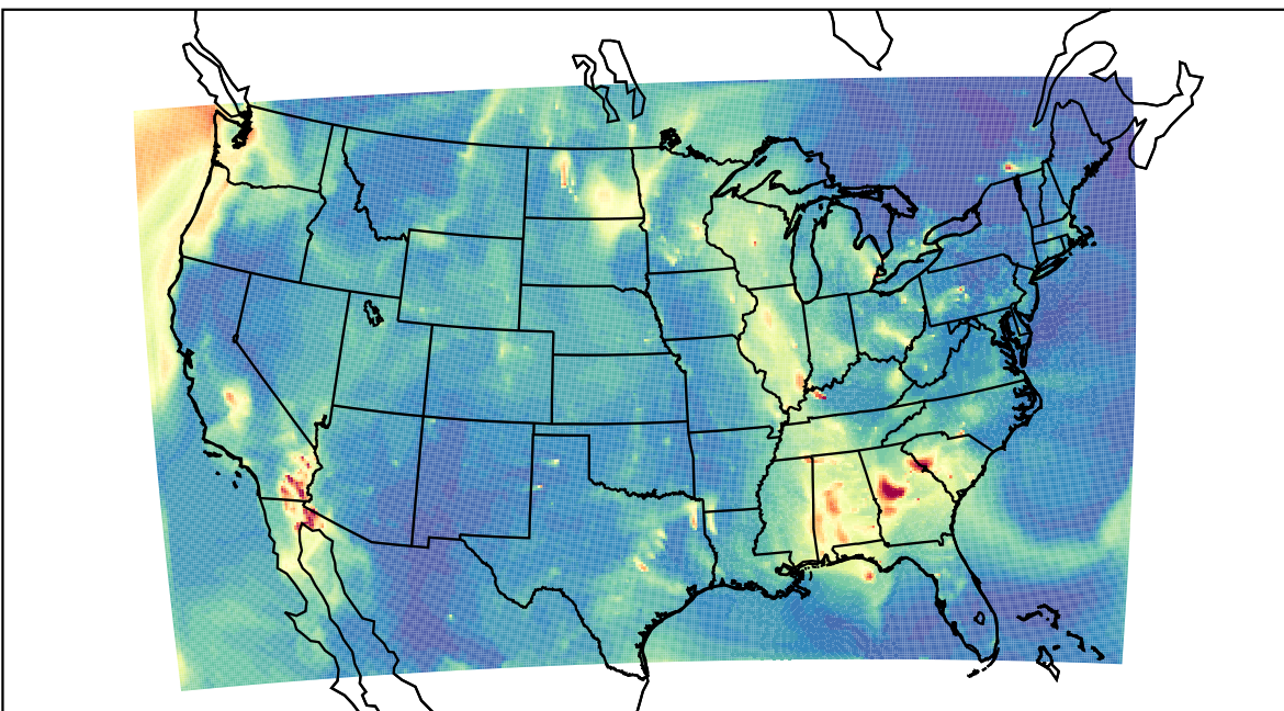
WRF 2021-10-01_11:00:00
