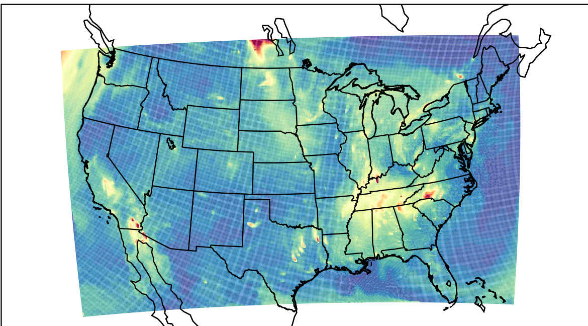
WRF 2021-10-02_13:00:00
