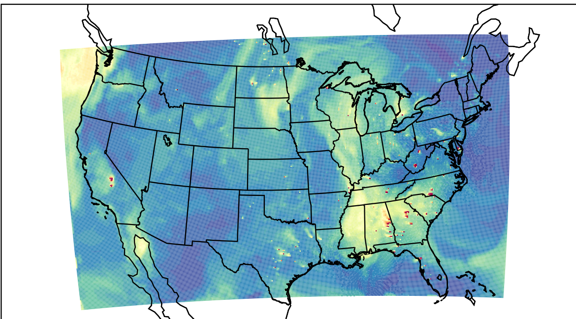
WRF 2021-10-01_22:00:00
