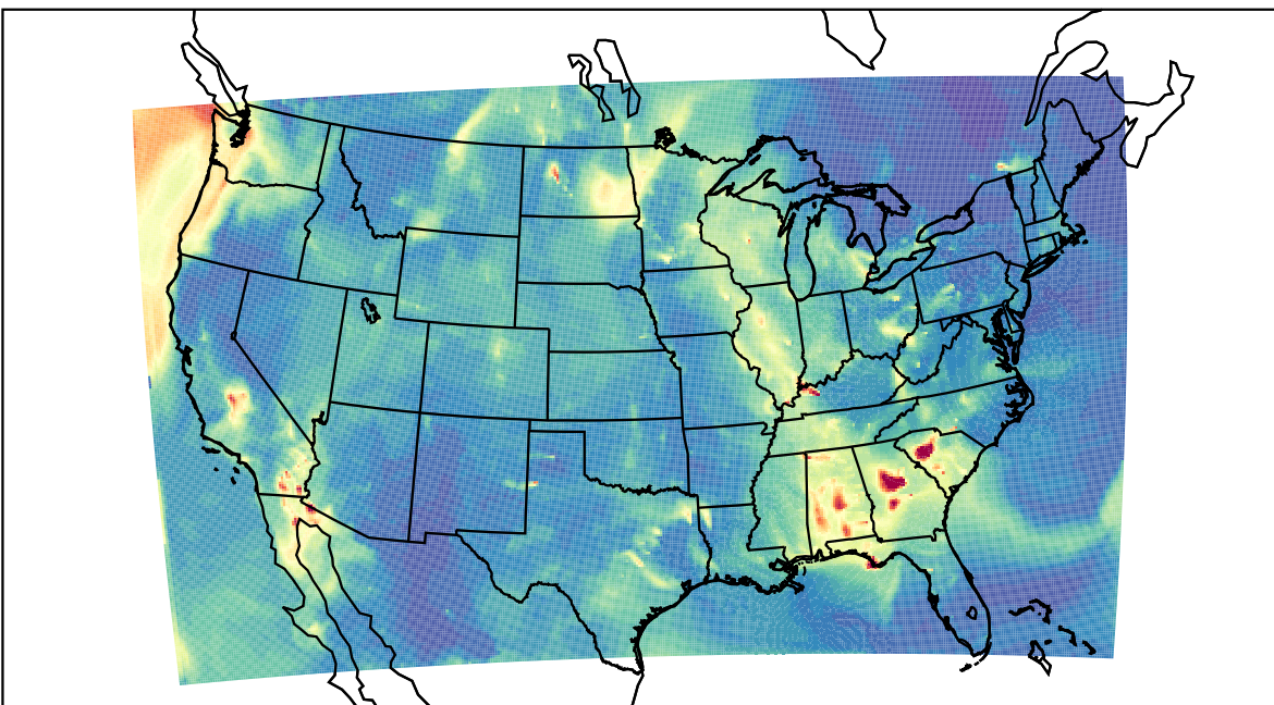
WRF 2021-10-01_08:00:00
