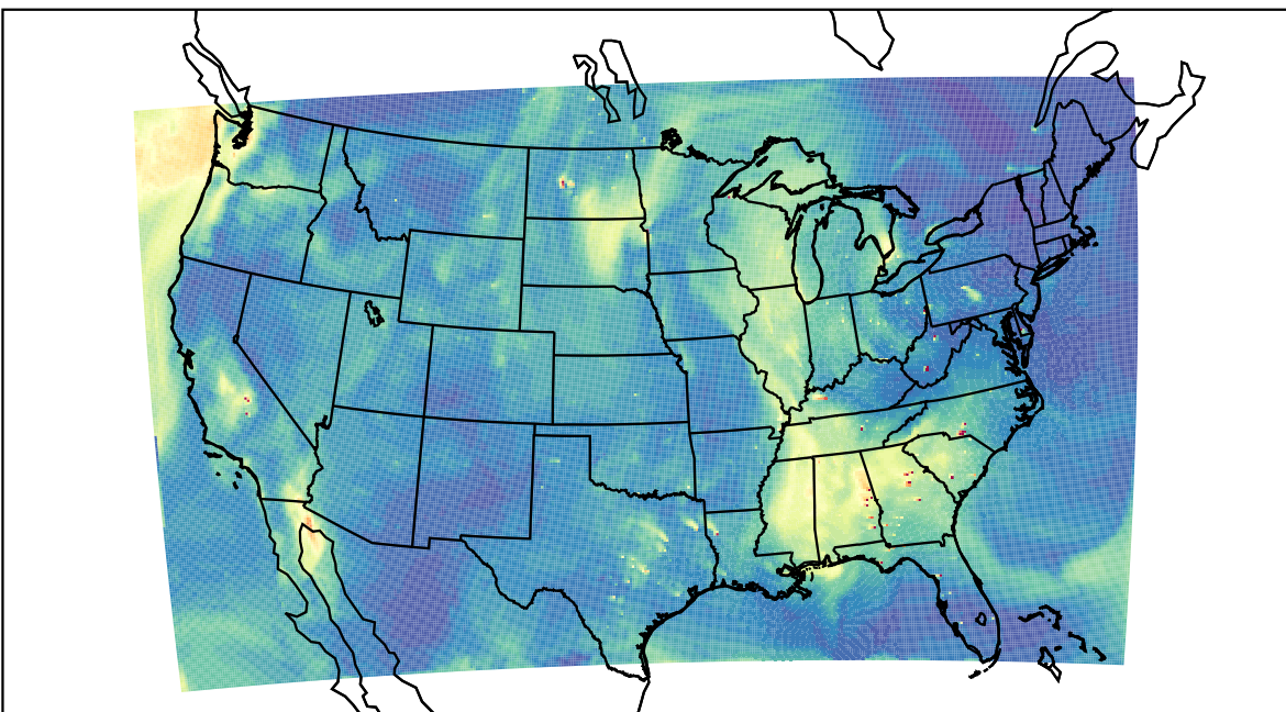
WRF 2021-10-01_19:00:00
