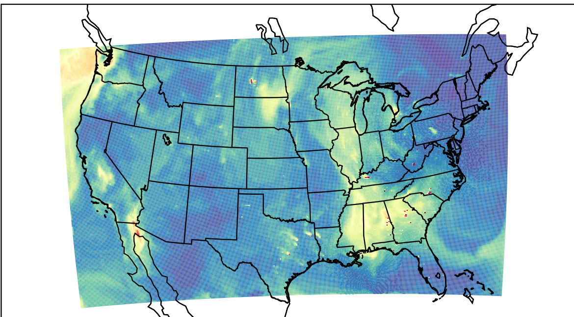
WRF 2021-10-01_18:00:00
