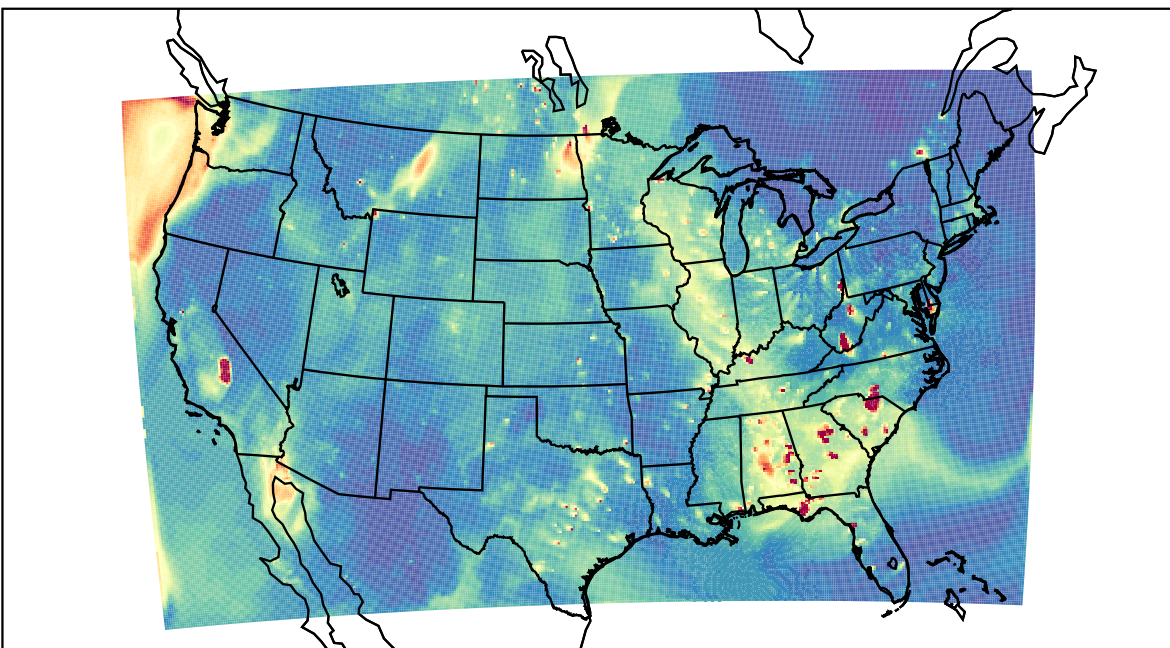
WRF 2021-10-01_01:00:00
