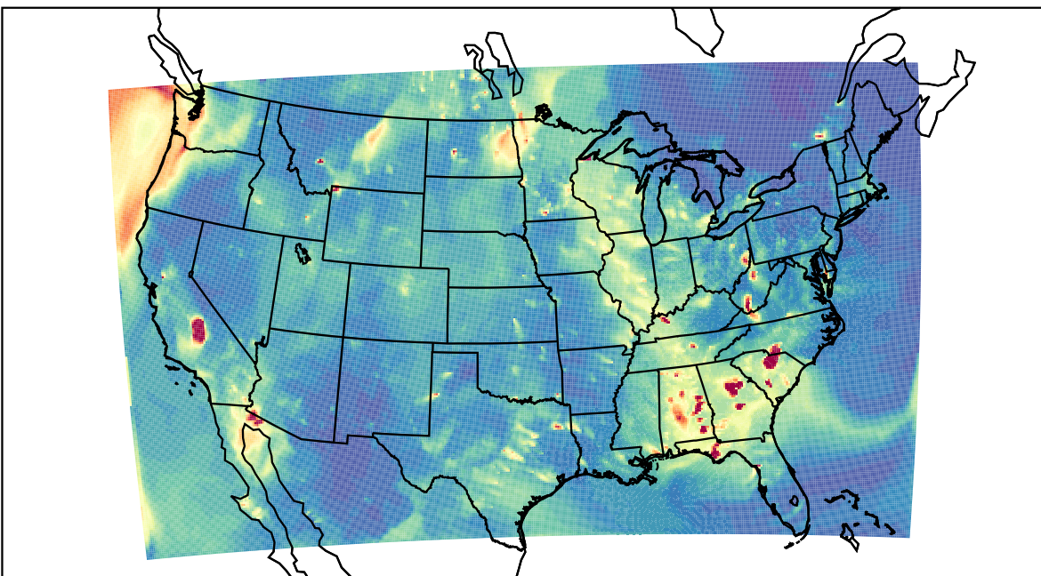
WRF 2021-10-01_03:00:00
