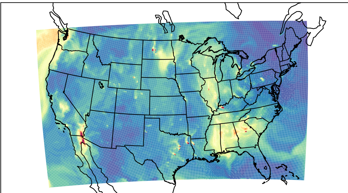
WRF 2021-10-01_16:00:00
