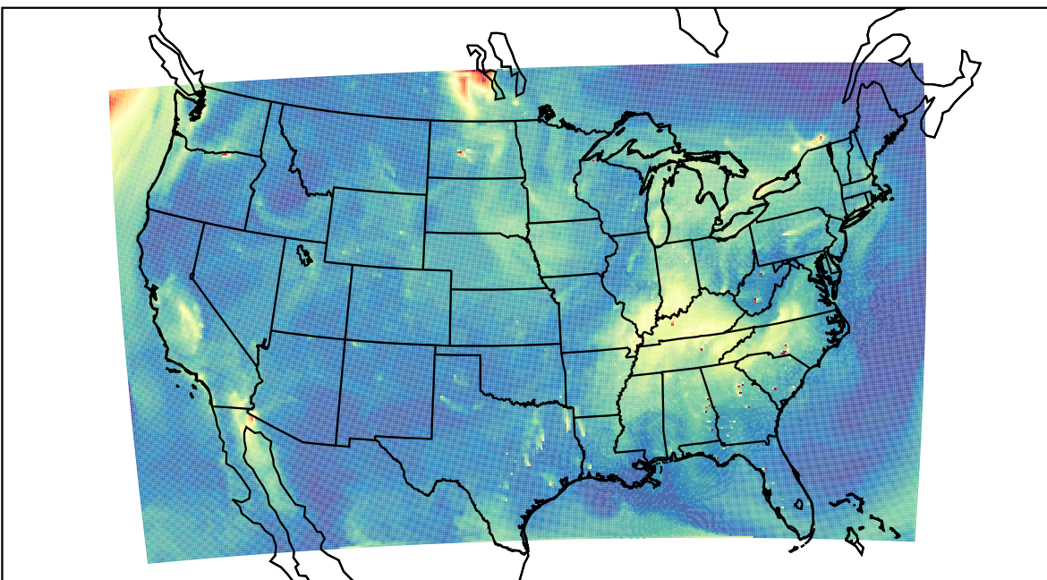
WRF 2021-10-02_18:00:00
