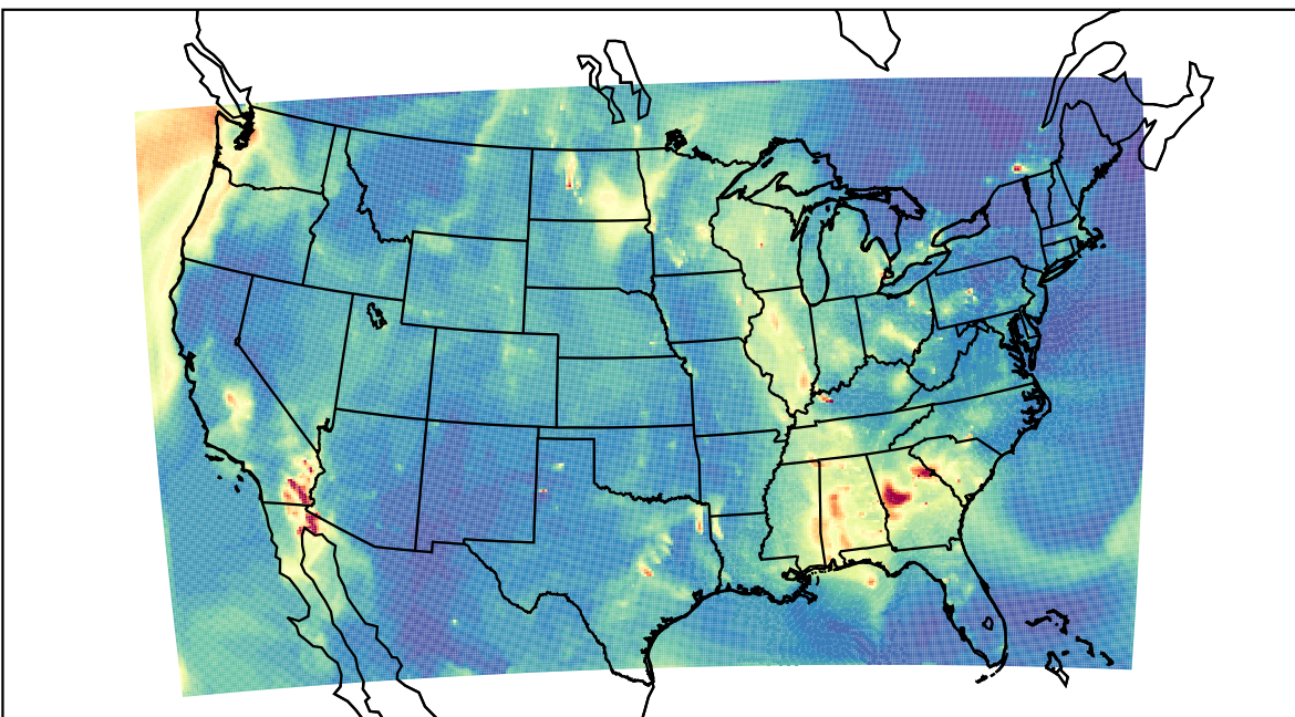
WRF 2021-10-01_12:00:00
