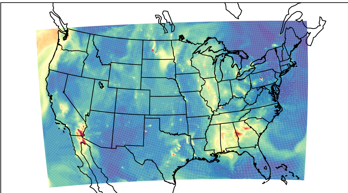
WRF 2021-10-01_14:00:00
