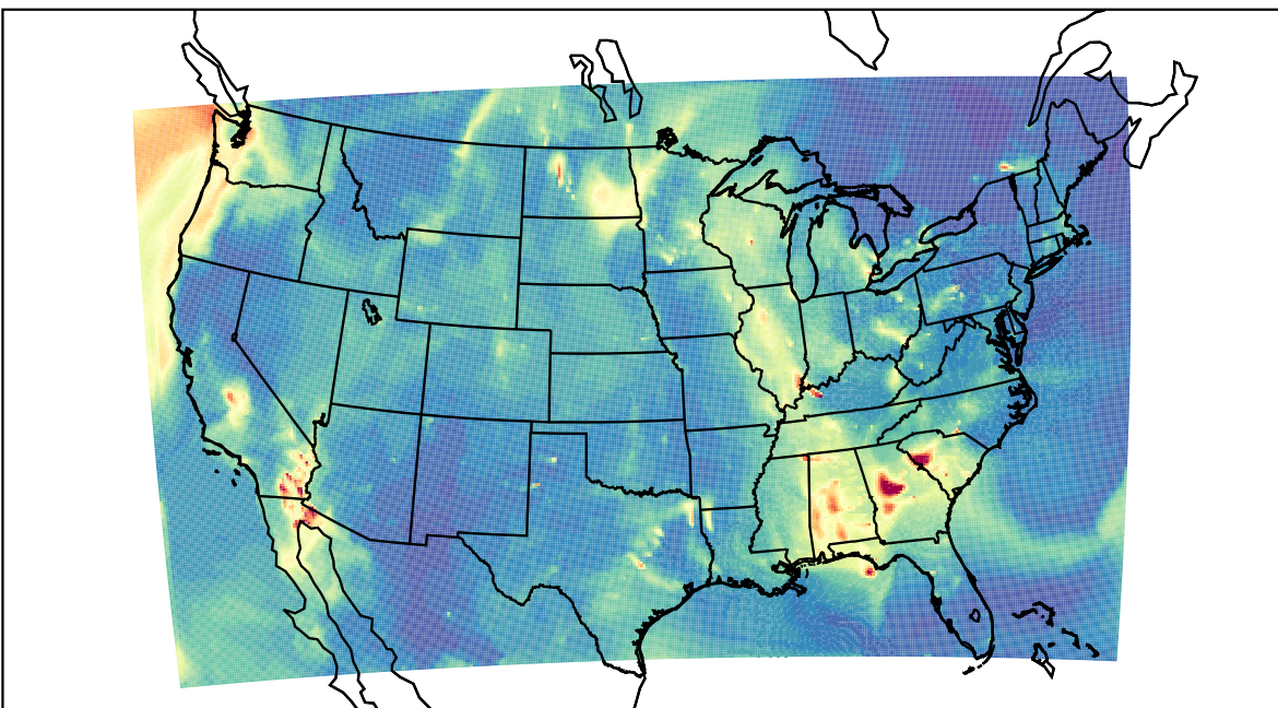
WRF 2021-10-01_10:00:00
