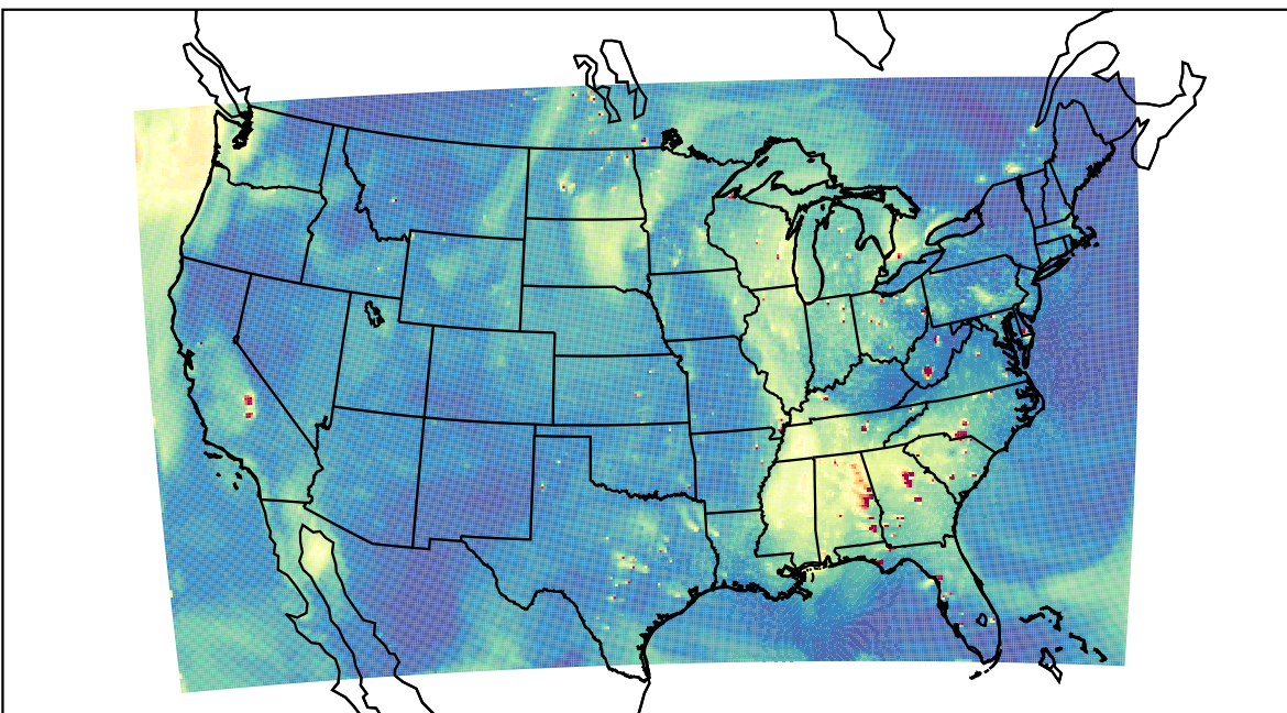
WRF 2021-10-01_23:00:00
