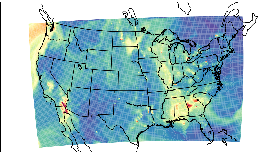
WRF 2021-10-01_13:00:00
