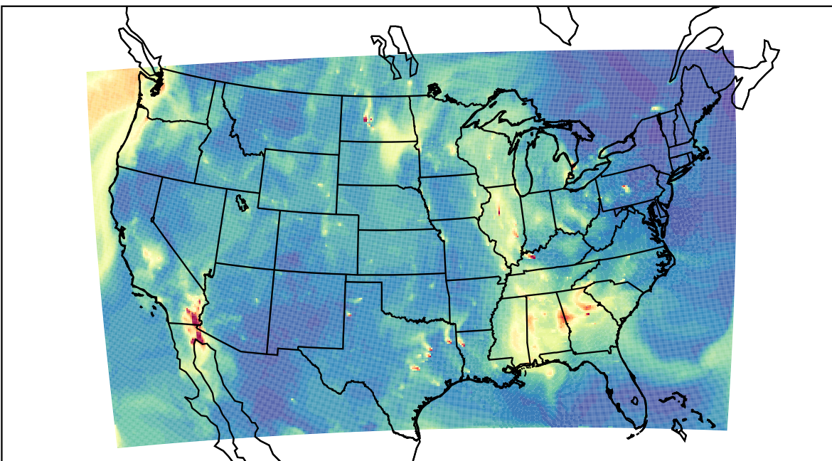
WRF 2021-10-01_15:00:00
