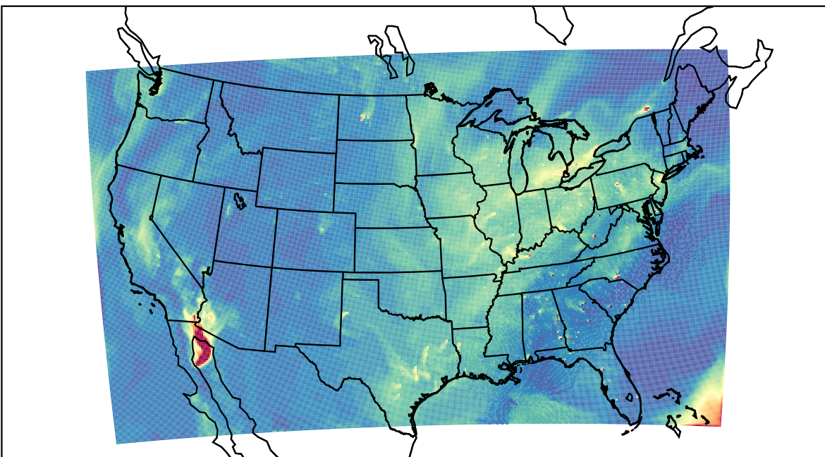
WRF 2021-10-05_18:00:00
