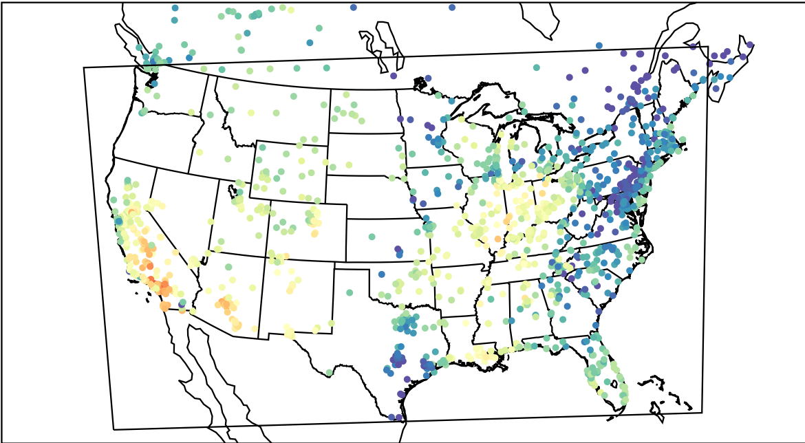
AirNOW (2021-10-10_22:00:00)
