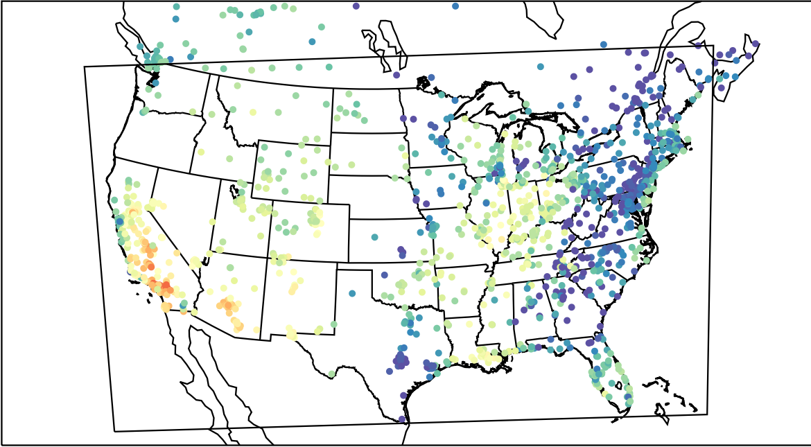
AirNOW (2021-10-10_23:00:00)
