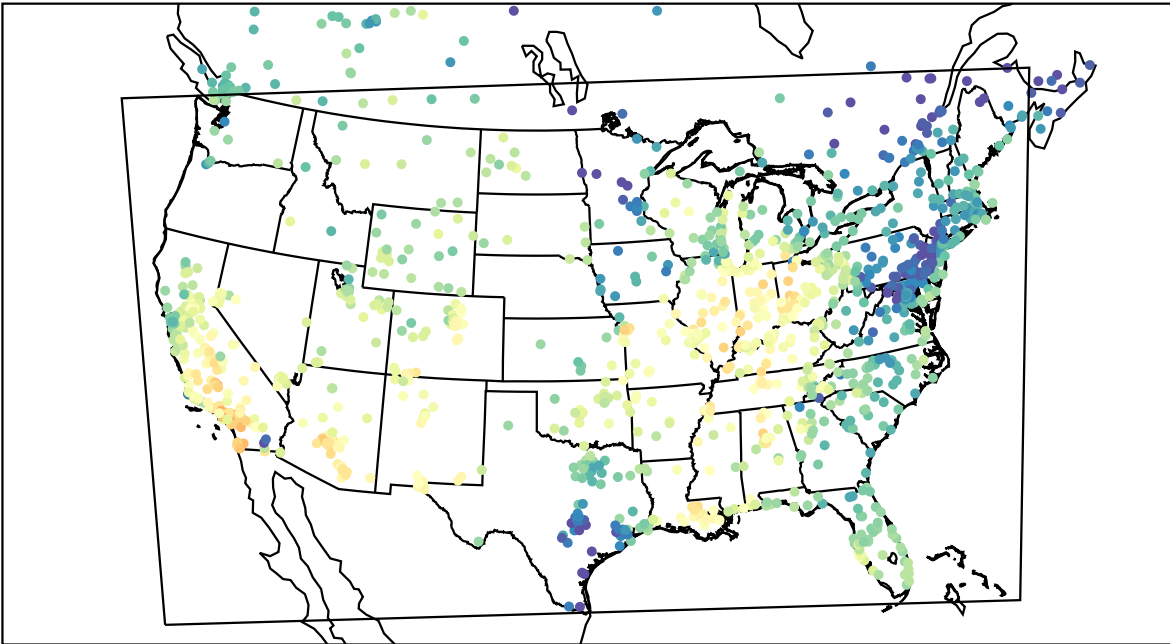
AirNOW (2021-10-10_20:00:00)
