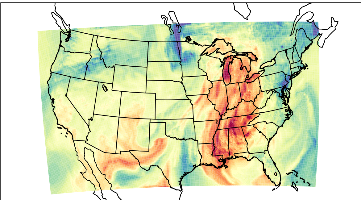
WRF (2021-10-10_22:00:00)
