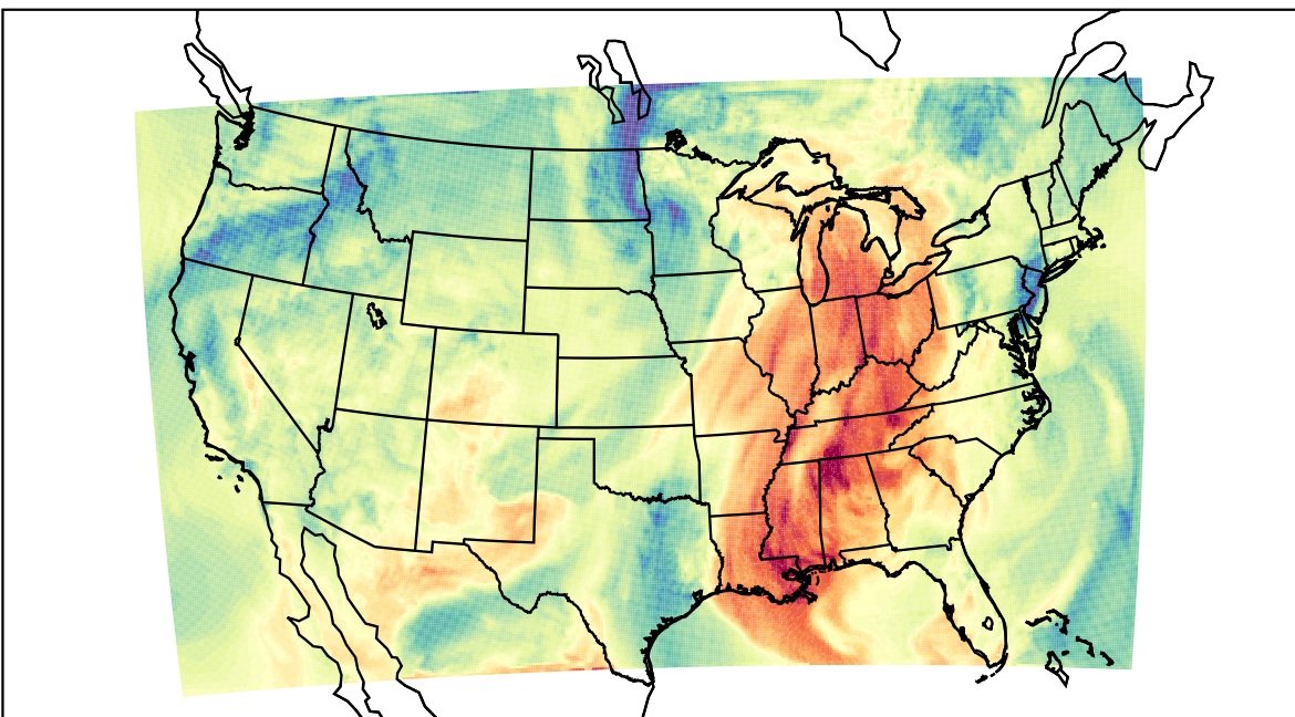
WRF (2021-10-10_18:00:00)
