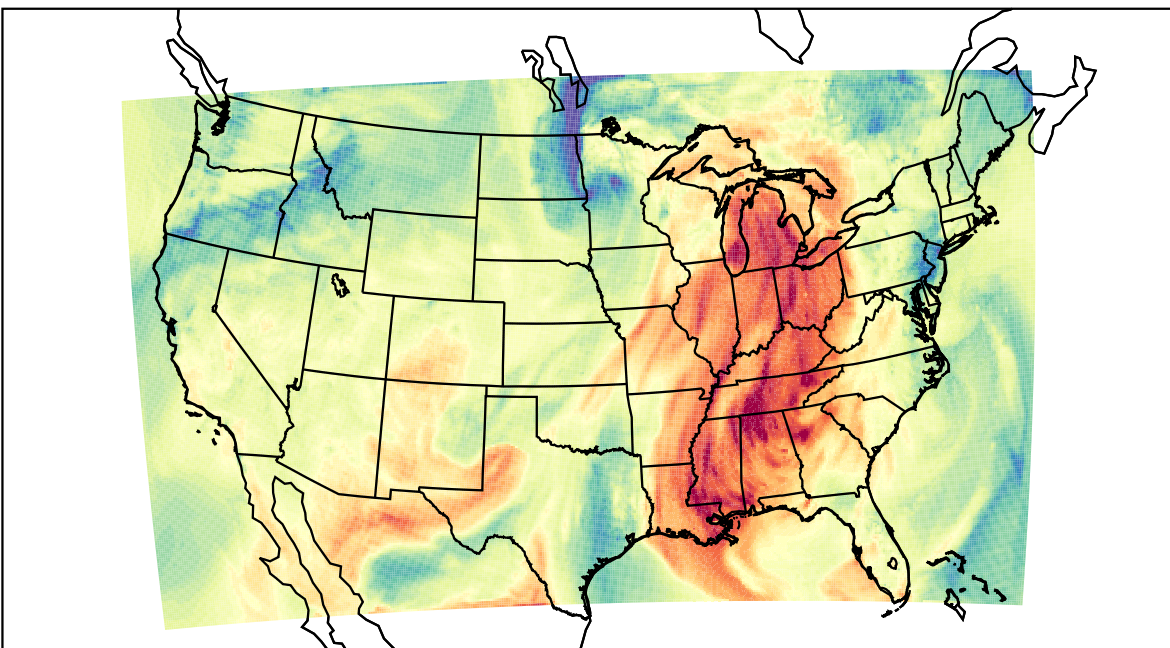
WRF (2021-10-10_20:00:00)
