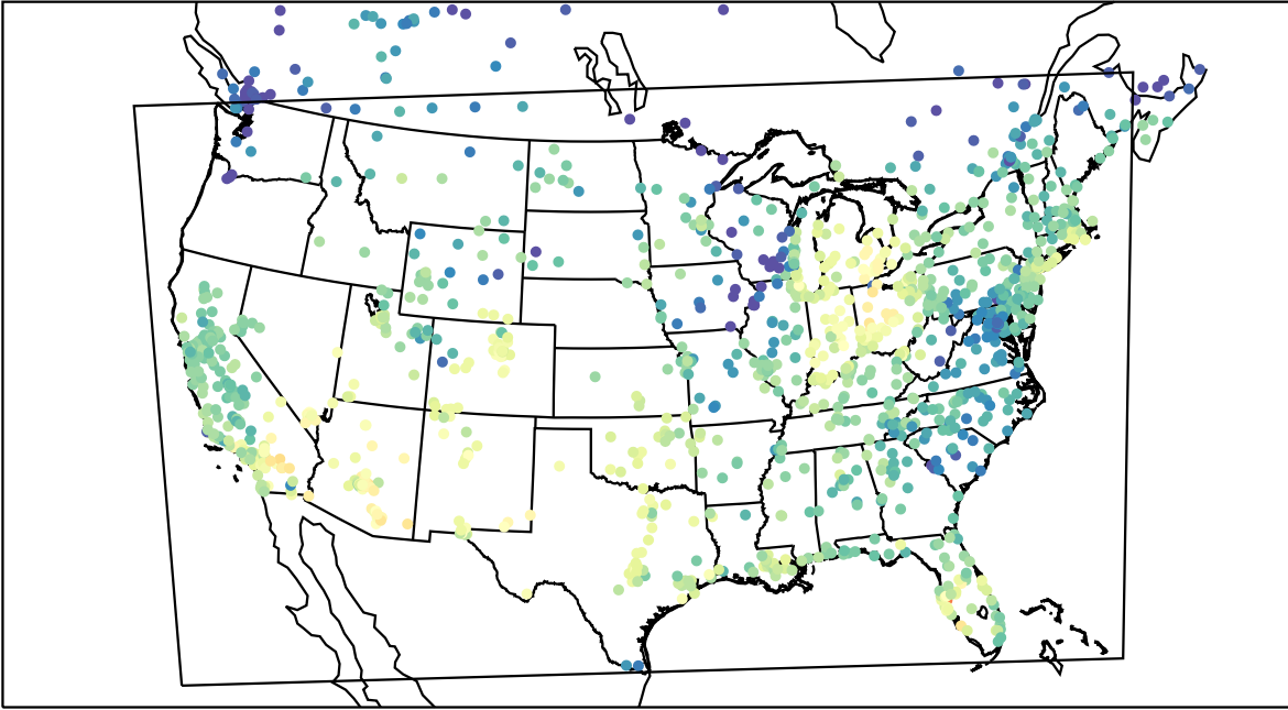
AirNOW (2021-10-11_18:00:00)
