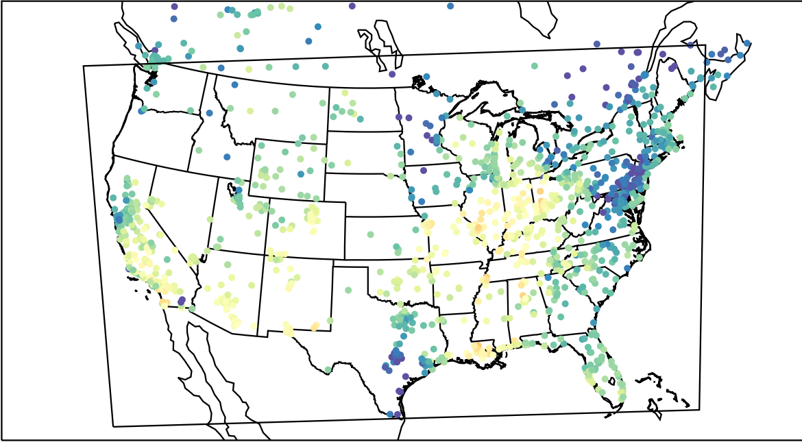
AirNOW (2021-10-10_18:00:00)
