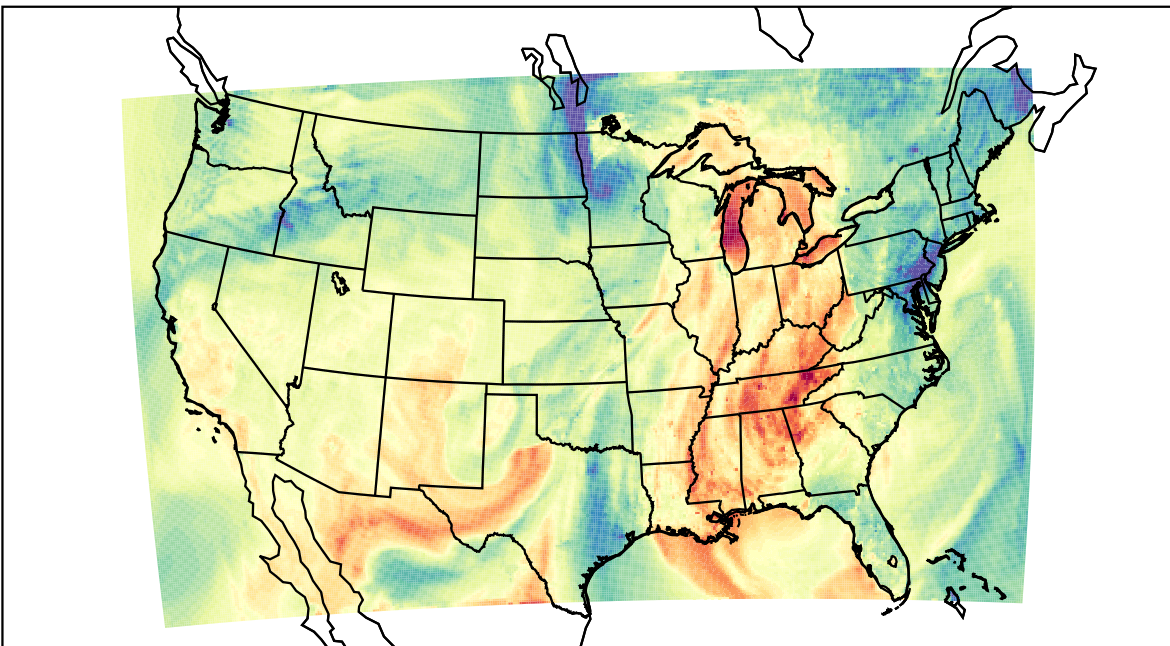
WRF (2021-10-10_23:00:00)
