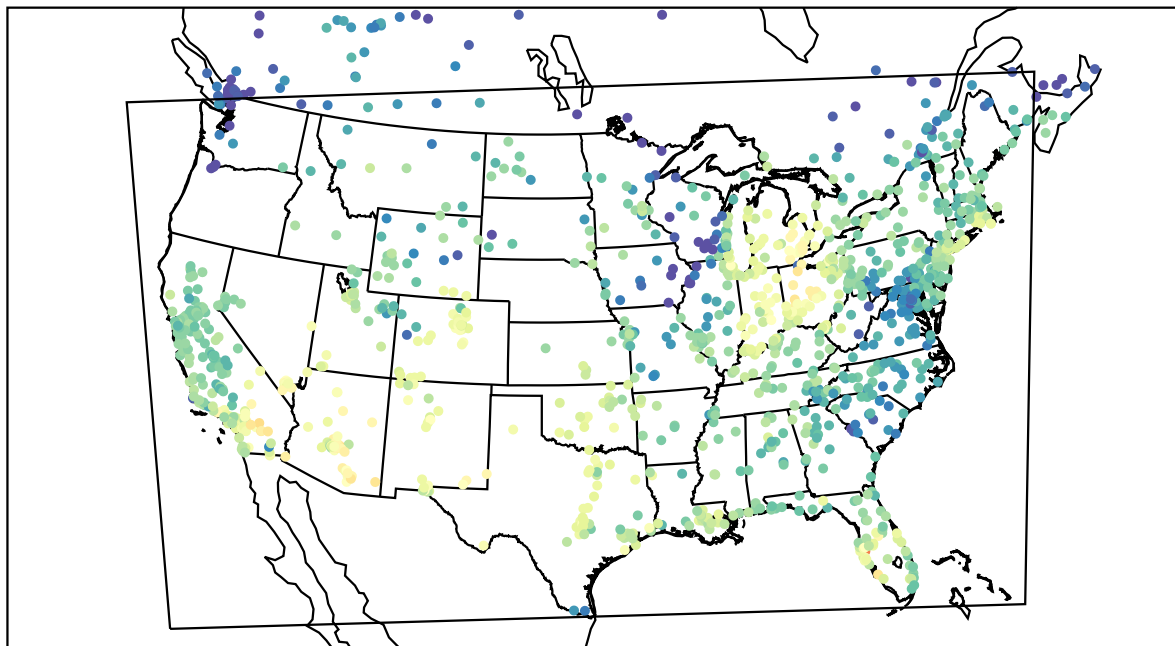
AirNOW (2021-10-11_18:00:00)
