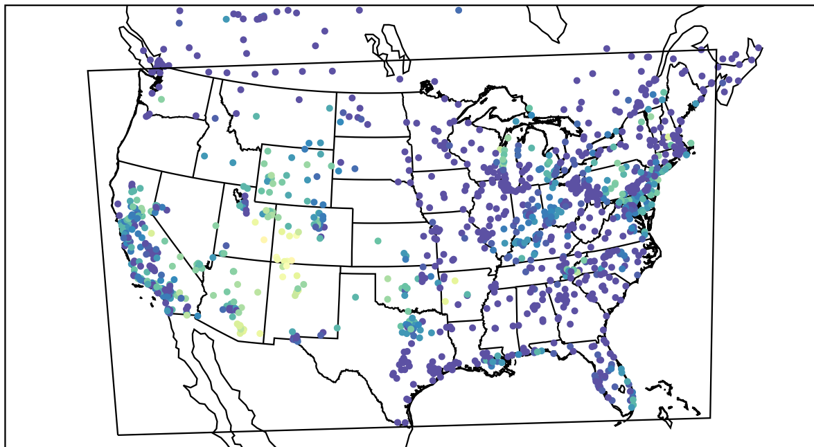
AirNOW (2021-10-12_13:00:00)
