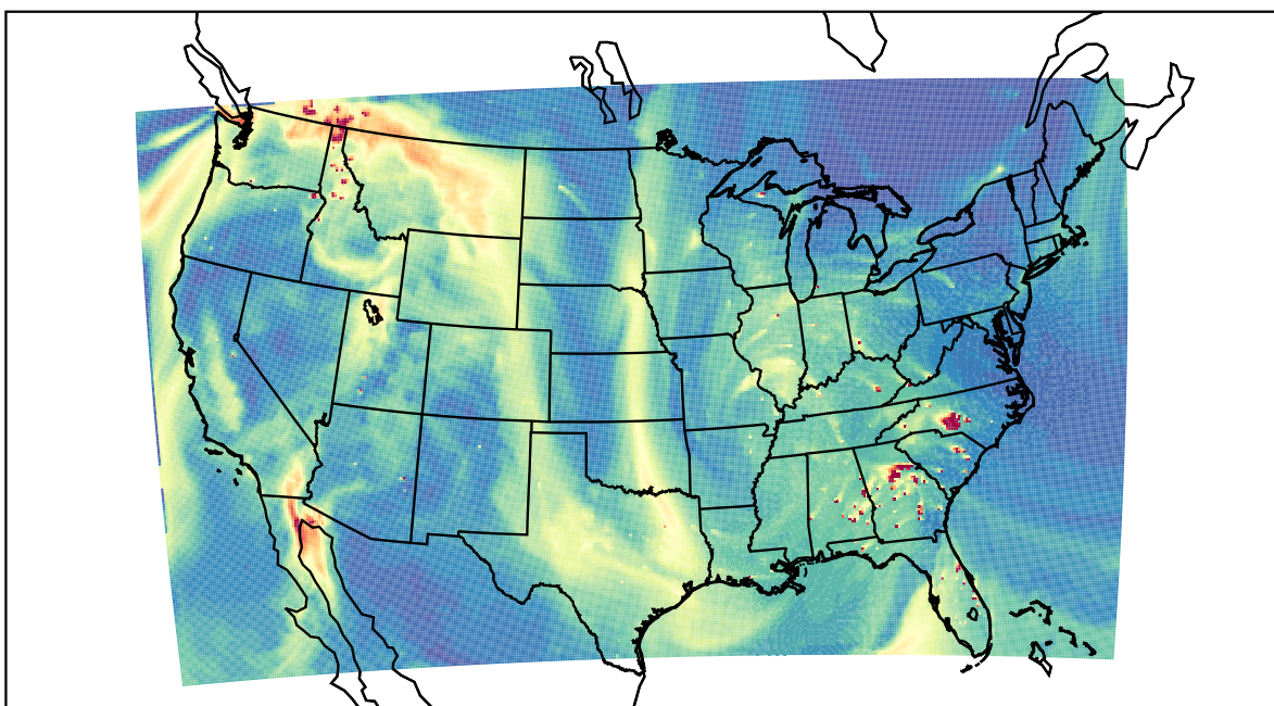
WRF 2021-10-28_20:00:00
