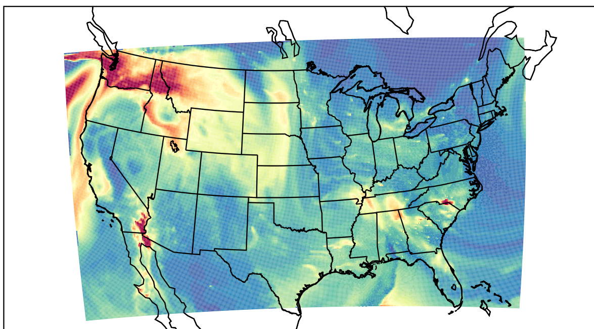
WRF 2021-10-28_10:00:00
