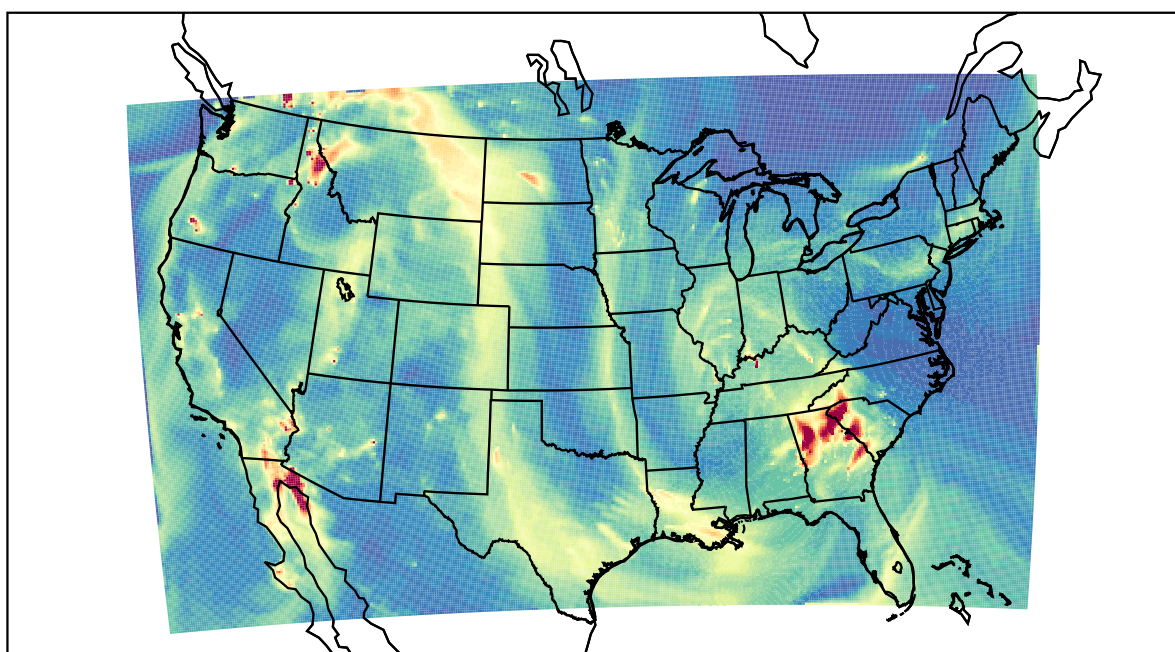
WRF 2021-10-29_04:00:00
