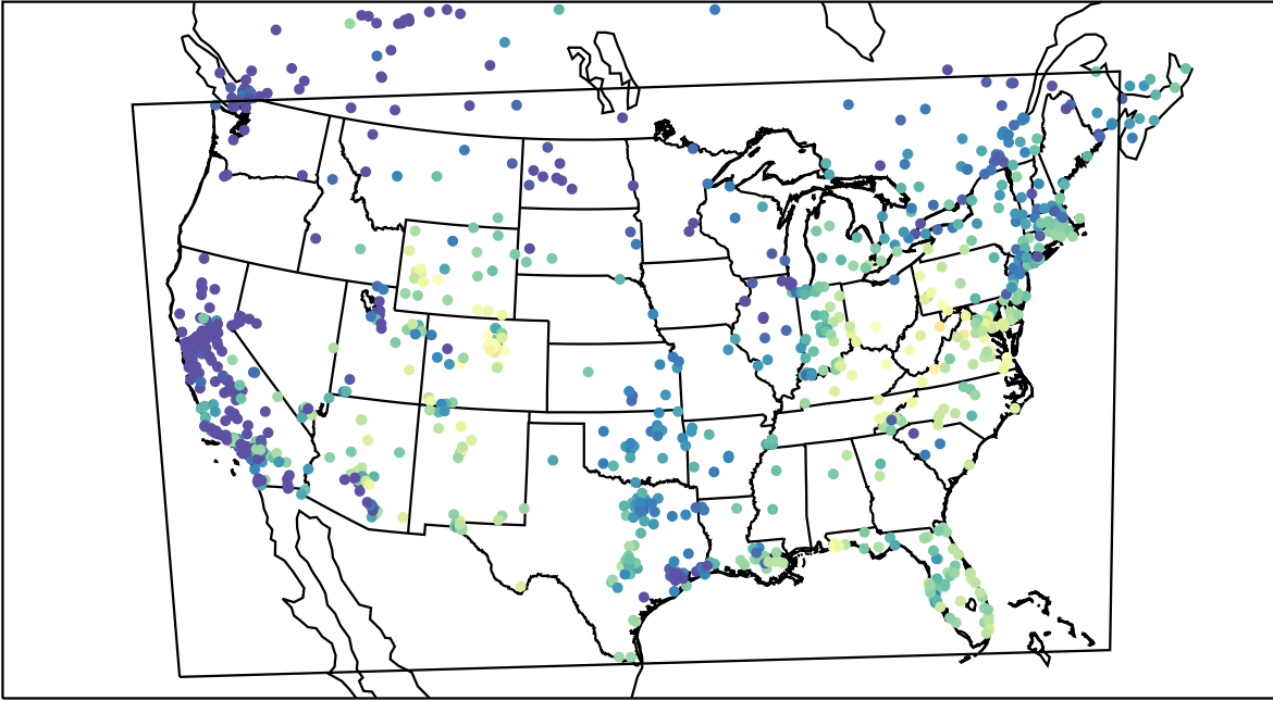
AirNOW (2021-11-11_16:00:00)
