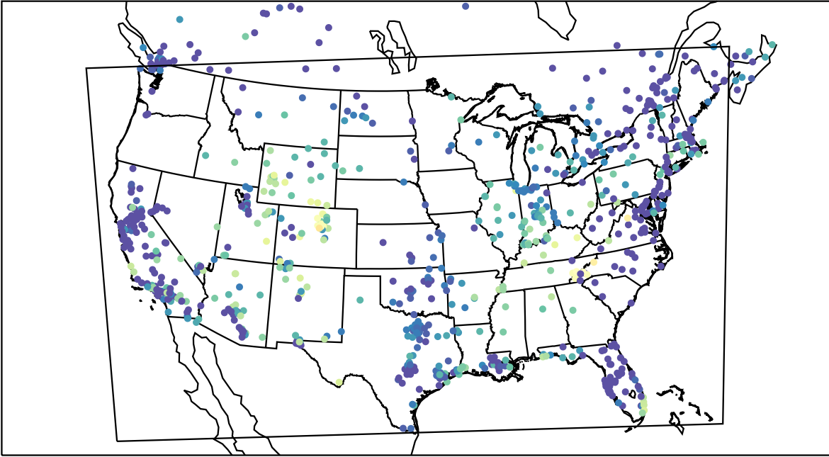
AirNOW (2021-11-11_10:00:00)
