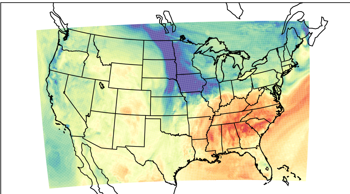
WRF (2021-11-10_20:00:00)
