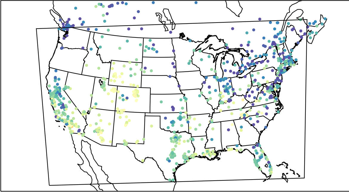
AirNOW (2021-11-10_23:00:00)
