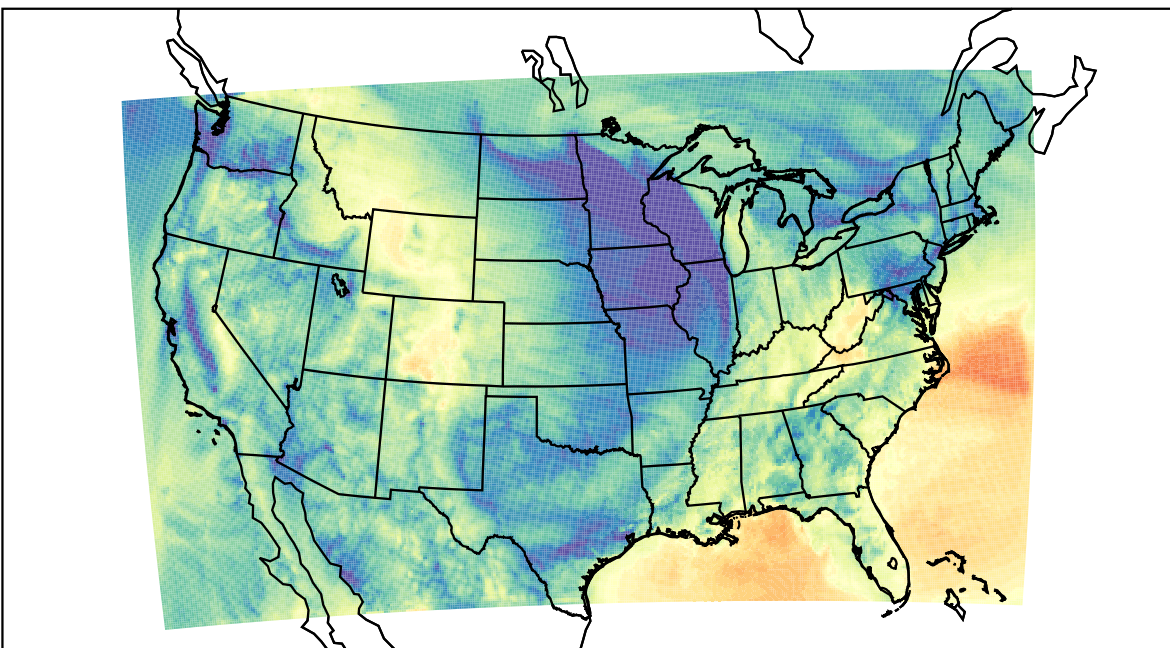
WRF (2021-11-11_15:00:00)
