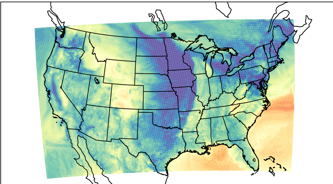
WRF (2021-11-11_10:00:00)
