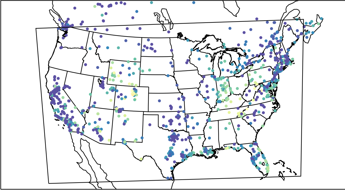
AirNOW (2021-11-11_14:00:00)
