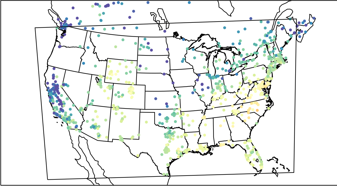
AirNOW (2021-11-10_18:00:00)
