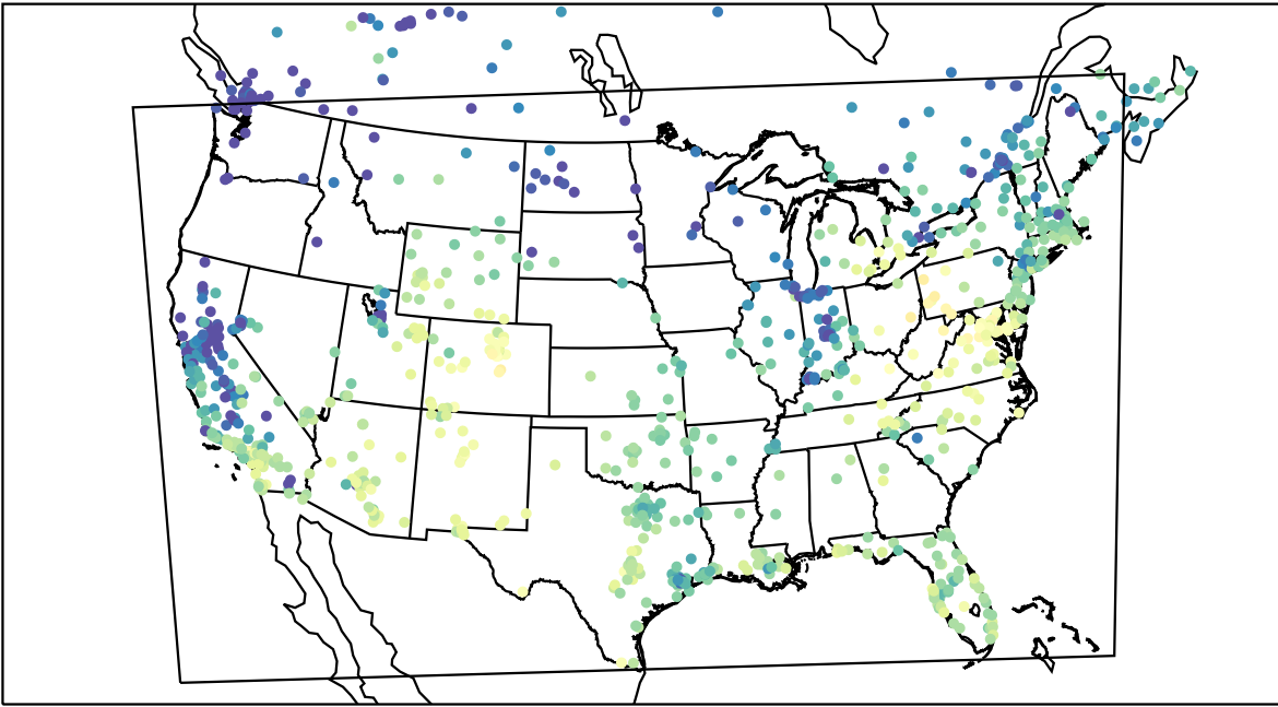
AirNOW (2021-11-11_19:00:00)
