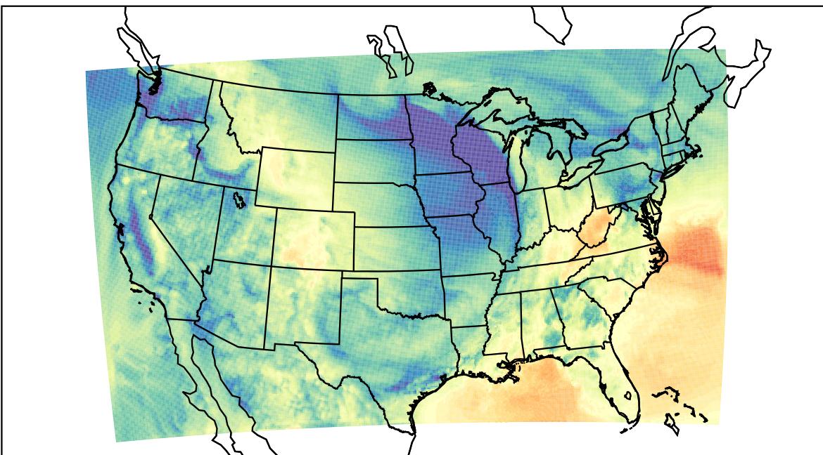
WRF (2021-11-11_16:00:00)
