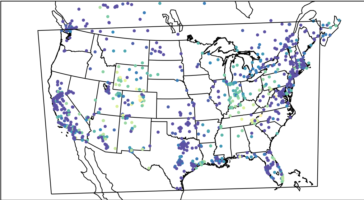
AirNOW (2021-11-11_13:00:00)
