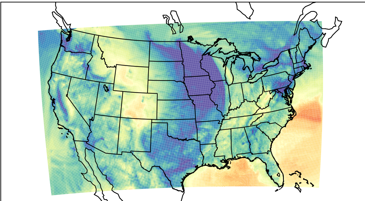
WRF (2021-11-11_14:00:00)
