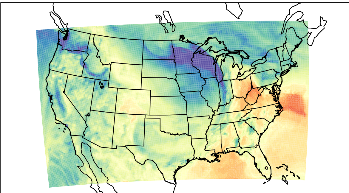
WRF (2021-11-11_18:00:00)
