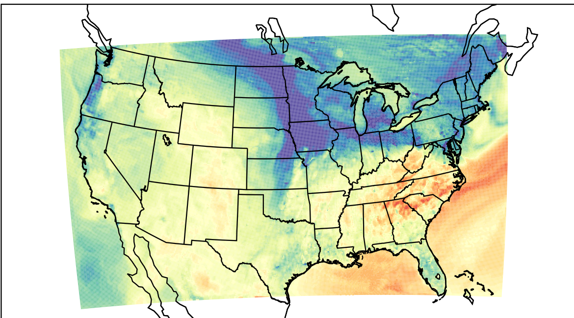
WRF (2021-11-10_23:00:00)
