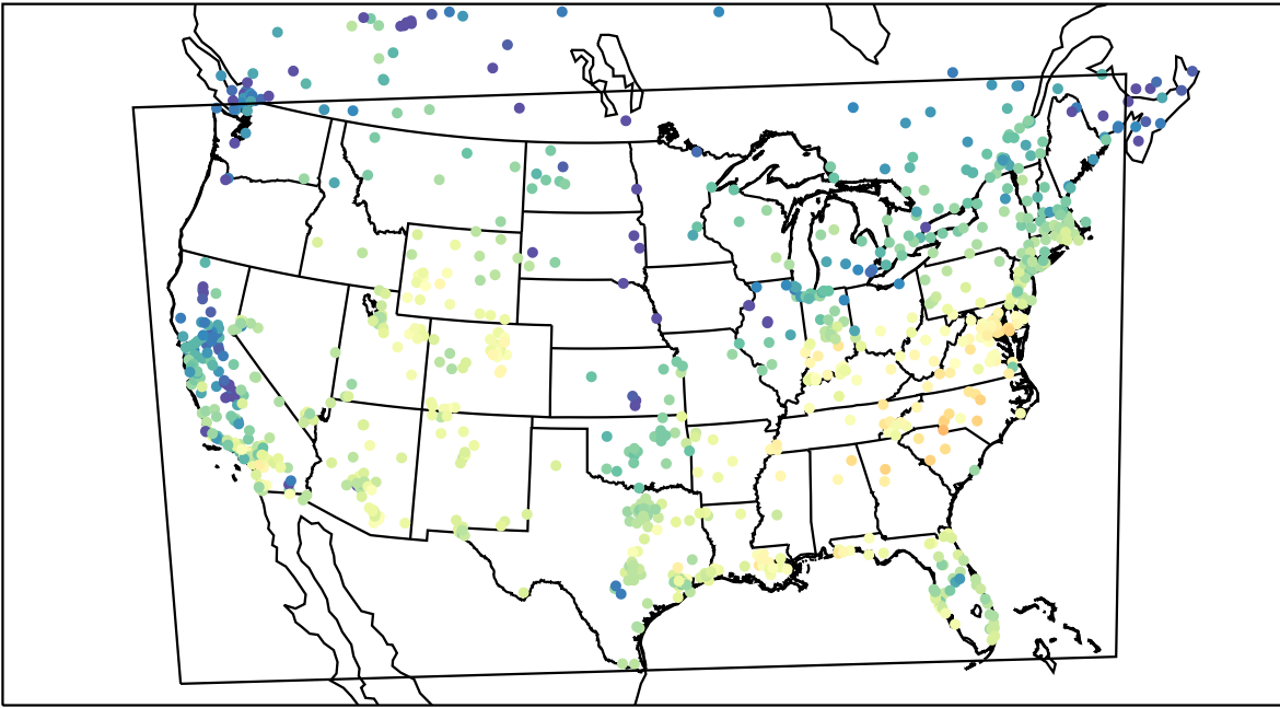
AirNOW (2021-11-10_20:00:00)
