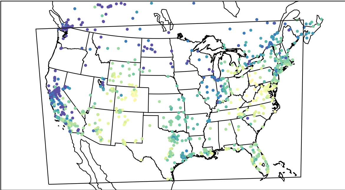
AirNOW (2021-11-11_18:00:00)
