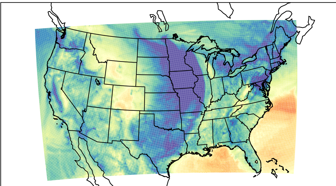
WRF (2021-11-11_13:00:00)
