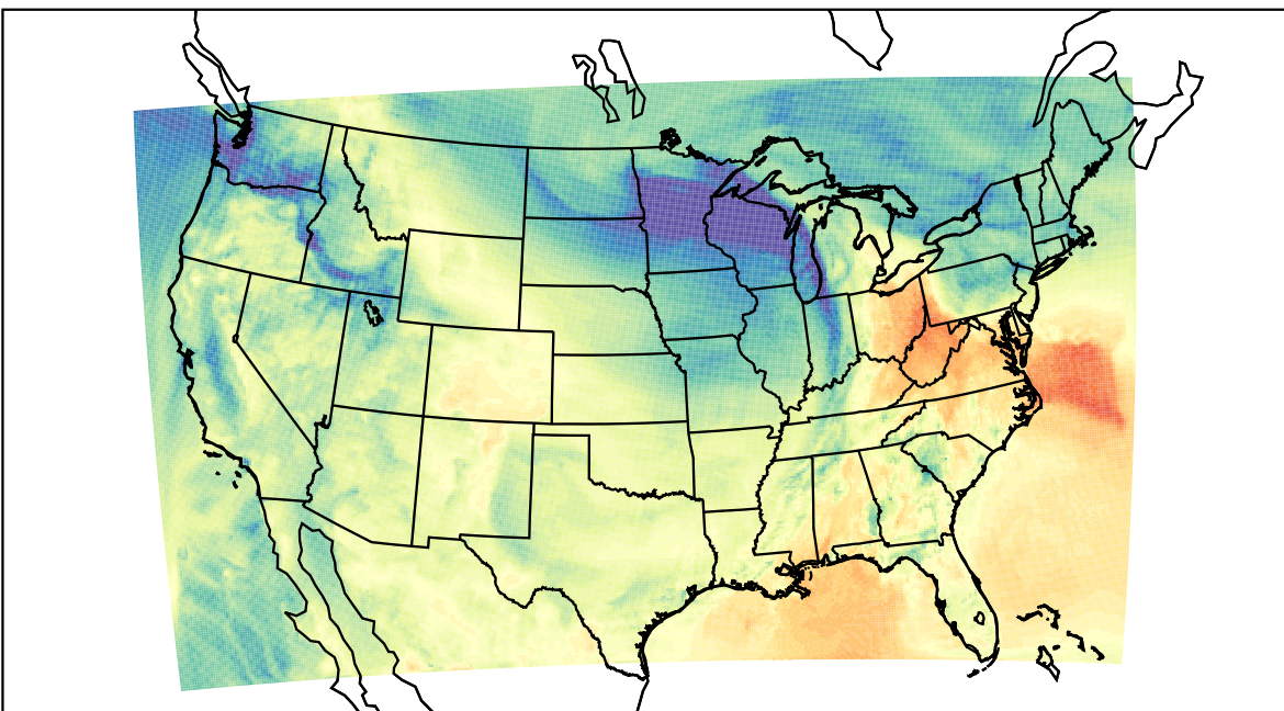
WRF (2021-11-11_19:00:00)
