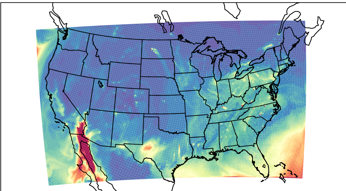
WRF 2021-12-18_18:00:00
