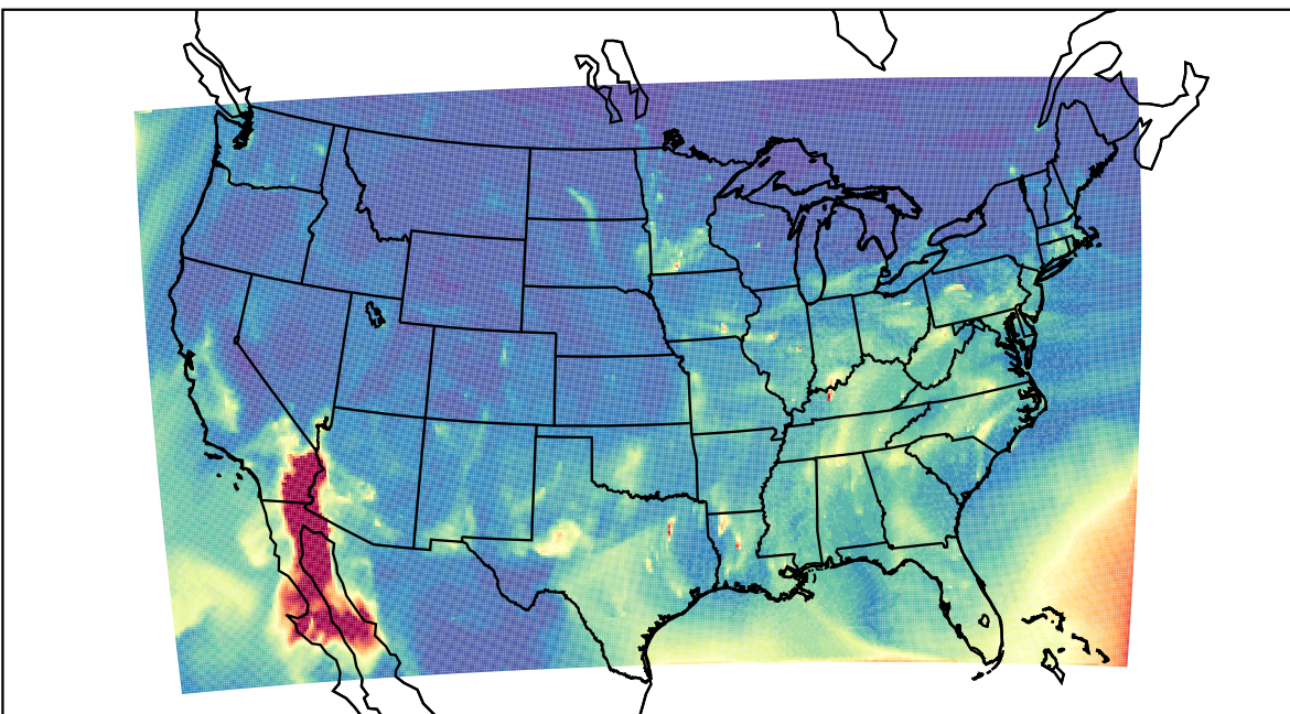
WRF 2021-12-18_10:00:00
