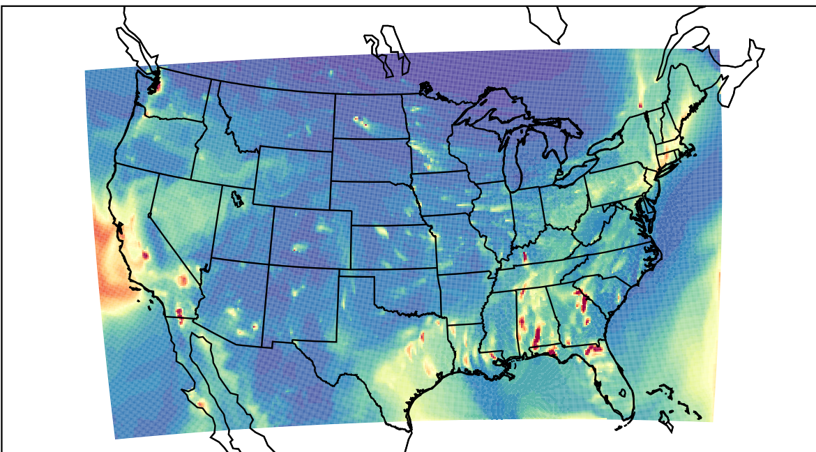
WRF 2021-12-17_04:00:00
