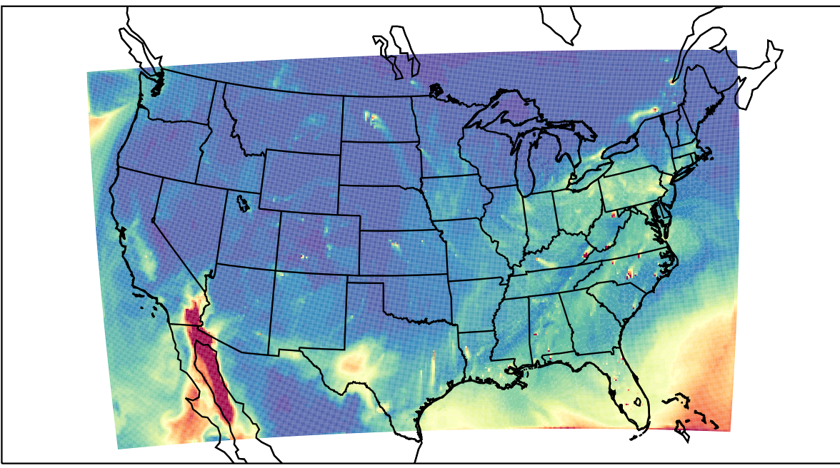
WRF 2021-12-18_20:00:00
