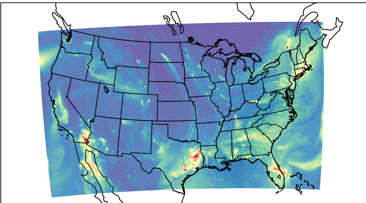
WRF 2022-01-06_10:00:00
