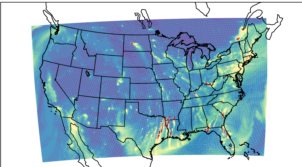
WRF 2022-01-07_01:00:00
