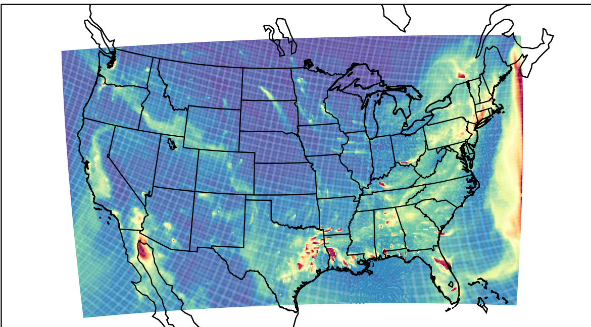
WRF 2022-01-06_03:00:00
