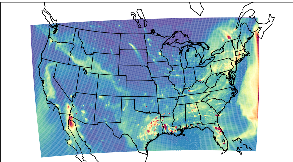
WRF 2022-01-06_01:00:00
