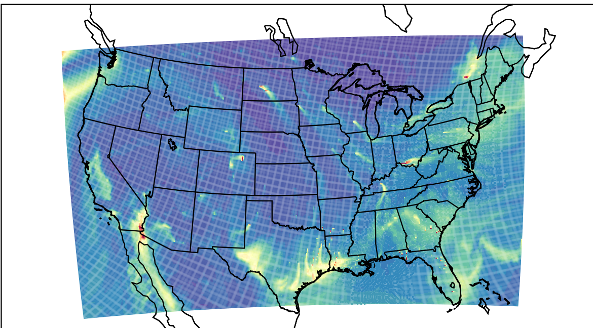
WRF 2022-01-06_18:00:00
