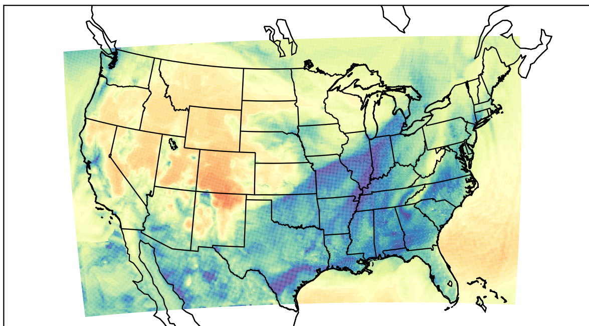
WRF (2022-01-12_10:00:00)
