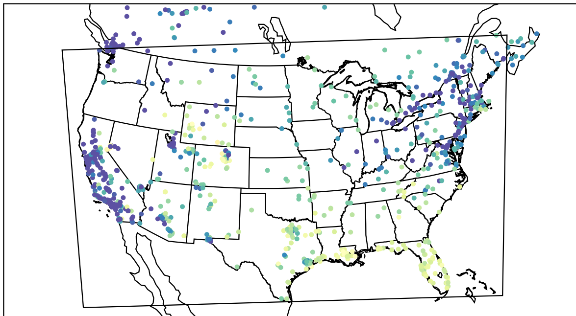
AirNOW (2022-01-13_18:00:00)
