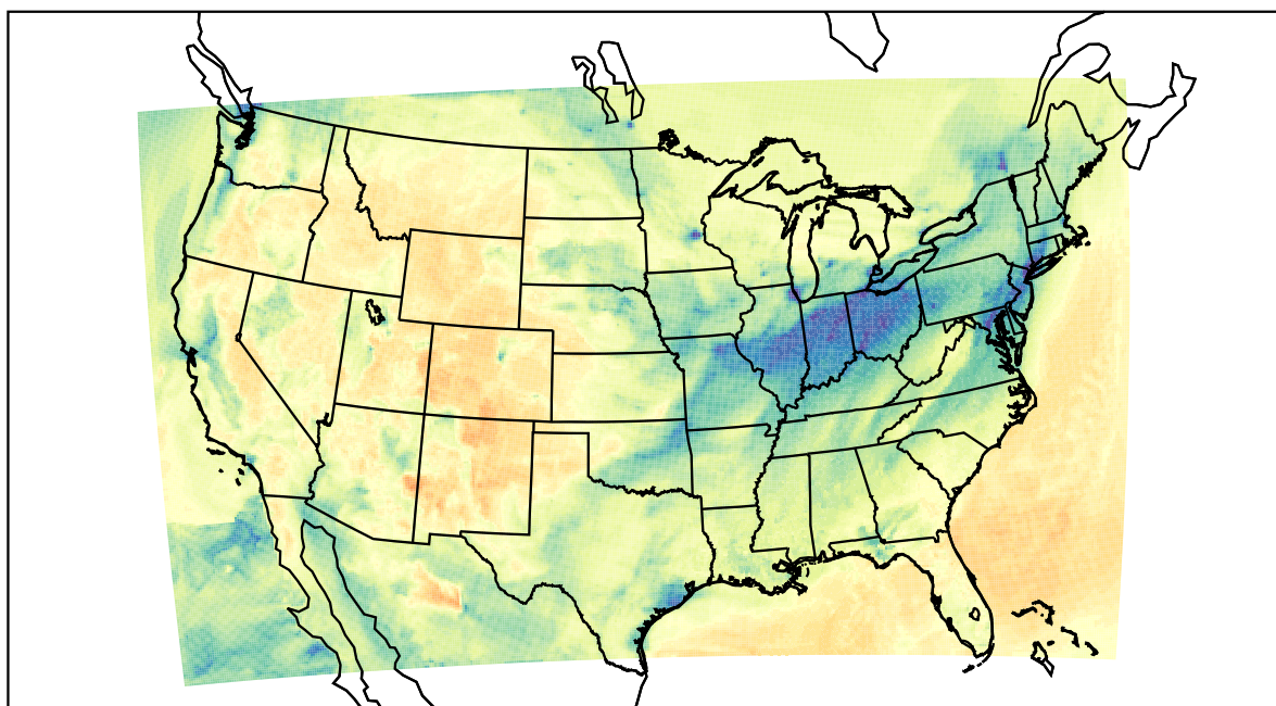
WRF (2022-01-12_20:00:00)
