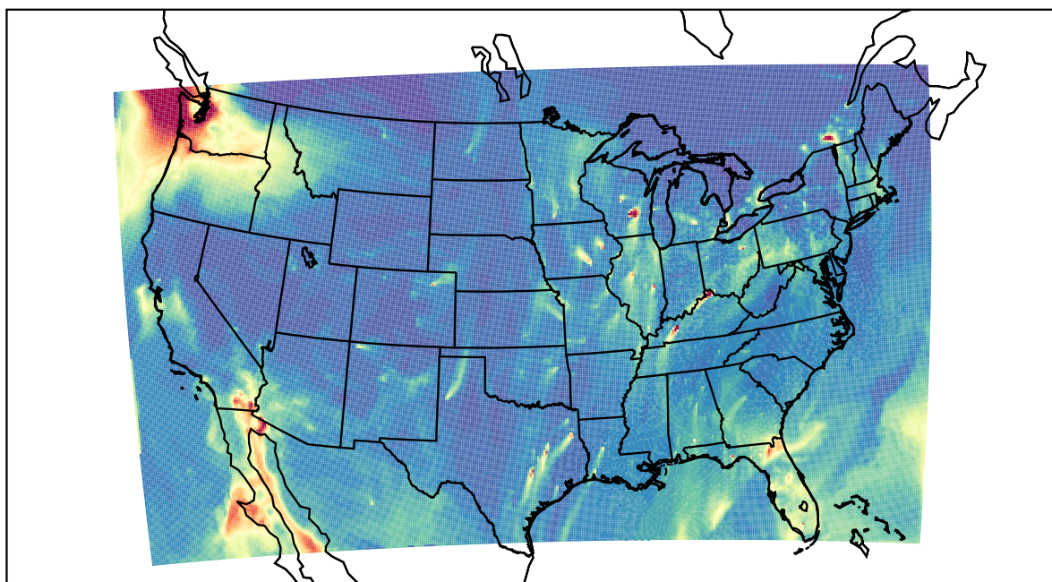
WRF 2022-01-21_12:00:00
