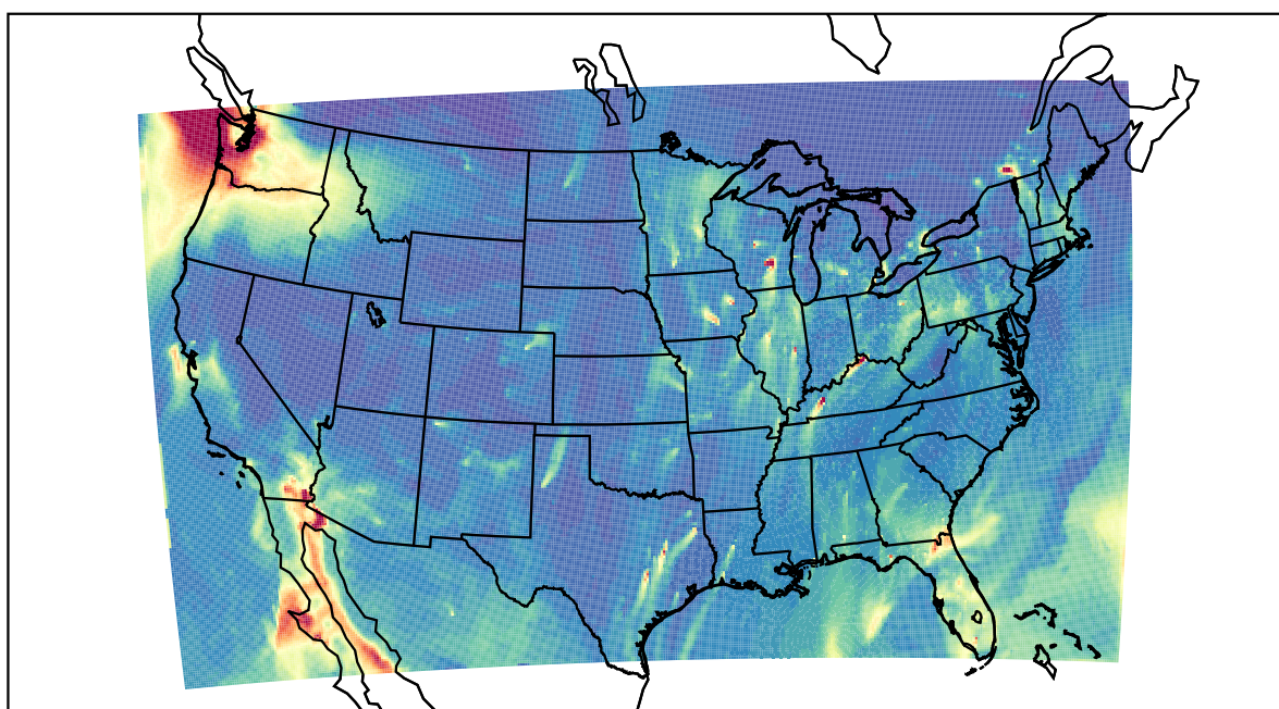
WRF 2022-01-21_11:00:00
