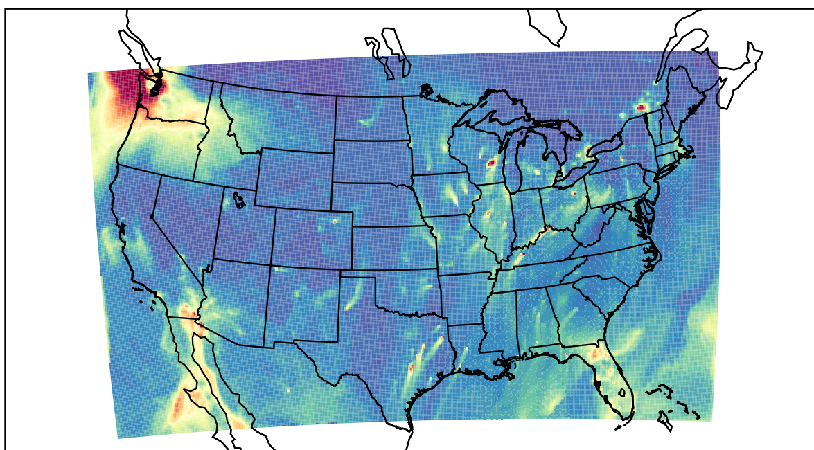
WRF 2022-01-21_14:00:00
