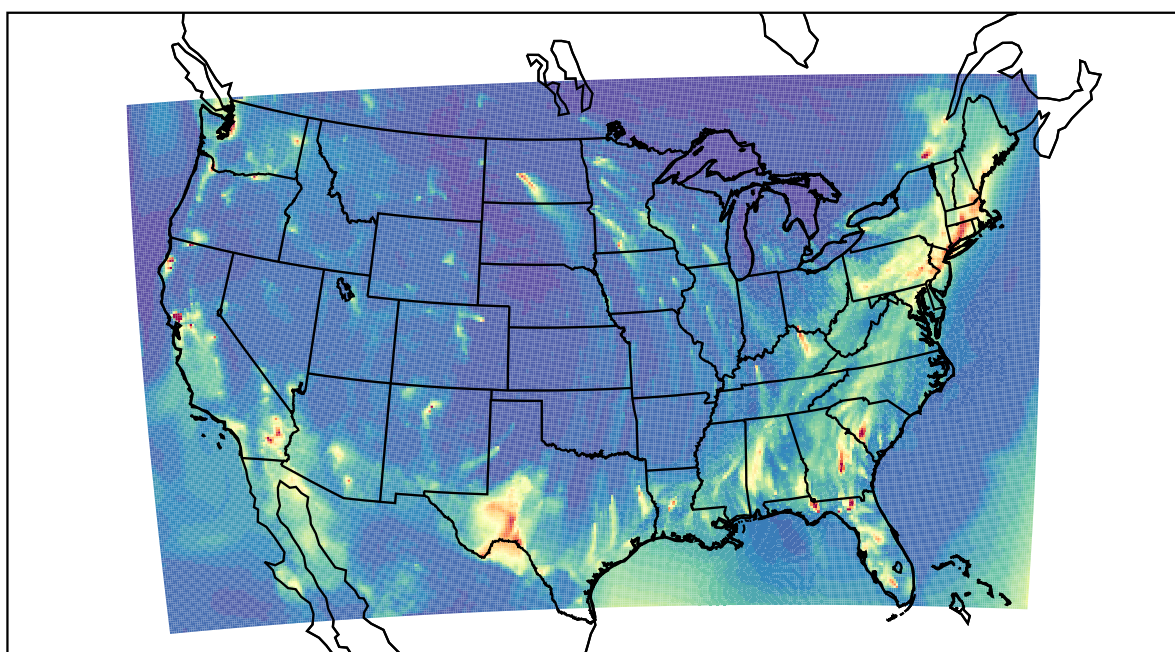
WRF 2022-01-20_04:00:00
