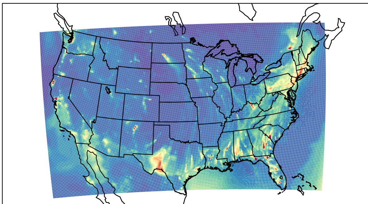
WRF 2022-01-20_03:00:00
