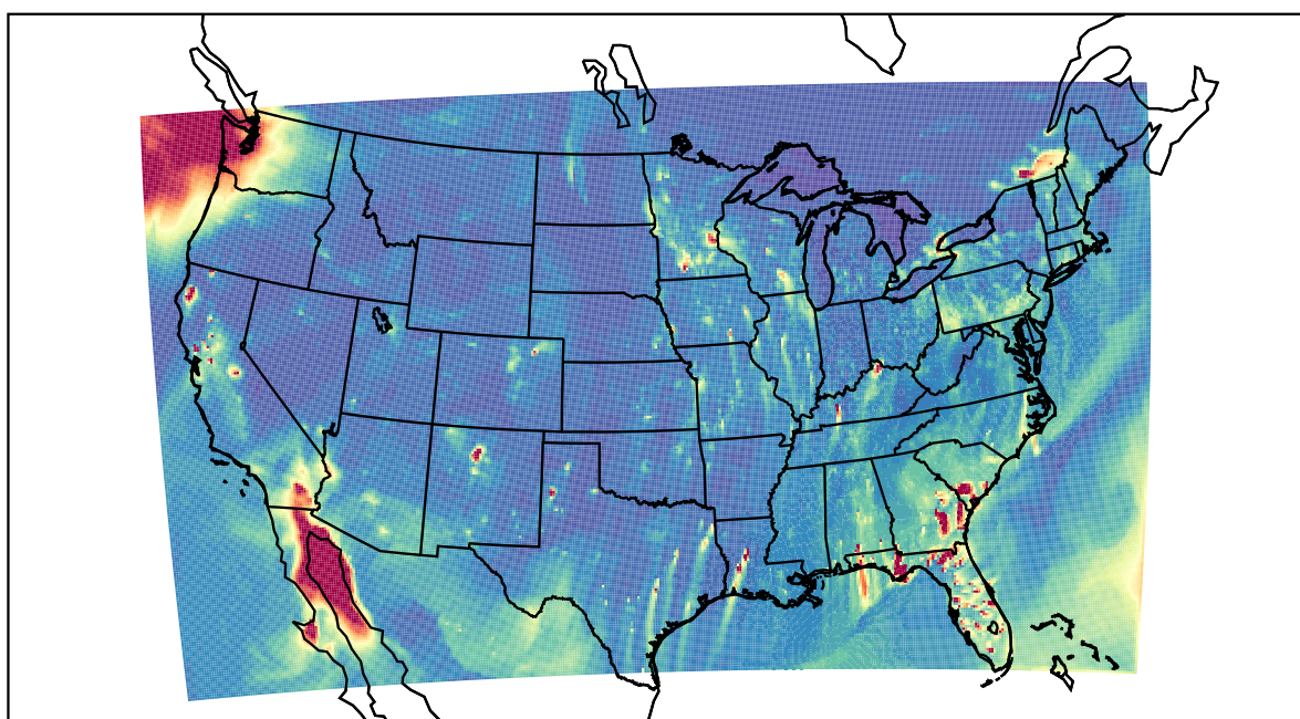
WRF 2022-01-21_01:00:00
