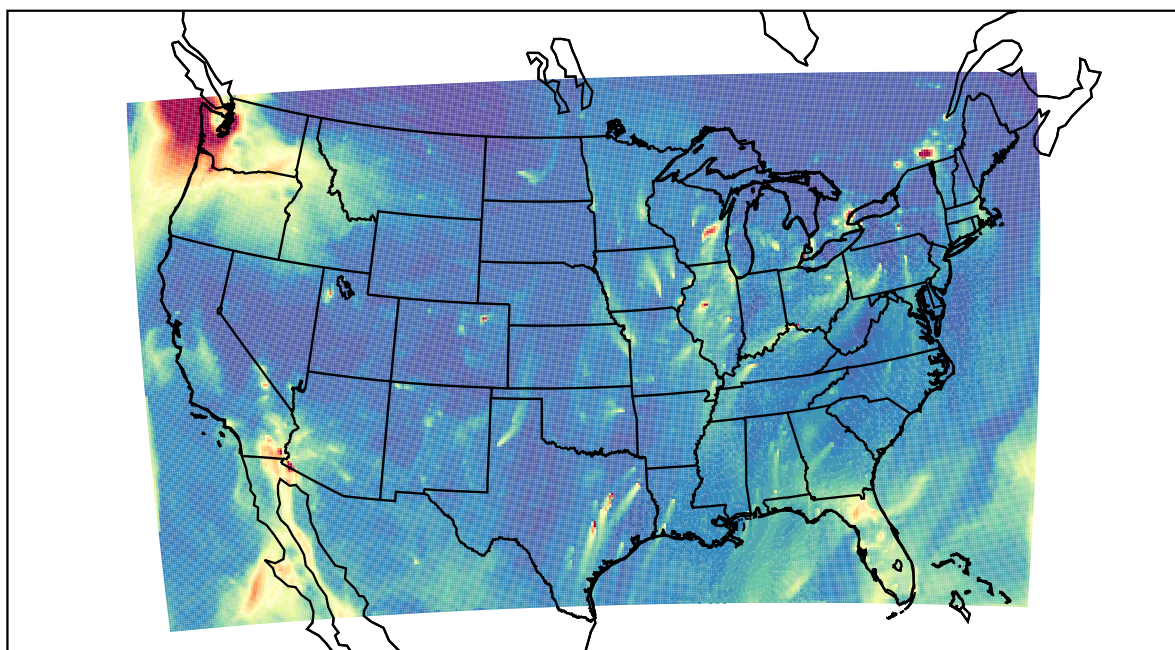
WRF 2022-01-21_15:00:00
