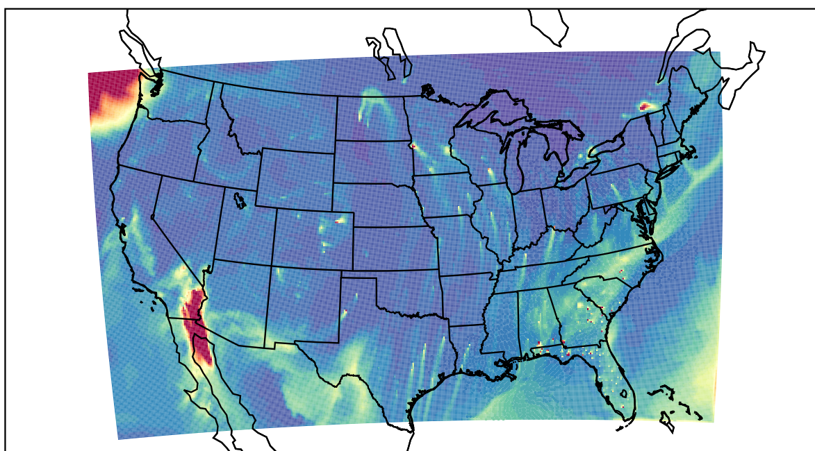
WRF 2022-01-20_18:00:00
