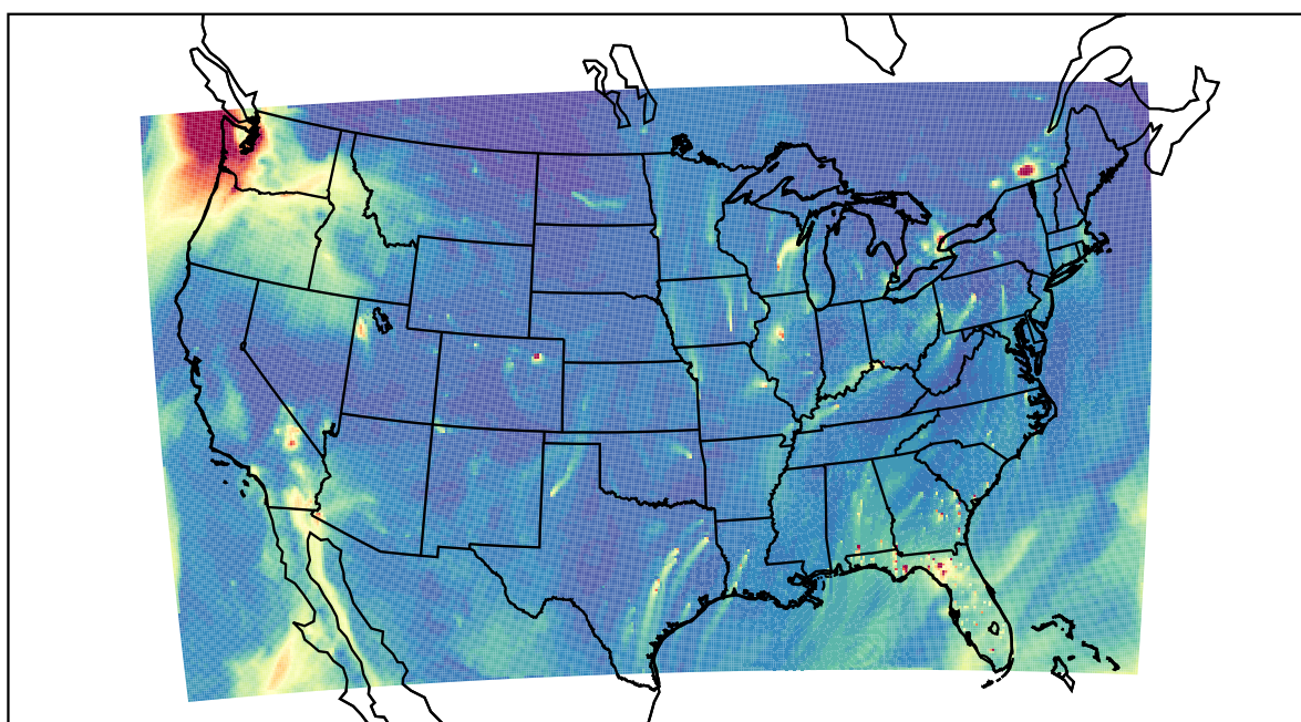
WRF 2022-01-21_18:00:00
