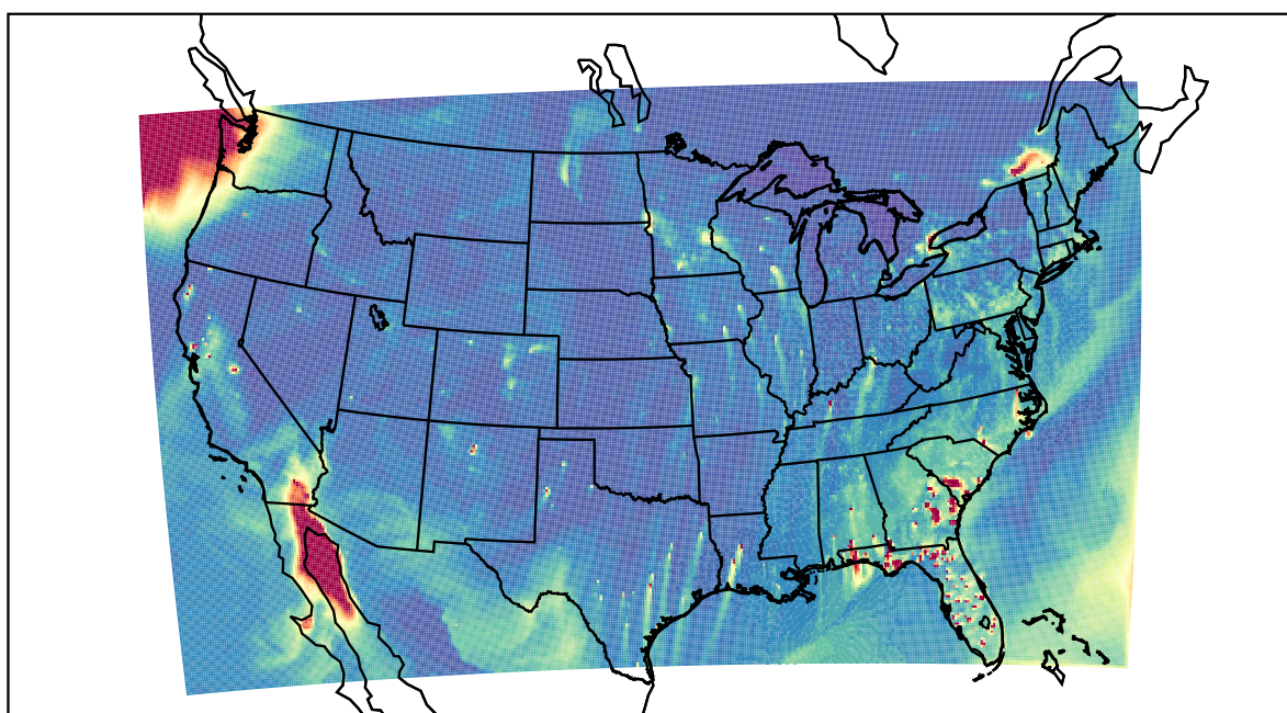
WRF 2022-01-20_23:00:00
