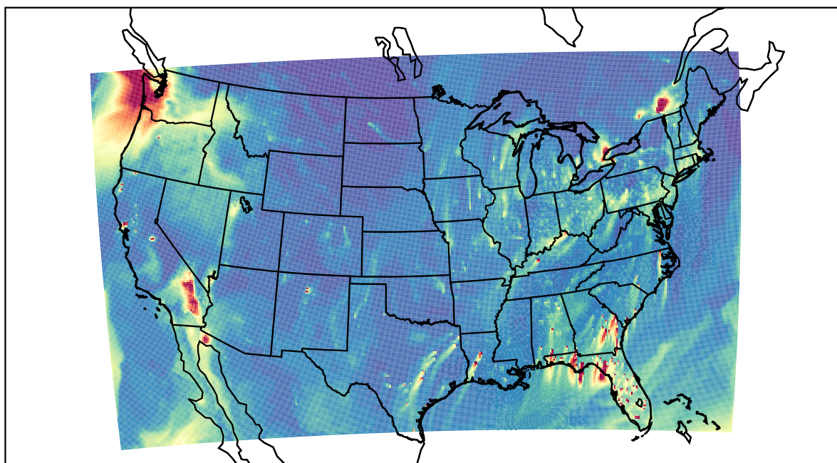
WRF 2022-01-21_23:00:00
