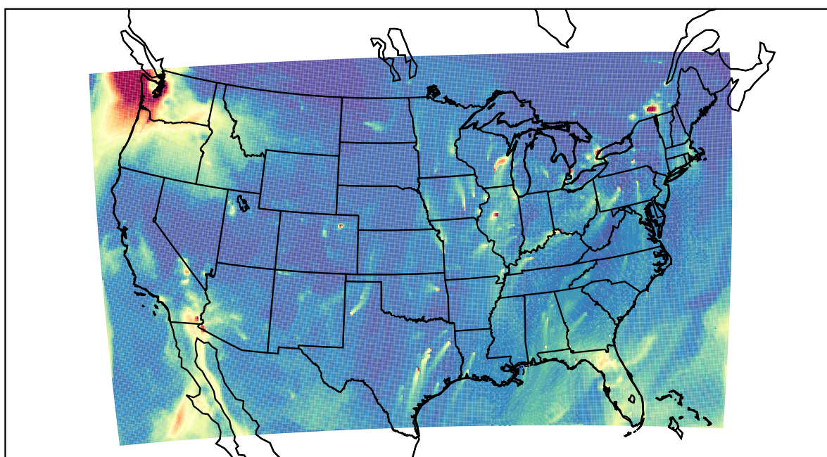
WRF 2022-01-21_16:00:00
