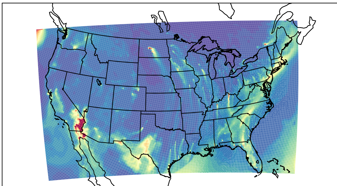
WRF 2022-01-20_10:00:00
