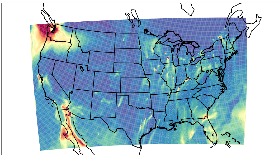
WRF 2022-01-21_10:00:00
