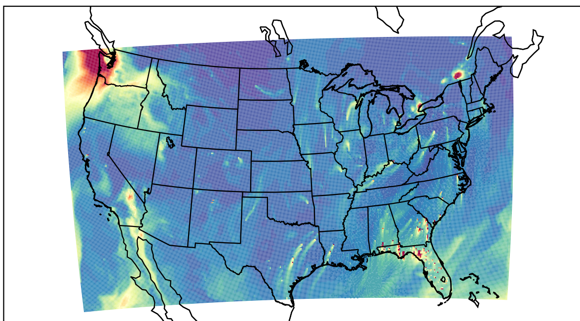
WRF 2022-01-21_20:00:00
