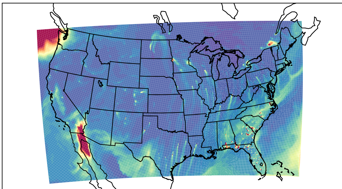
WRF 2022-01-20_20:00:00
