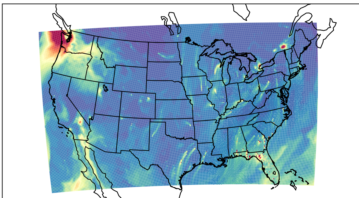
WRF 2022-01-21_19:00:00
