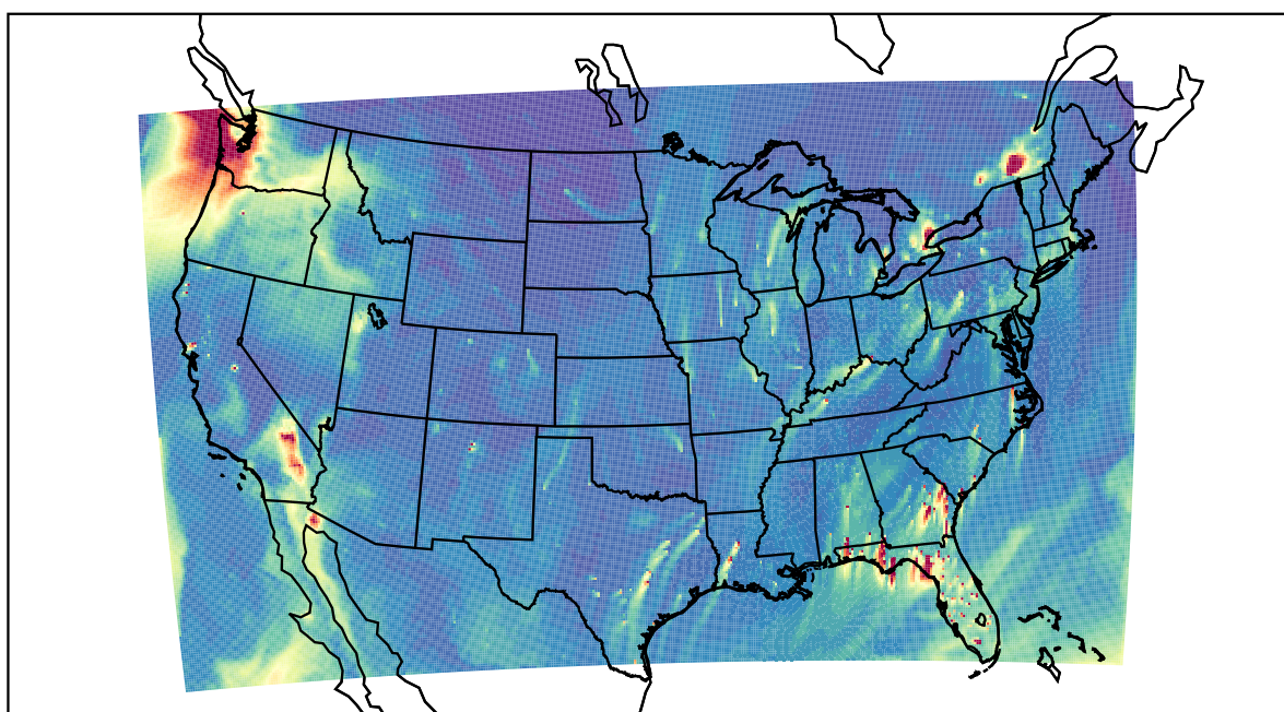
WRF 2022-01-21_22:00:00
