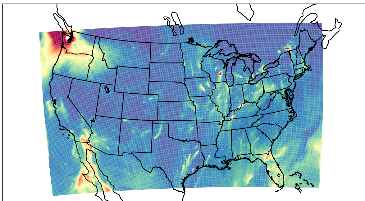
WRF 2022-01-21_13:00:00
