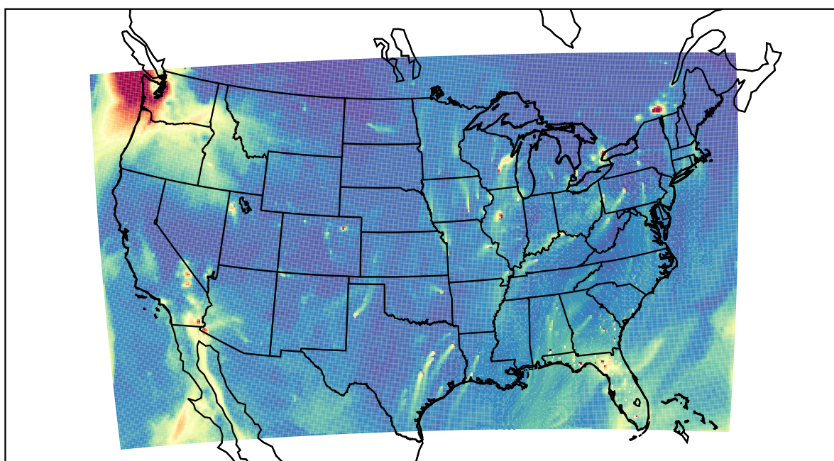
WRF 2022-01-21_17:00:00
