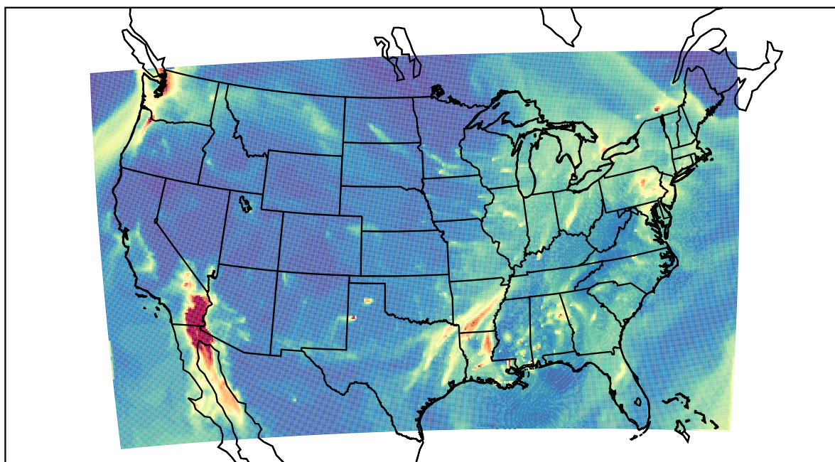
WRF 2022-02-09_10:00:00
