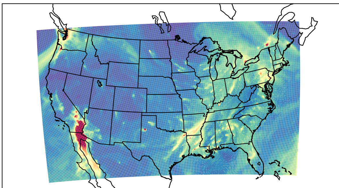
WRF 2022-02-09_13:00:00
