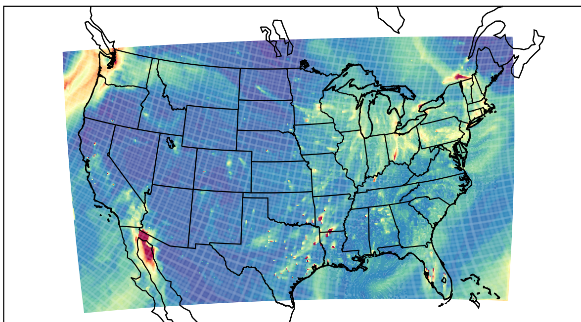
WRF 2022-02-09_00:00:00
