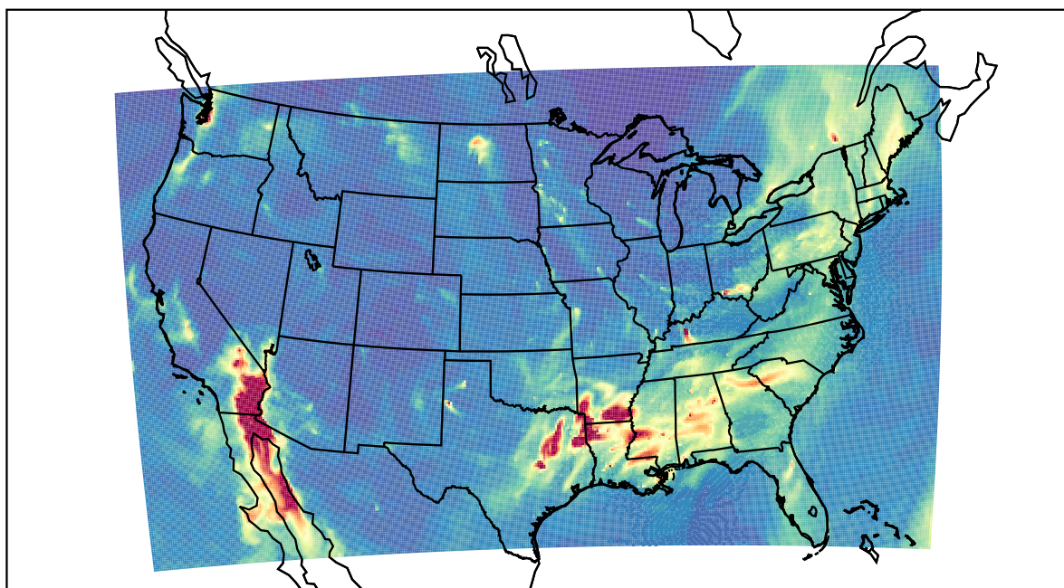
WRF 2022-02-10_10:00:00
