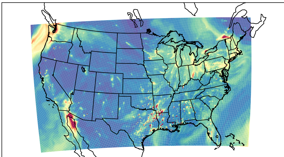
WRF 2022-02-09_01:00:00
