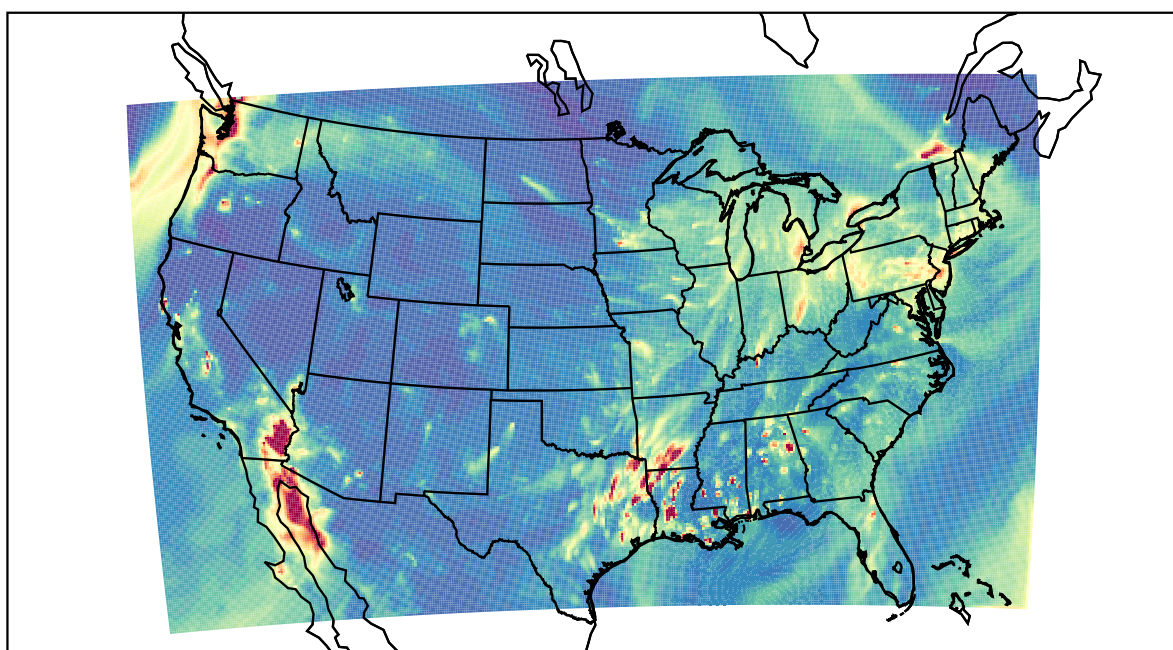
WRF 2022-02-09_04:00:00
