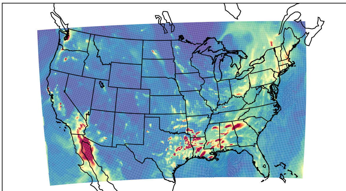
WRF 2022-02-10_03:00:00
