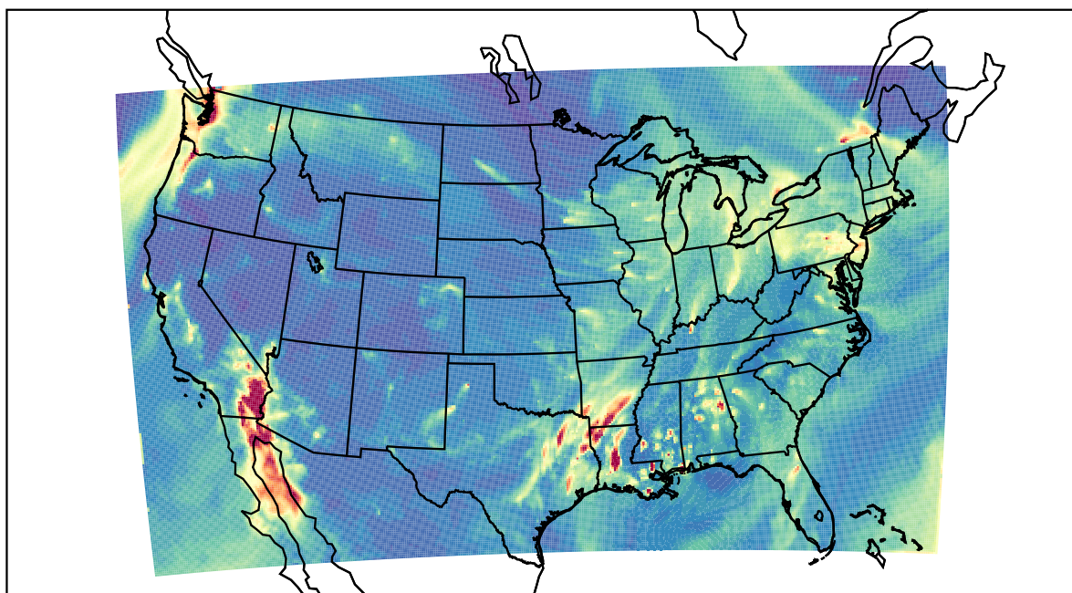
WRF 2022-02-09_06:00:00
