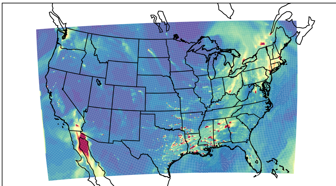
WRF 2022-02-09_23:00:00
