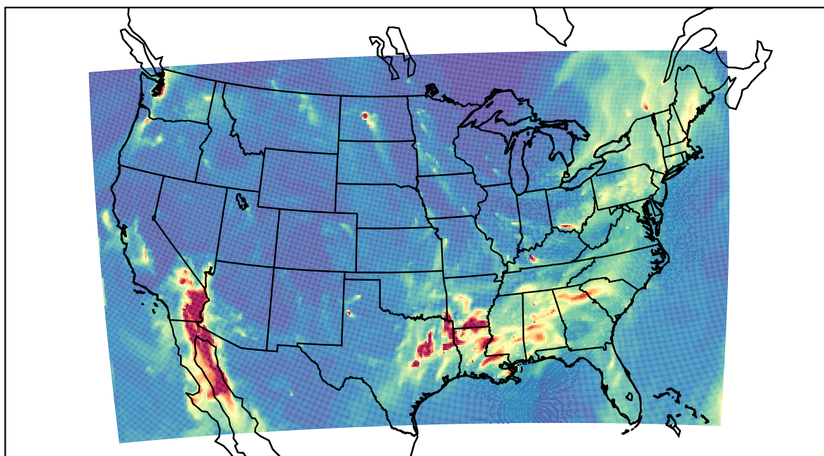
WRF 2022-02-10_08:00:00
