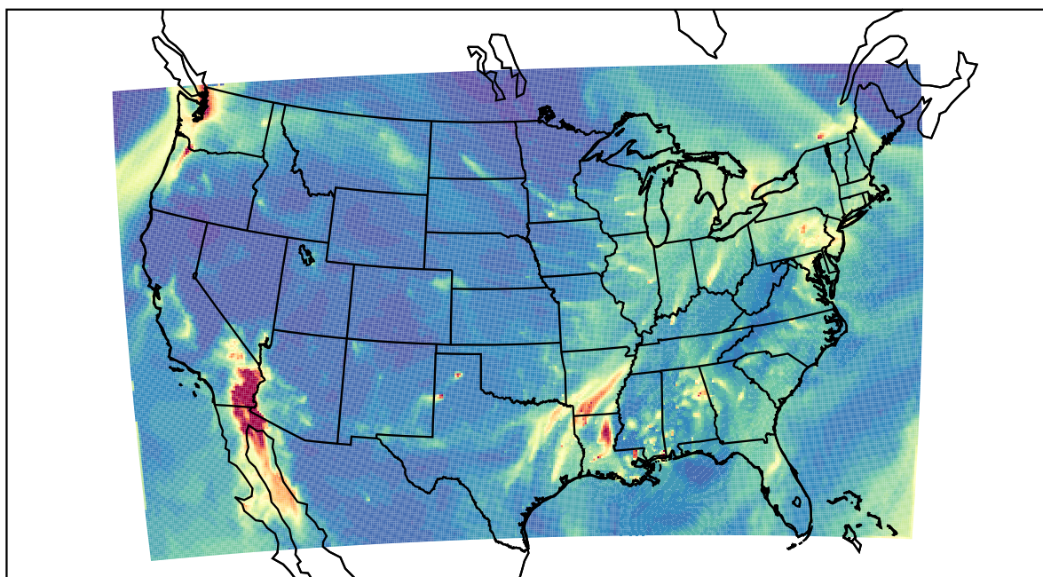
WRF 2022-02-09_09:00:00
