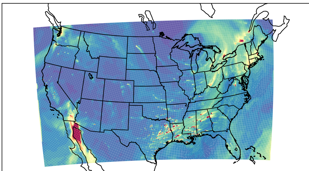
WRF 2022-02-09_22:00:00
