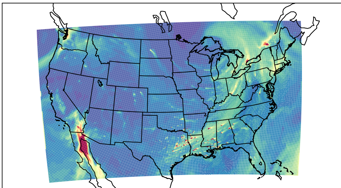
WRF 2022-02-09_20:00:00
