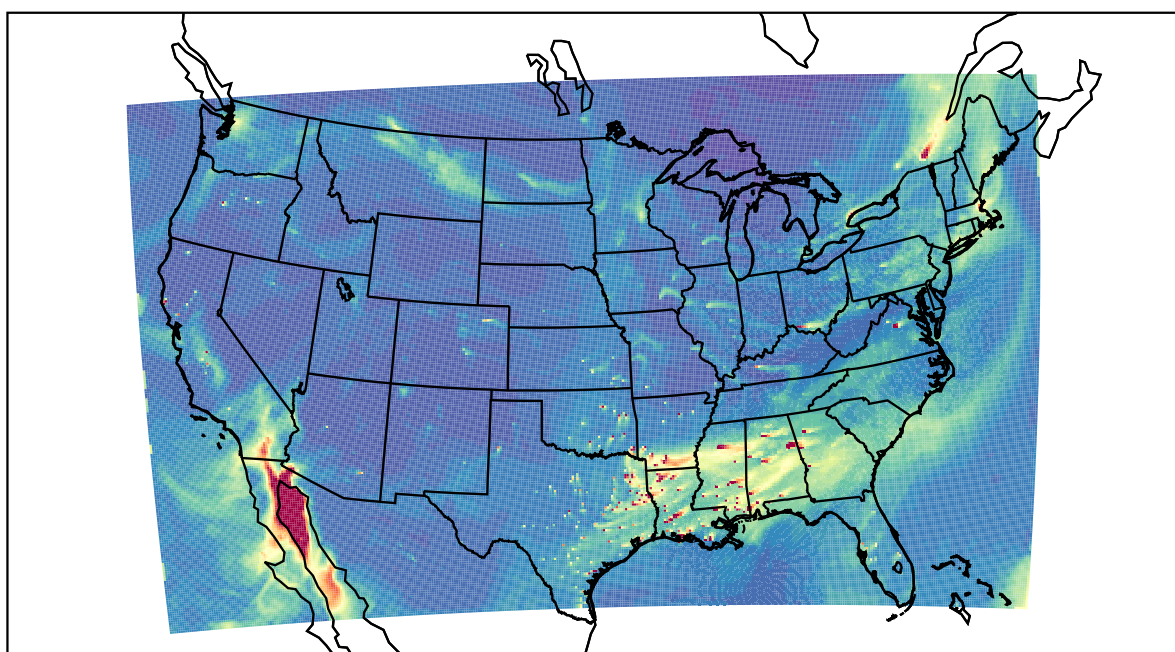
WRF 2022-02-10_22:00:00
