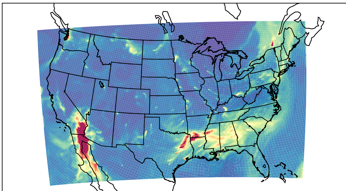
WRF 2022-02-10_16:00:00
