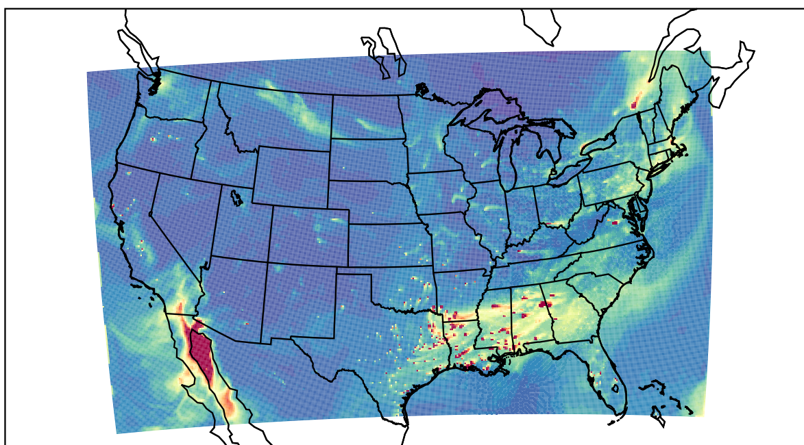
WRF 2022-02-10_23:00:00
