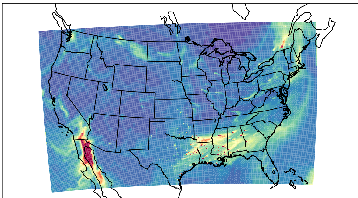
WRF 2022-02-10_20:00:00
