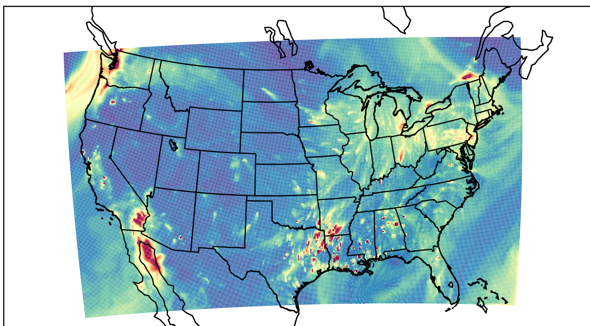
WRF 2022-02-09_03:00:00
