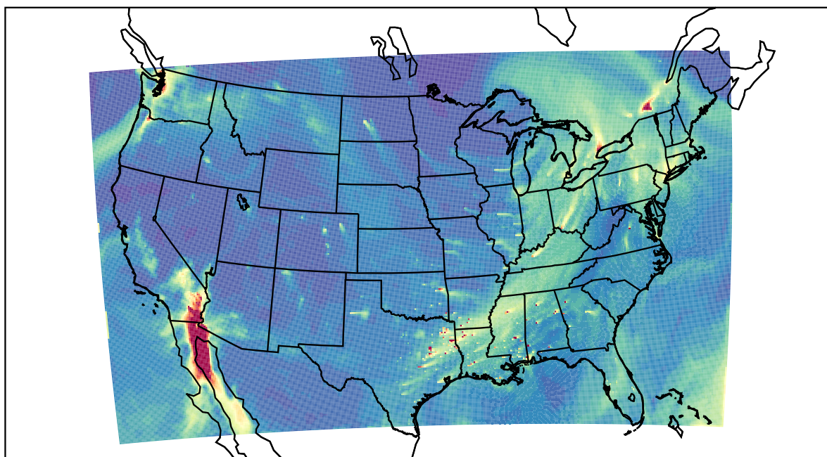
WRF 2022-02-09_18:00:00
