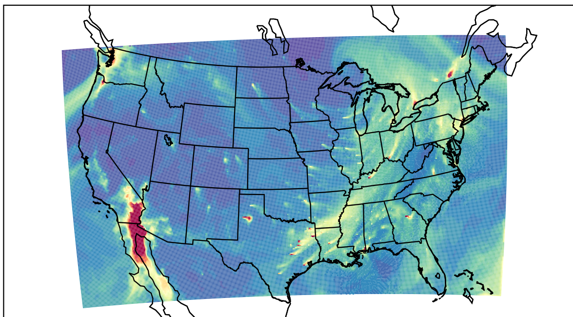
WRF 2022-02-09_16:00:00
