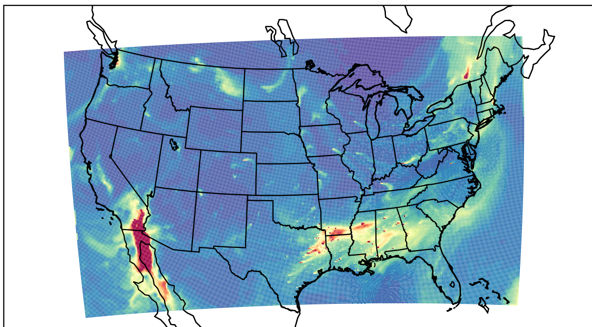
WRF 2022-02-10_18:00:00
