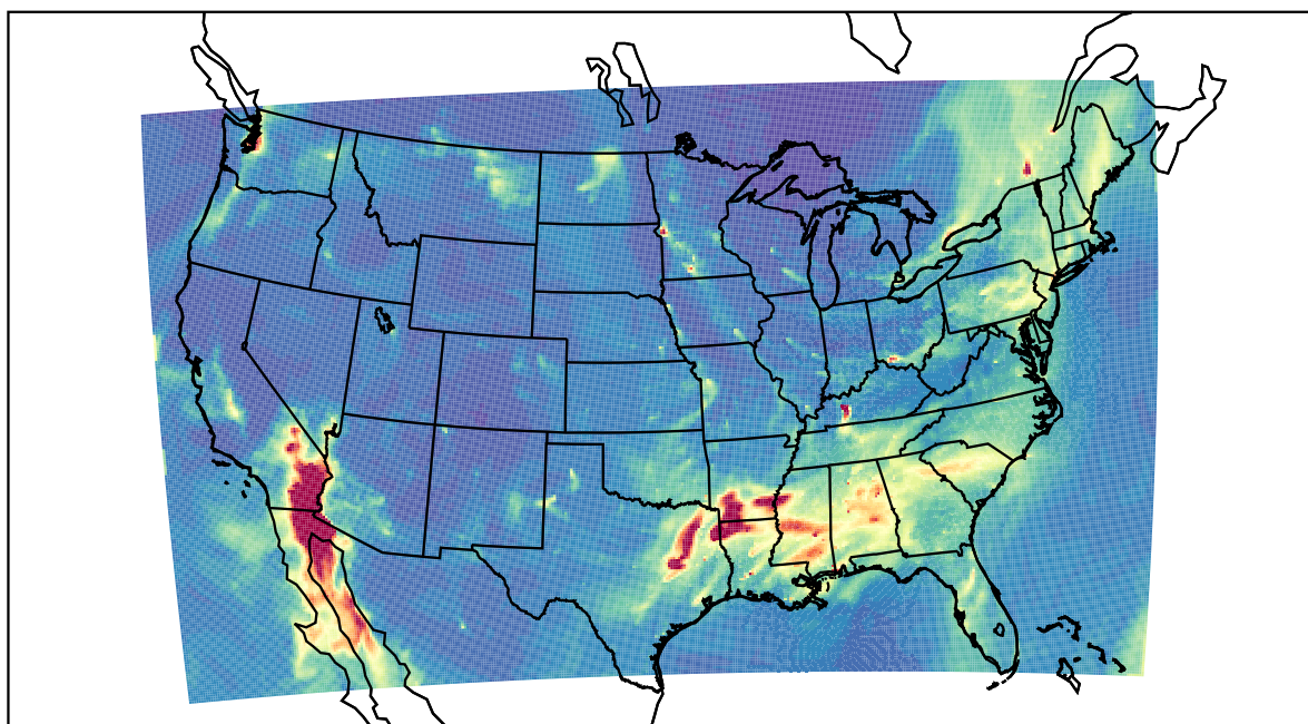
WRF 2022-02-10_13:00:00
