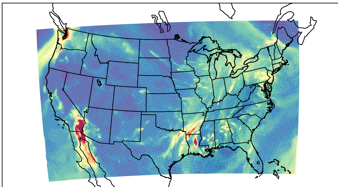
WRF 2022-02-09_08:00:00
