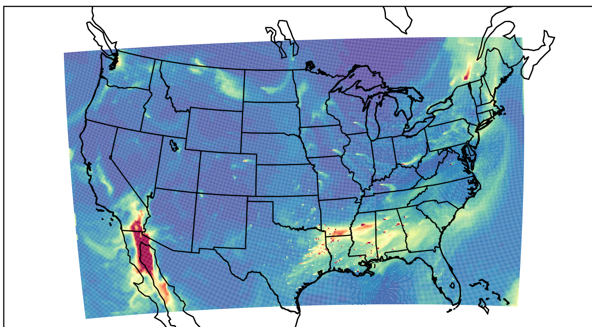
WRF 2022-02-10_19:00:00
