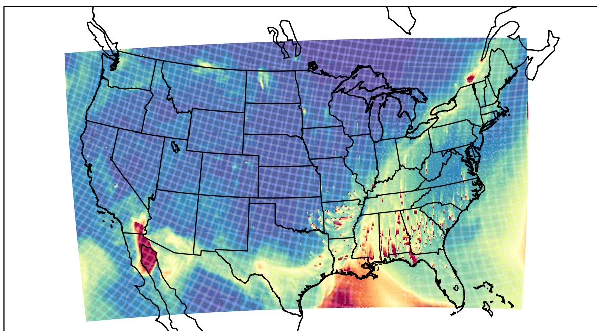
WRF 2022-02-17_20:00:00
