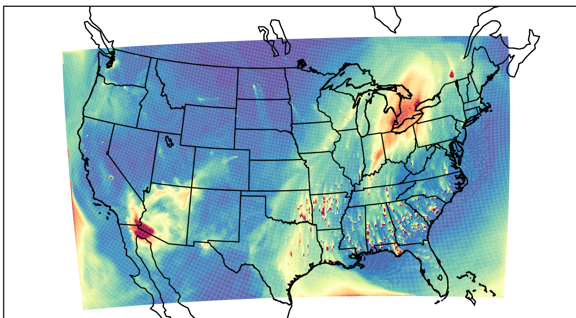
WRF 2022-02-16_20:00:00
