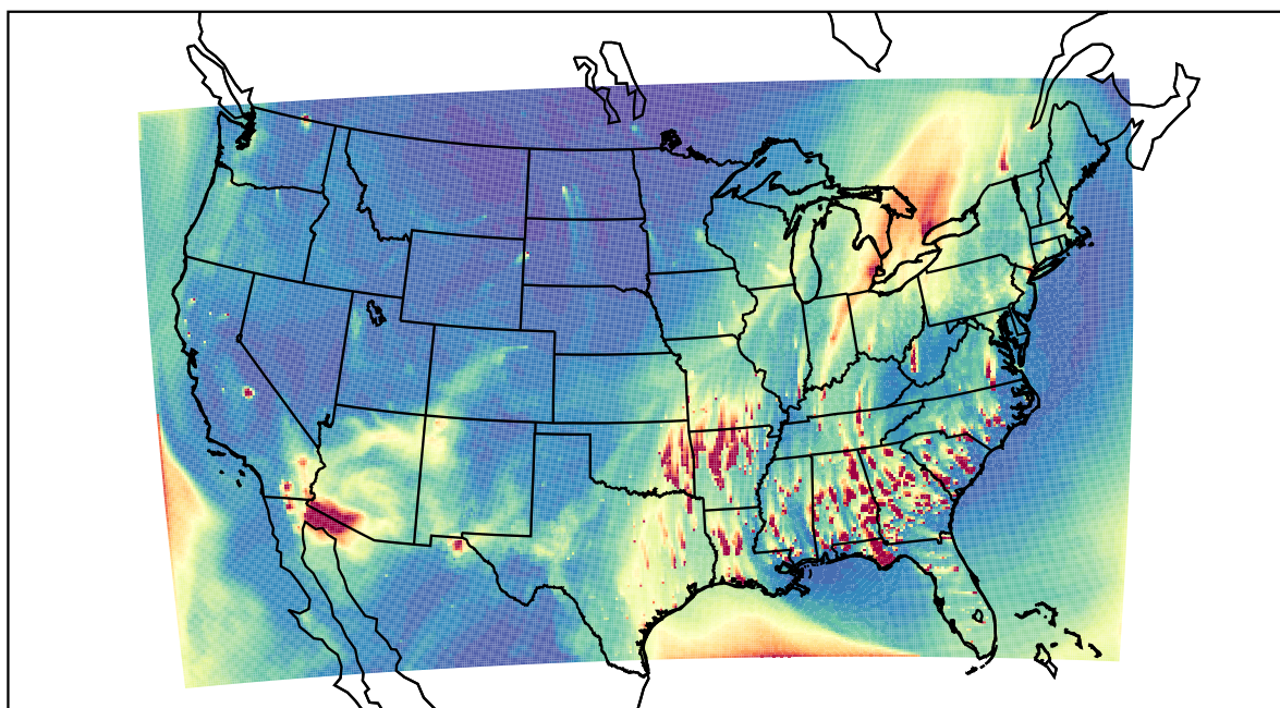
WRF 2022-02-16_23:00:00
