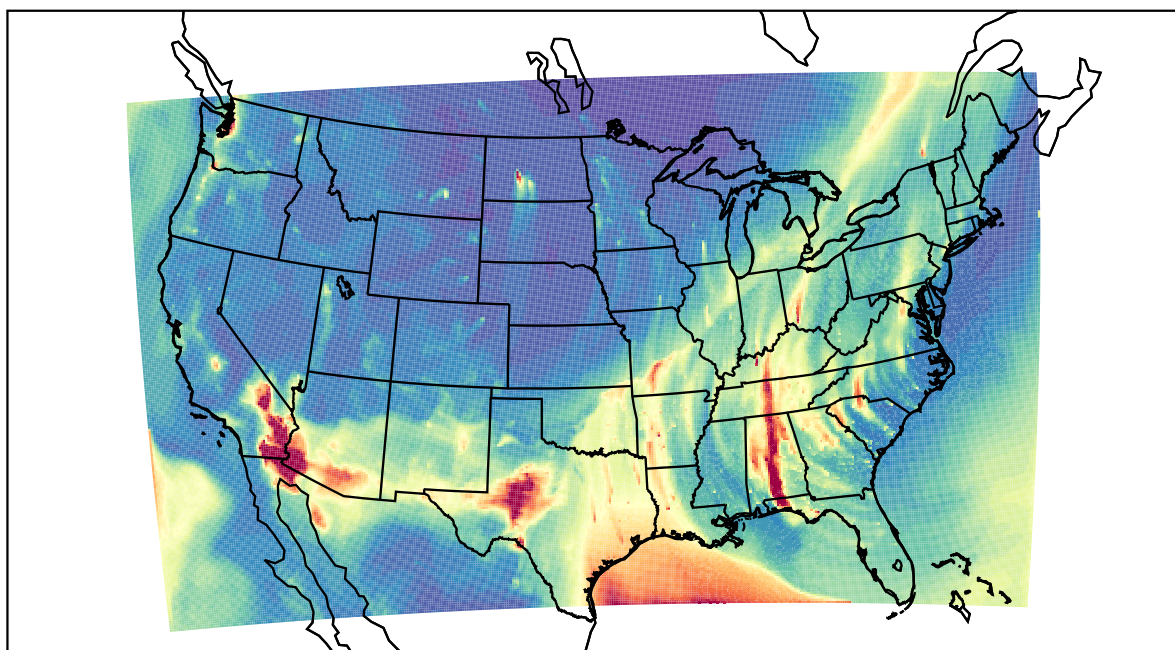
WRF 2022-02-17_07:00:00
