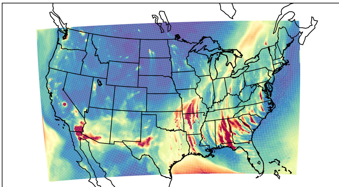
WRF 2022-02-17_03:00:00
