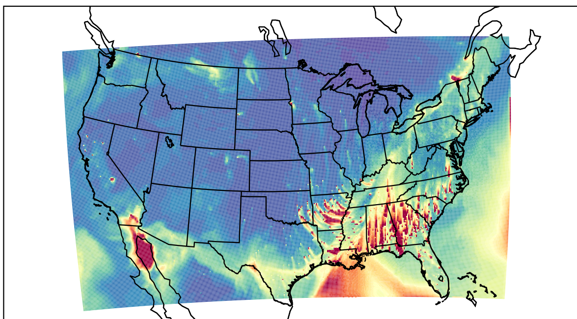
WRF 2022-02-17_23:00:00
