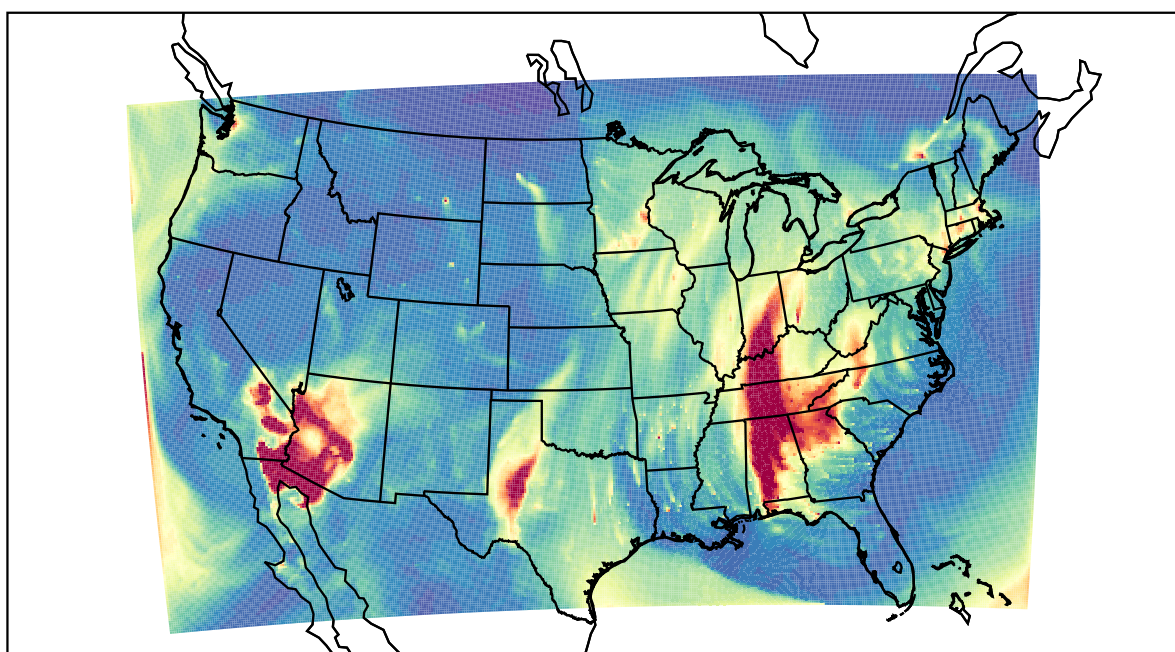
WRF 2022-02-16_10:00:00
