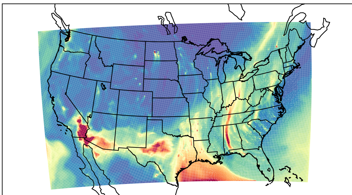
WRF 2022-02-17_10:00:00
