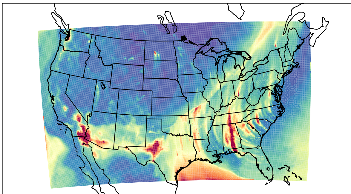
WRF 2022-02-17_06:00:00
