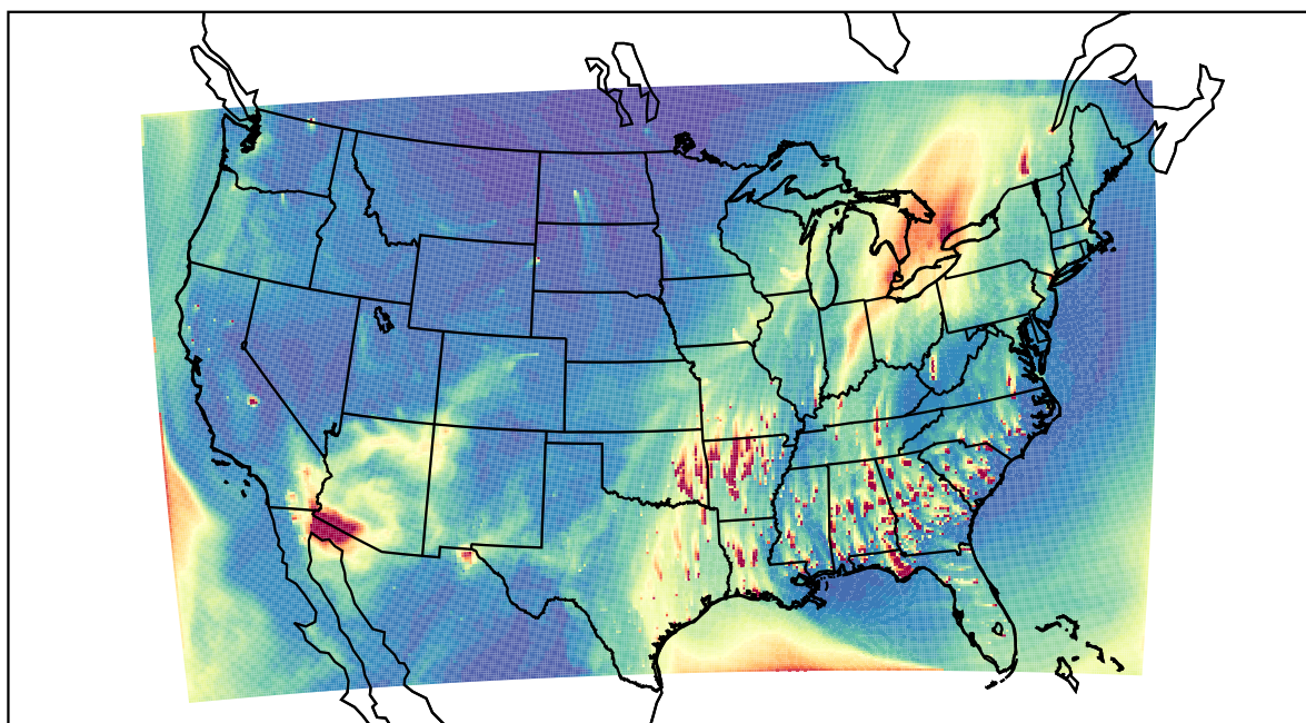
WRF 2022-02-16_22:00:00
