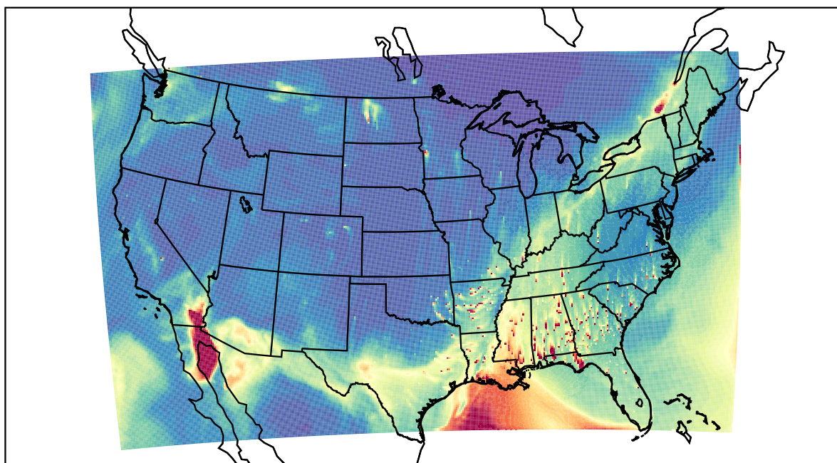
WRF 2022-02-17_19:00:00
