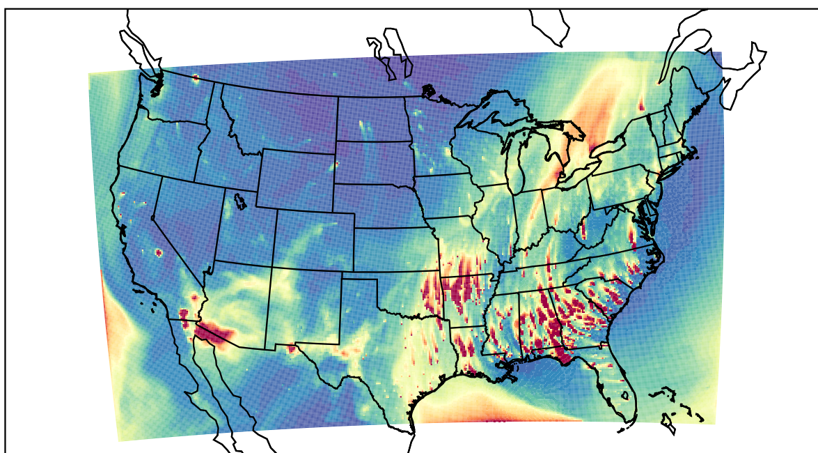
WRF 2022-02-17_00:00:00
