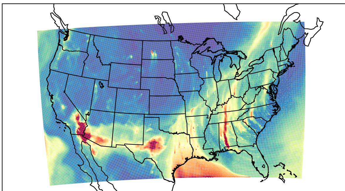
WRF 2022-02-17_08:00:00
