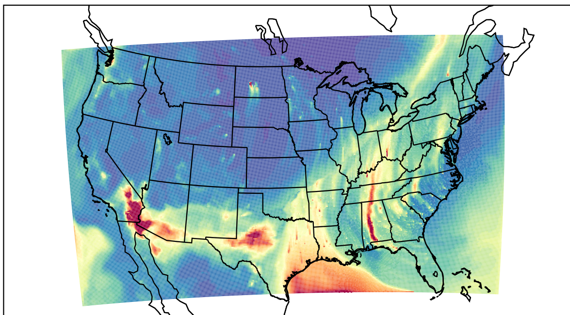
WRF 2022-02-17_09:00:00
