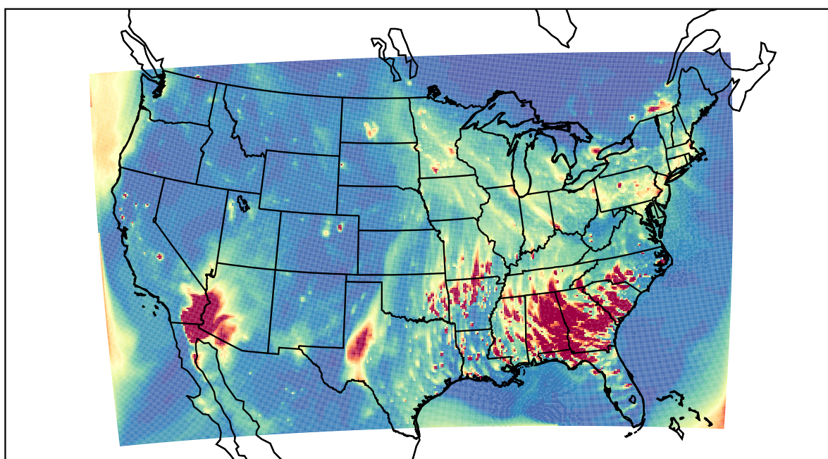
WRF 2022-02-16_01:00:00
