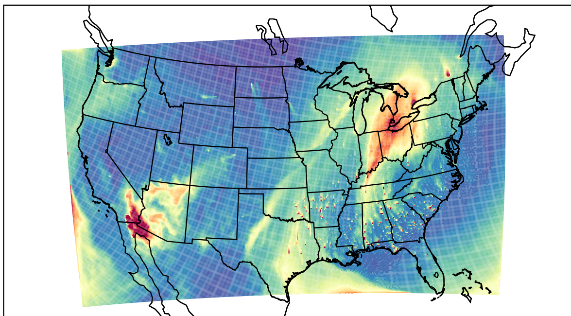
WRF 2022-02-16_18:00:00
