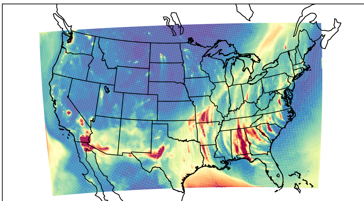
WRF 2022-02-17_04:00:00
