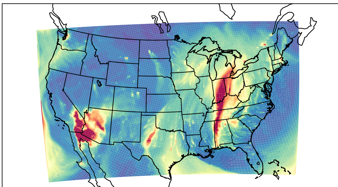
WRF 2022-02-16_14:00:00
