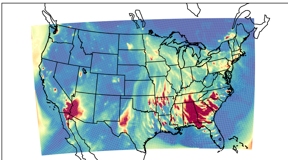
WRF 2022-02-16_03:00:00
