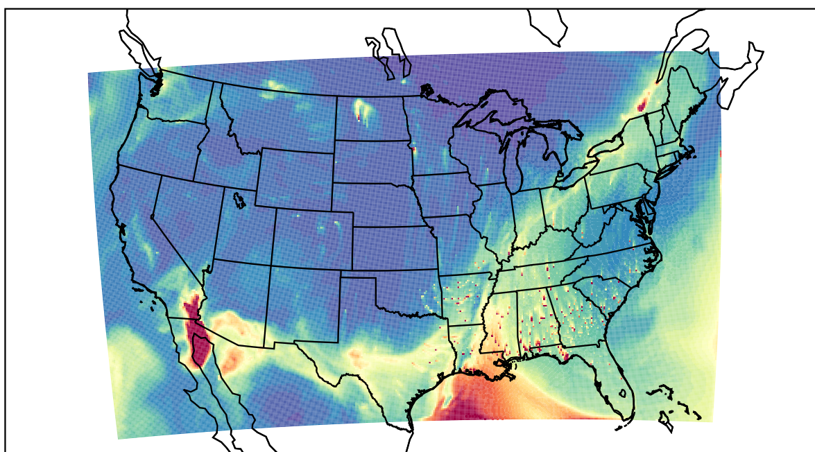
WRF 2022-02-17_18:00:00
