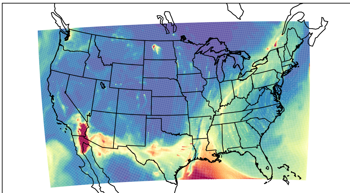
WRF 2022-02-17_16:00:00
