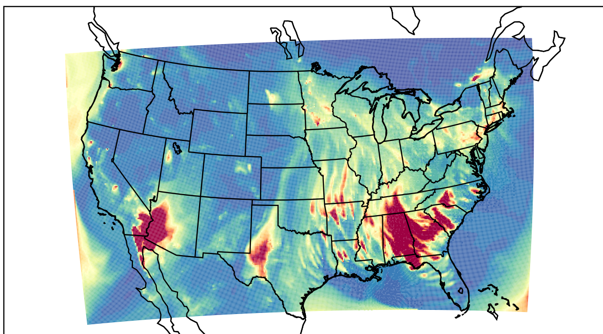
WRF 2022-02-16_04:00:00
