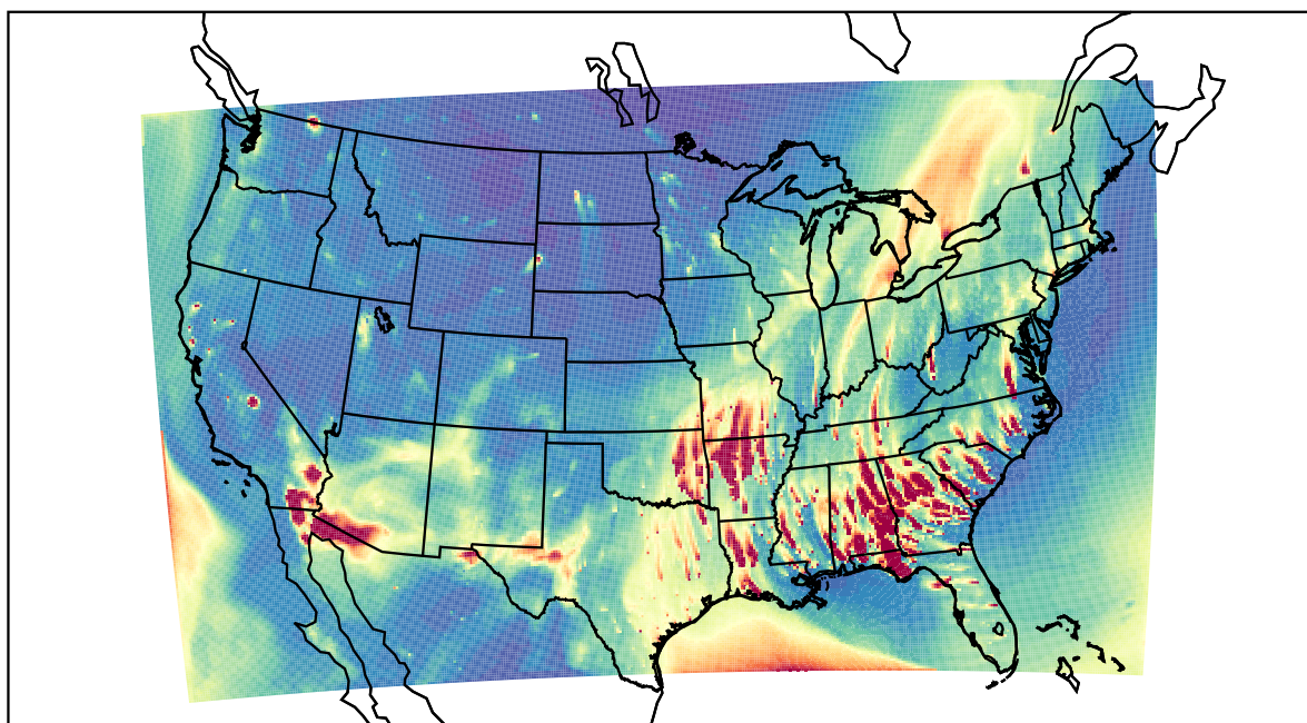
WRF 2022-02-17_01:00:00
