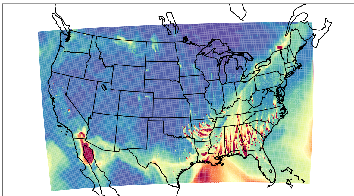
WRF 2022-02-17_22:00:00
