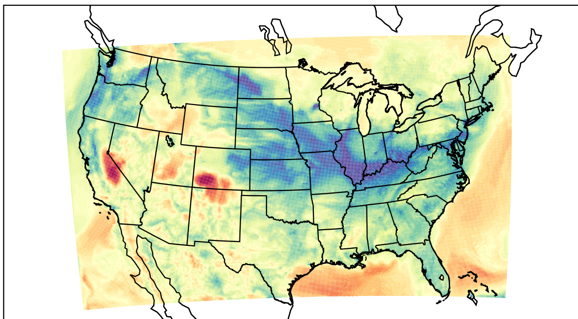
WRF (2022-03-02_10:00:00)
