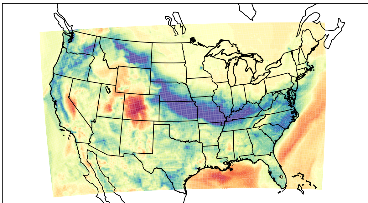
WRF (2022-03-03_13:00:00)
