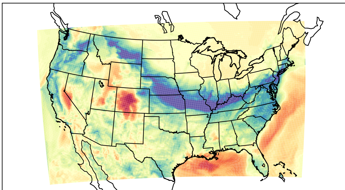
WRF (2022-03-03_10:00:00)
