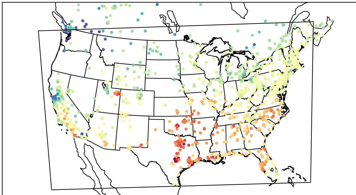
AirNOW (2022-03-02_20:00:00)
