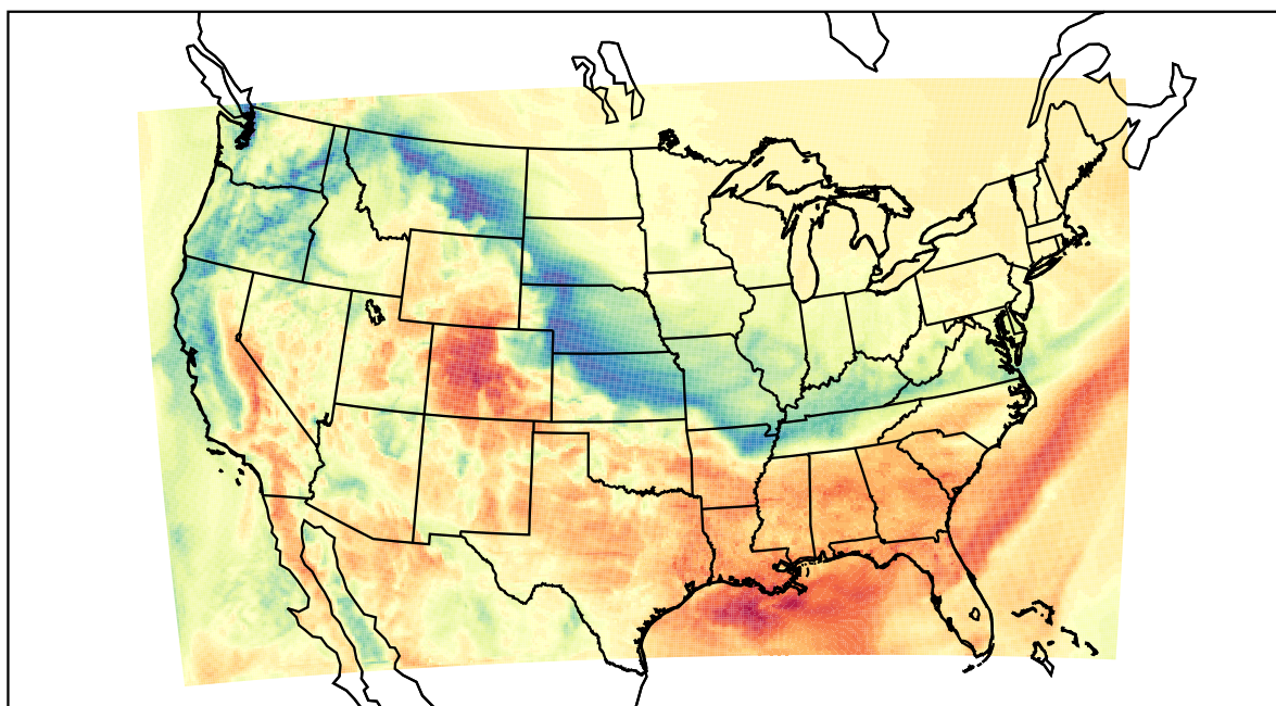
WRF (2022-03-03_18:00:00)
