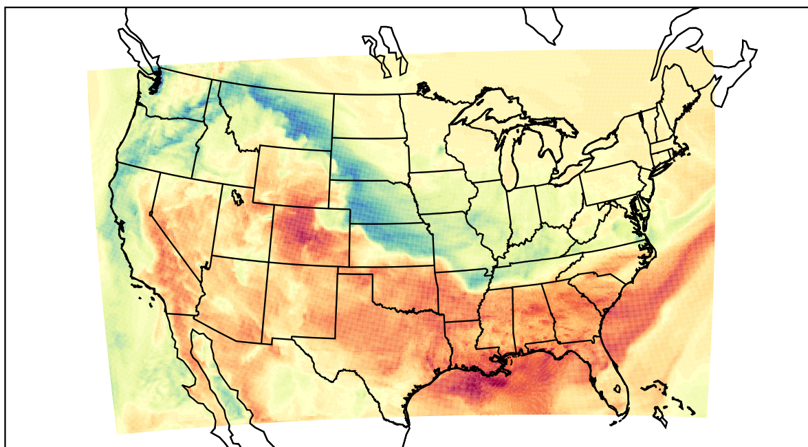
WRF (2022-03-03_20:00:00)
