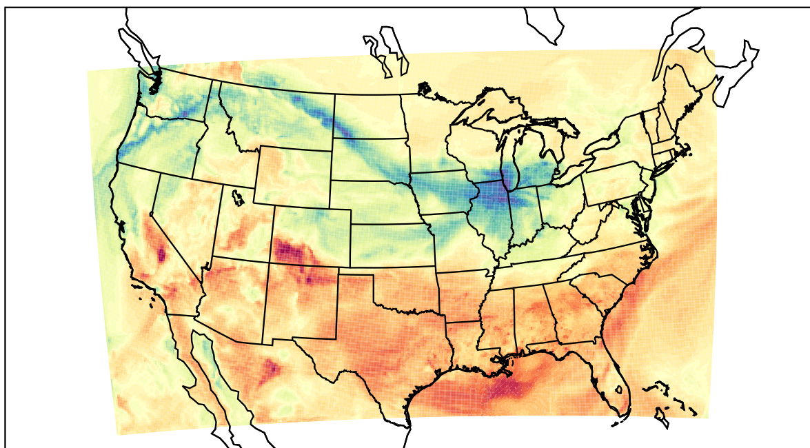
WRF (2022-03-02_20:00:00)
