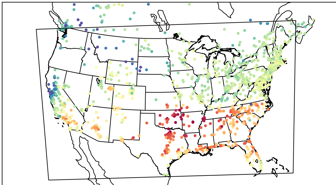
AirNOW (2022-03-03_20:00:00)
