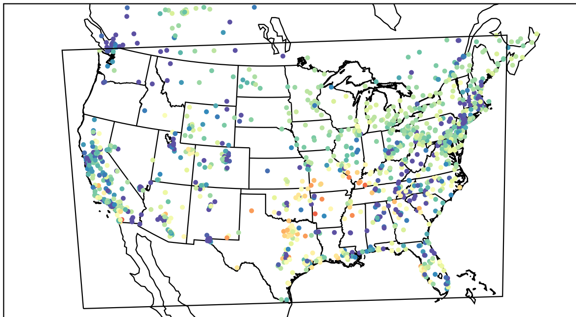
AirNOW (2022-03-03_03:00:00)
