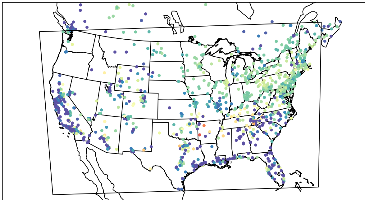
AirNOW (2022-03-03_10:00:00)
