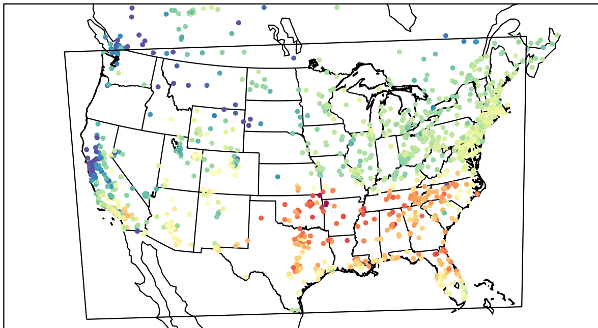
AirNOW (2022-03-03_18:00:00)
