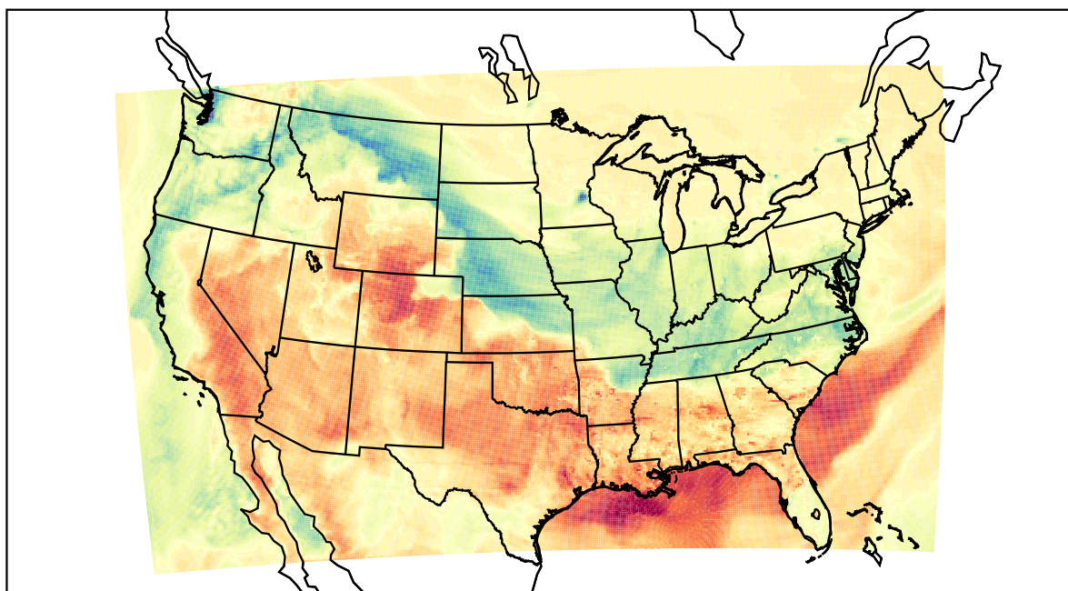
WRF (2022-03-03_23:00:00)
