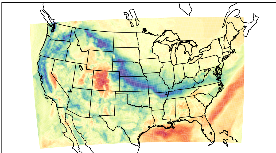
WRF (2022-03-03_16:00:00)
