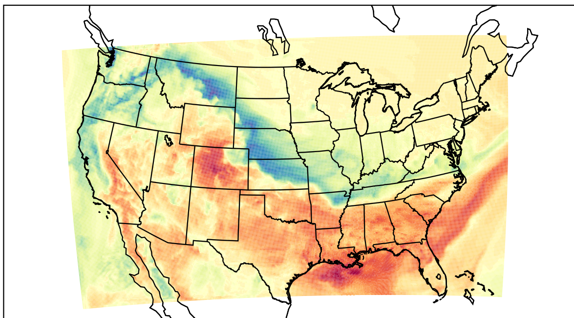
WRF (2022-03-03_19:00:00)
