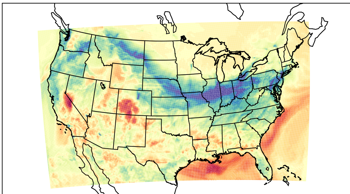
WRF (2022-03-03_03:00:00)
