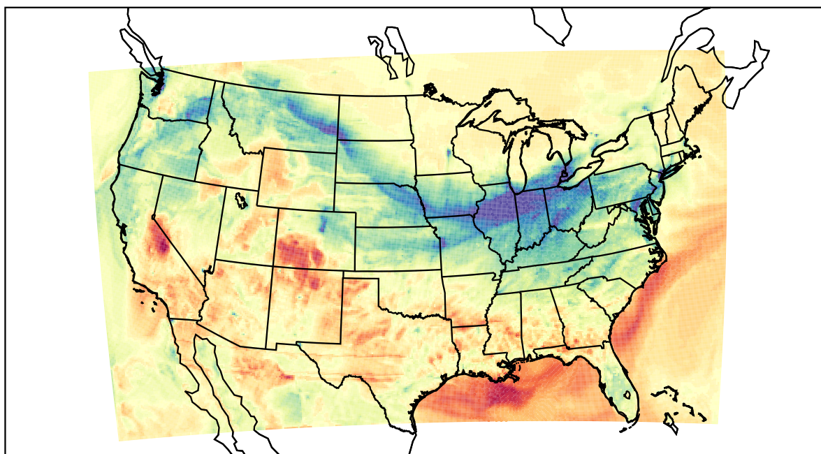
WRF (2022-03-03_01:00:00)
