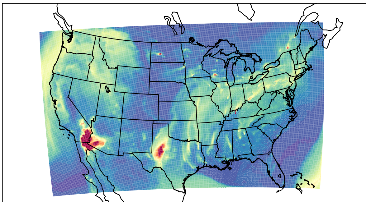
WRF 2022-03-14_10:00:00
