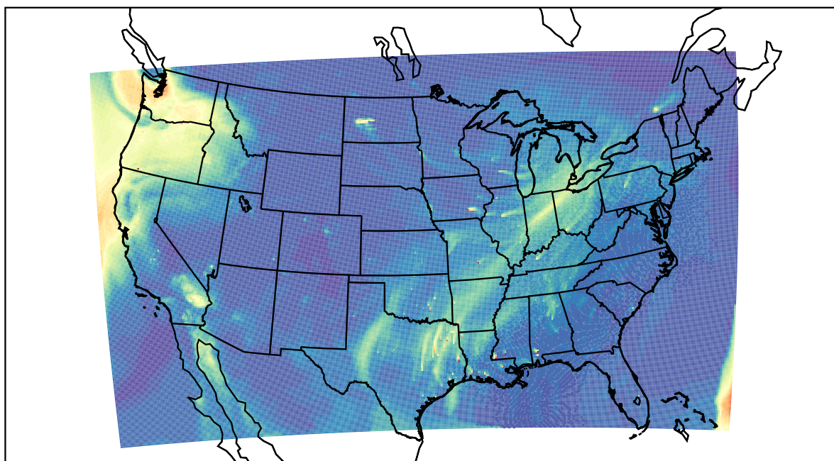
WRF 2022-03-13_20:00:00
