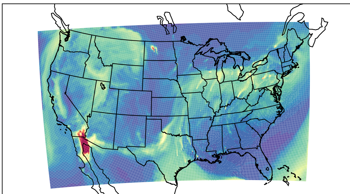
WRF 2022-03-14_18:00:00
