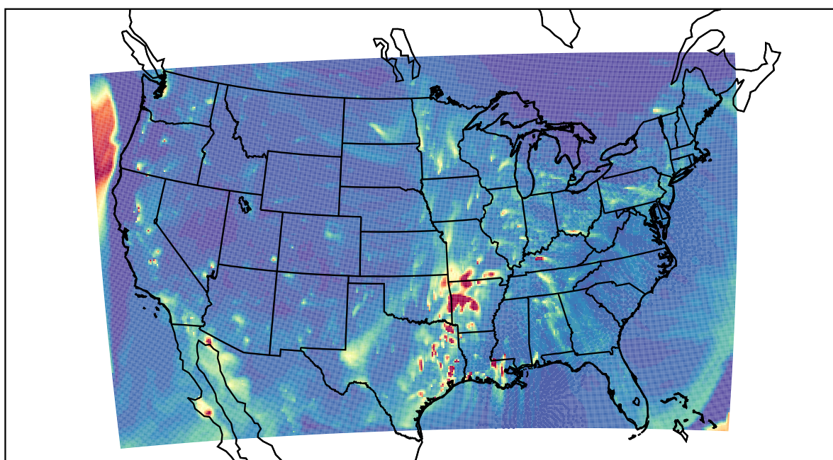
WRF 2022-03-13_03:00:00
