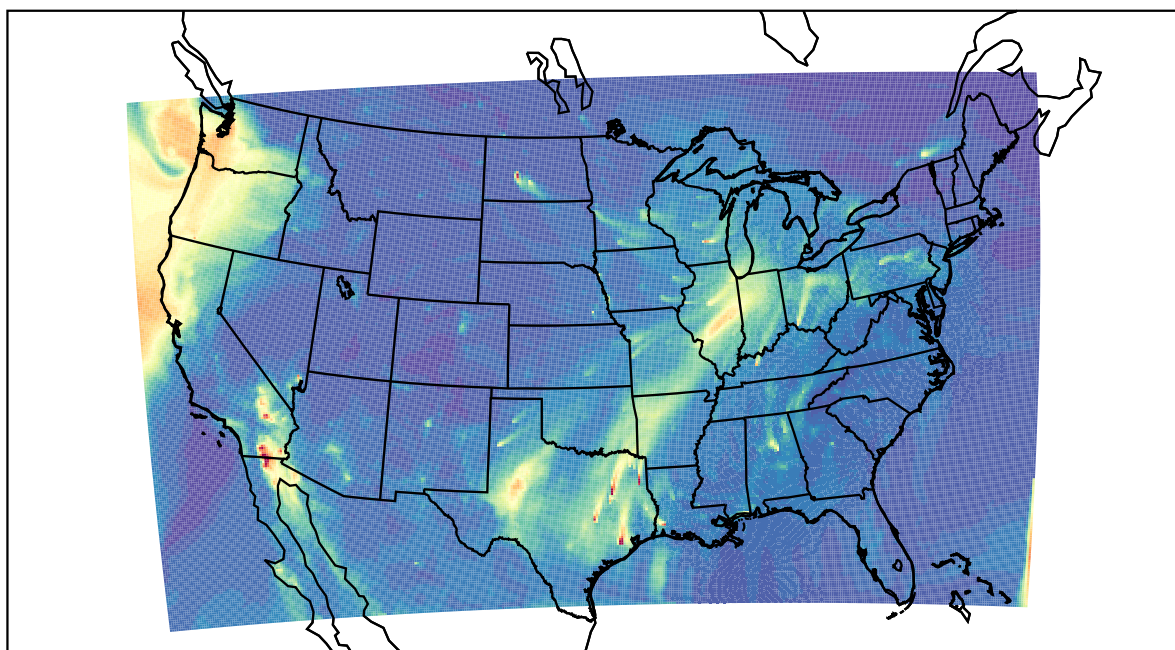
WRF 2022-03-13_15:00:00
