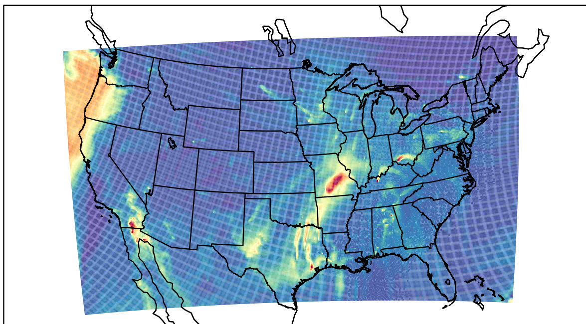
WRF 2022-03-13_10:00:00
