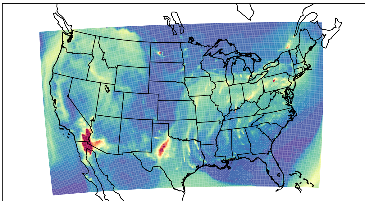
WRF 2022-03-14_14:00:00
