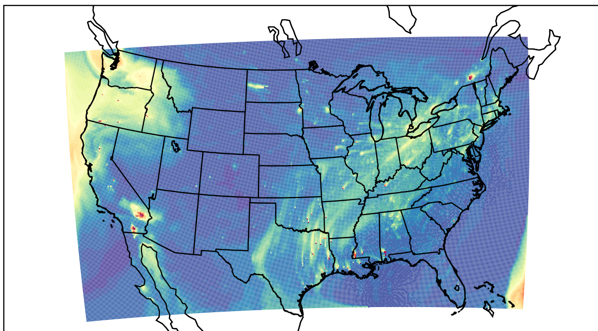
WRF 2022-03-13_23:00:00
