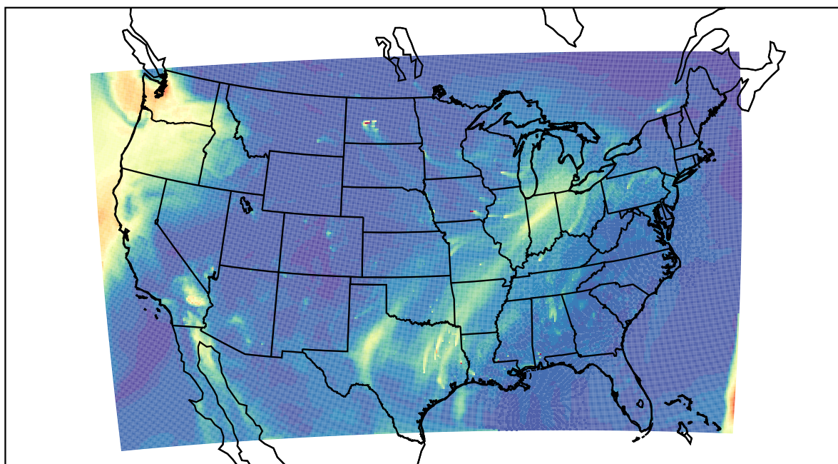
WRF 2022-03-13_18:00:00
