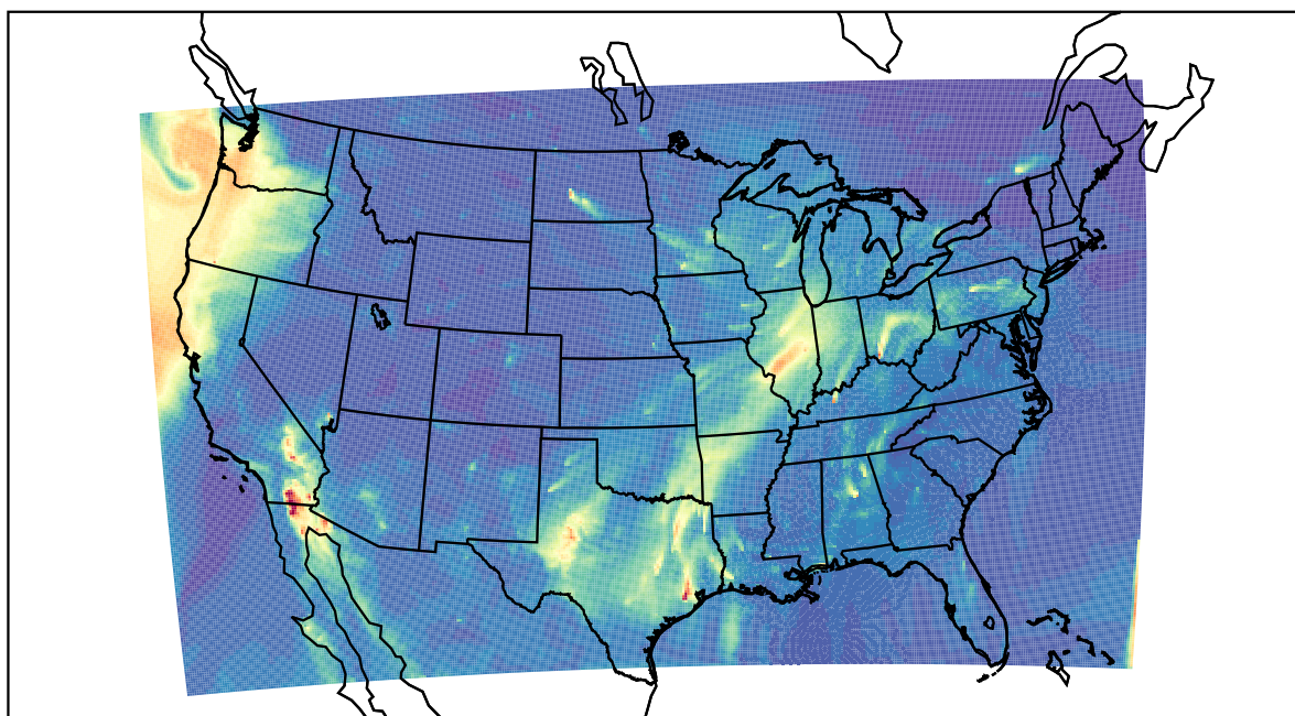
WRF 2022-03-13_14:00:00
