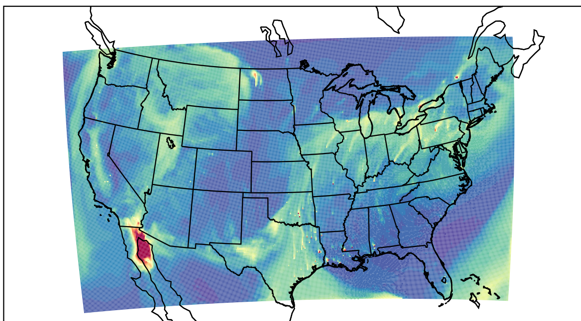
WRF 2022-03-14_20:00:00
