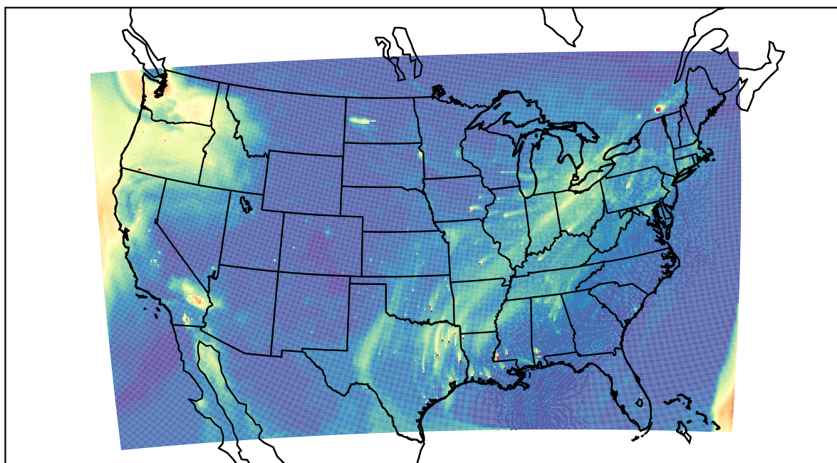
WRF 2022-03-13_22:00:00
