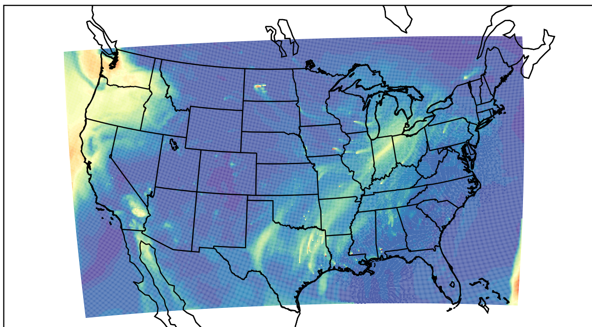
WRF 2022-03-13_19:00:00
