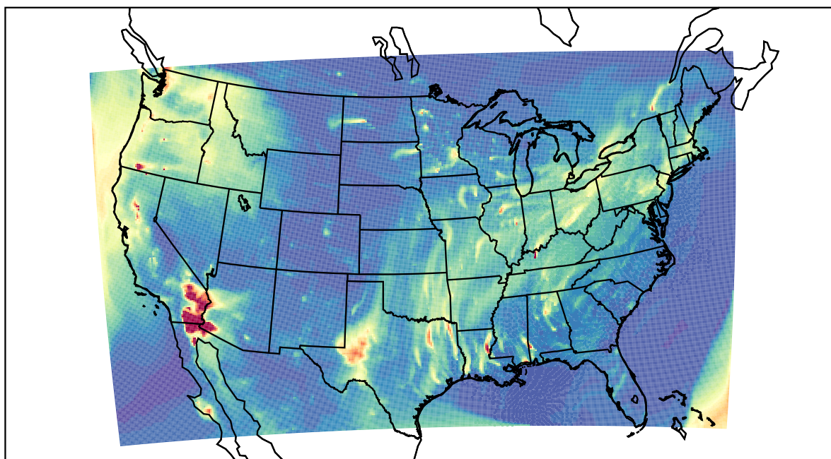
WRF 2022-03-14_04:00:00
