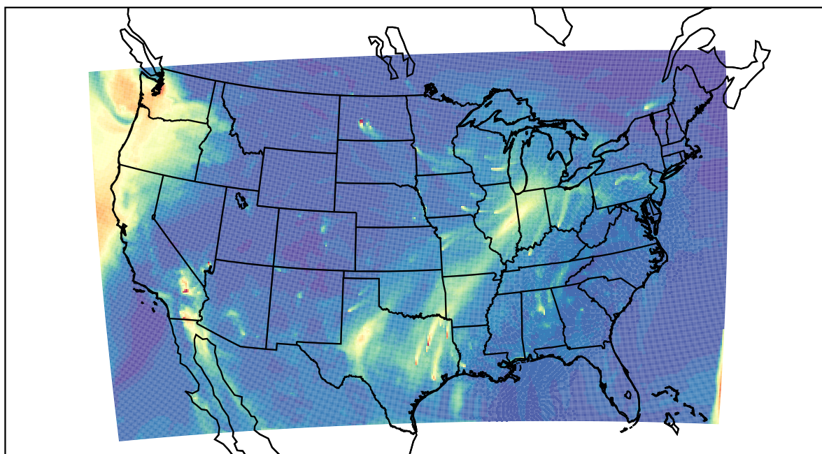
WRF 2022-03-13_16:00:00
