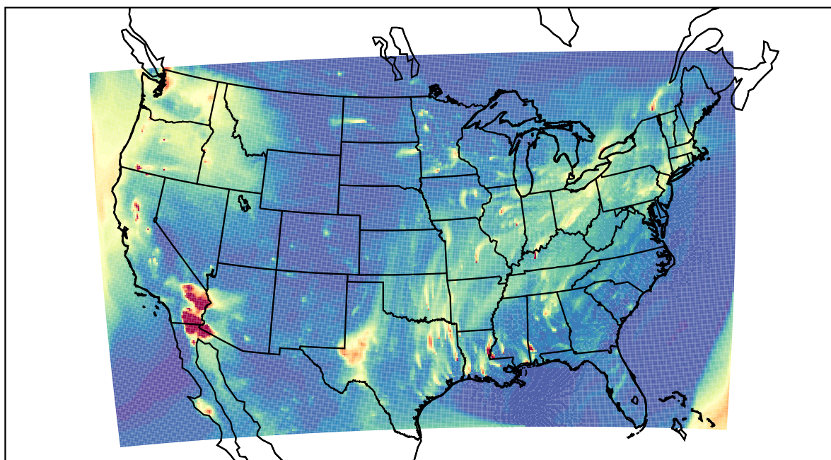
WRF 2022-03-14_03:00:00
