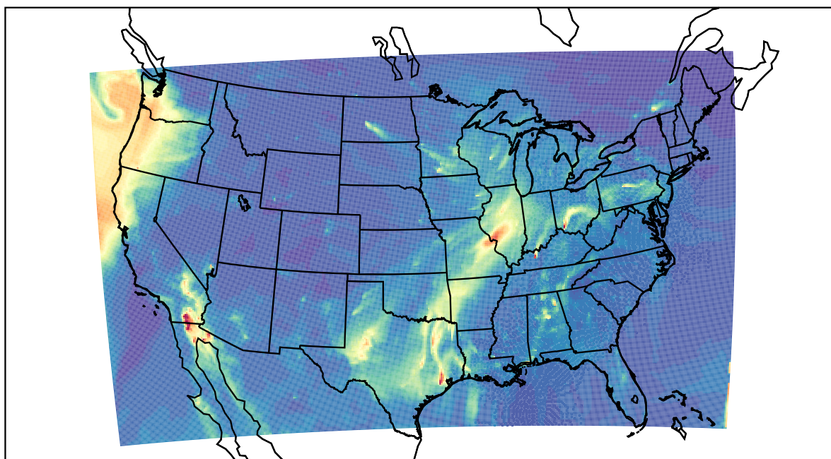
WRF 2022-03-13_13:00:00
