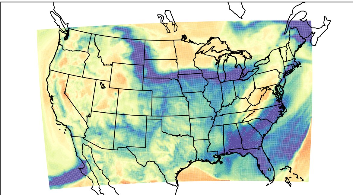
WRF (2022-03-14_10:00:00)
