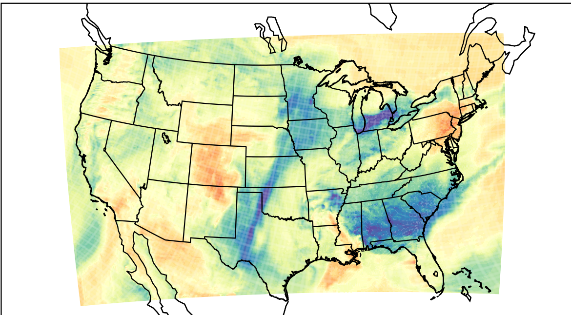
WRF (2022-03-15_20:00:00)
