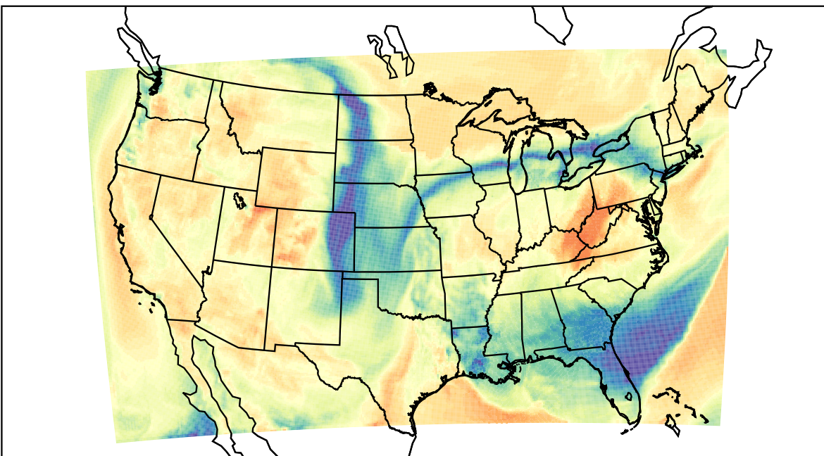
WRF (2022-03-14_20:00:00)
