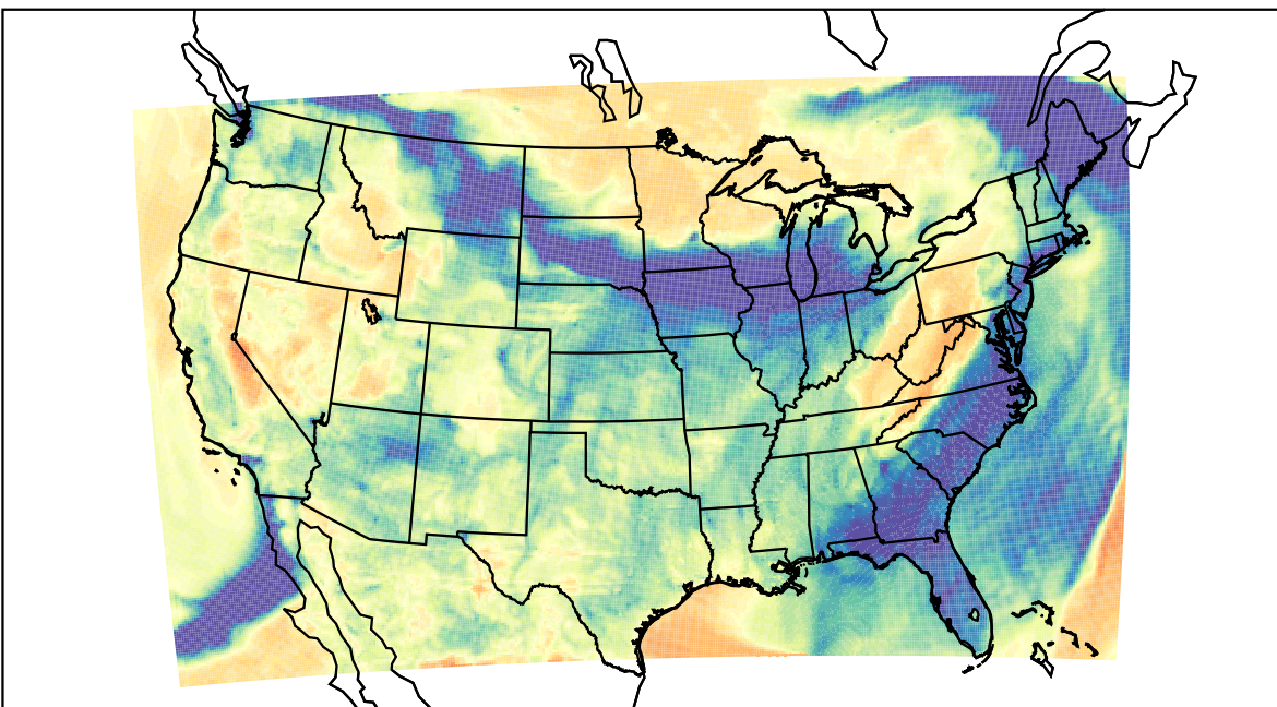
WRF (2022-03-14_04:00:00)
