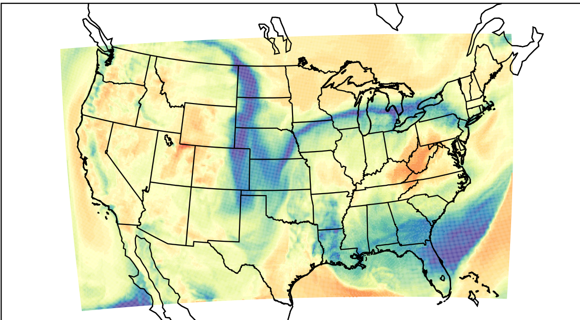
WRF (2022-03-14_18:00:00)
