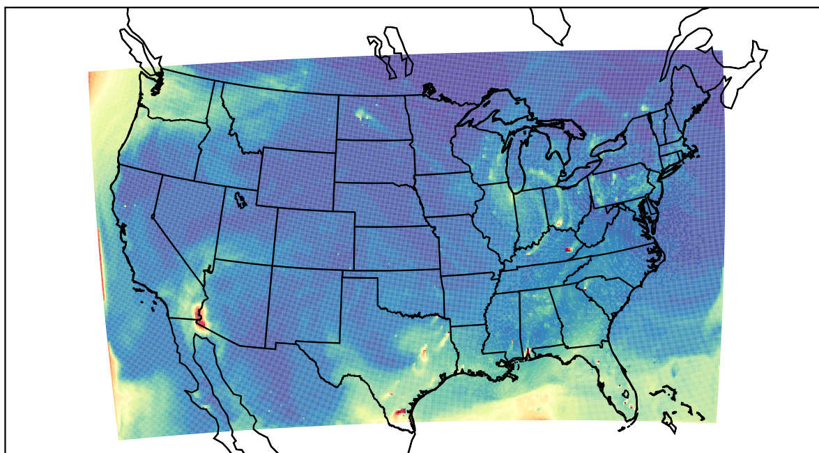
WRF 2022-04-02_23:00:00
