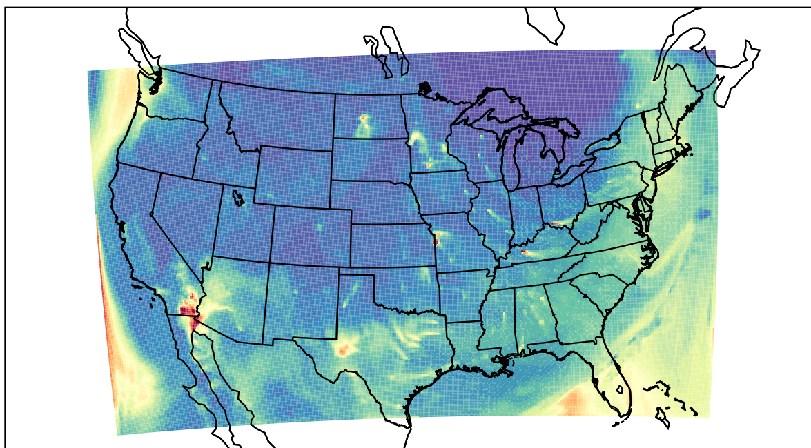
WRF 2022-04-01_13:00:00
