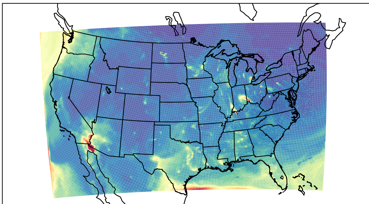
WRF 2022-04-02_13:00:00
