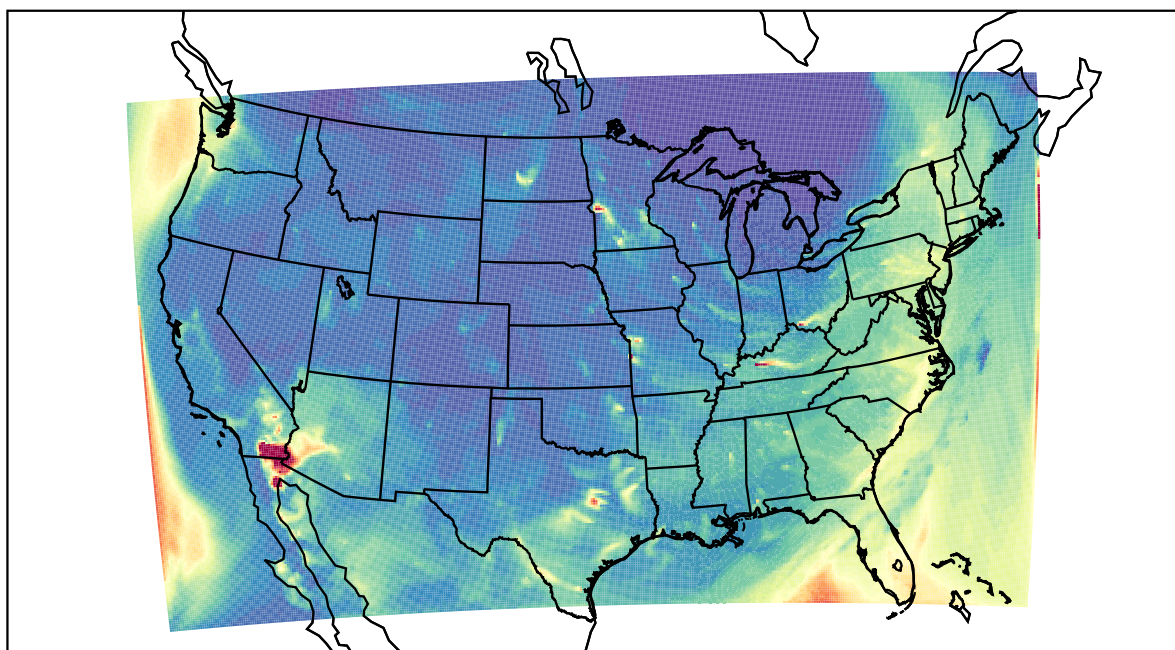
WRF 2022-04-01_08:00:00
