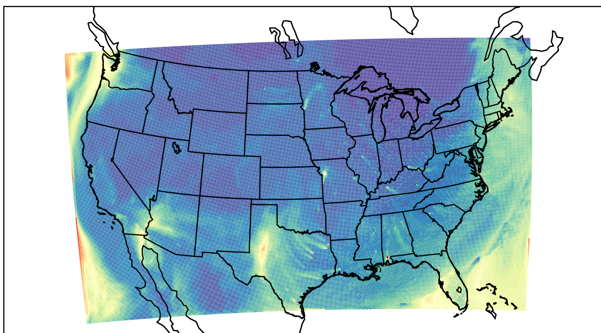
WRF 2022-04-01_19:00:00
