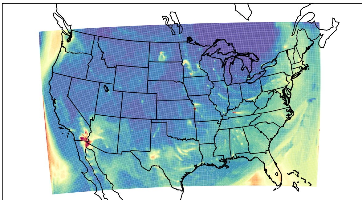
WRF 2022-04-01_12:00:00
