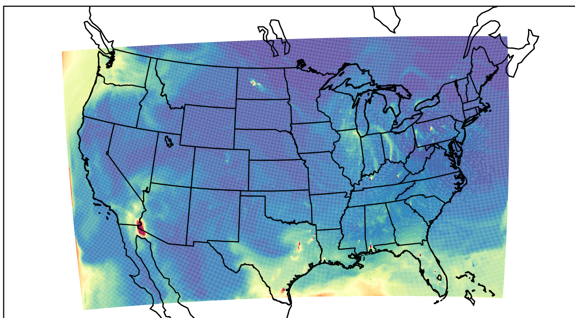
WRF 2022-04-02_20:00:00
