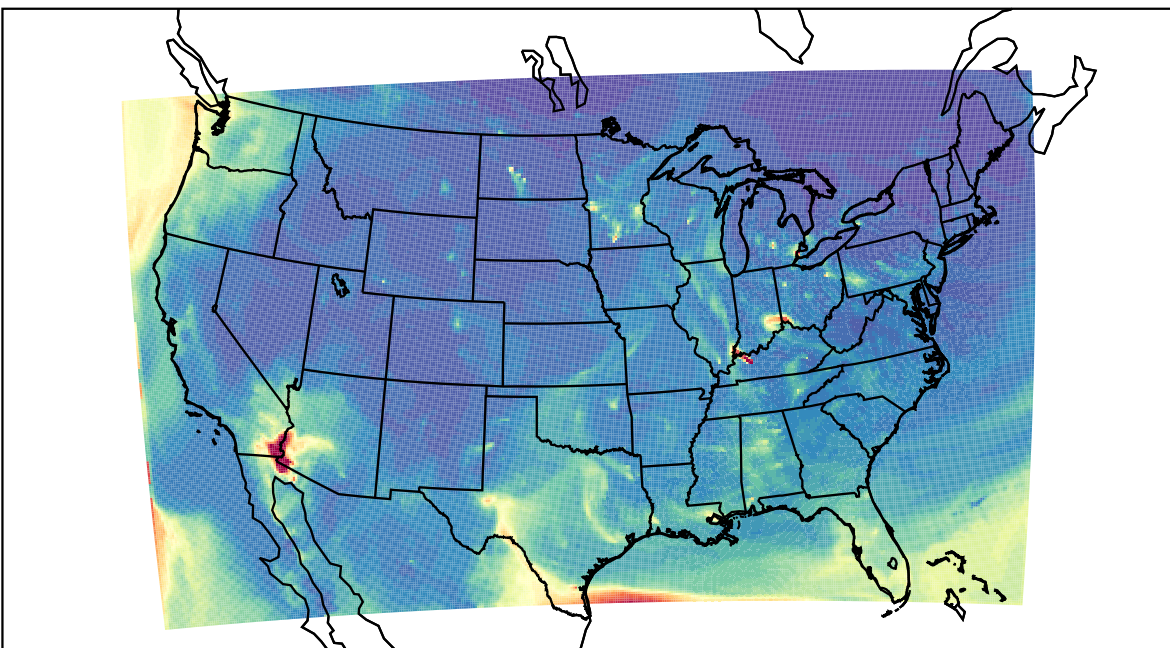
WRF 2022-04-02_10:00:00
