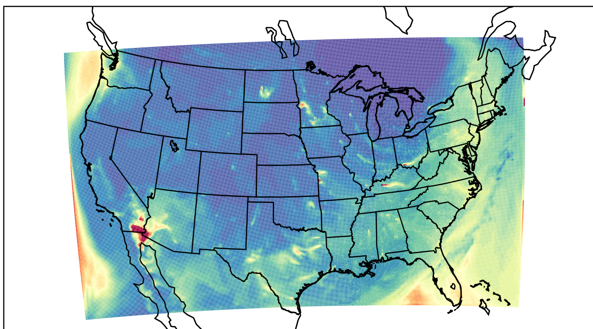
WRF 2022-04-01_10:00:00
