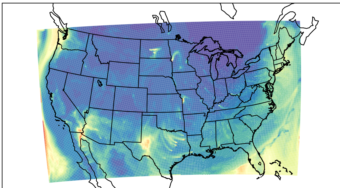
WRF 2022-04-01_16:00:00
