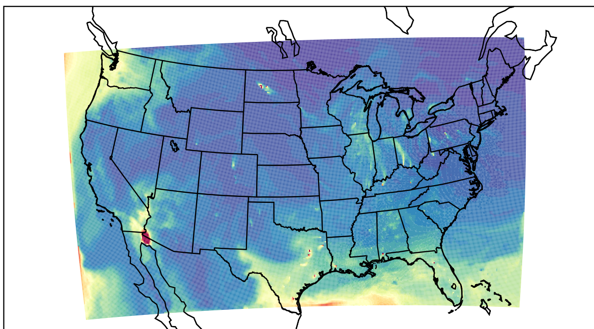
WRF 2022-04-02_18:00:00
