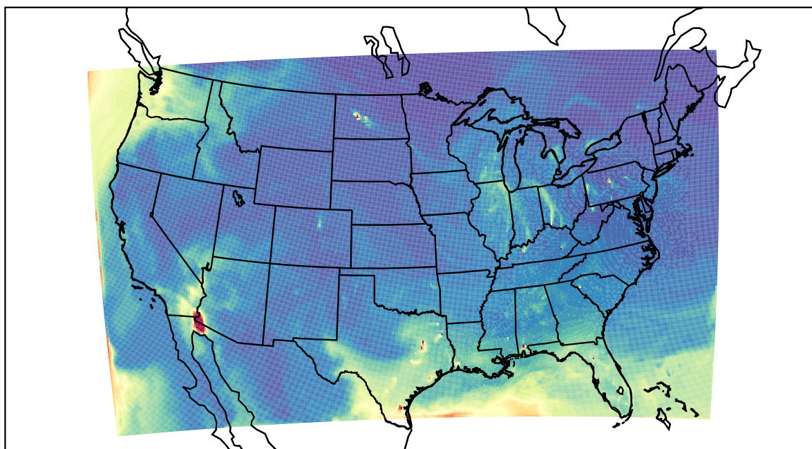
WRF 2022-04-02_19:00:00
