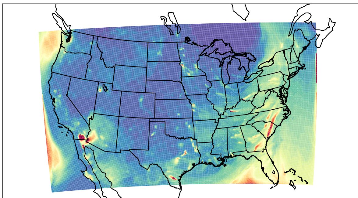
WRF 2022-04-01_04:00:00
