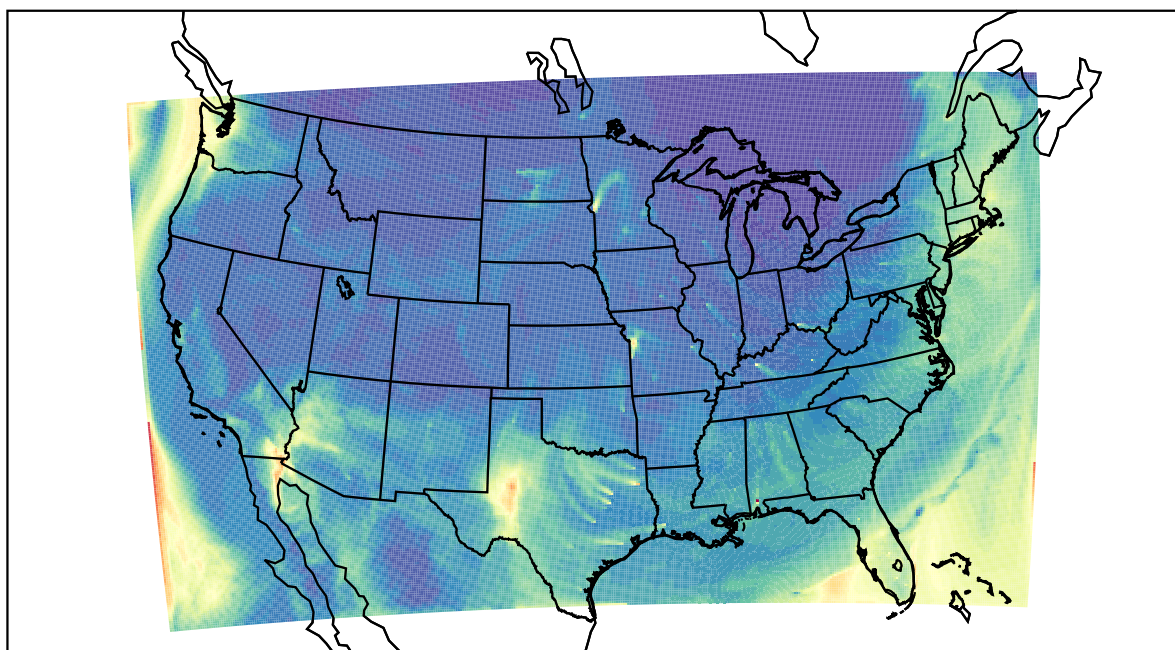
WRF 2022-04-01_17:00:00
