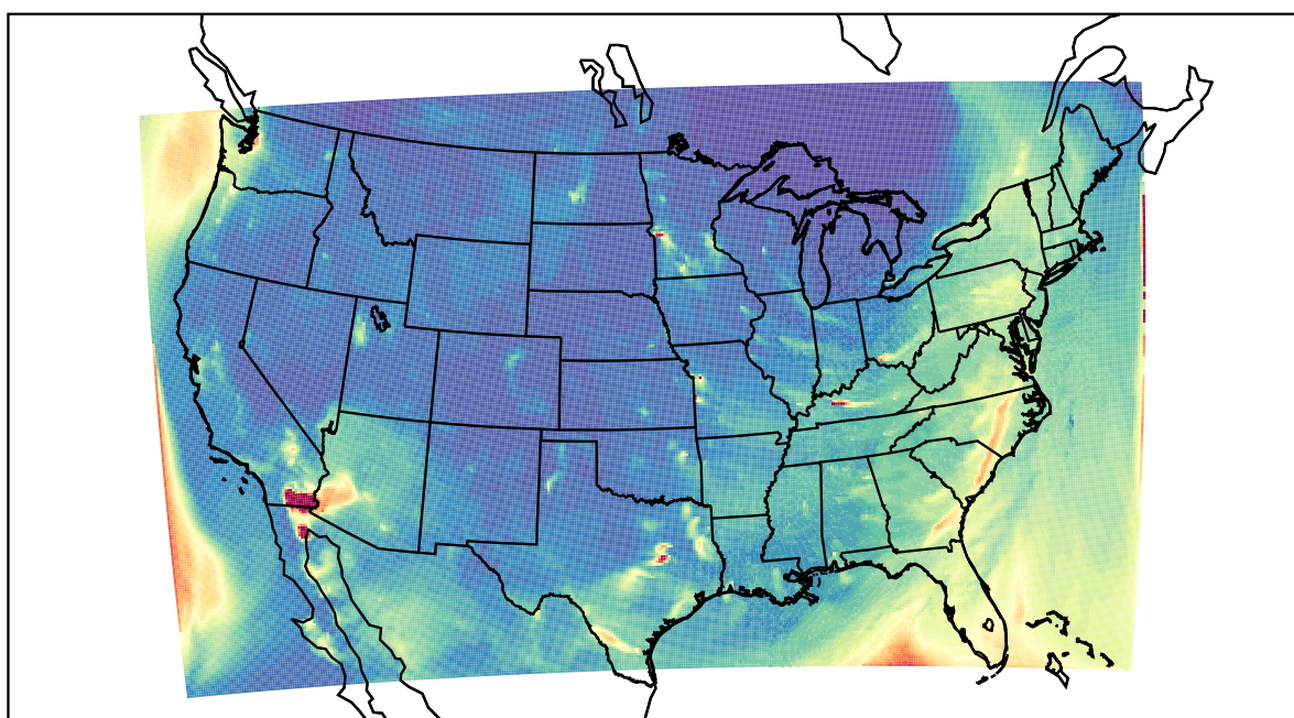
WRF 2022-04-01_06:00:00
