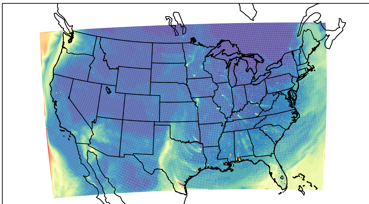
WRF 2022-04-01_23:00:00
