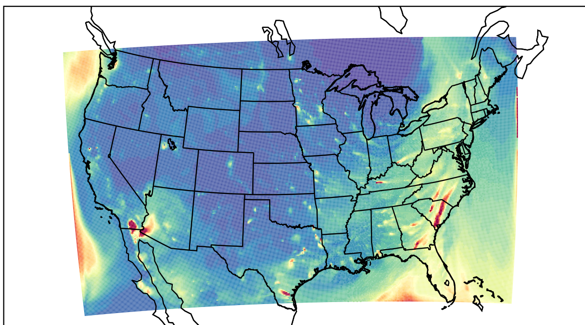
WRF 2022-04-01_03:00:00
