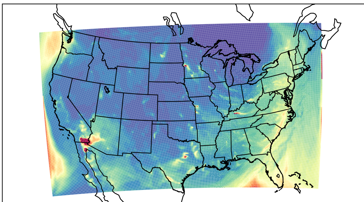
WRF 2022-04-01_07:00:00
