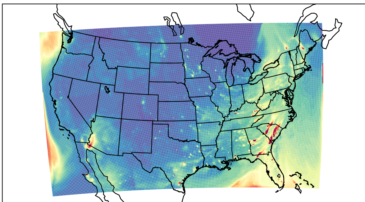
WRF 2022-04-01_01:00:00
