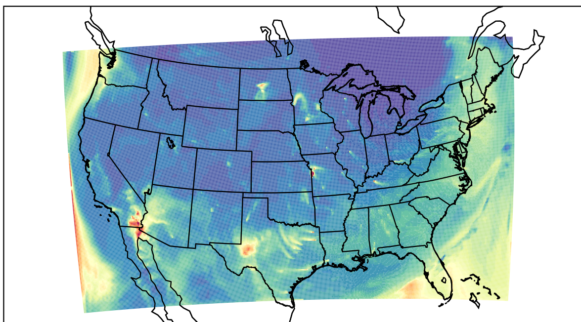
WRF 2022-04-01_14:00:00
