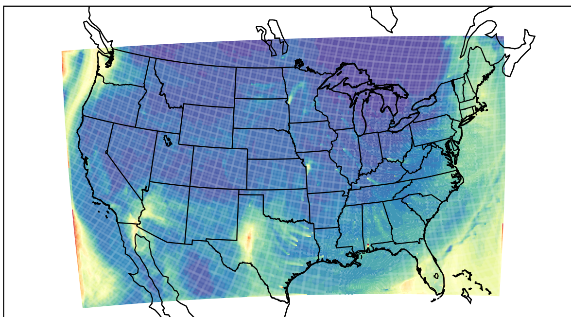
WRF 2022-04-01_18:00:00
