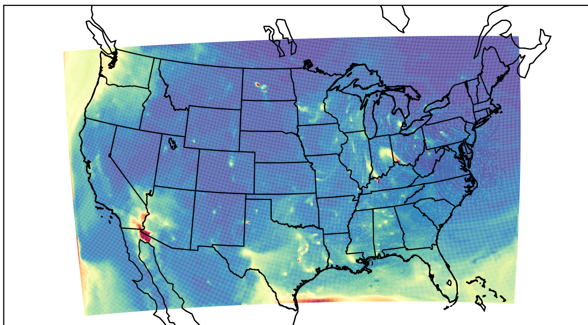
WRF 2022-04-02_14:00:00
