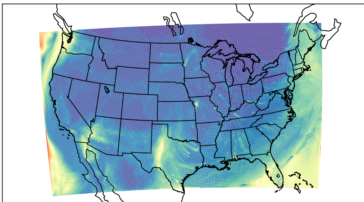
WRF 2022-04-01_20:00:00
