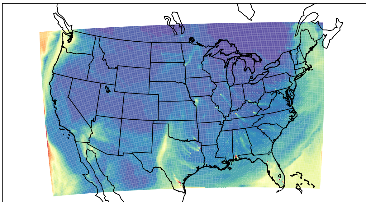
WRF 2022-04-01_22:00:00
