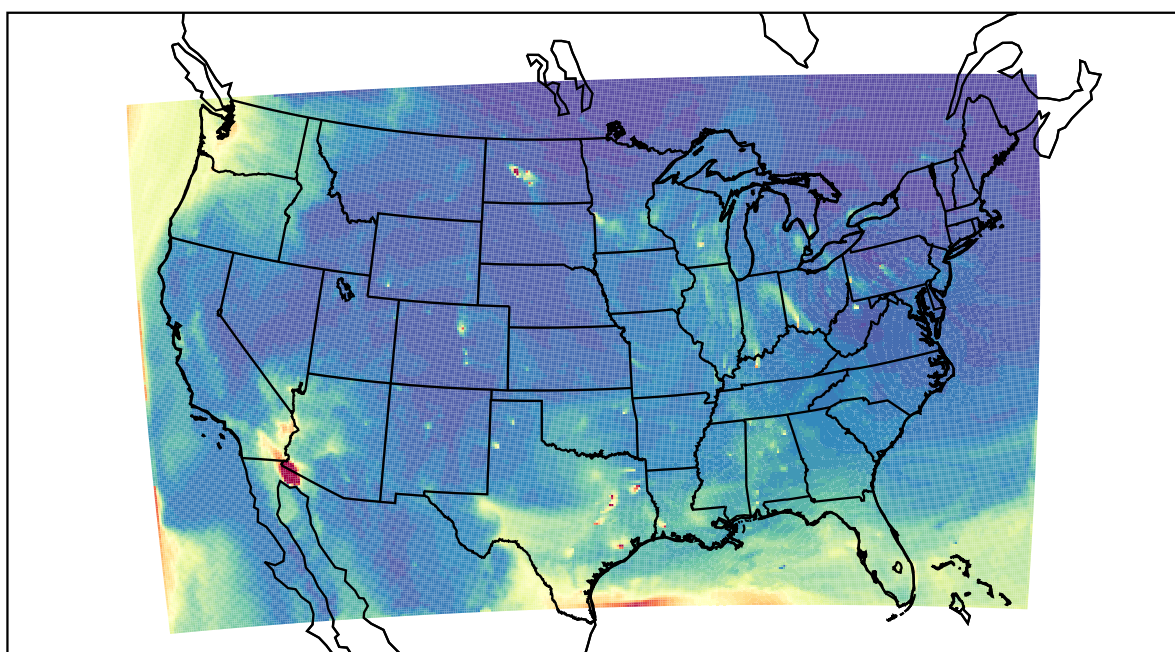
WRF 2022-04-02_16:00:00
