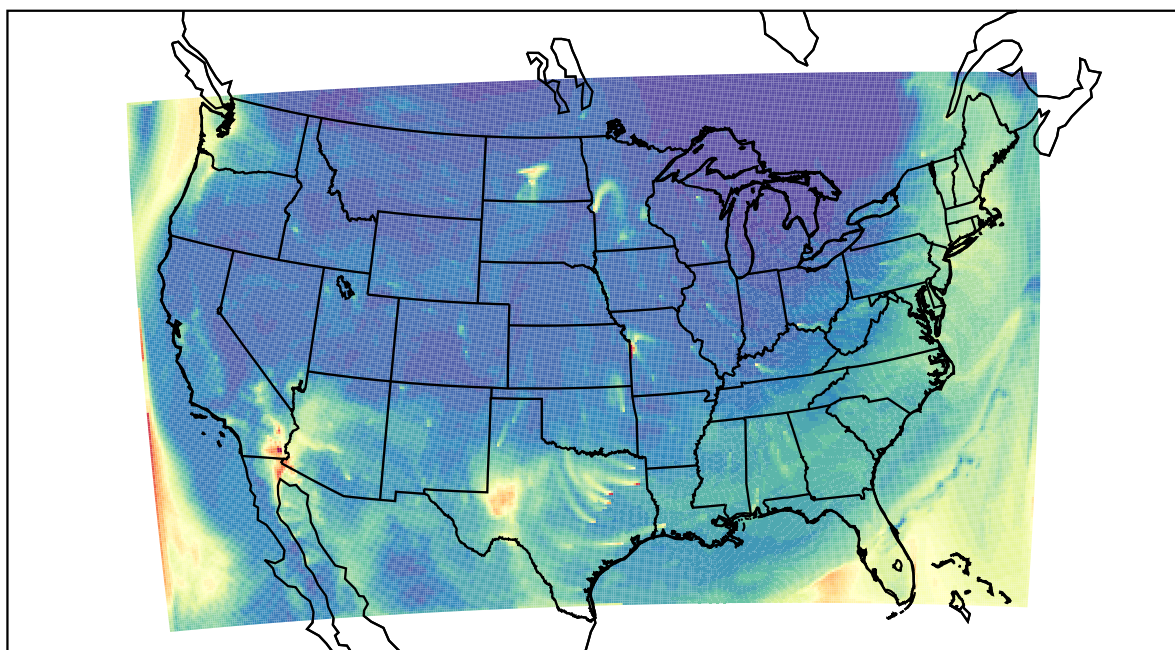
WRF 2022-04-01_15:00:00
