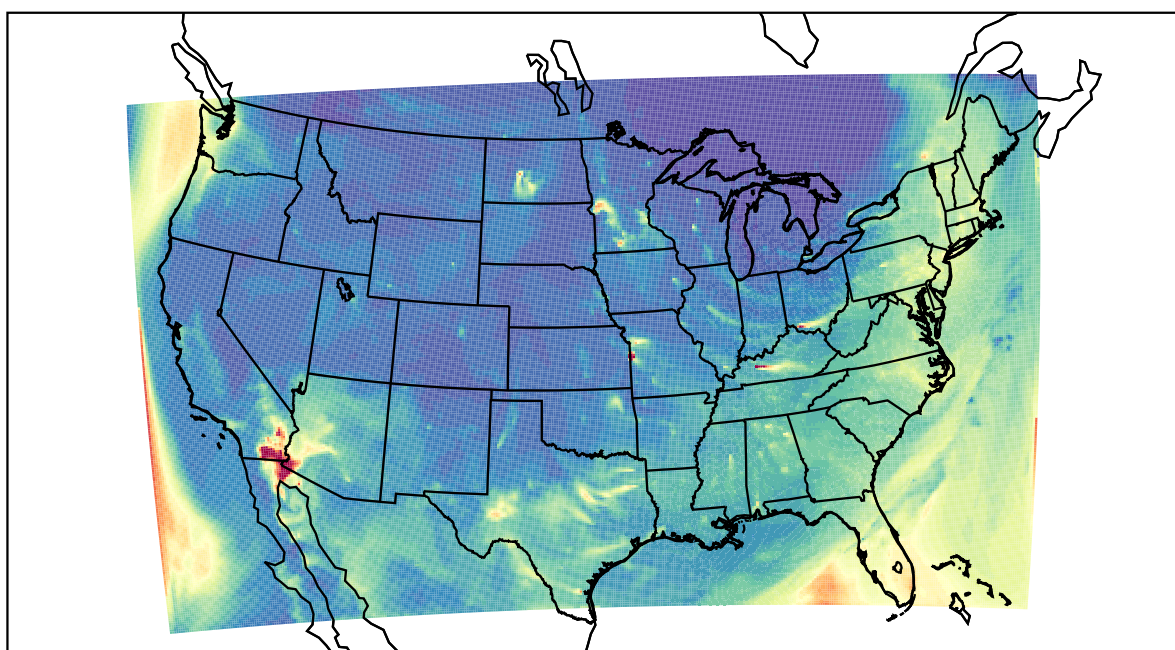
WRF 2022-04-01_11:00:00
