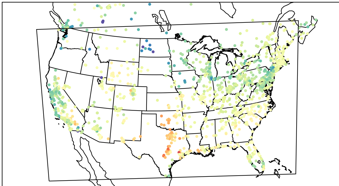
AirNOW (2022-04-03_18:00:00)
