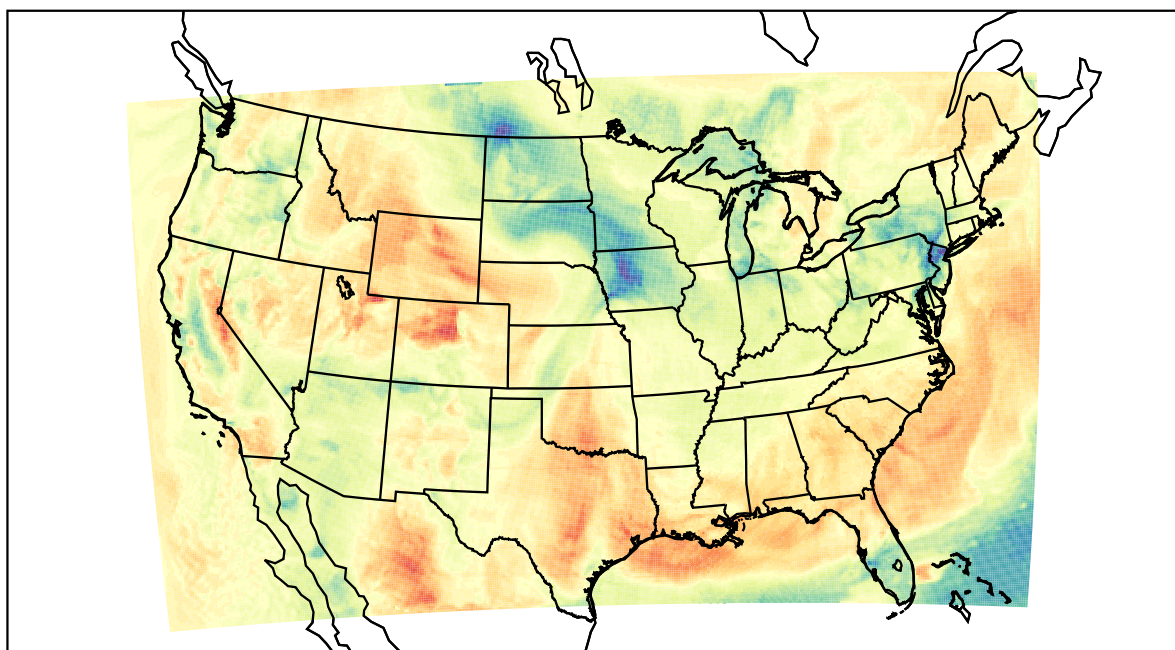
WRF (2022-04-03_18:00:00)
