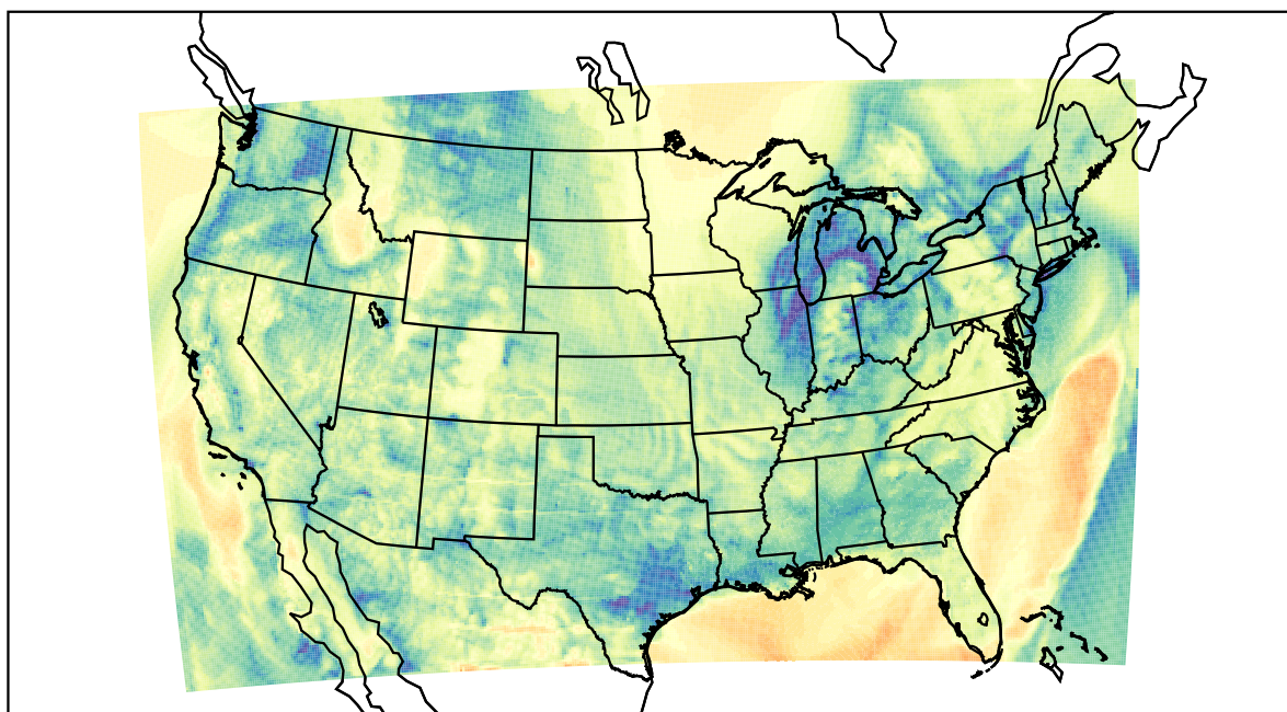
WRF (2022-04-08_14:00:00)
