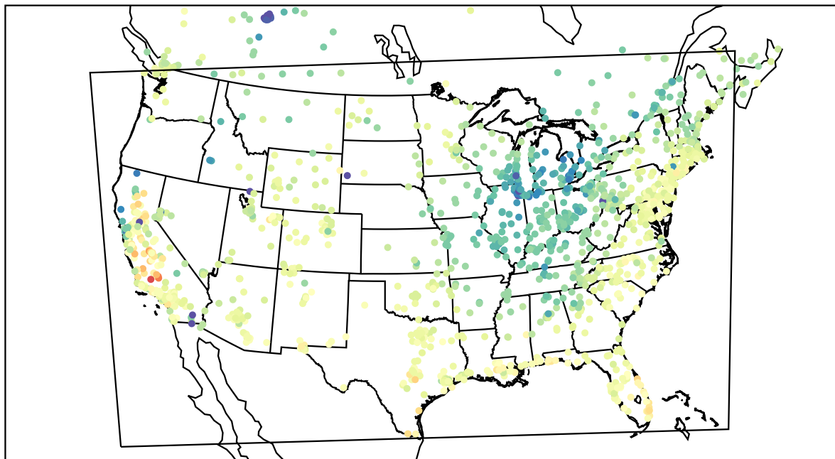
AirNOW (2022-04-08_18:00:00)
