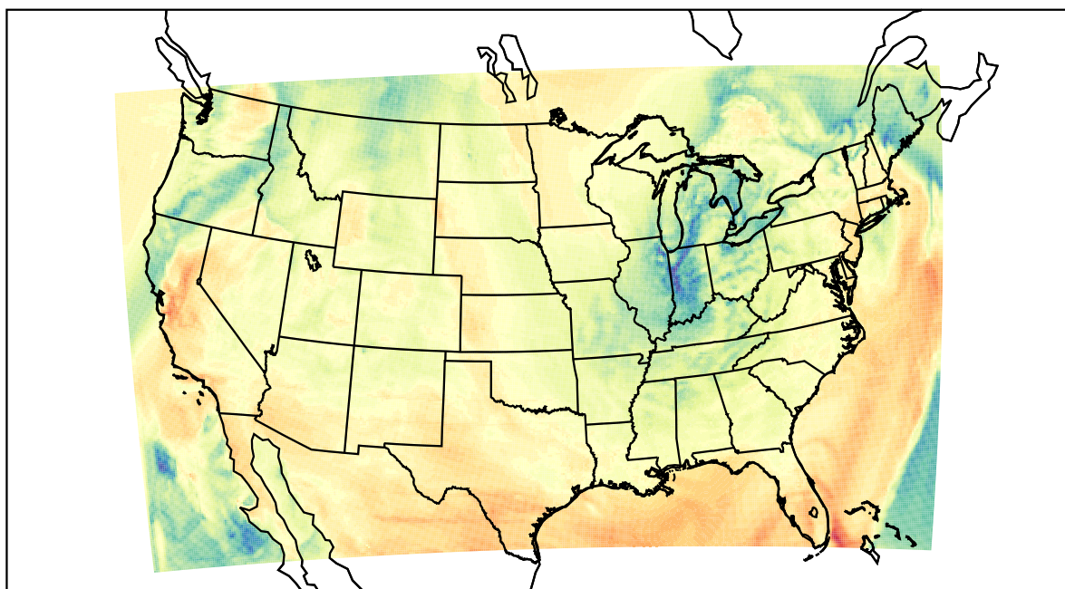
WRF (2022-04-08_20:00:00)
