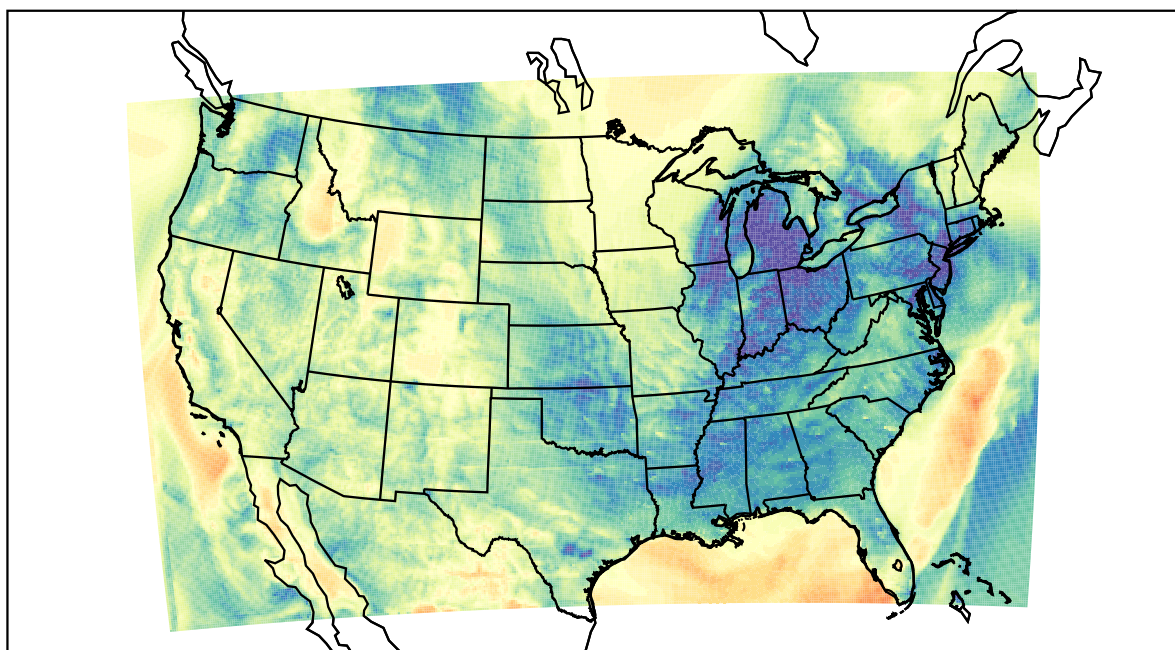
WRF (2022-04-08_10:00:00)
