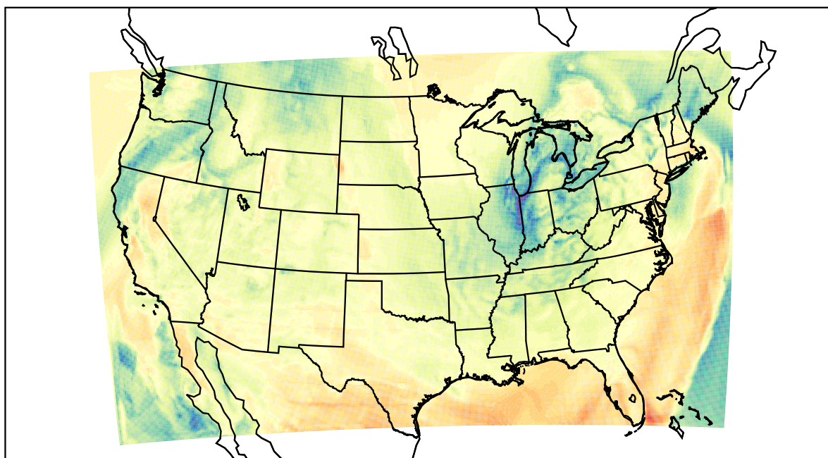
WRF (2022-04-08_18:00:00)
