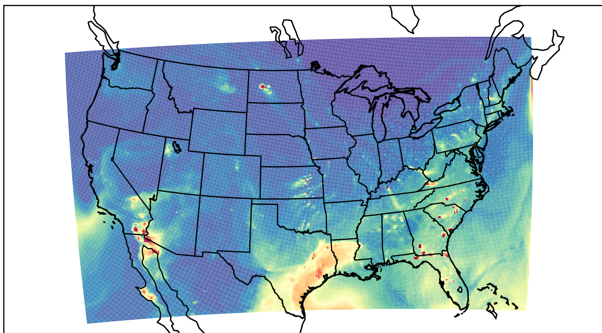
WRF 2022-04-17_00:00:00
