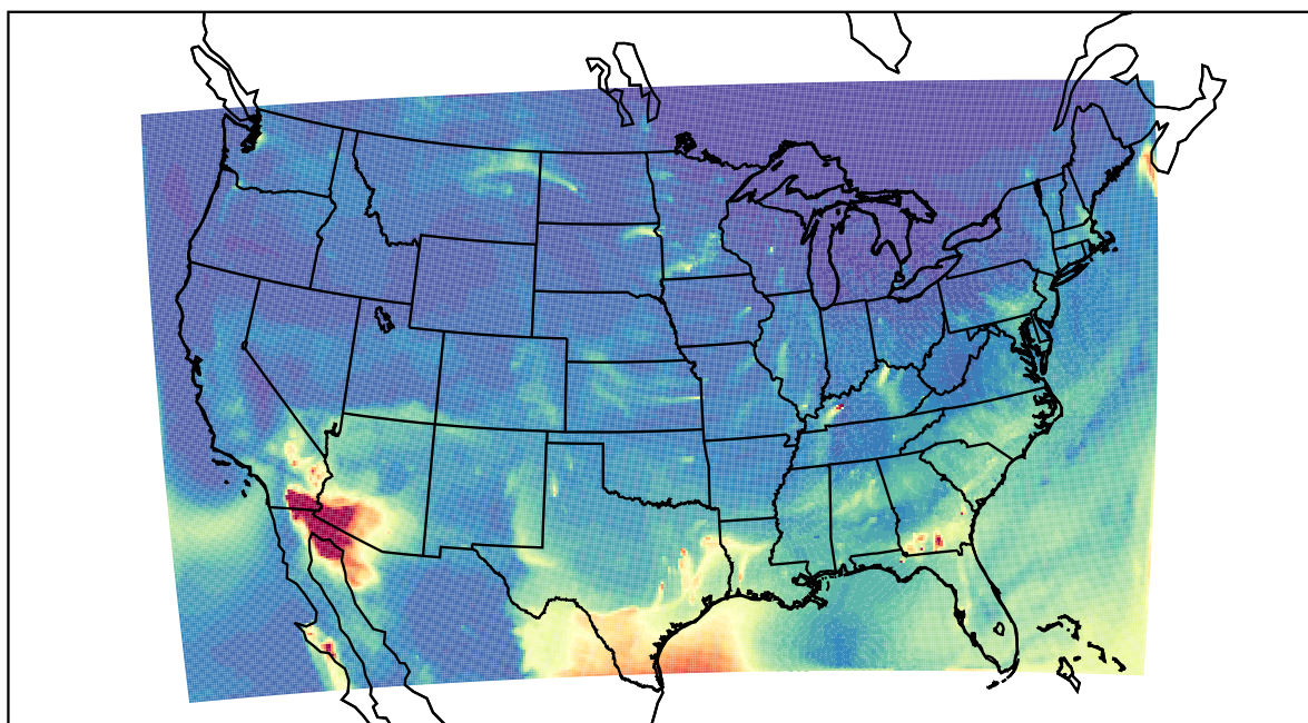
WRF 2022-04-17_09:00:00
