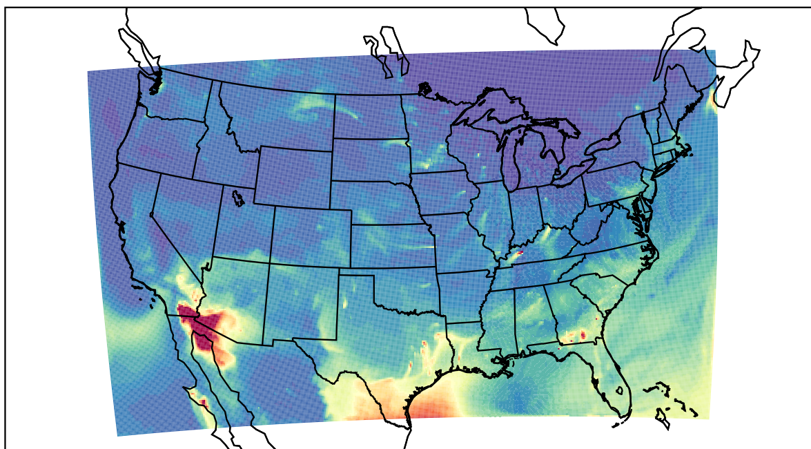
WRF 2022-04-17_10:00:00
