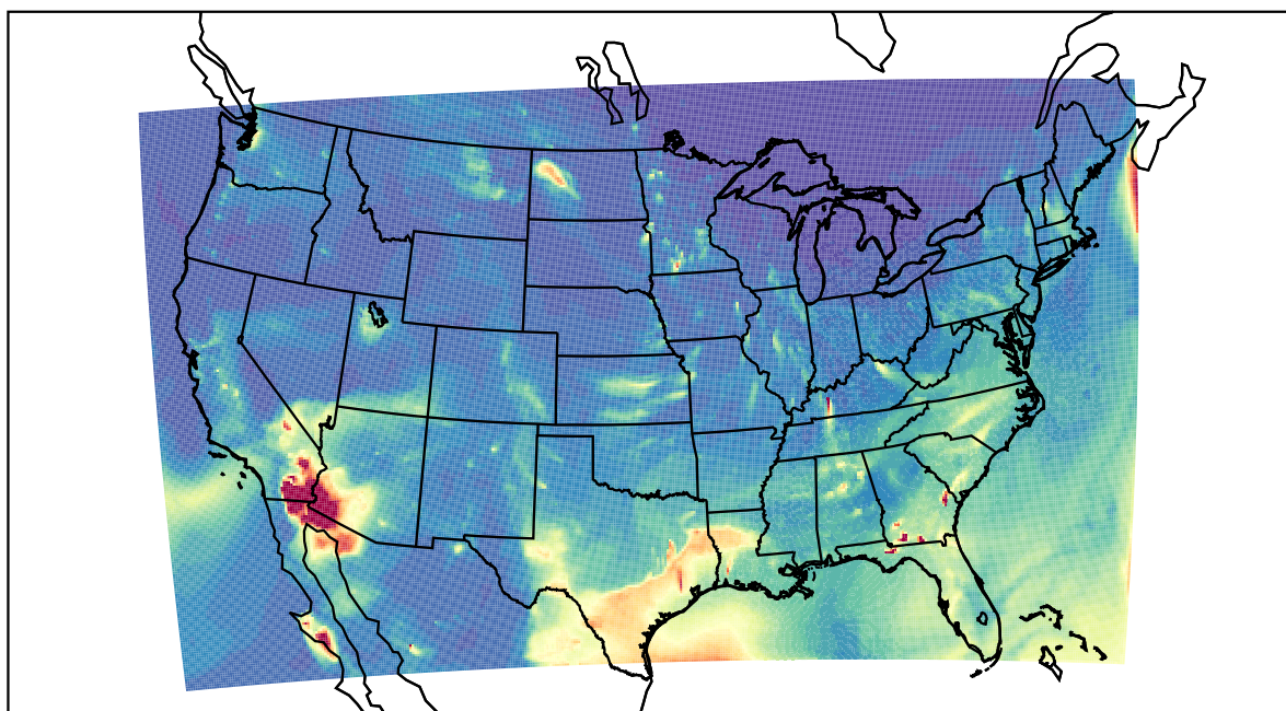
WRF 2022-04-17_04:00:00
