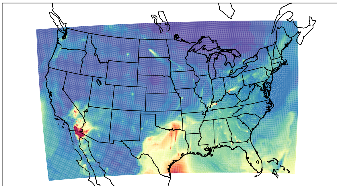
WRF 2022-04-16_10:00:00
