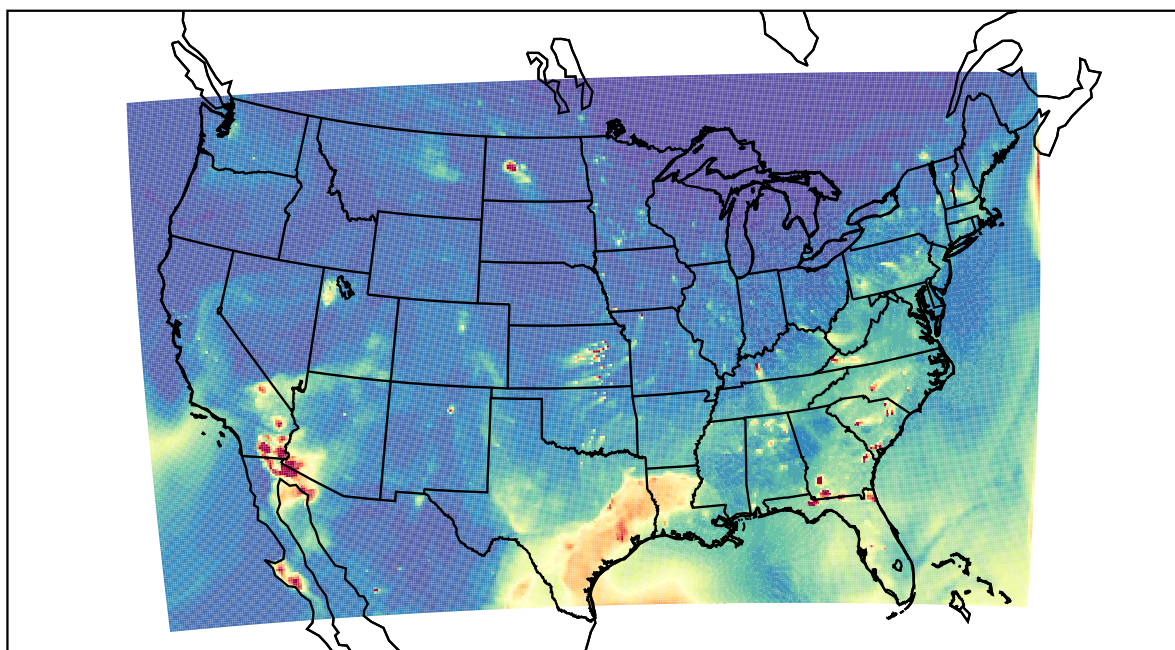
WRF 2022-04-17_01:00:00
