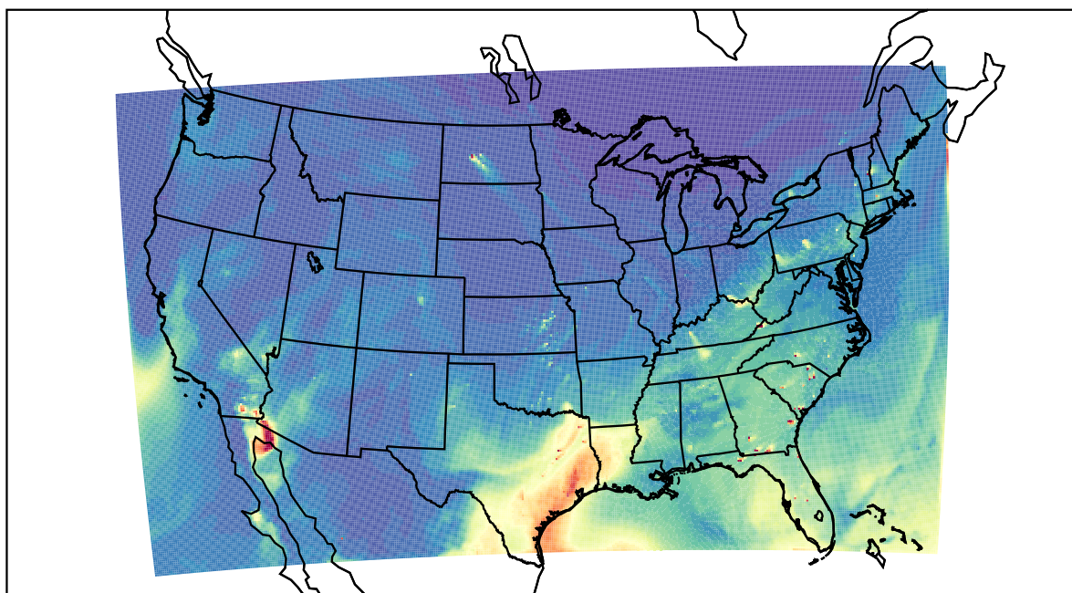
WRF 2022-04-16_20:00:00
