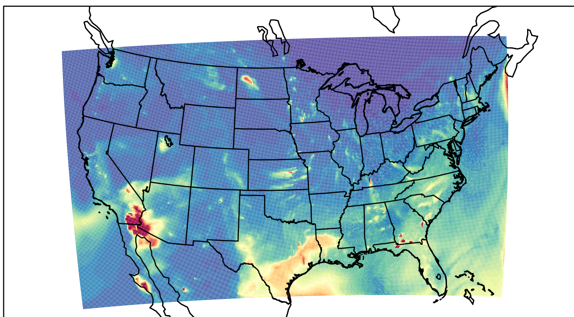
WRF 2022-04-17_03:00:00
