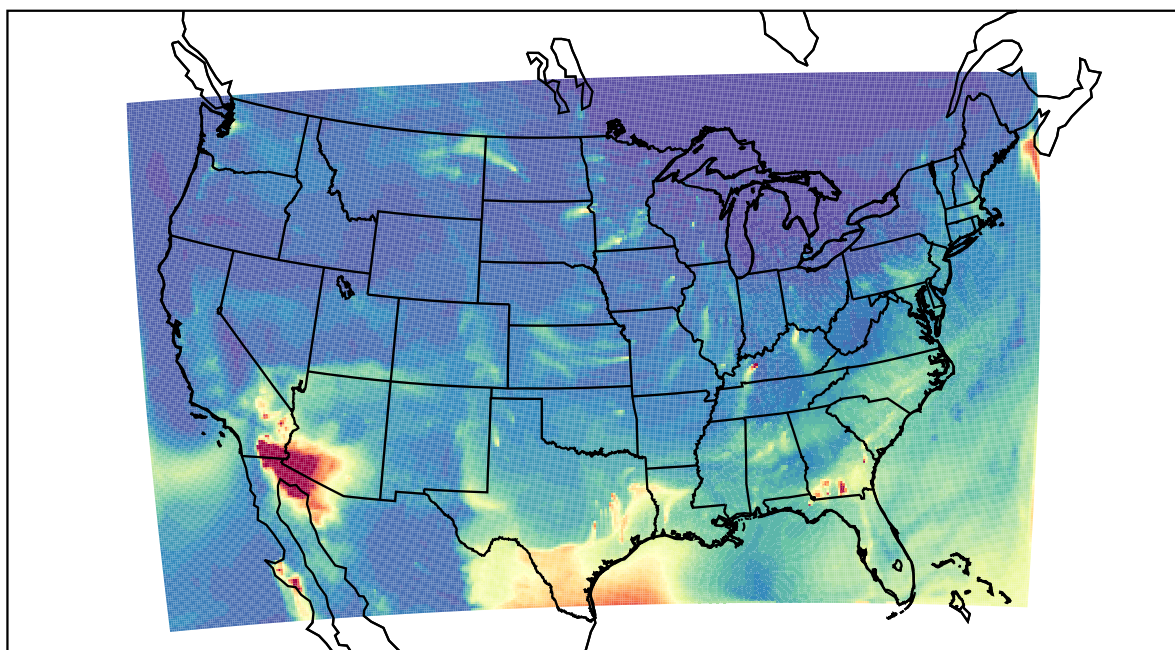
WRF 2022-04-17_08:00:00
