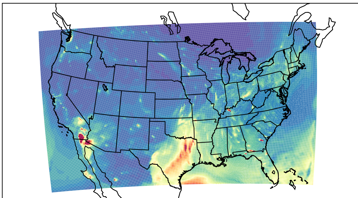
WRF 2022-04-16_03:00:00
