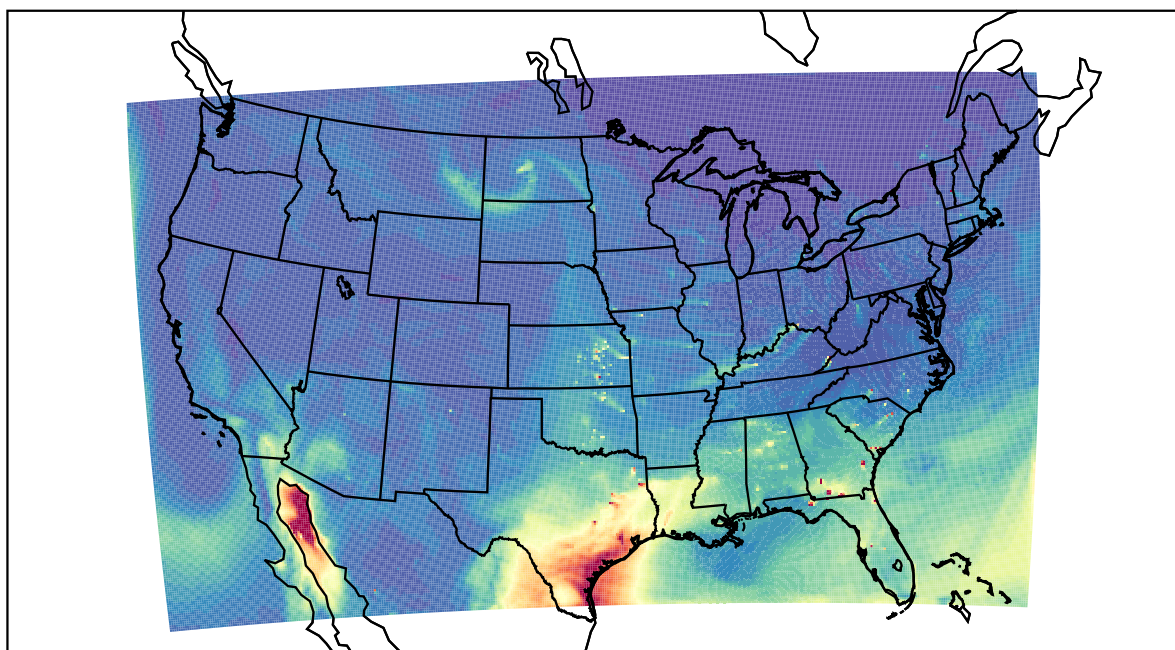
WRF 2022-04-17_20:00:00
