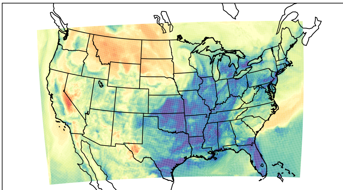
WRF (2022-04-18_10:00:00)
