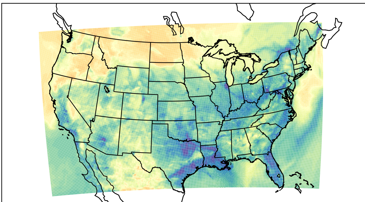
WRF (2022-04-17_04:00:00)
