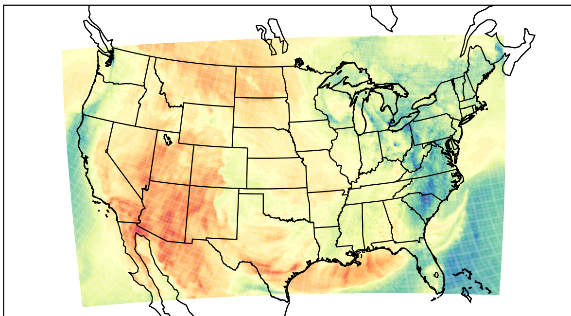
WRF (2022-04-18_23:00:00)
