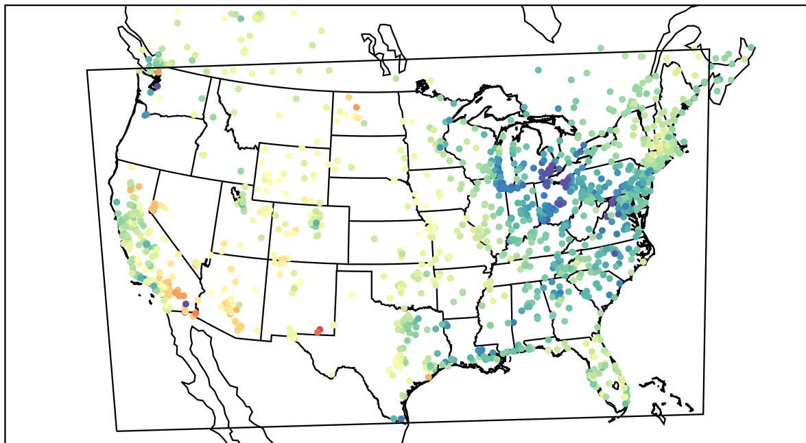
AirNOW (2022-04-18_18:00:00)
