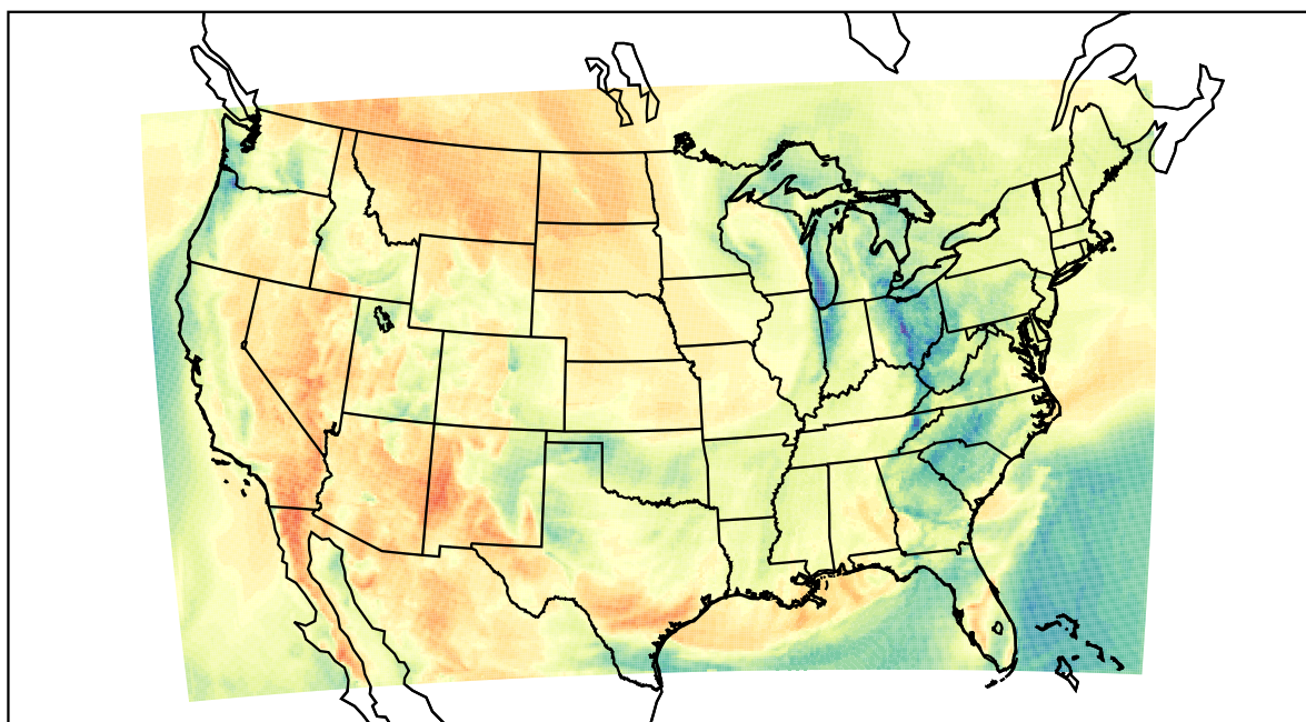
WRF (2022-04-18_18:00:00)
