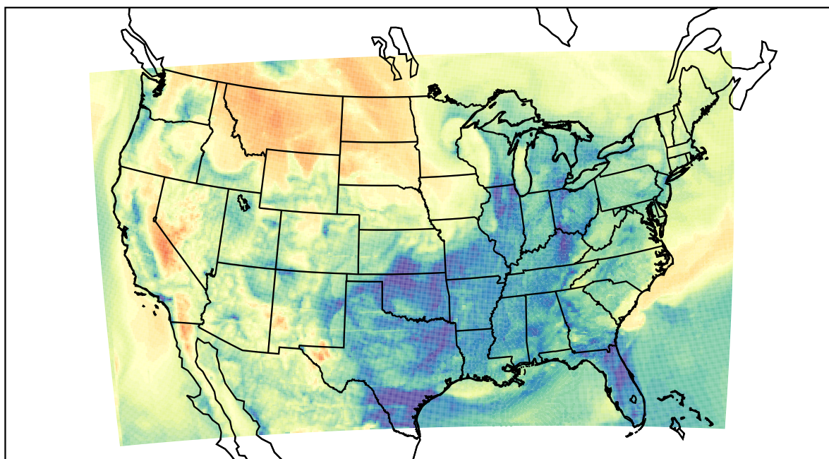
WRF (2022-04-18_13:00:00)
