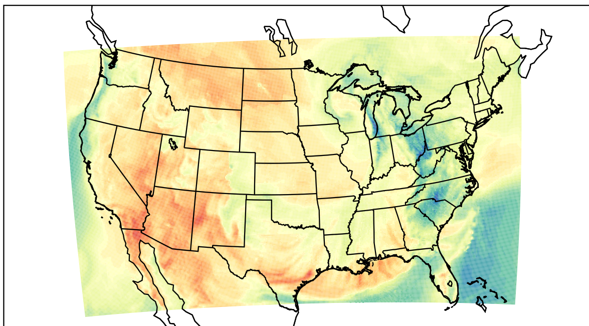
WRF (2022-04-18_20:00:00)
