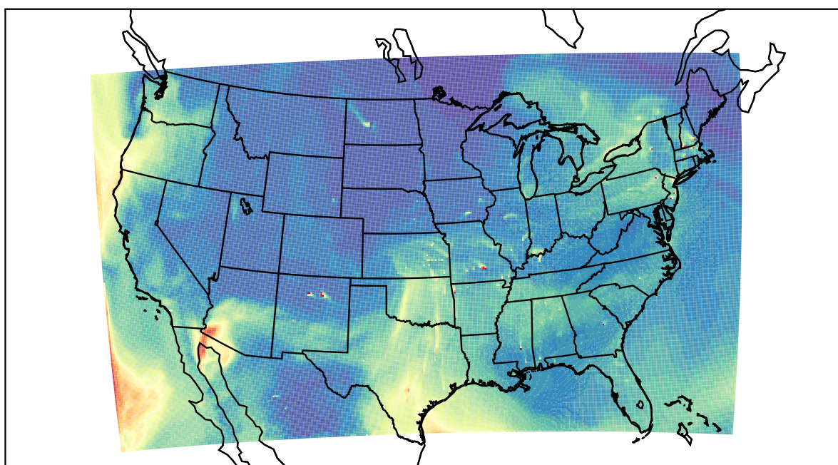
WRF 2022-05-02_20:00:00
