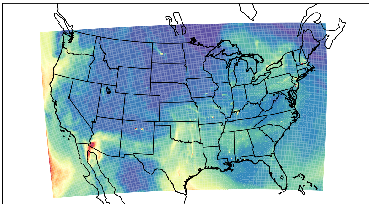
WRF 2022-05-02_19:00:00
