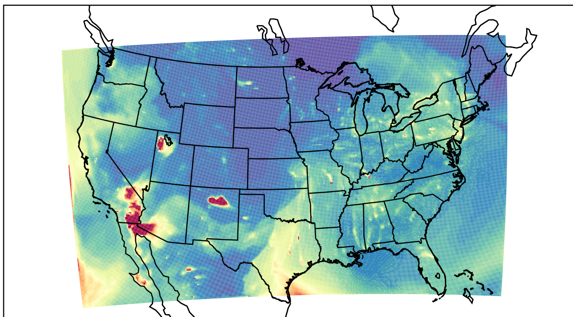
WRF 2022-05-03_03:00:00
