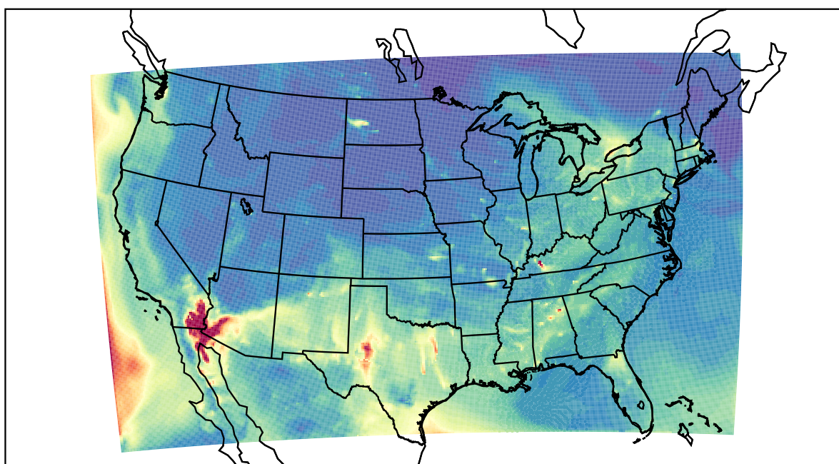
WRF 2022-05-02_10:00:00
