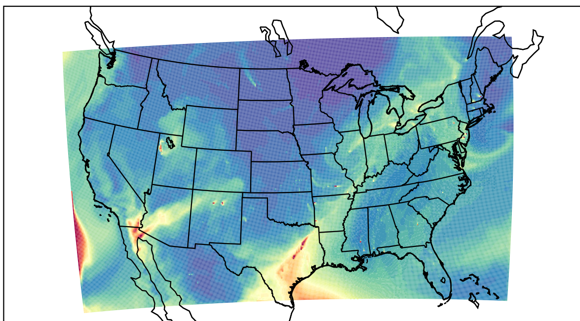
WRF 2022-05-03_19:00:00
