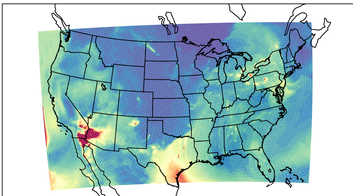
WRF 2022-05-03_10:00:00
