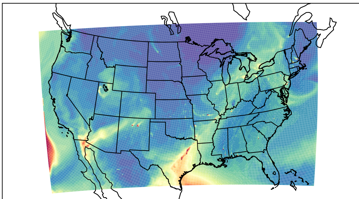
WRF 2022-05-03_20:00:00
