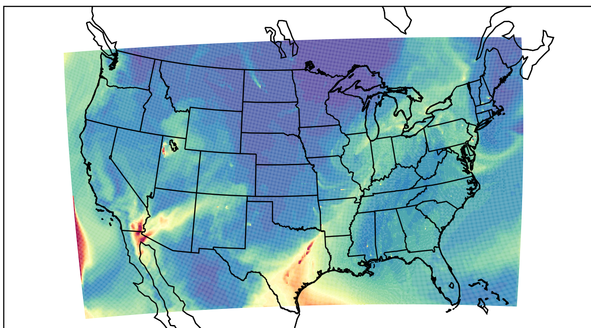
WRF 2022-05-03_18:00:00
