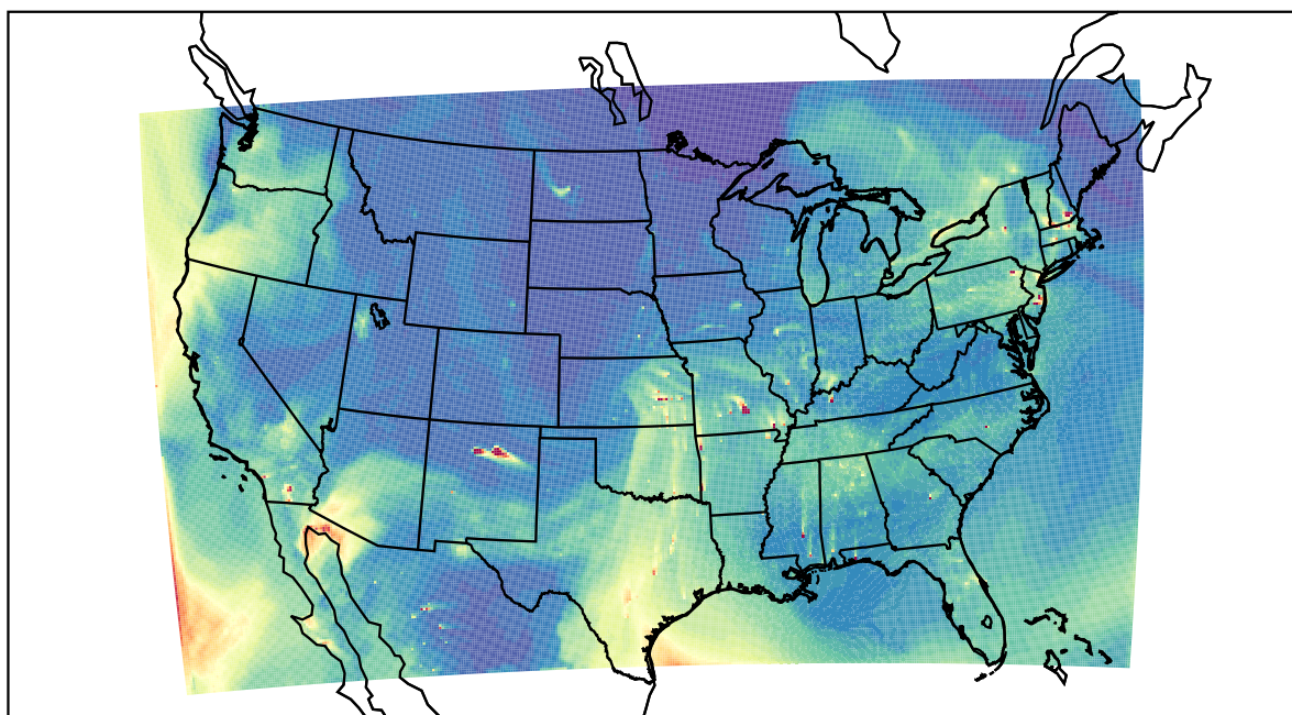
WRF 2022-05-02_23:00:00
