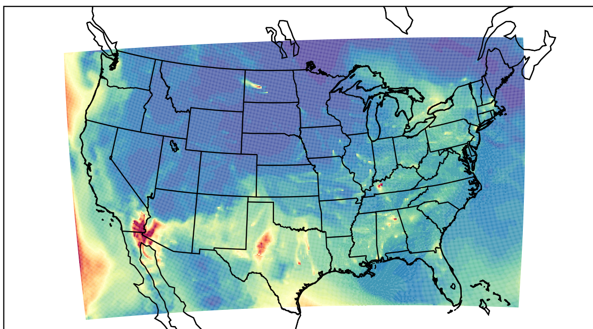
WRF 2022-05-02_13:00:00
