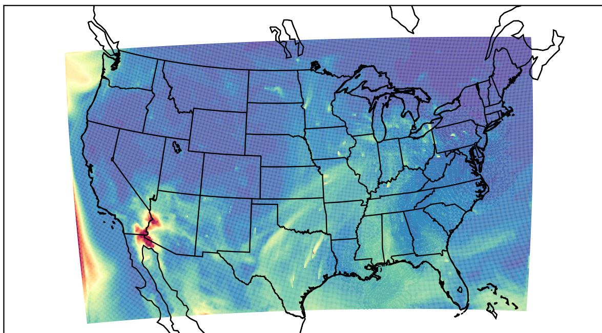
WRF 2022-05-18_16:00:00
