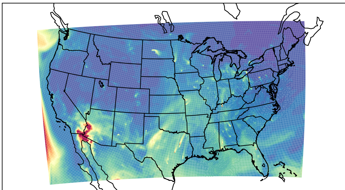
WRF 2022-05-18_14:00:00
