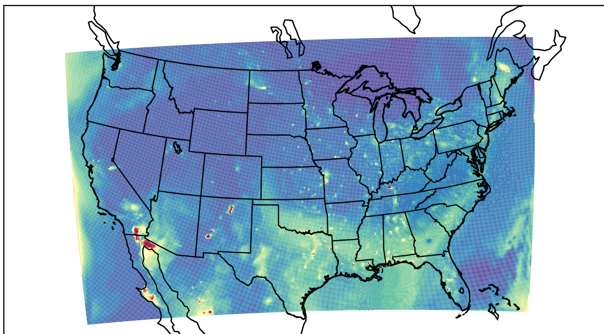
WRF 2022-05-17_01:00:00
