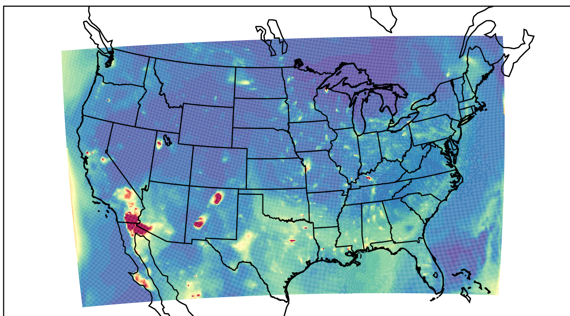
WRF 2022-05-17_03:00:00
