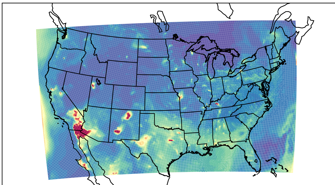
WRF 2022-05-17_04:00:00
