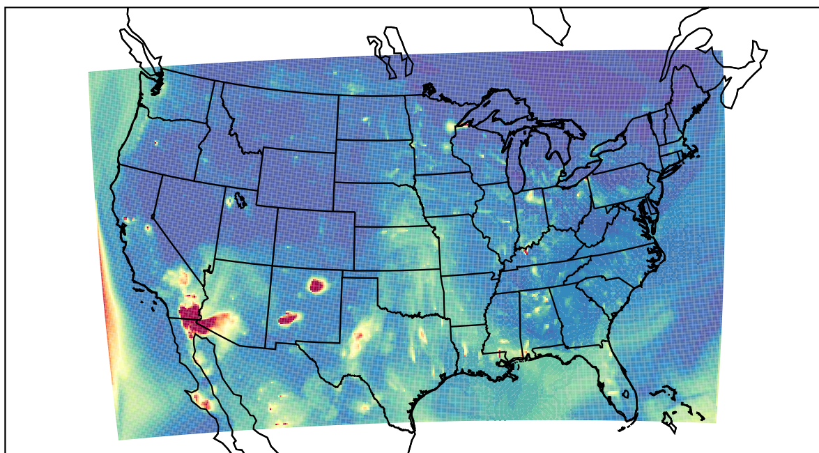
WRF 2022-05-18_03:00:00
