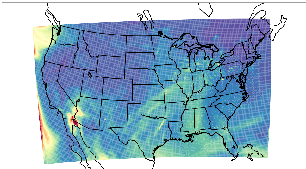
WRF 2022-05-18_18:00:00
