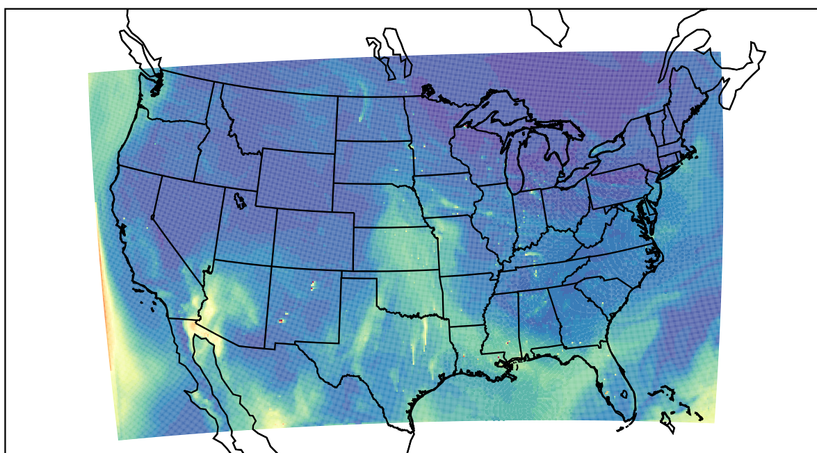
WRF 2022-05-17_20:00:00
