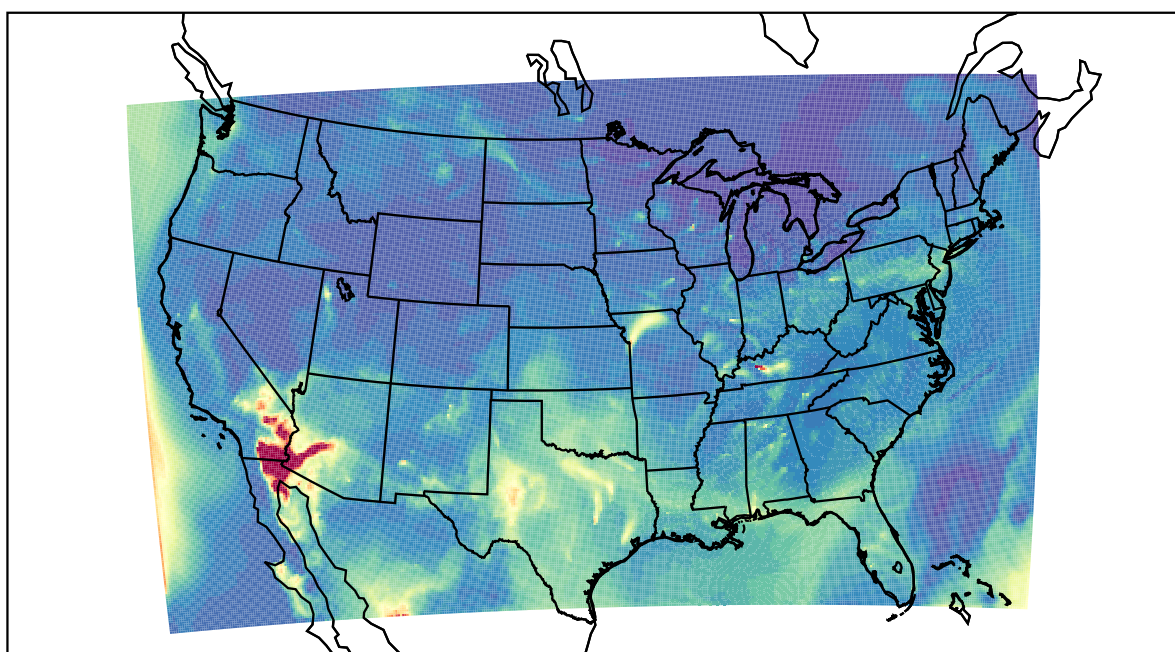
WRF 2022-05-17_10:00:00
