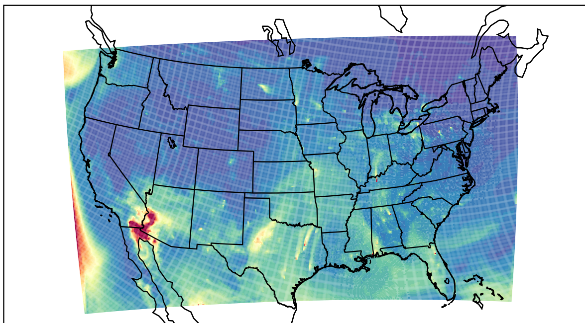
WRF 2022-05-18_13:00:00
