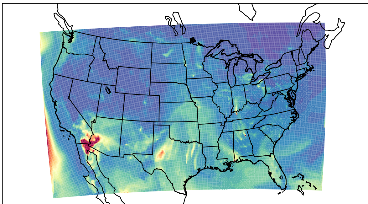
WRF 2022-05-18_10:00:00
