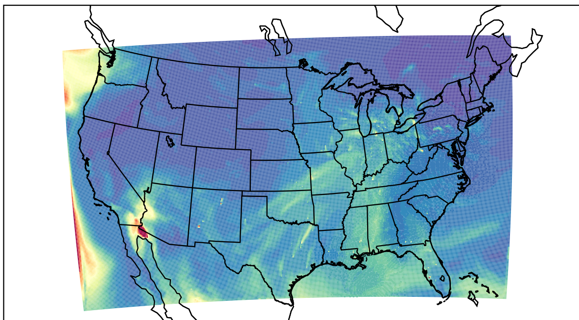
WRF 2022-05-18_19:00:00
