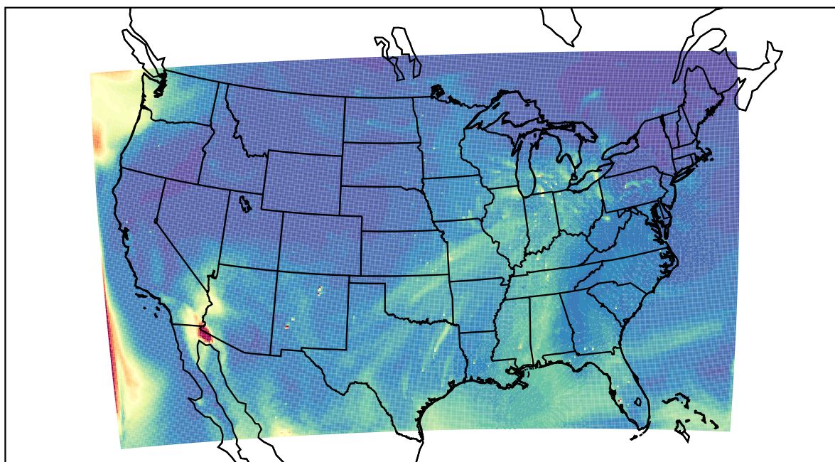
WRF 2022-05-18_20:00:00
