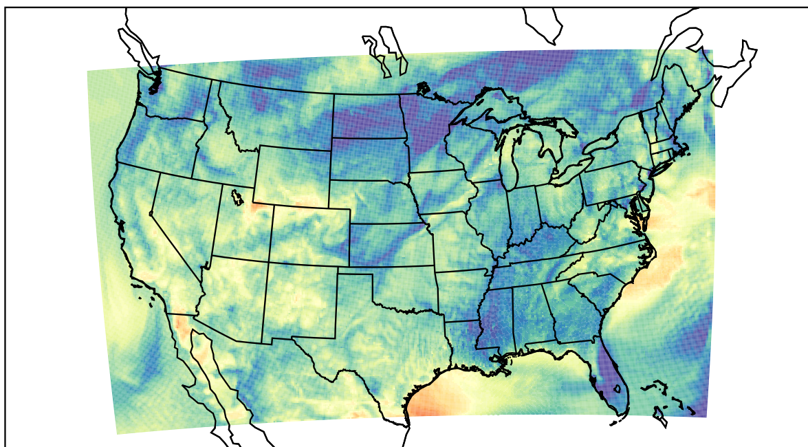
WRF (2022-05-20_10:00:00)
