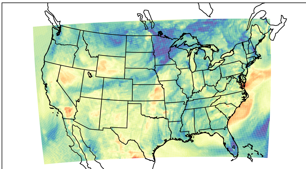
WRF (2022-05-20_03:00:00)
