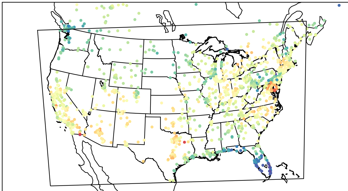
AirNOW (2022-05-20_20:00:00)
