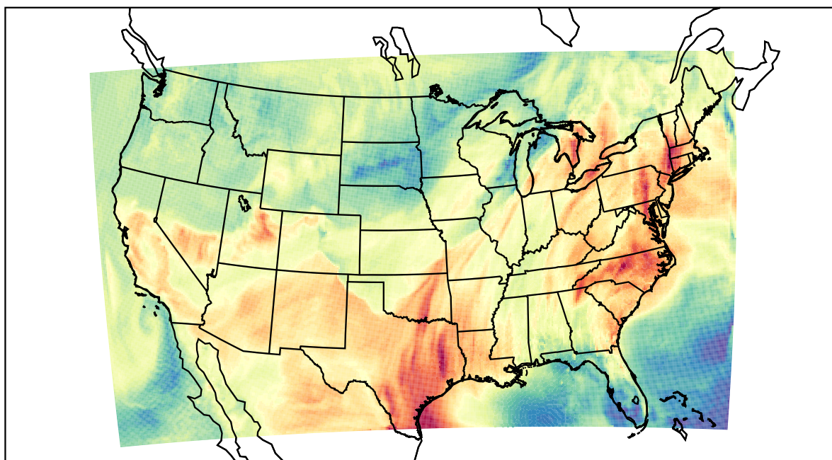
WRF (2022-05-20_20:00:00)
