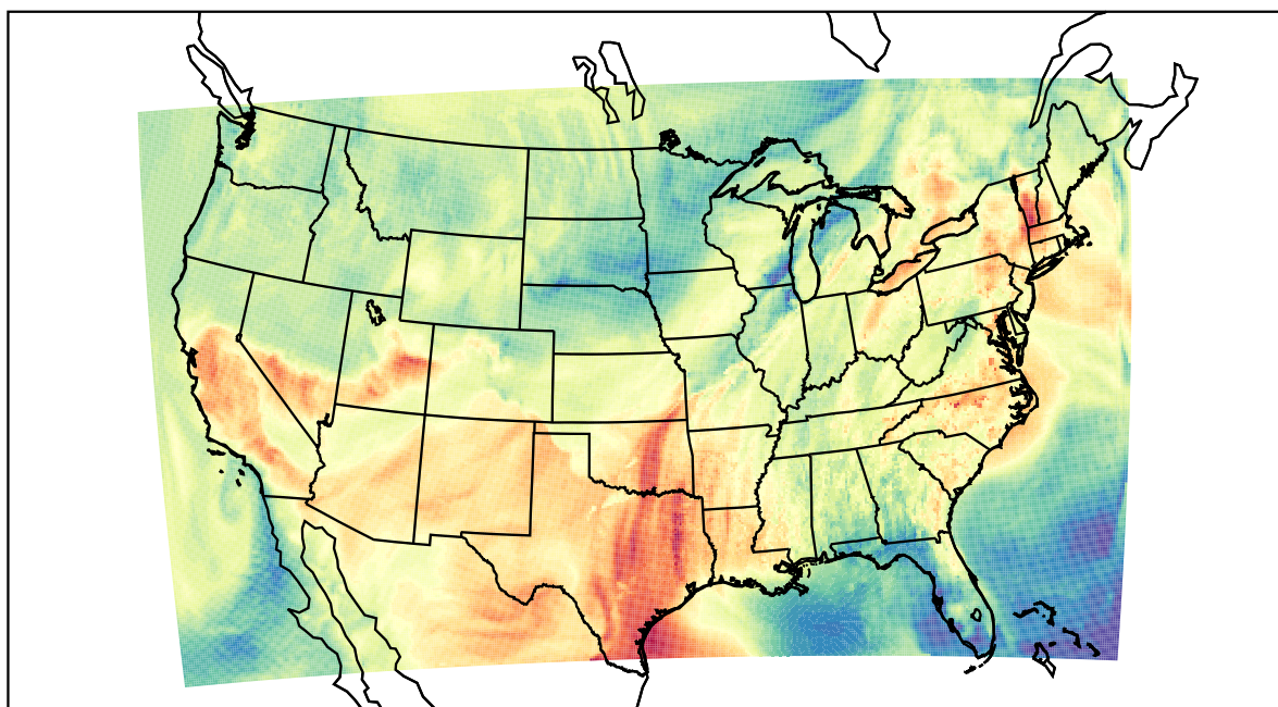
WRF (2022-05-20_23:00:00)
