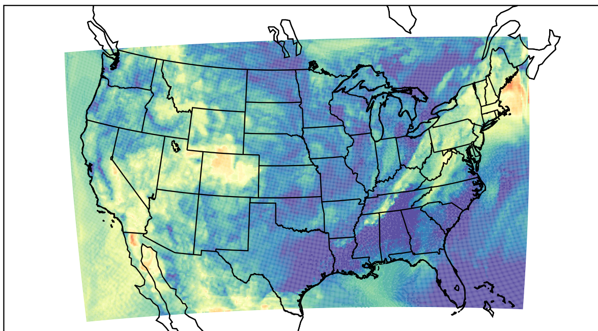
WRF (2022-05-22_13:00:00)
