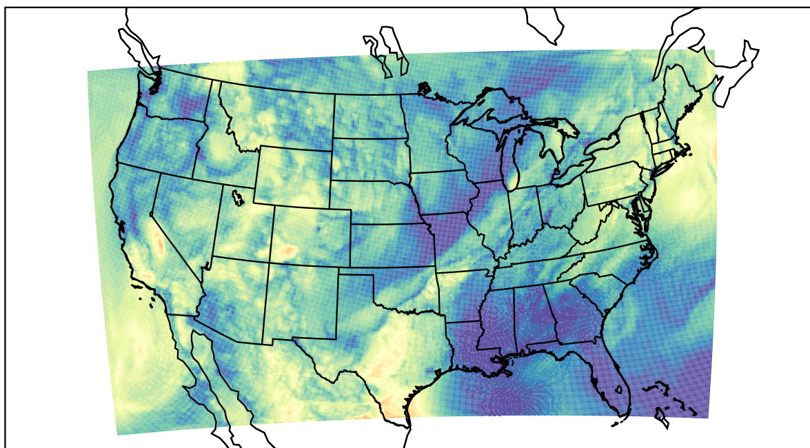
WRF (2022-05-21_13:00:00)
