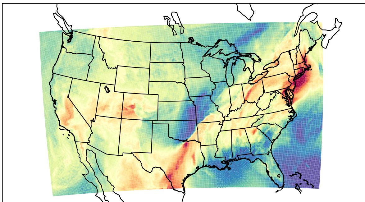
WRF (2022-05-21_19:00:00)
