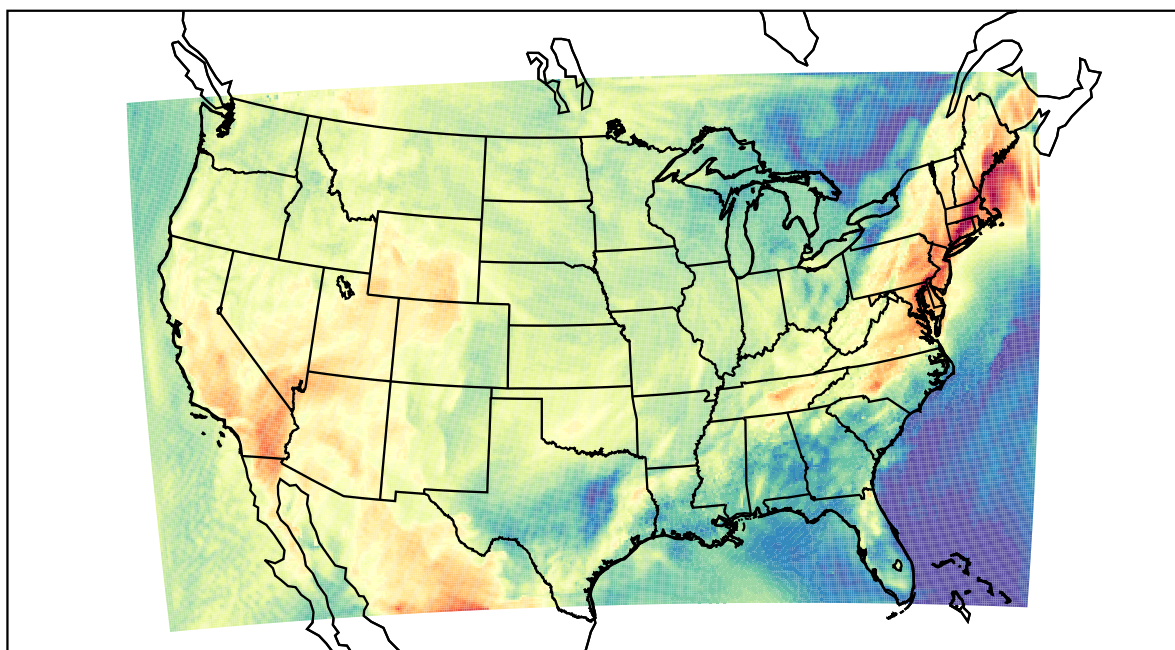
WRF (2022-05-22_20:00:00)
