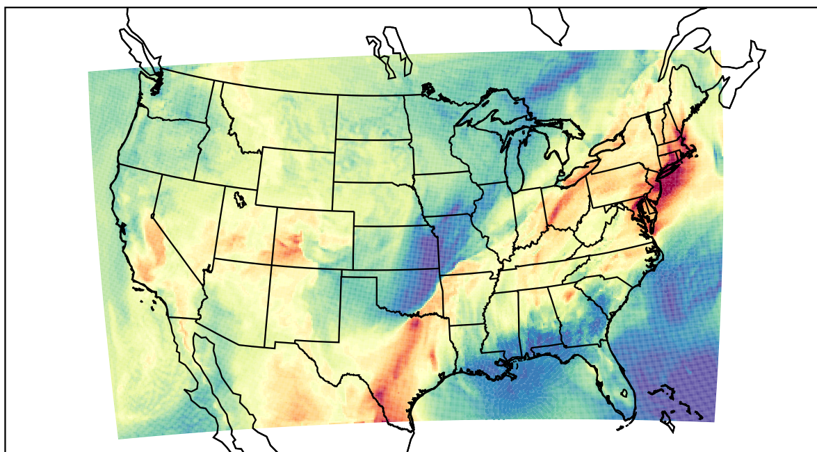
WRF (2022-05-21_18:00:00)
