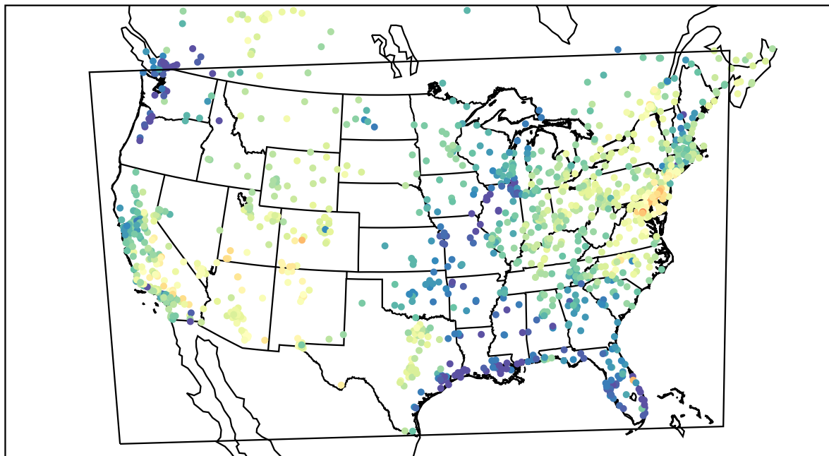
AirNOW (2022-05-21_16:00:00)
