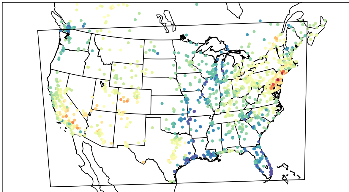
AirNOW (2022-05-21_19:00:00)
