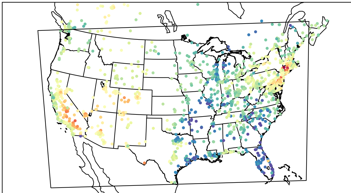
AirNOW (2022-05-21_23:00:00)
