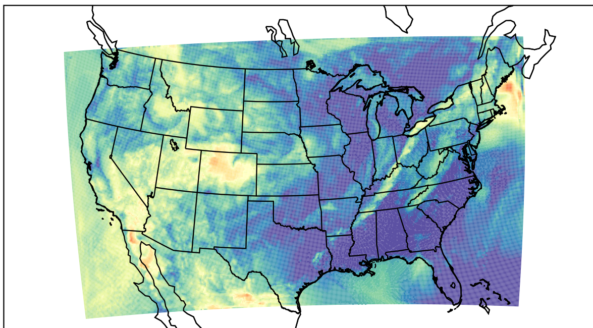
WRF (2022-05-22_10:00:00)
