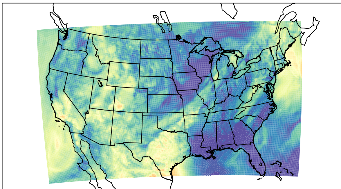
WRF (2022-05-21_10:00:00)
