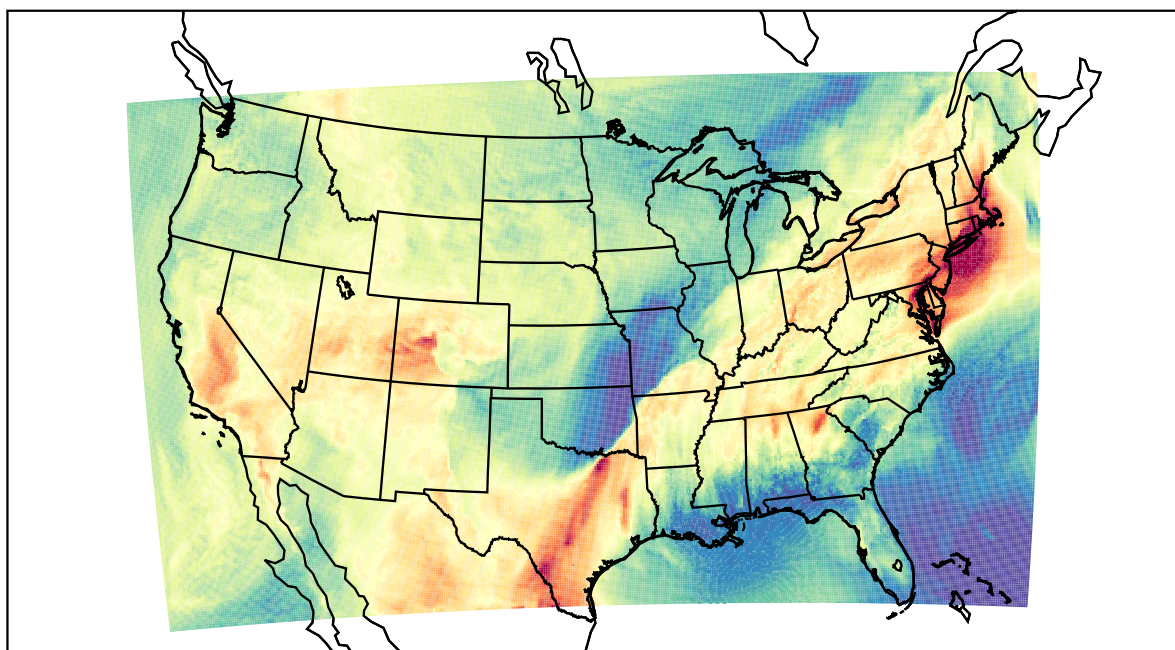
WRF (2022-05-21_20:00:00)
