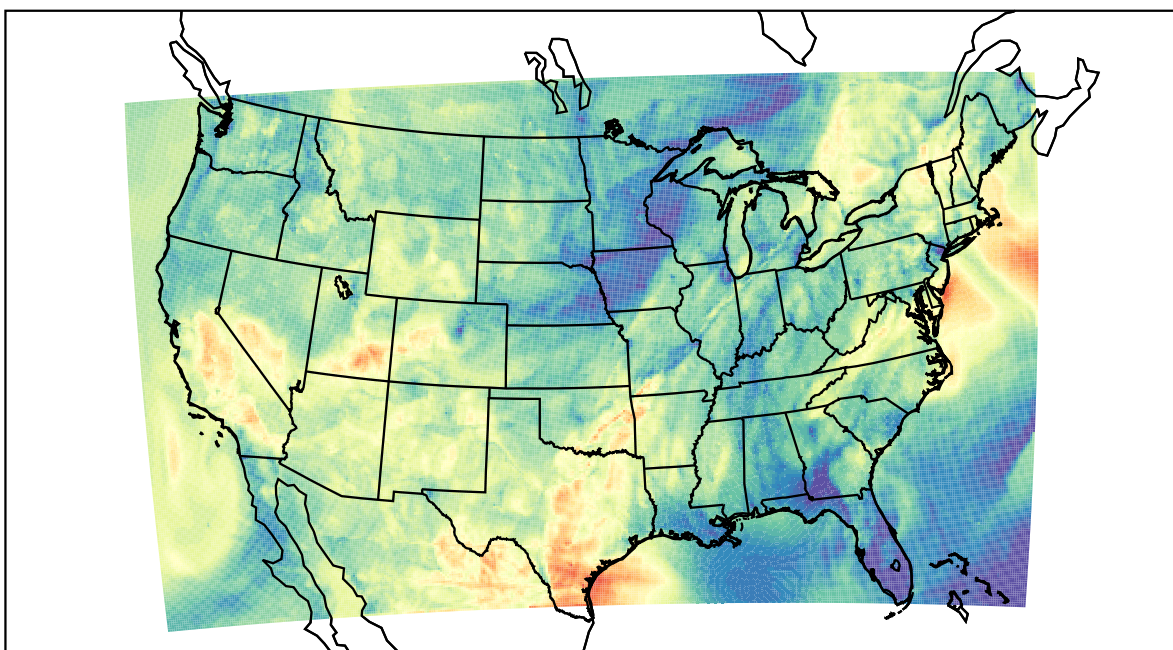
WRF (2022-05-21_03:00:00)
