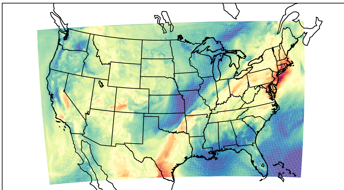
WRF (2022-05-21_16:00:00)
