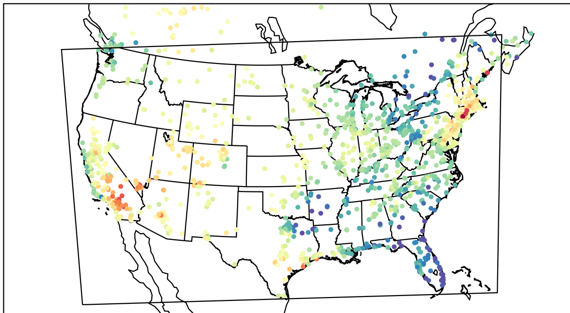
AirNOW (2022-05-22_20:00:00)
