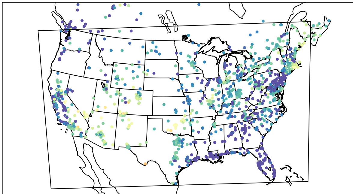
AirNOW (2022-05-21_10:00:00)
