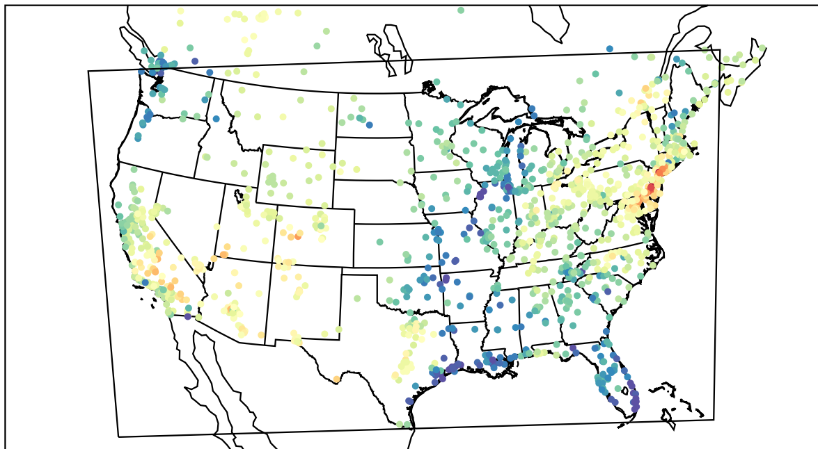
AirNOW (2022-05-21_18:00:00)
