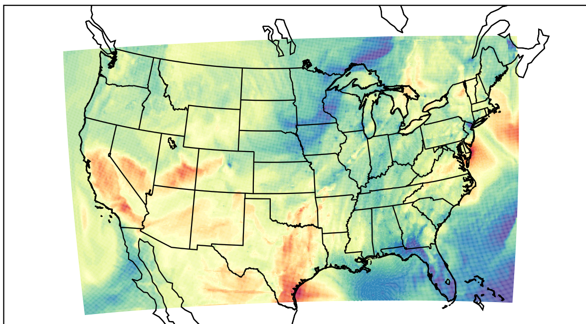
WRF (2022-05-21_01:00:00)
