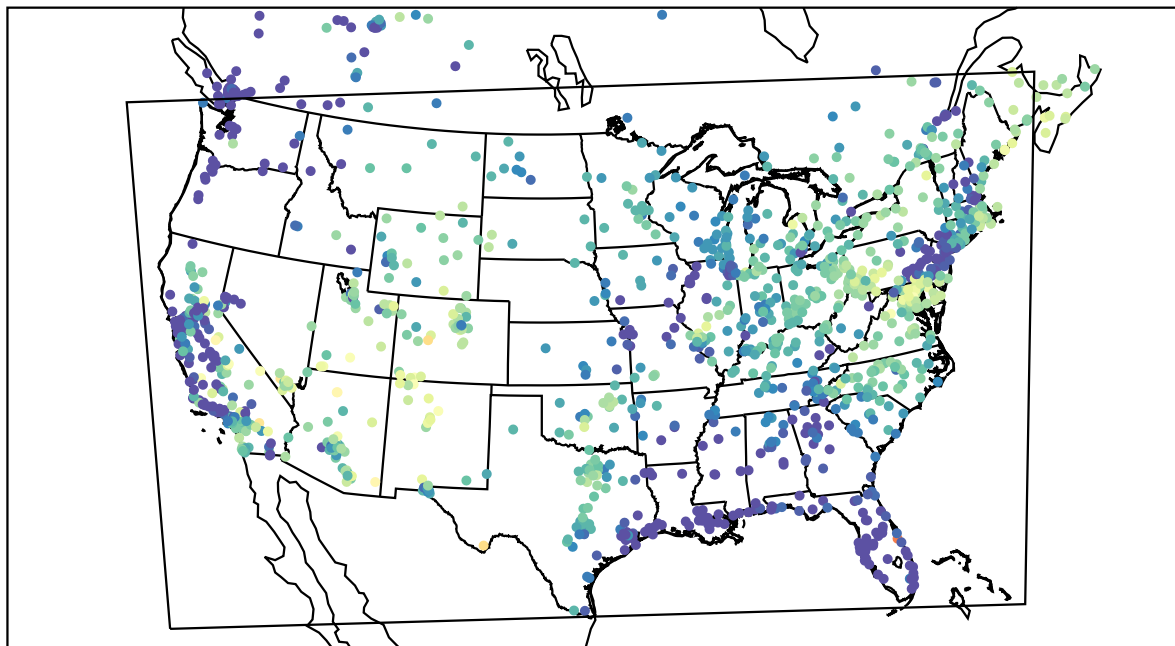
AirNOW (2022-05-21_13:00:00)
