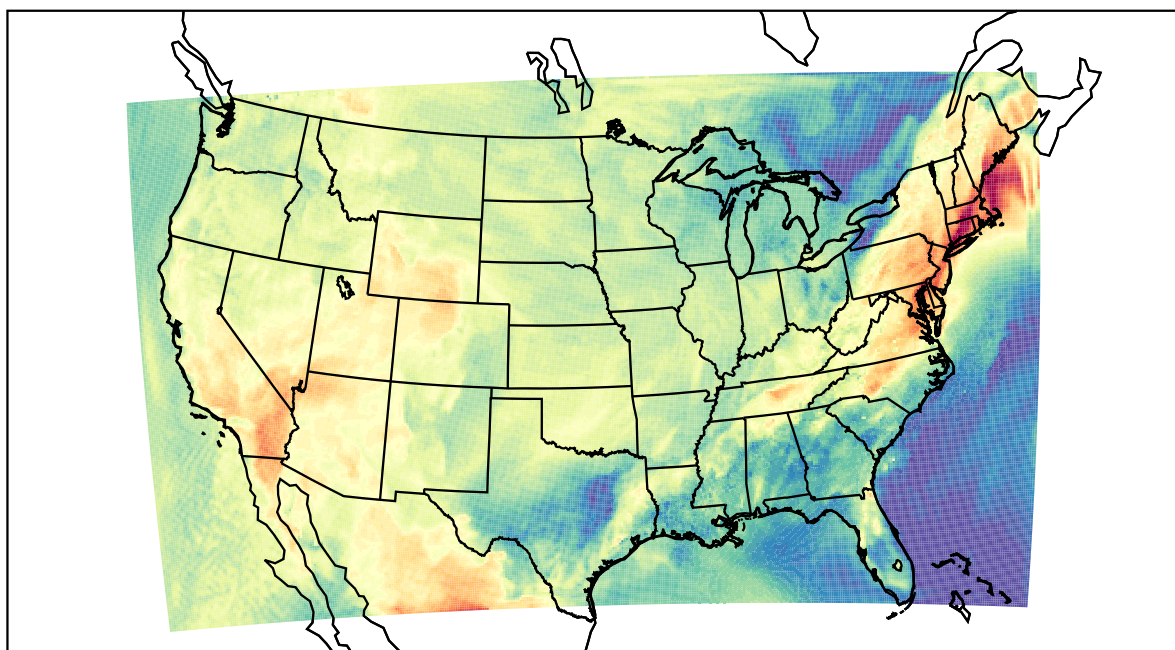
WRF (2022-05-22_19:00:00)
