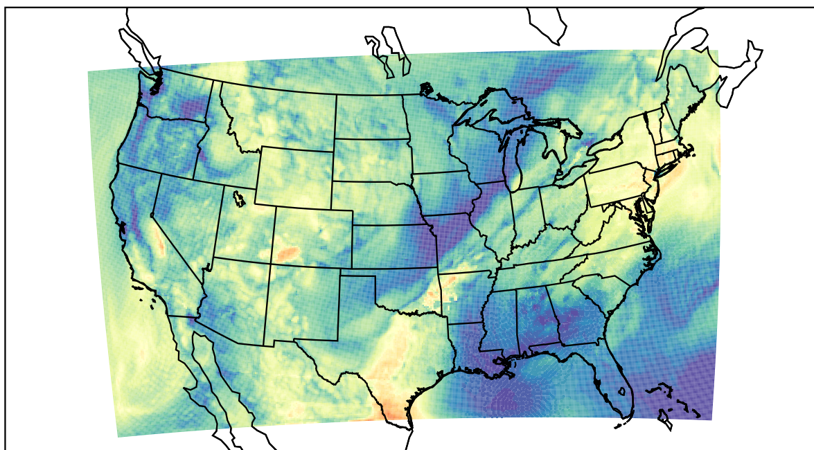
WRF (2022-05-21_14:00:00)
