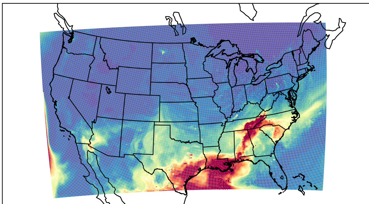
WRF 2022-05-23_18:00:00
