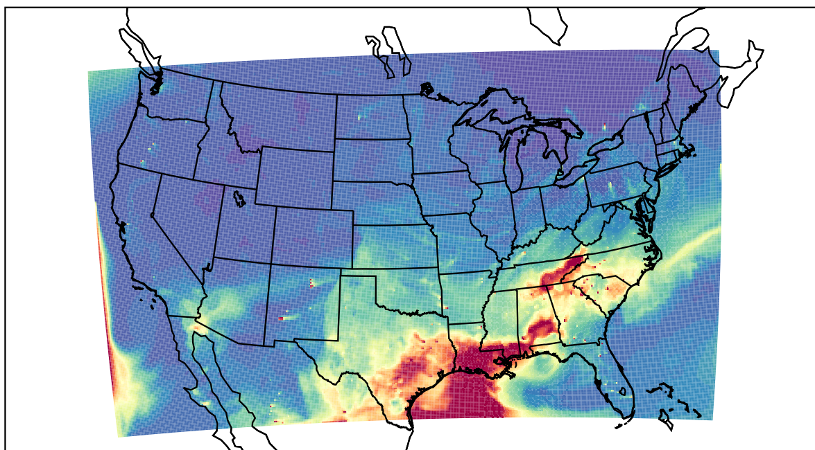
WRF 2022-05-23_23:00:00
