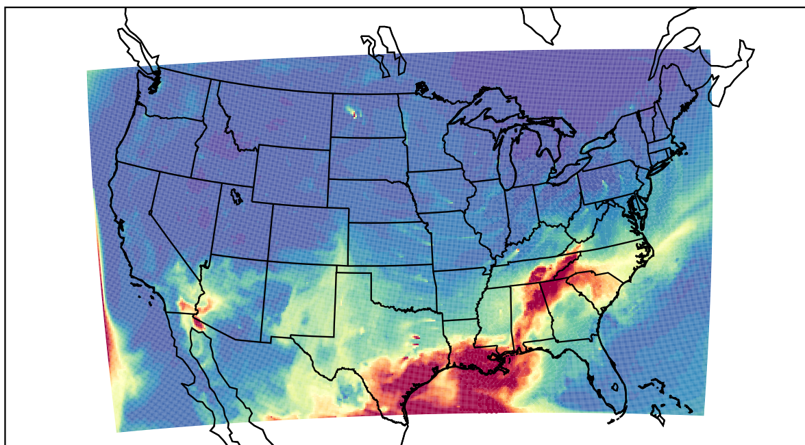
WRF 2022-05-23_16:00:00
