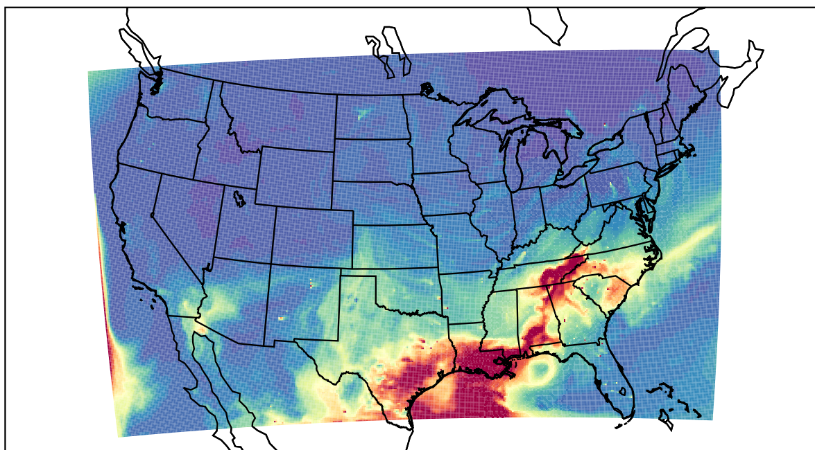
WRF 2022-05-23_20:00:00
