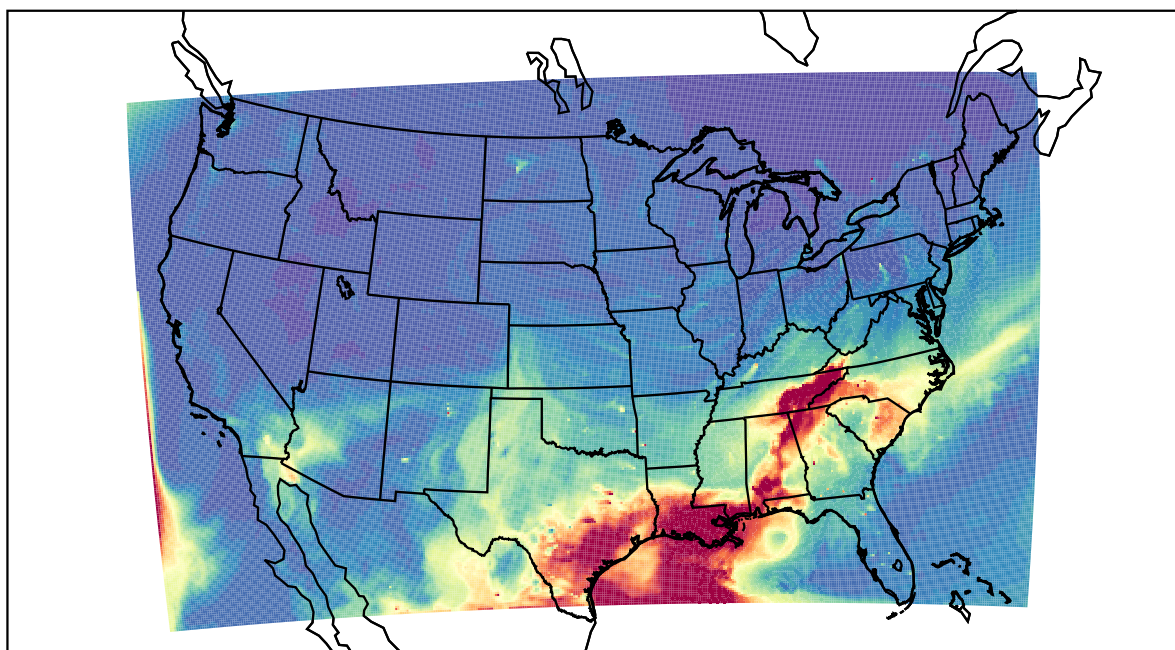
WRF 2022-05-23_19:00:00
