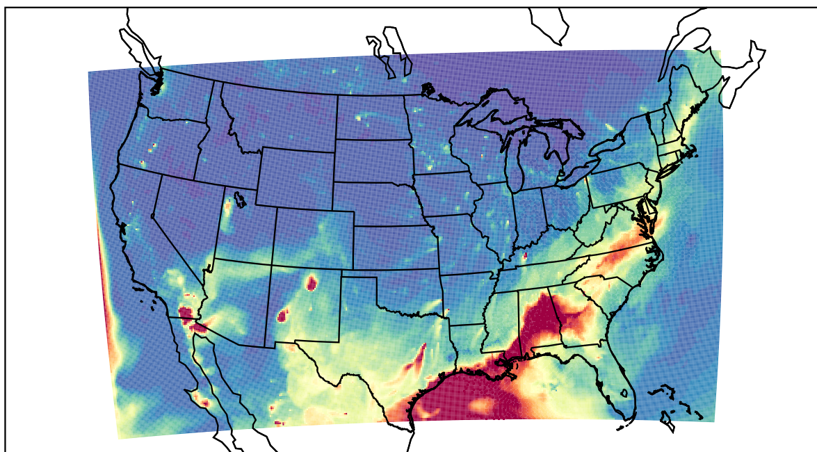
WRF 2022-05-23_03:00:00
