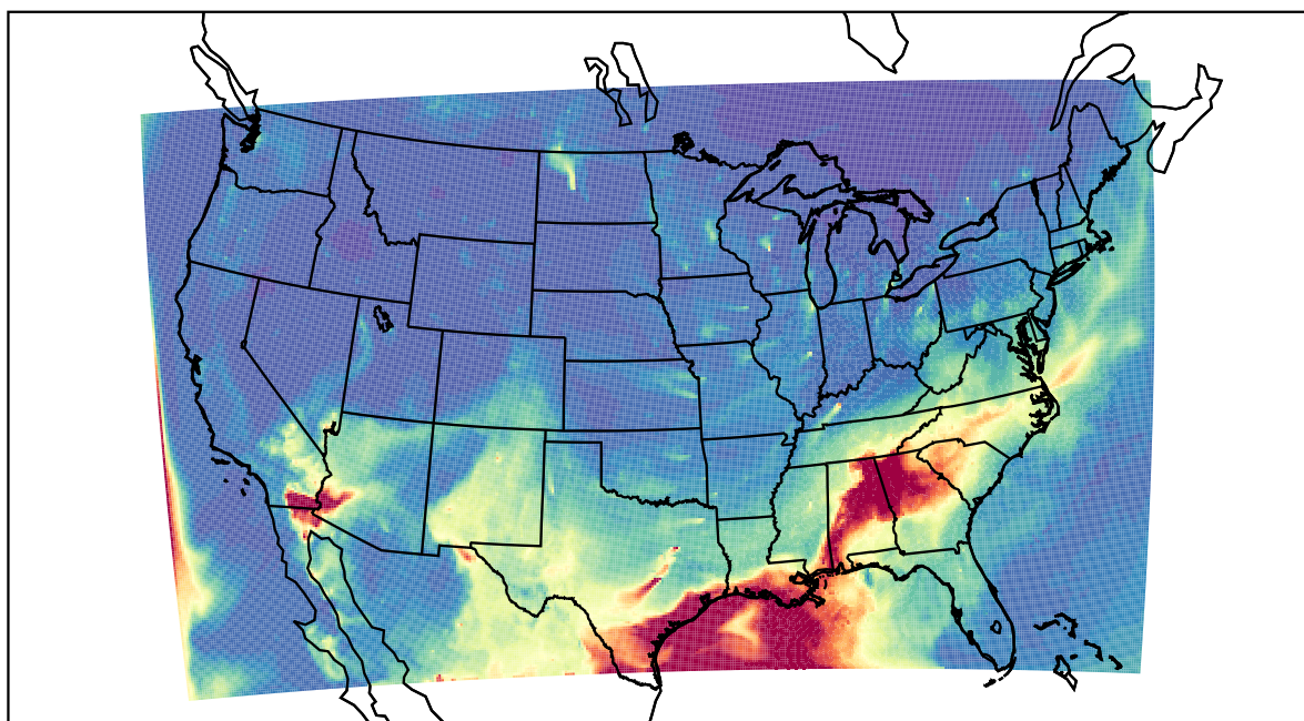
WRF 2022-05-23_10:00:00
