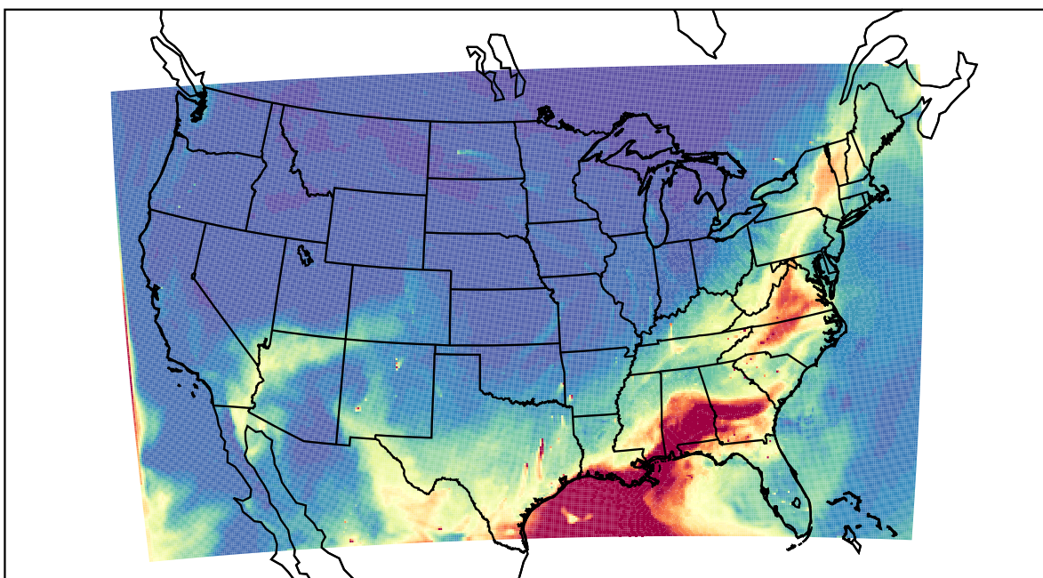
WRF 2022-05-22_20:00:00
