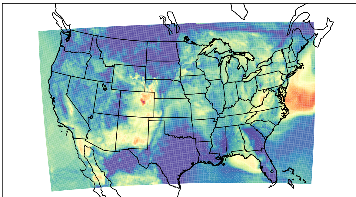
WRF (2022-05-30_10:00:00)
