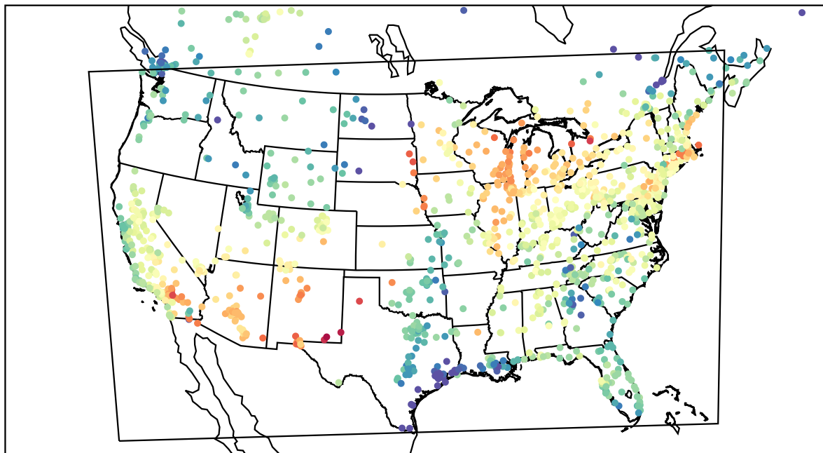
AirNOW (2022-05-30_23:00:00)
