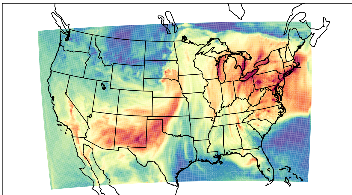
WRF (2022-05-30_20:00:00)
