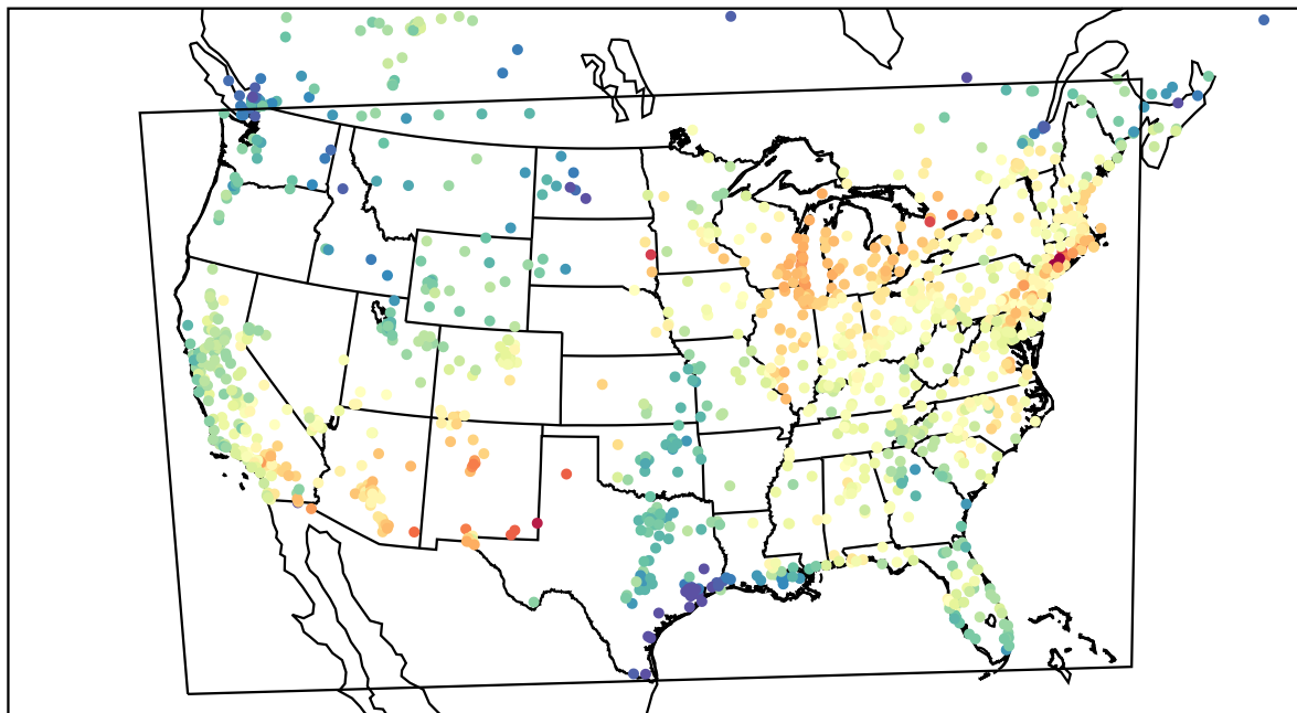
AirNOW (2022-05-30_20:00:00)
