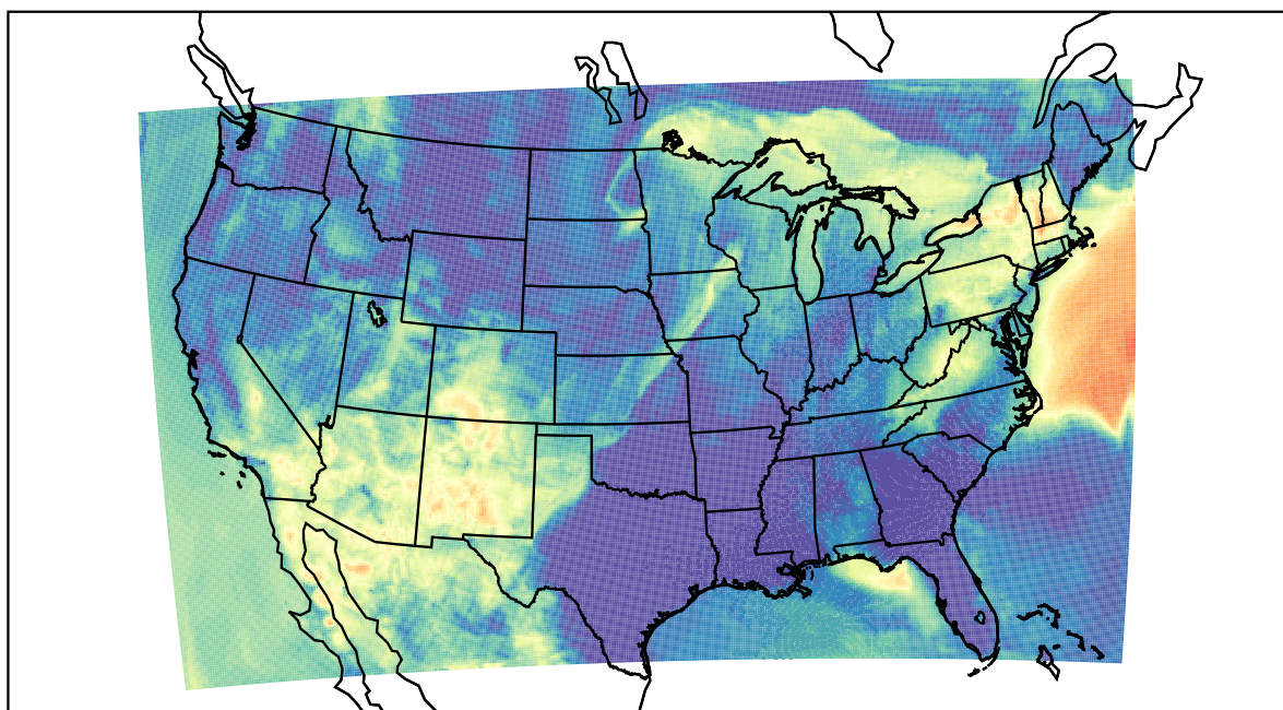
WRF (2022-05-31_10:00:00)
