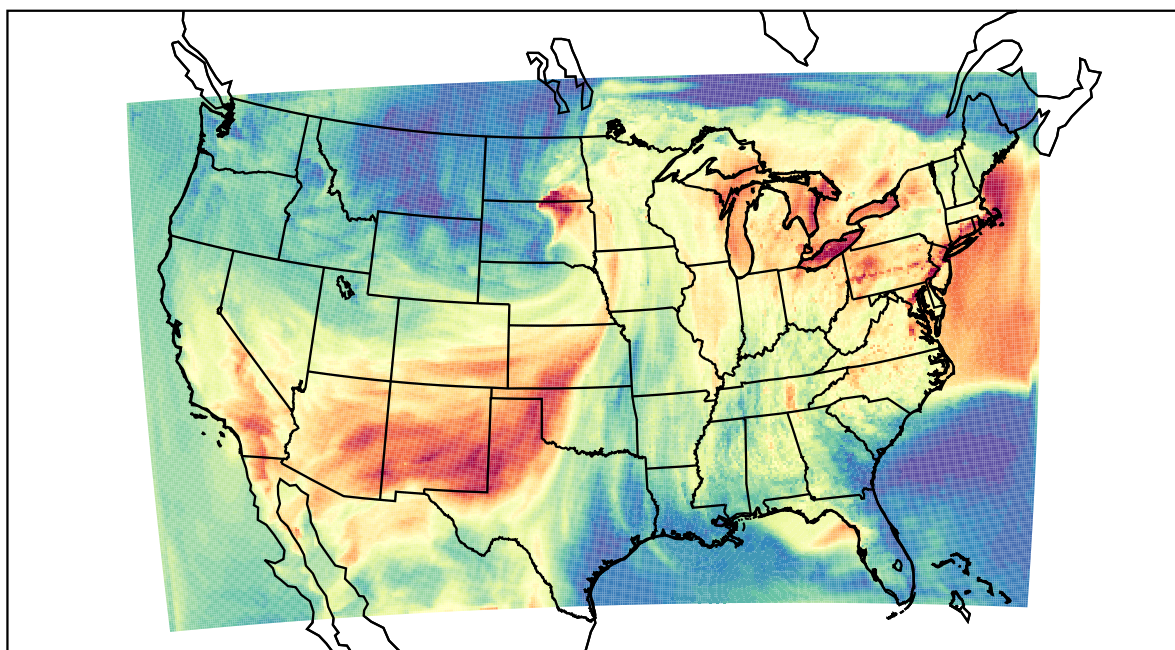
WRF (2022-05-30_23:00:00)
