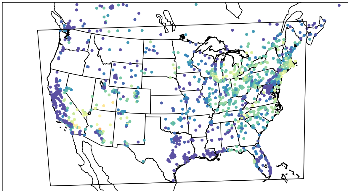
AirNOW (2022-06-12_13:00:00)
