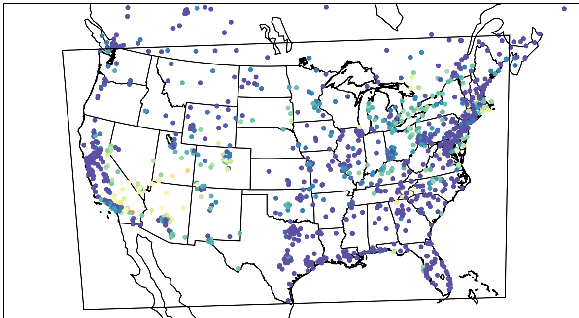
AirNOW (2022-06-12_10:00:00)
