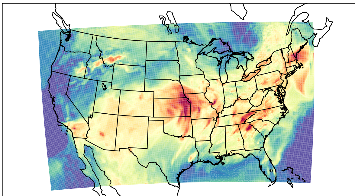
WRF (2022-06-12_20:00:00)
