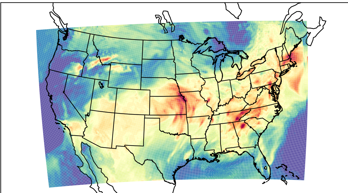
WRF (2022-06-12_18:00:00)
