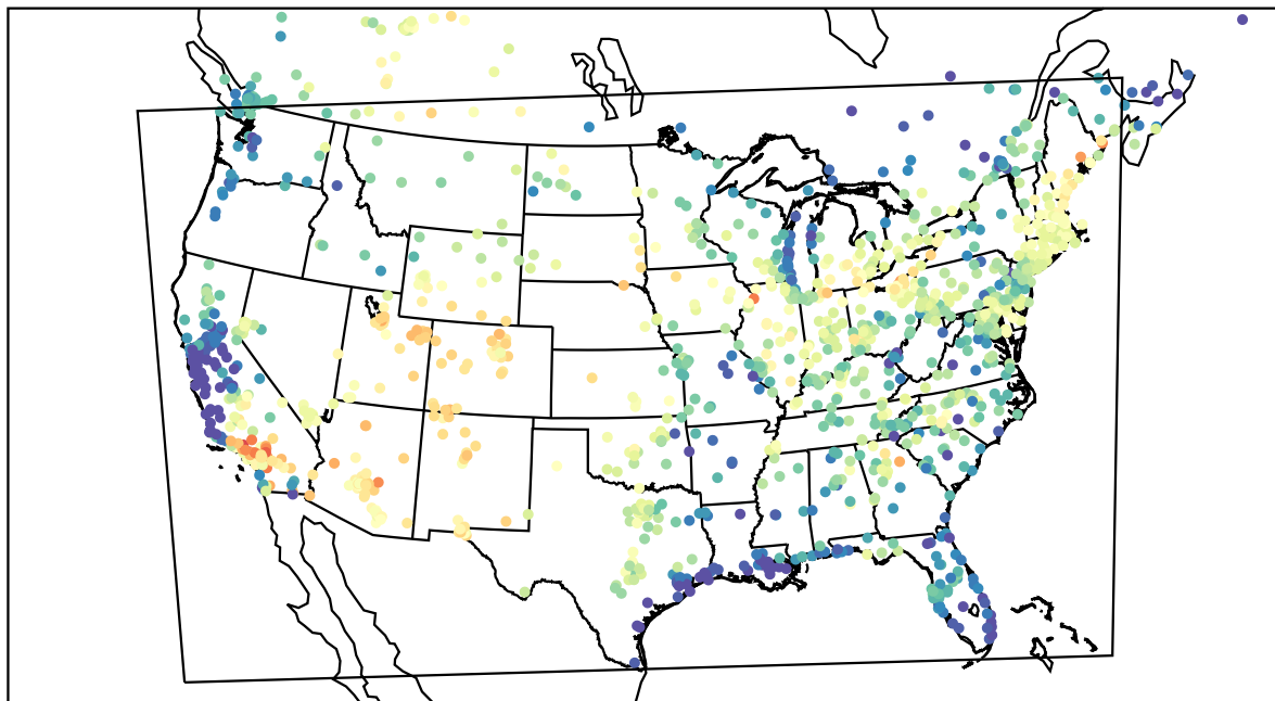
AirNOW (2022-06-12_23:00:00)
