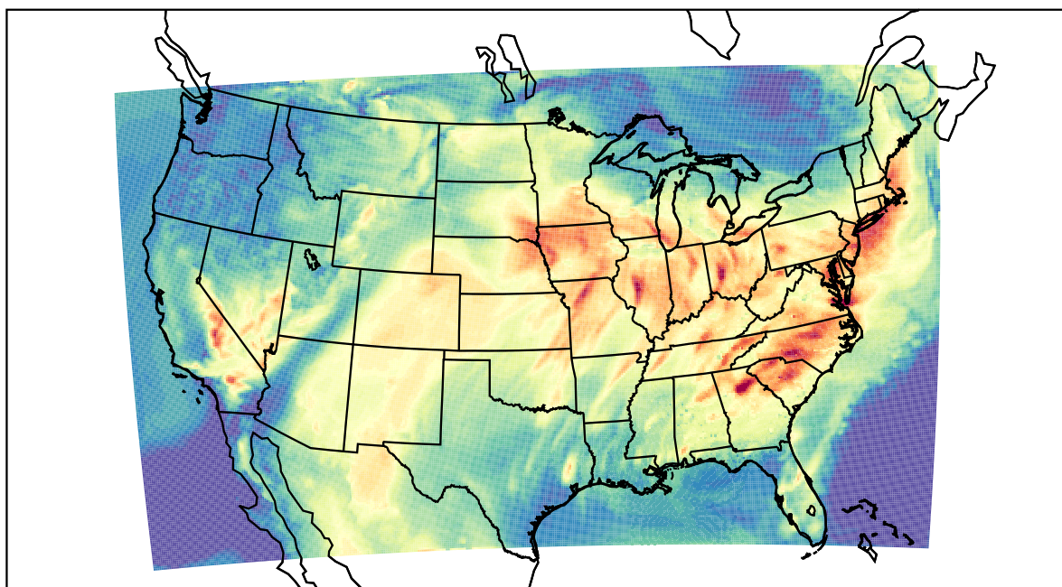
WRF (2022-06-13_18:00:00)
