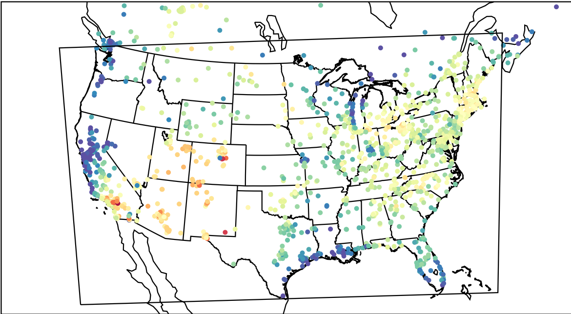
AirNOW (2022-06-12_18:00:00)
