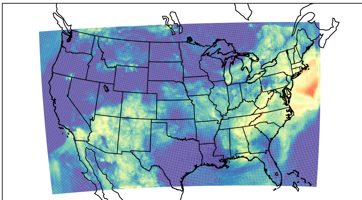
WRF (2022-06-12_13:00:00)
