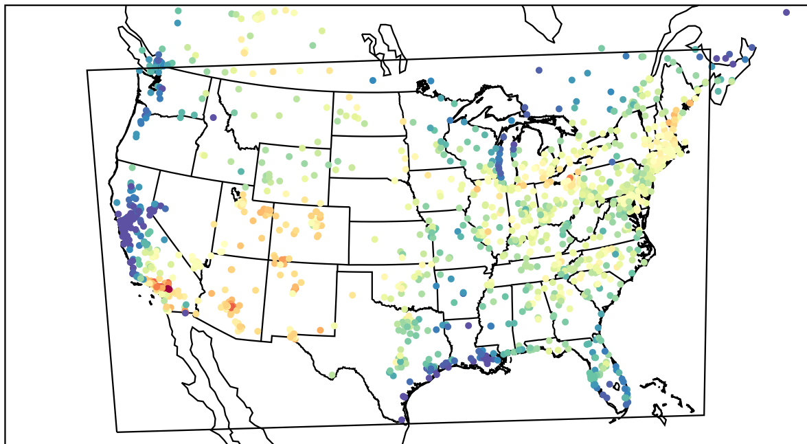
AirNOW (2022-06-12_20:00:00)
