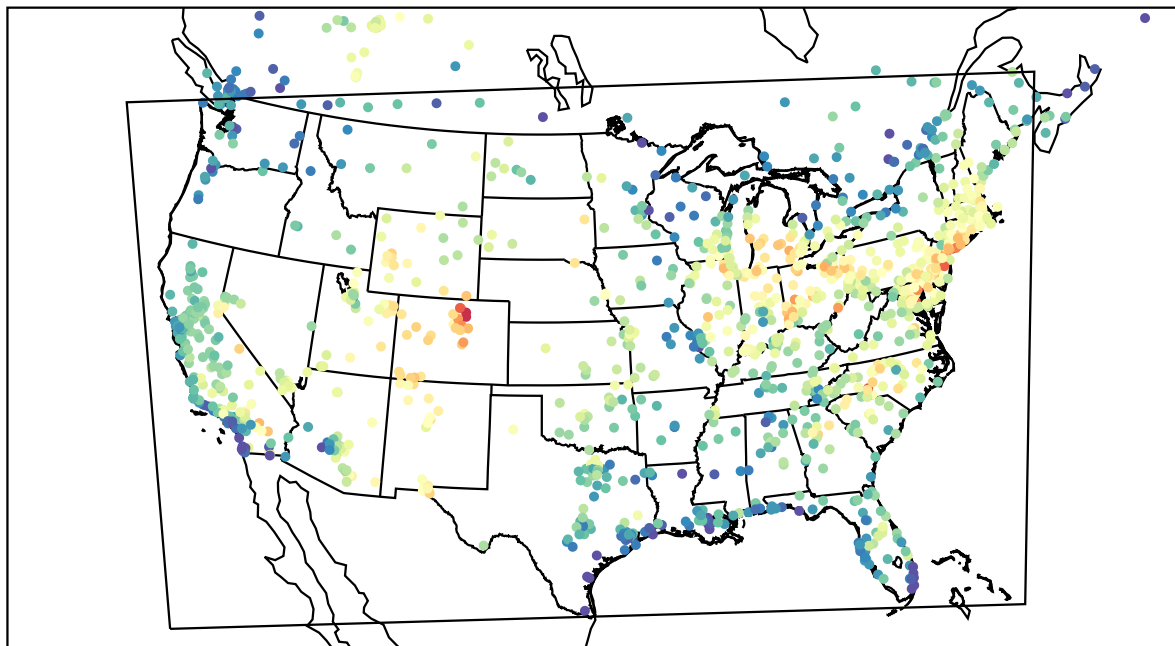
AirNOW (2022-06-13_18:00:00)
