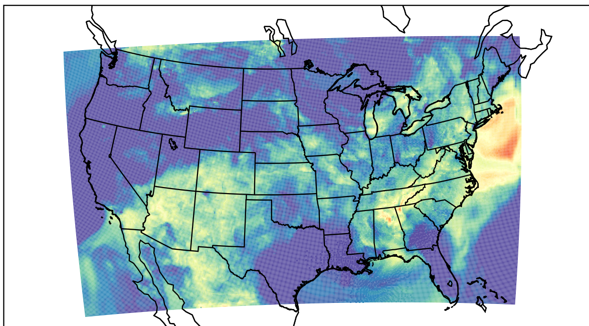
WRF (2022-06-12_10:00:00)
