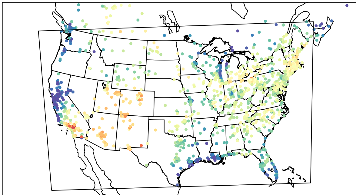
AirNOW (2022-06-12_19:00:00)
