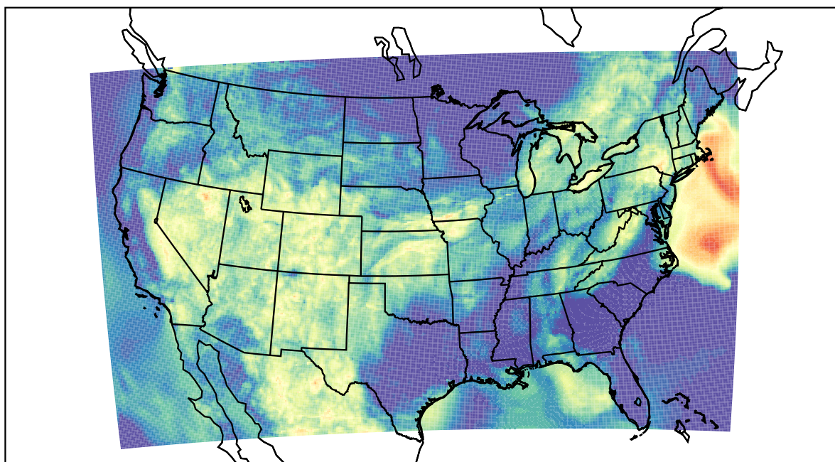
WRF (2022-07-01_10:00:00)
