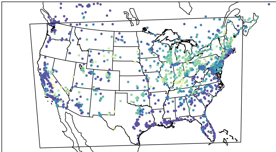
AirNOW (2022-07-02_13:00:00)
