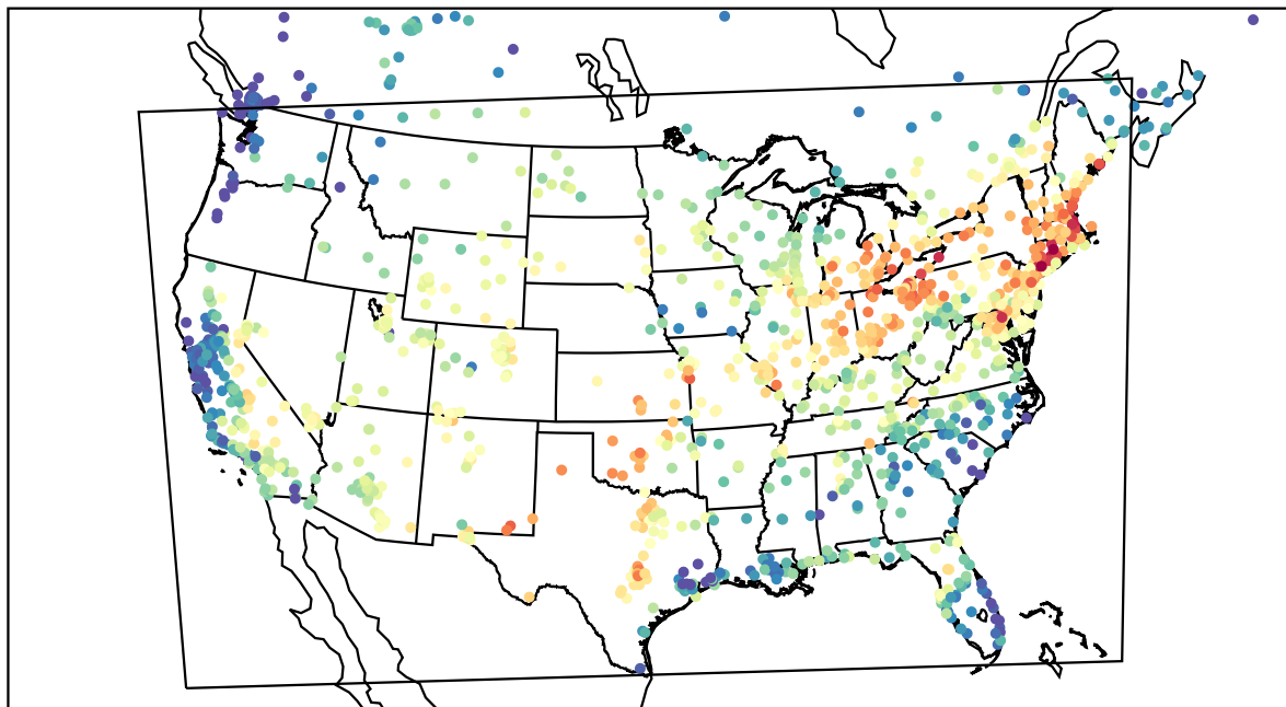
AirNOW (2022-07-01_16:00:00)
