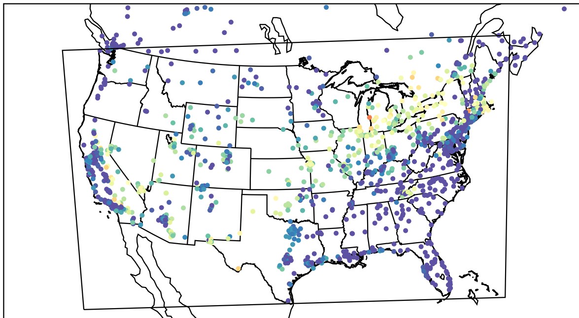
AirNOW (2022-07-01_10:00:00)
