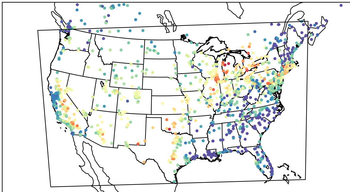
AirNOW (2022-07-01_03:00:00)
