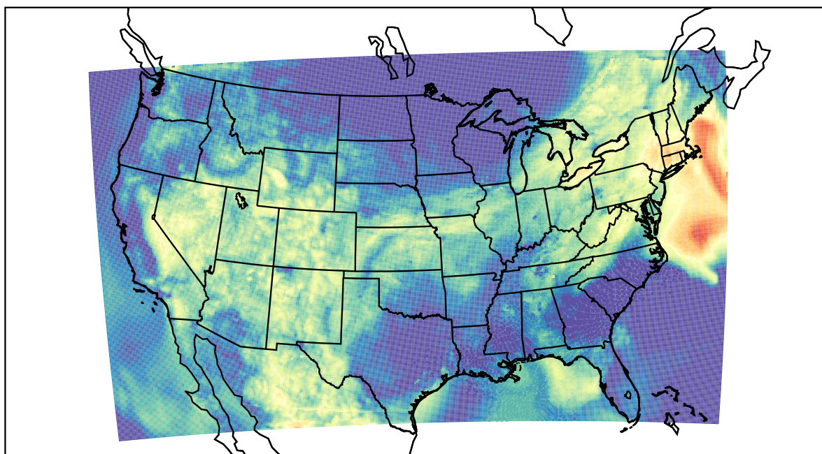
WRF (2022-07-01_13:00:00)
