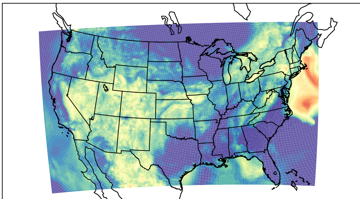
WRF (2022-07-01_11:00:00)
