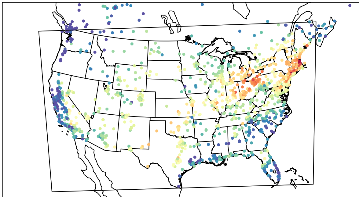
AirNOW (2022-07-01_15:00:00)
