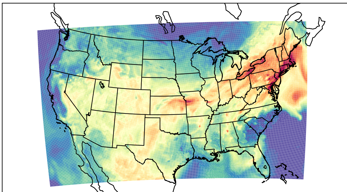
WRF (2022-07-01_16:00:00)
