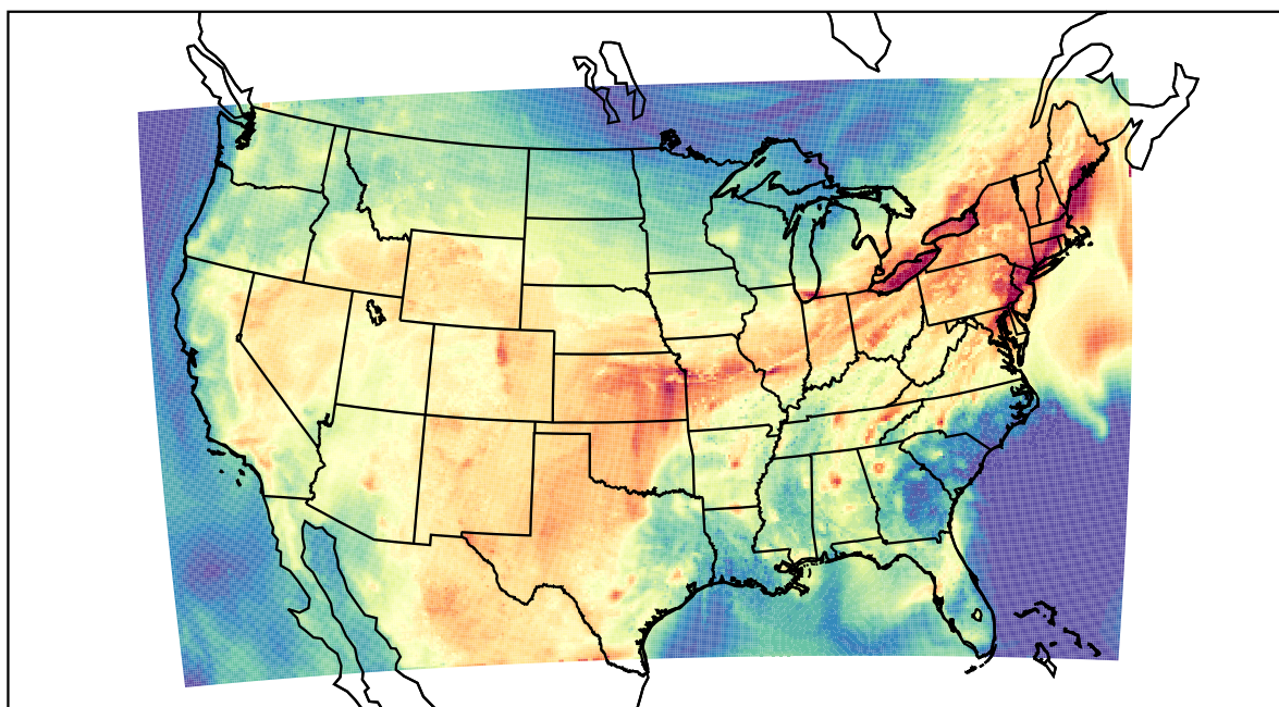
WRF (2022-07-01_20:00:00)
