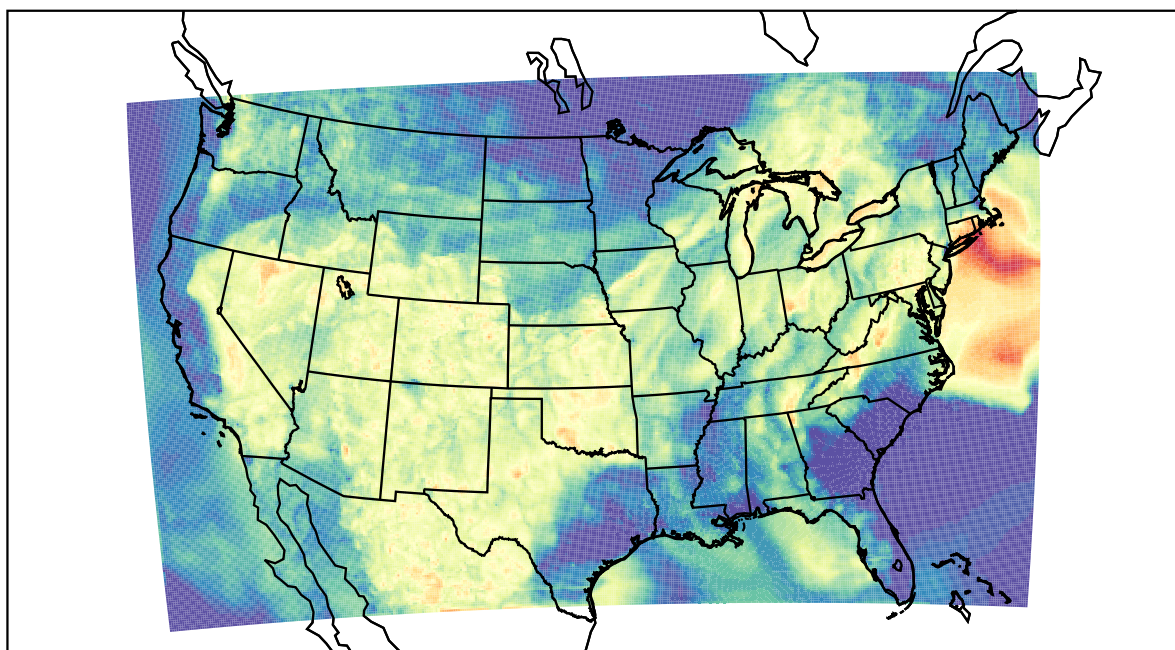
WRF (2022-07-01_04:00:00)
