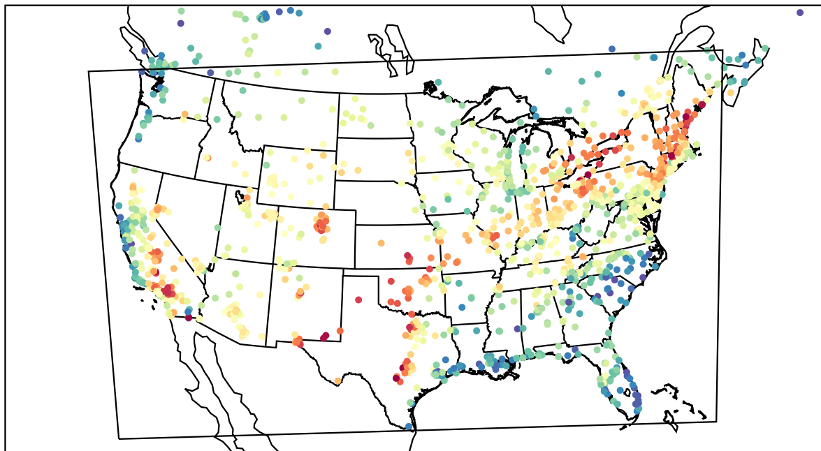
AirNOW (2022-07-01_20:00:00)
