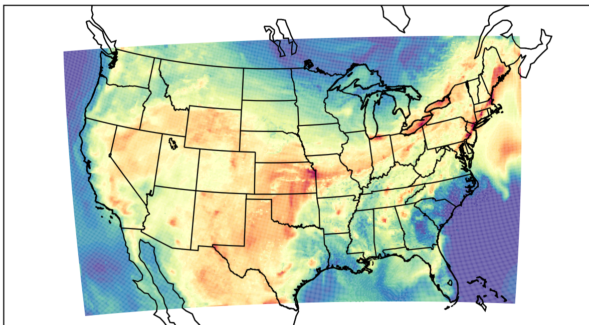
WRF (2022-07-01_23:00:00)
