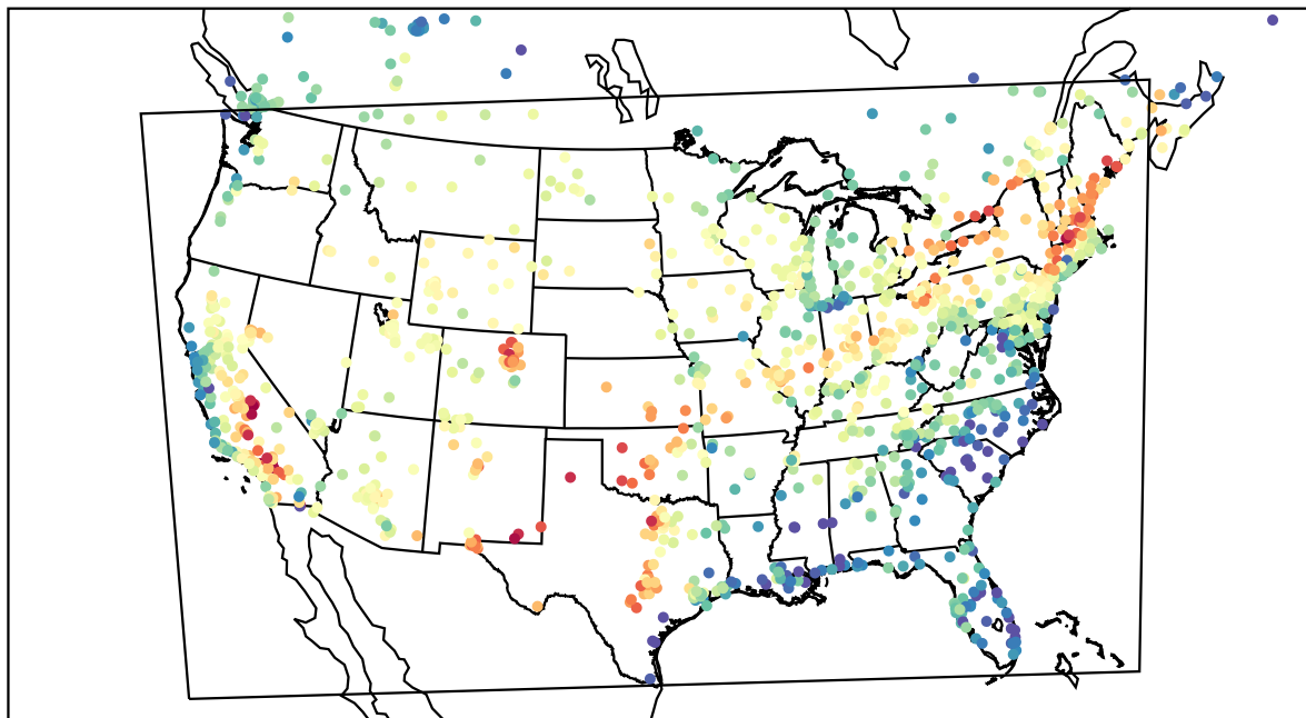
AirNOW (2022-07-01_23:00:00)
