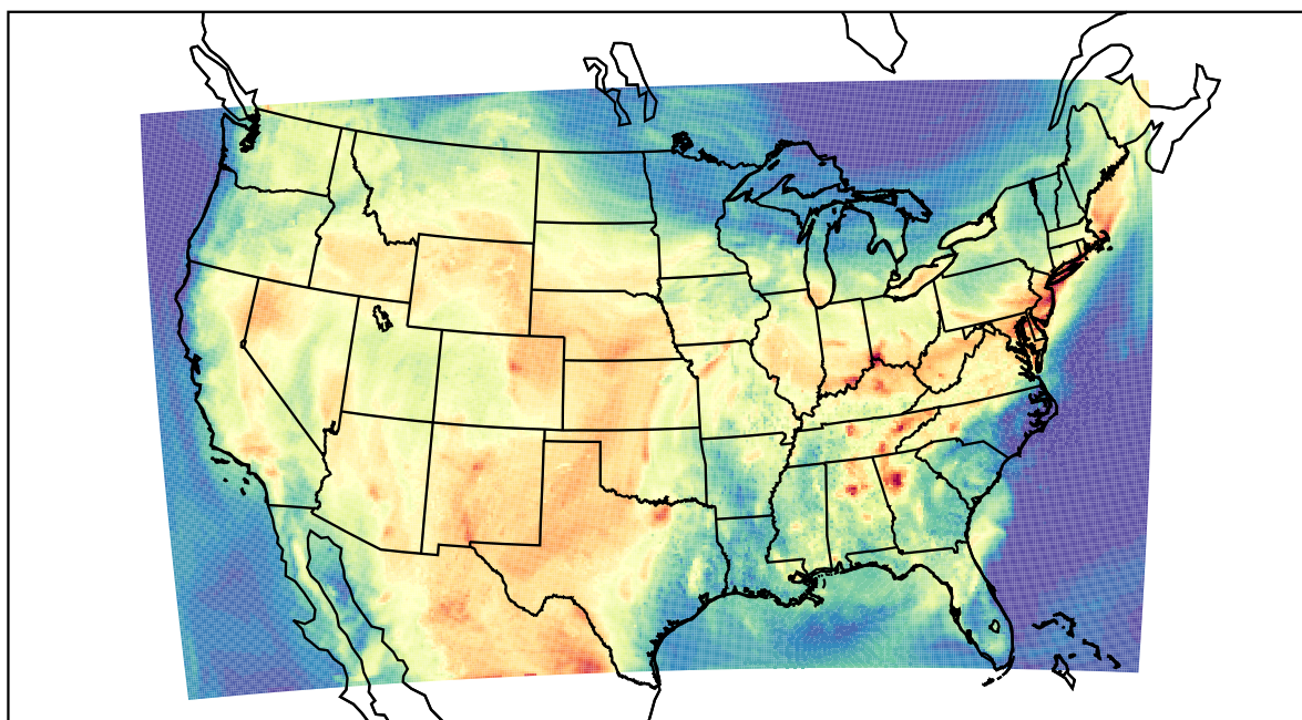
WRF (2022-07-02_20:00:00)
