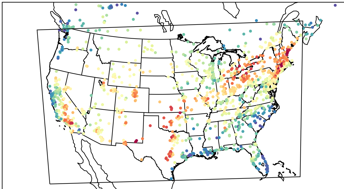
AirNOW (2022-07-01_19:00:00)
