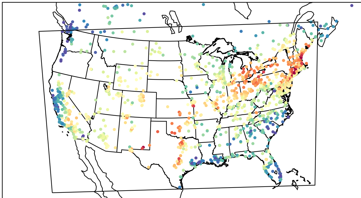
AirNOW (2022-07-01_17:00:00)
