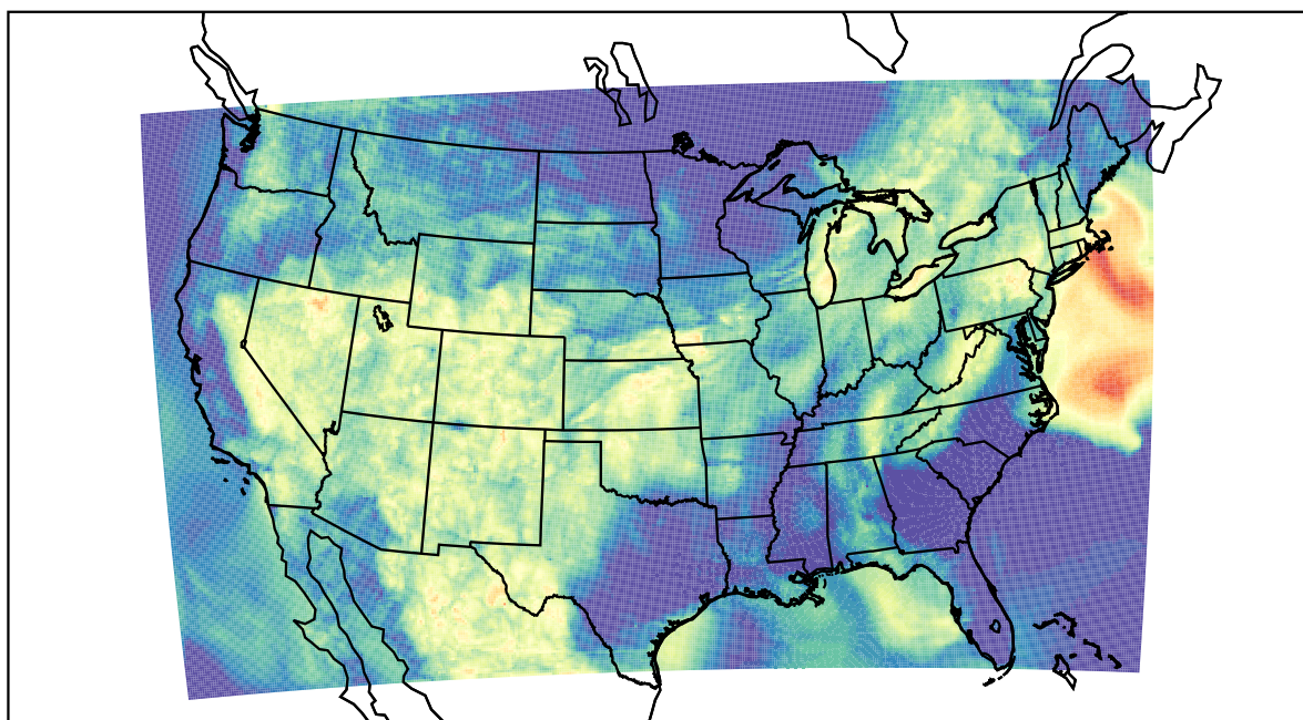
WRF (2022-07-01_08:00:00)
