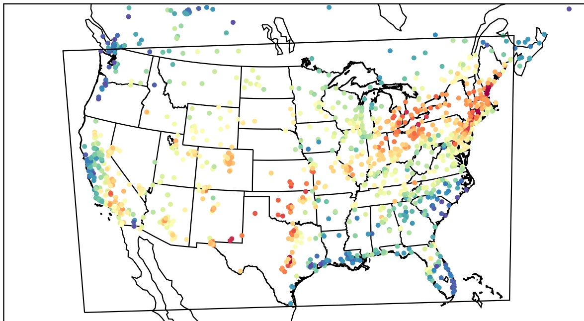
AirNOW (2022-07-01_18:00:00)
