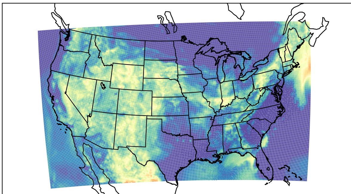
WRF (2022-07-02_10:00:00)
