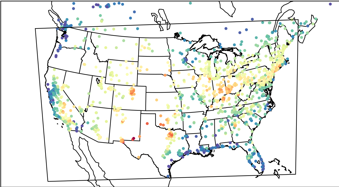
AirNOW (2022-07-02_18:00:00)
