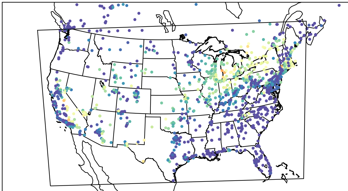
AirNOW (2022-07-01_11:00:00)
