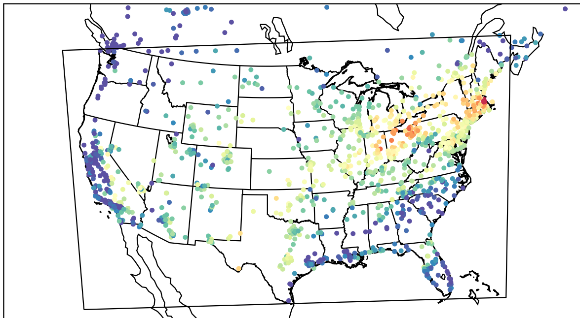
AirNOW (2022-07-01_14:00:00)
