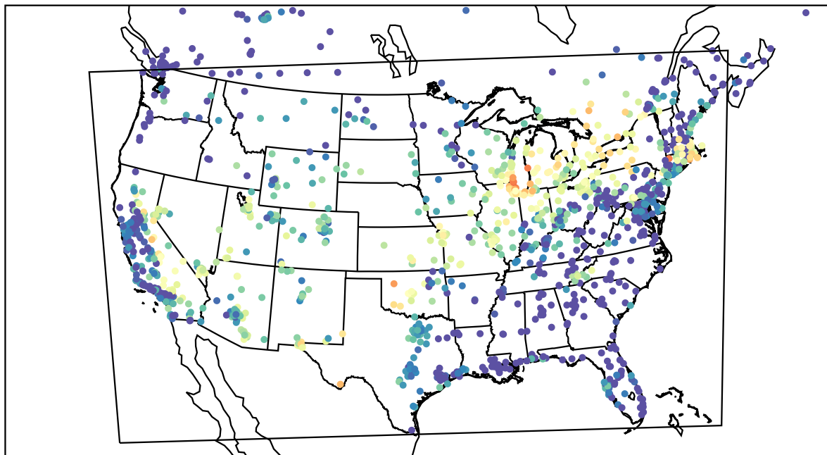
AirNOW (2022-07-01_08:00:00)
