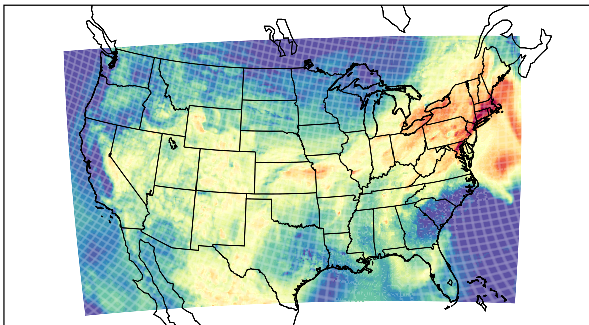
WRF (2022-07-01_15:00:00)
