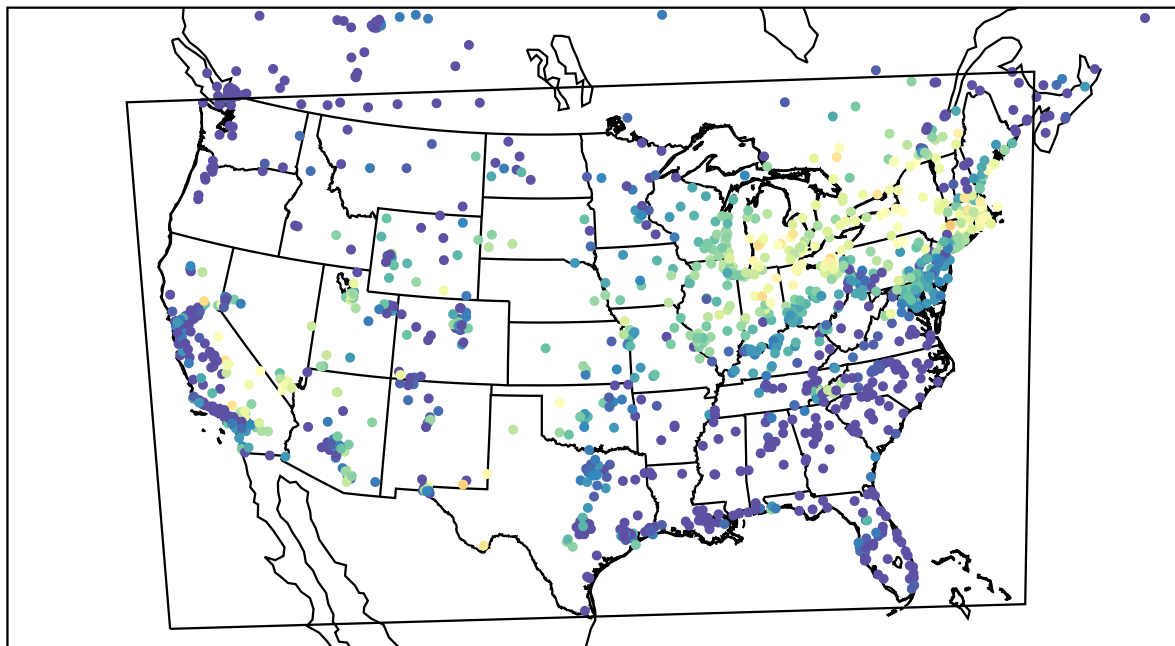
AirNOW (2022-07-01_12:00:00)
