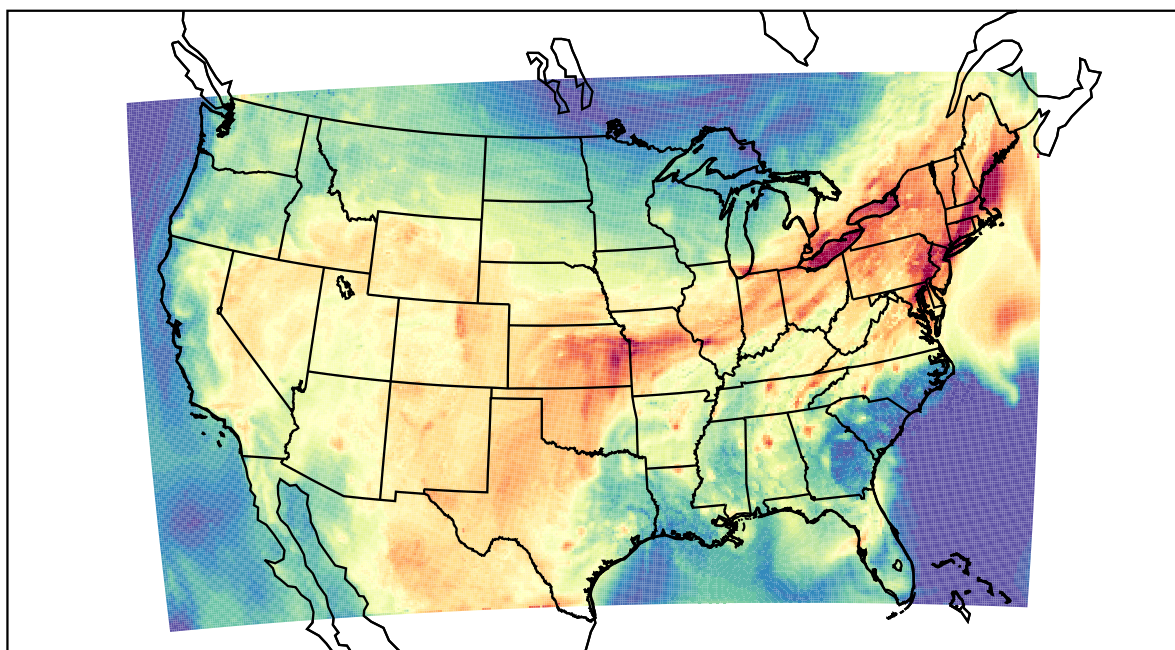
WRF (2022-07-01_19:00:00)
