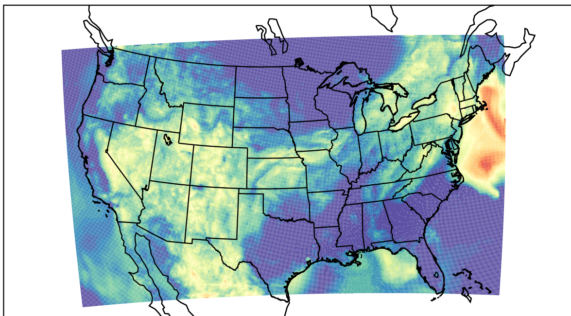
WRF (2022-07-01_12:00:00)
