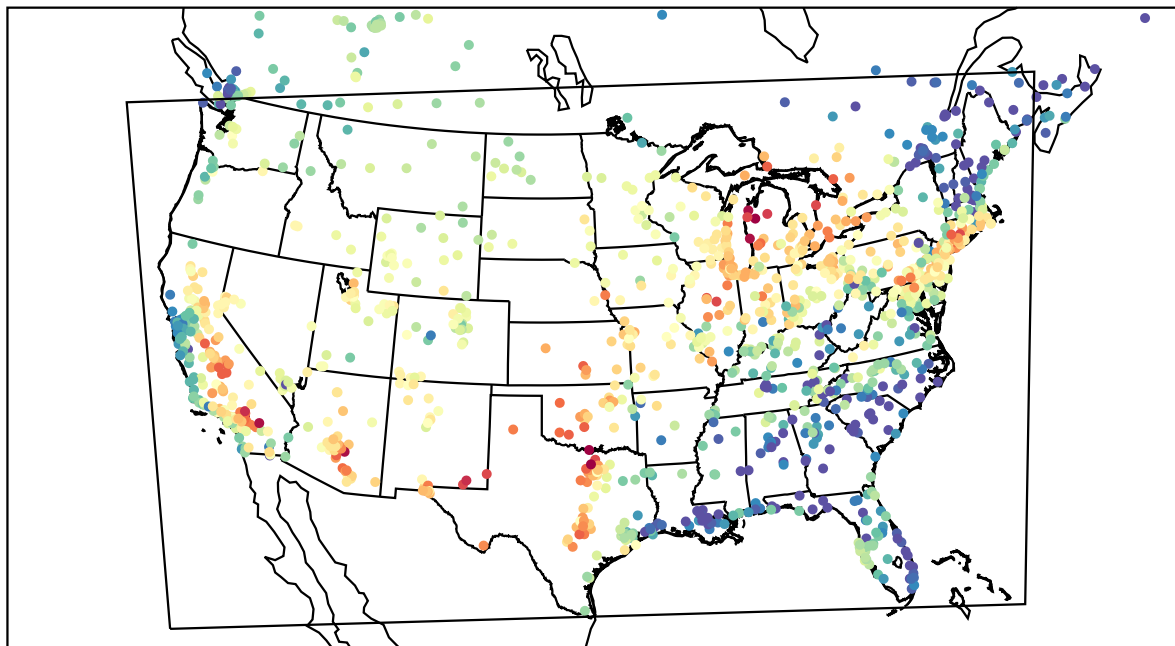
AirNOW (2022-07-01_01:00:00)
