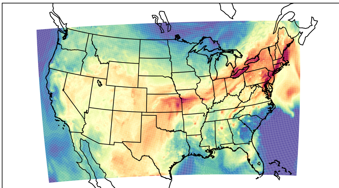
WRF (2022-07-01_18:00:00)
