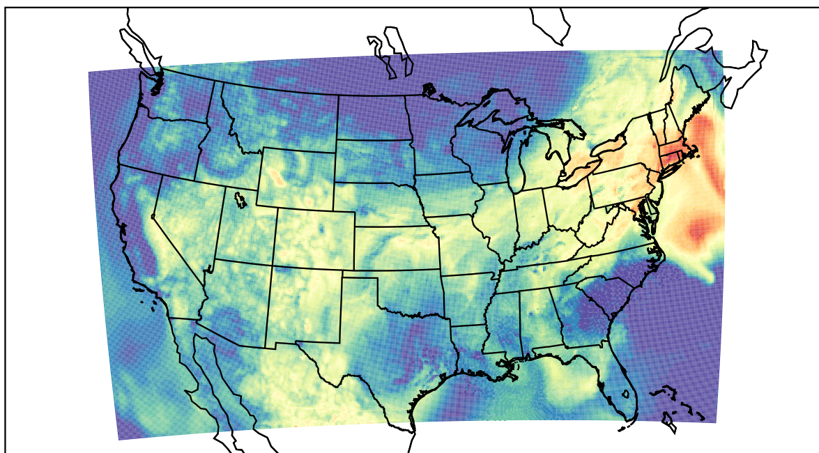
WRF (2022-07-01_14:00:00)
