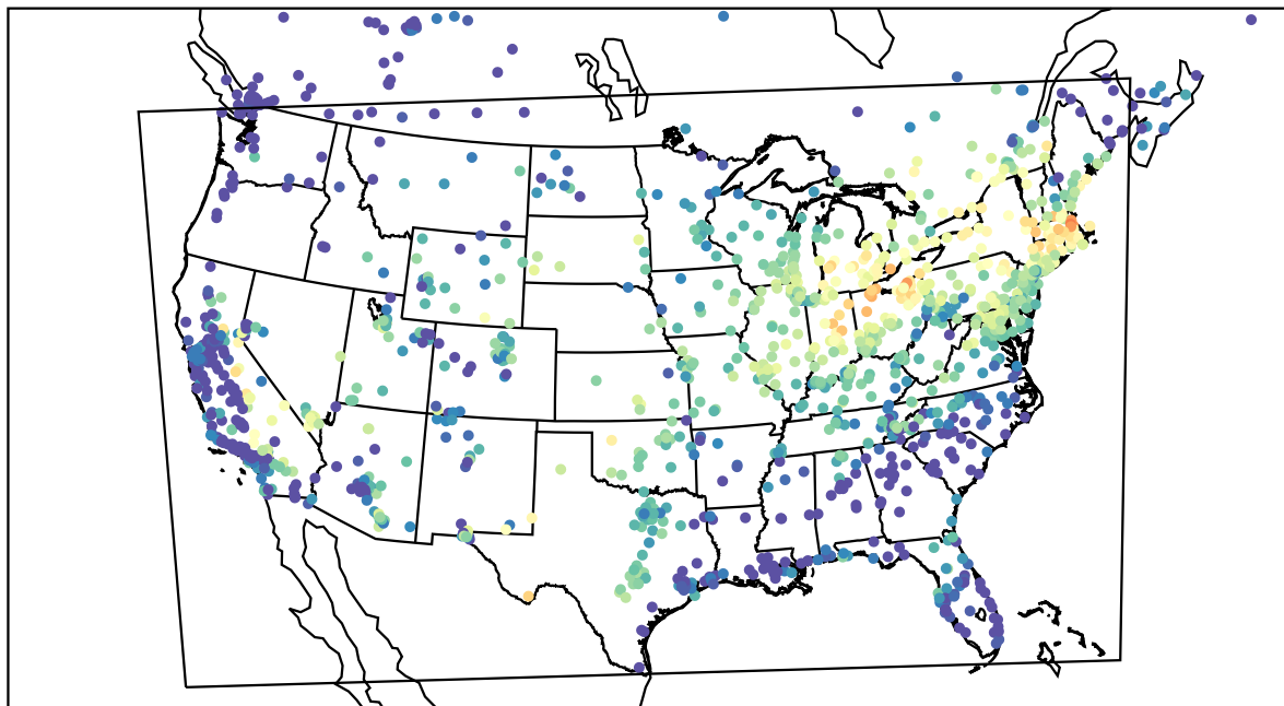
AirNOW (2022-07-01_13:00:00)
