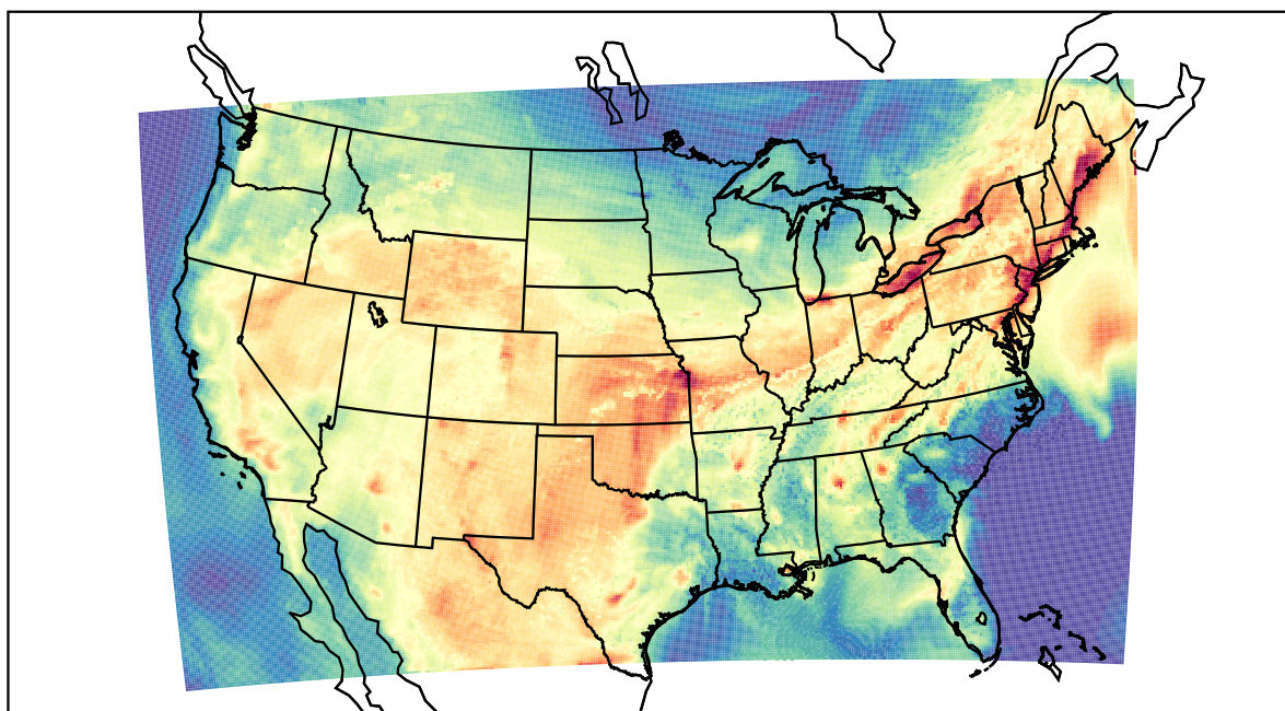
WRF (2022-07-01_22:00:00)
