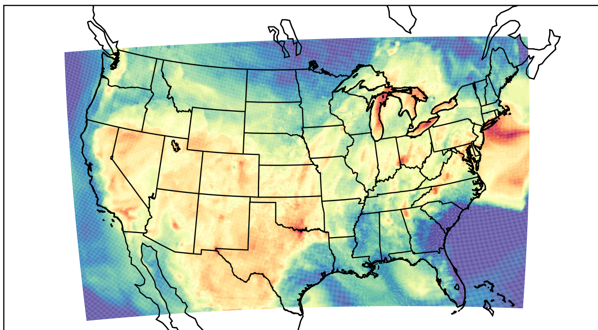
WRF (2022-07-01_01:00:00)
