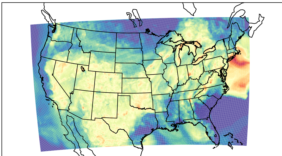
WRF (2022-07-01_03:00:00)
