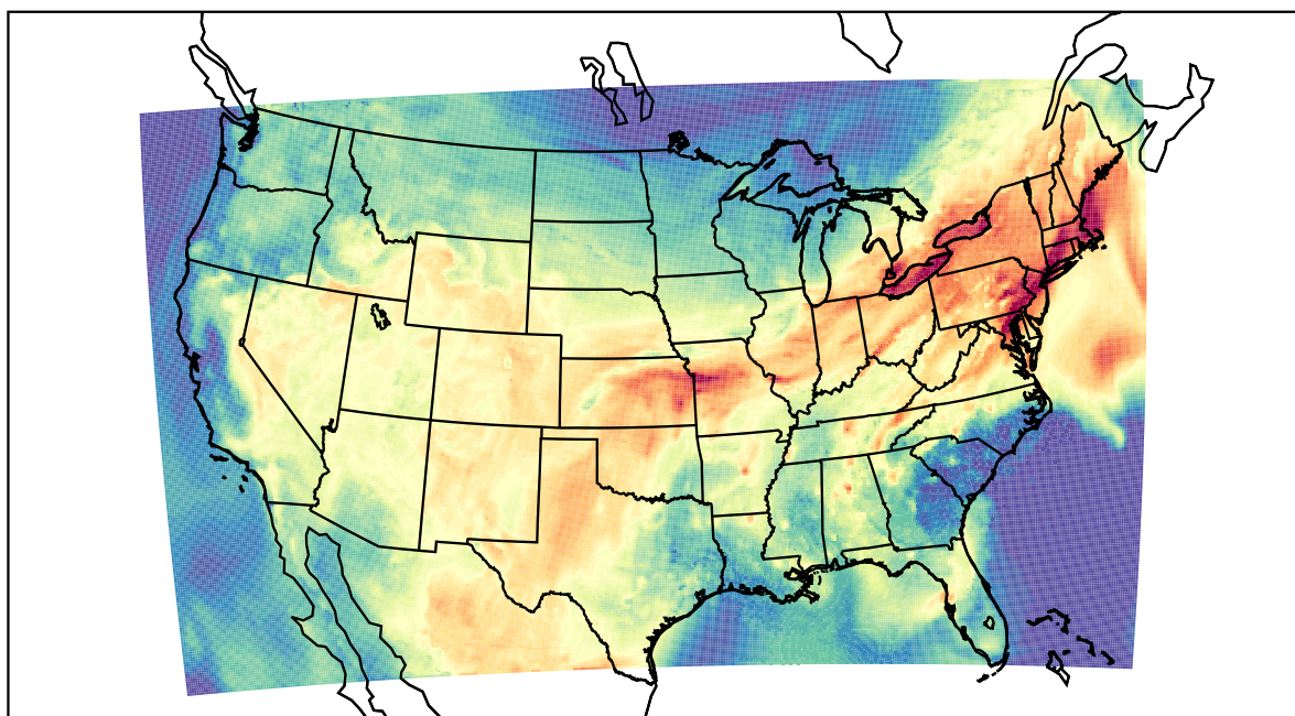
WRF (2022-07-01_17:00:00)
