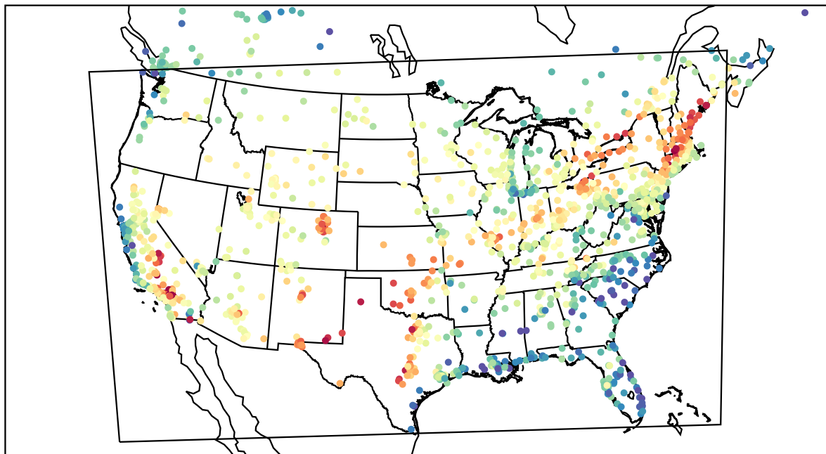
AirNOW (2022-07-01_22:00:00)
