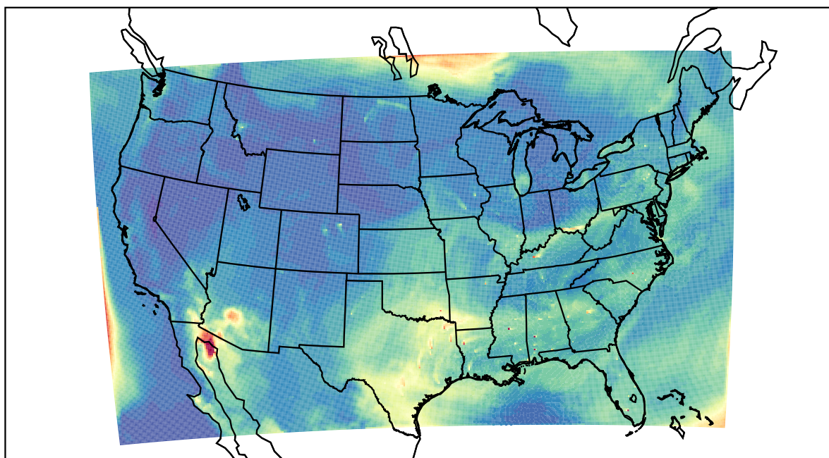
WRF 2022-07-22_18:00:00
