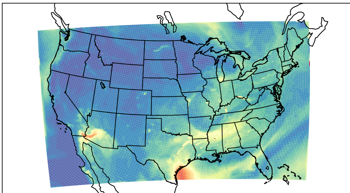
WRF 2022-07-21_18:00:00
