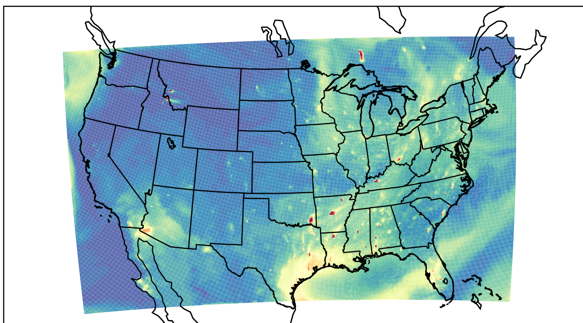
WRF 2022-07-21_01:00:00
