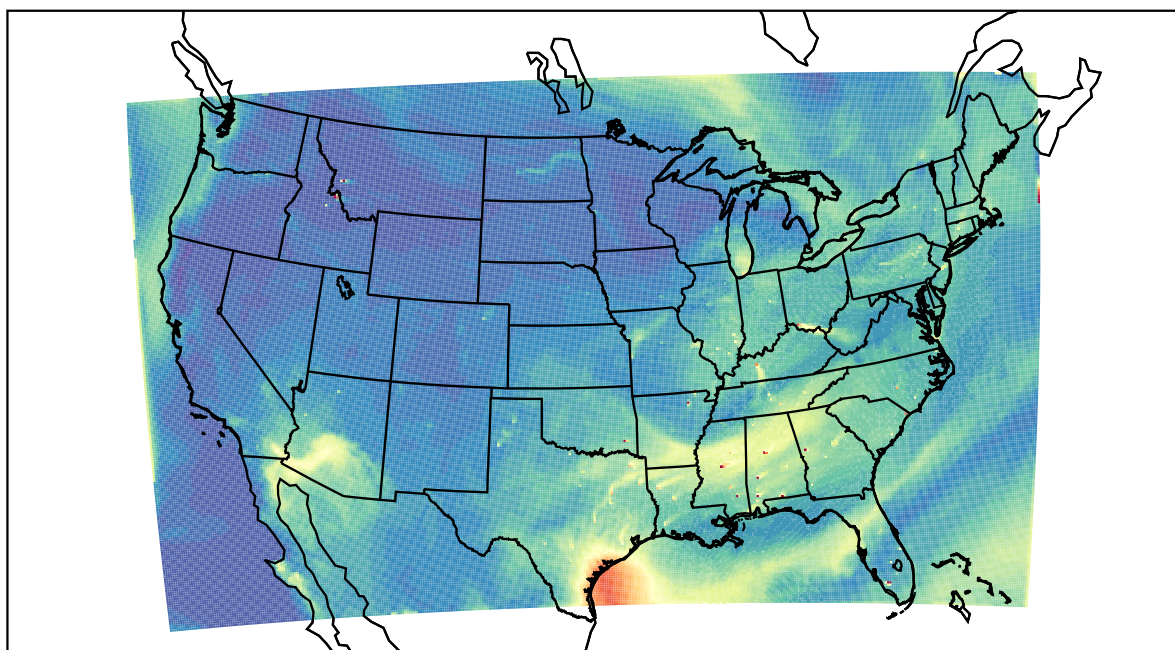
WRF 2022-07-21_20:00:00
