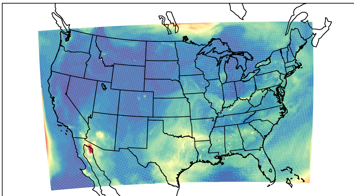
WRF 2022-07-22_19:00:00
