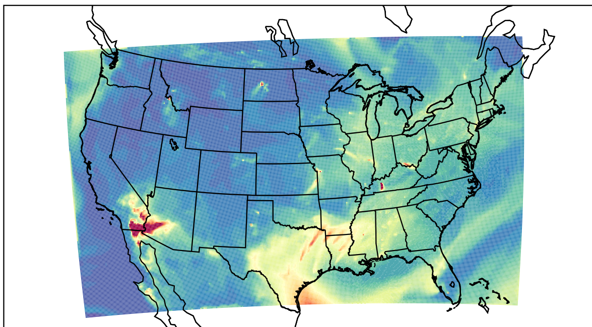
WRF 2022-07-21_10:00:00
