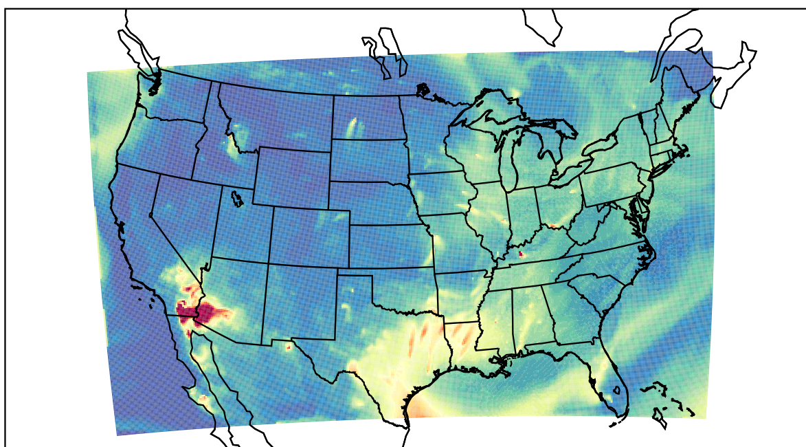
WRF 2022-07-21_07:00:00
