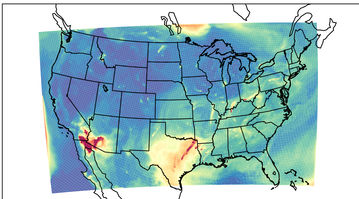
WRF 2022-07-22_14:00:00
