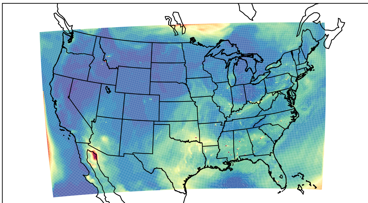
WRF 2022-07-22_20:00:00
