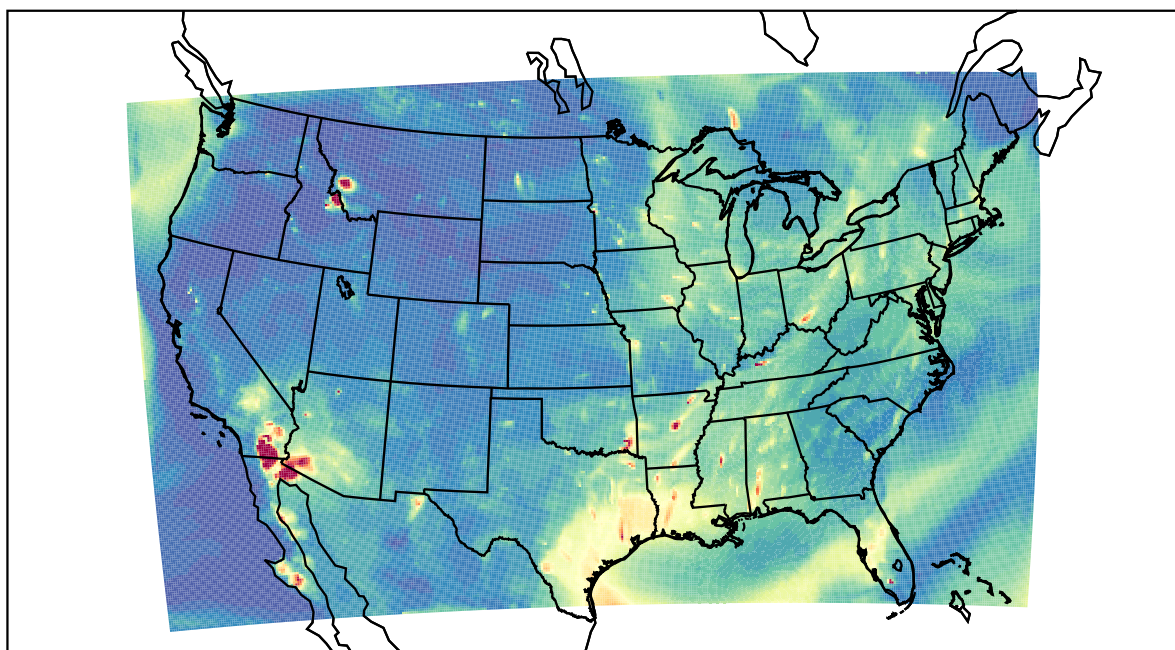
WRF 2022-07-21_03:00:00
