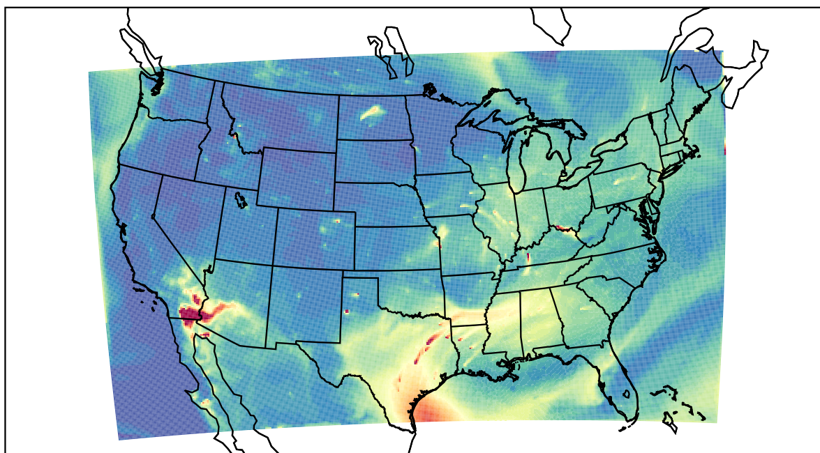
WRF 2022-07-21_14:00:00
