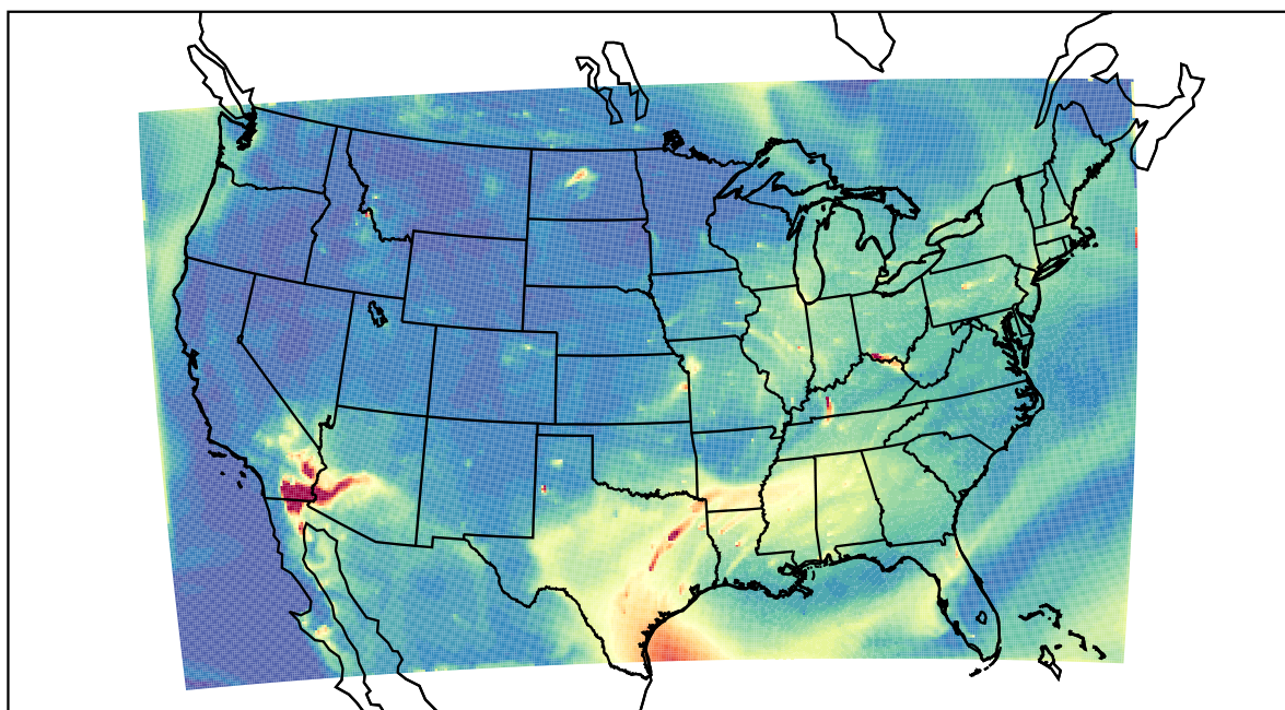
WRF 2022-07-21_13:00:00
