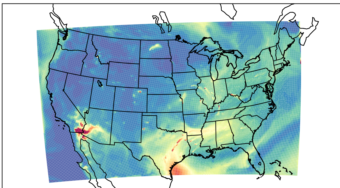
WRF 2022-07-21_15:00:00
