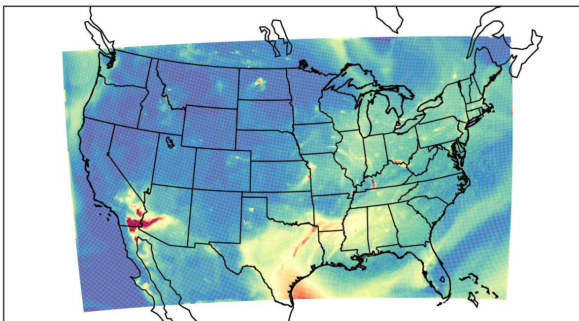
WRF 2022-07-21_12:00:00
