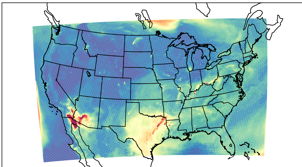
WRF 2022-07-22_15:00:00
