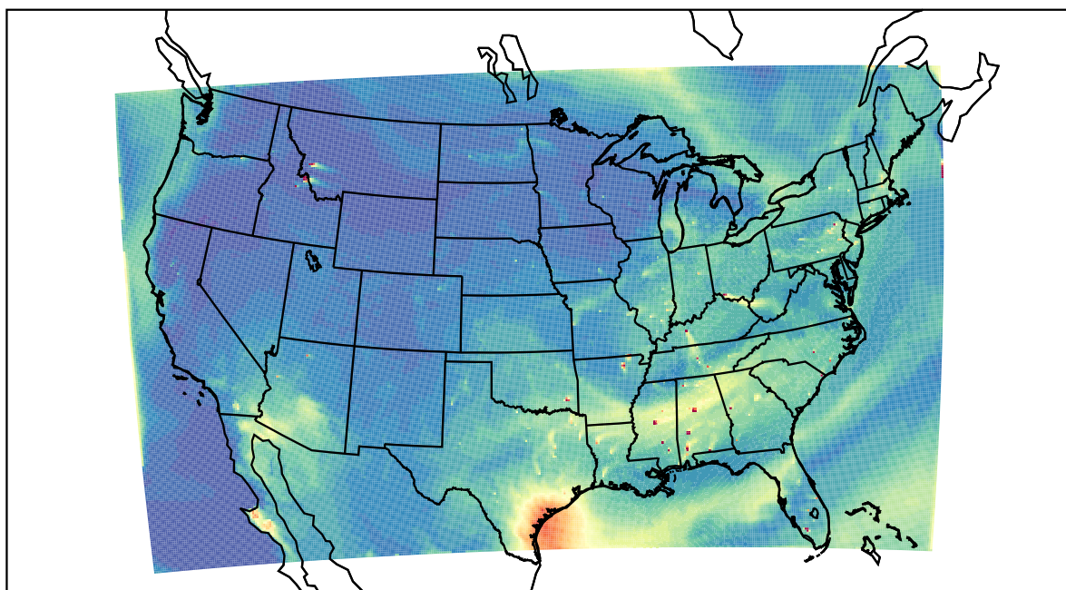
WRF 2022-07-21_23:00:00
