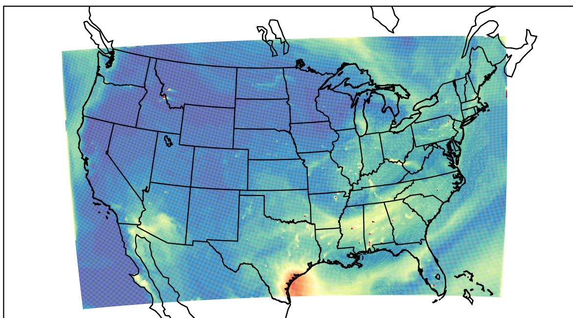
WRF 2022-07-21_22:00:00
