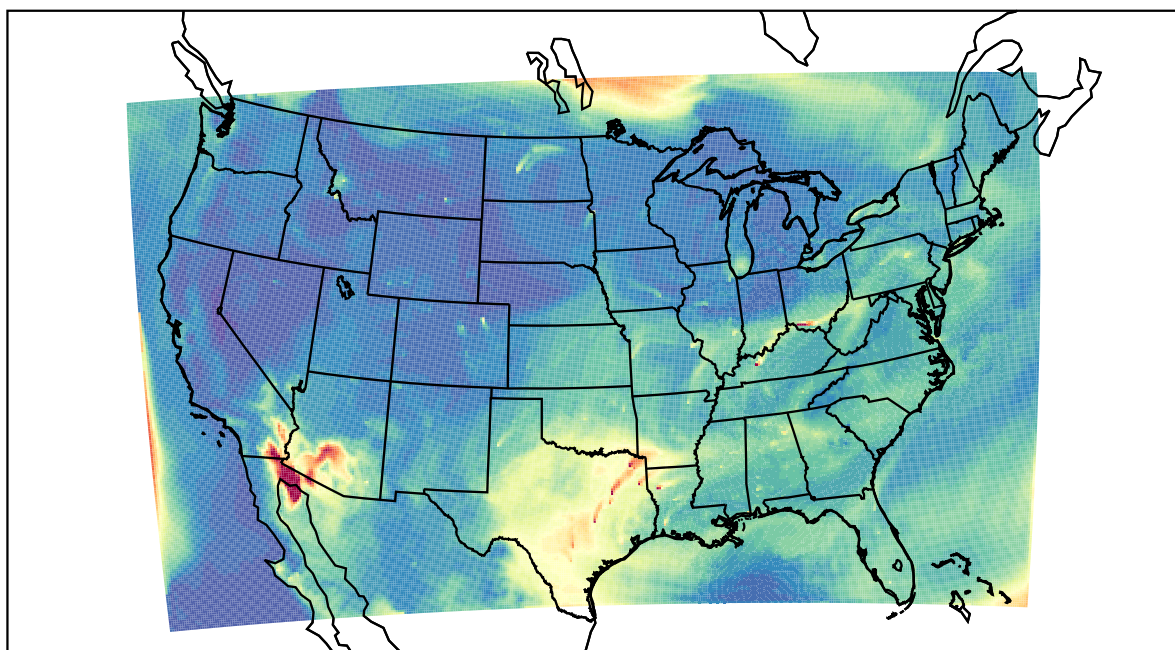
WRF 2022-07-22_16:00:00
