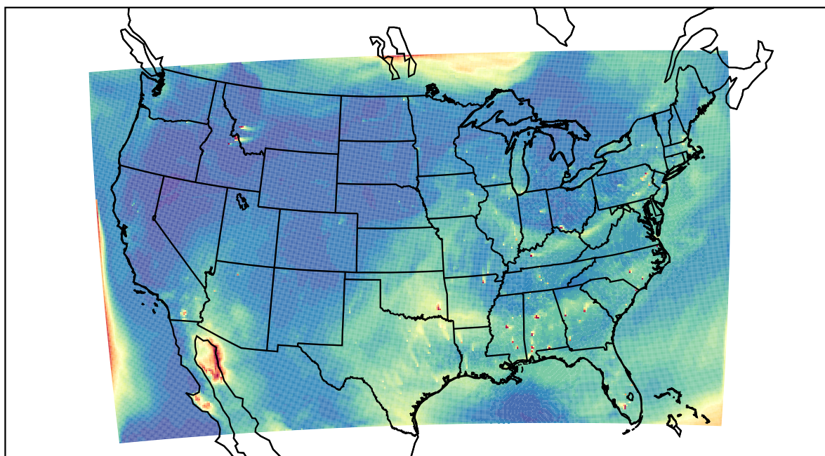
WRF 2022-07-22_23:00:00
