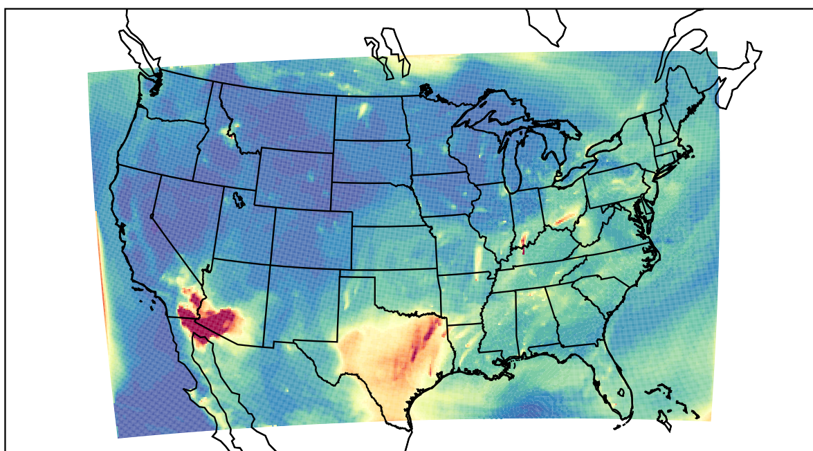
WRF 2022-07-22_12:00:00
