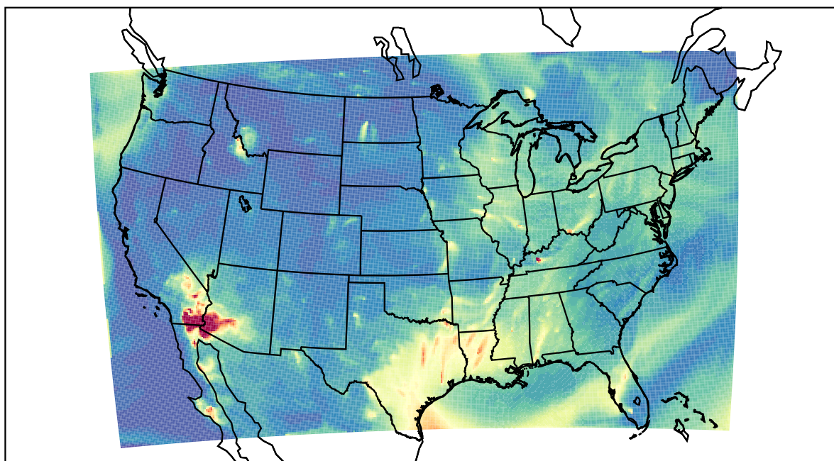
WRF 2022-07-21_06:00:00
