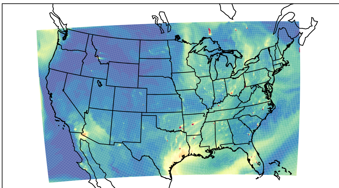
WRF 2022-07-21_00:00:00
