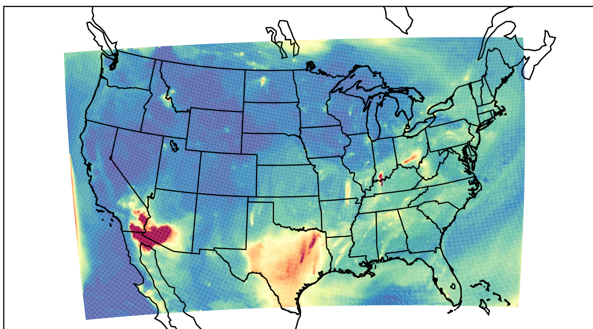
WRF 2022-07-22_11:00:00
