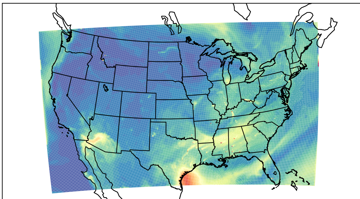
WRF 2022-07-21_19:00:00
