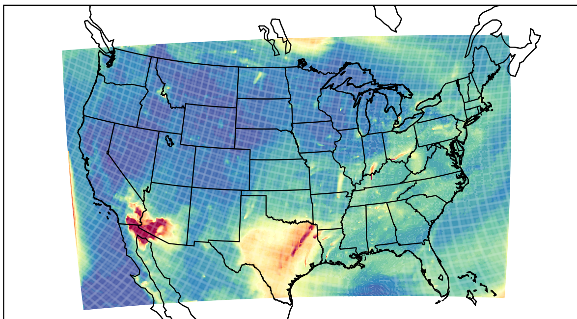
WRF 2022-07-22_13:00:00
