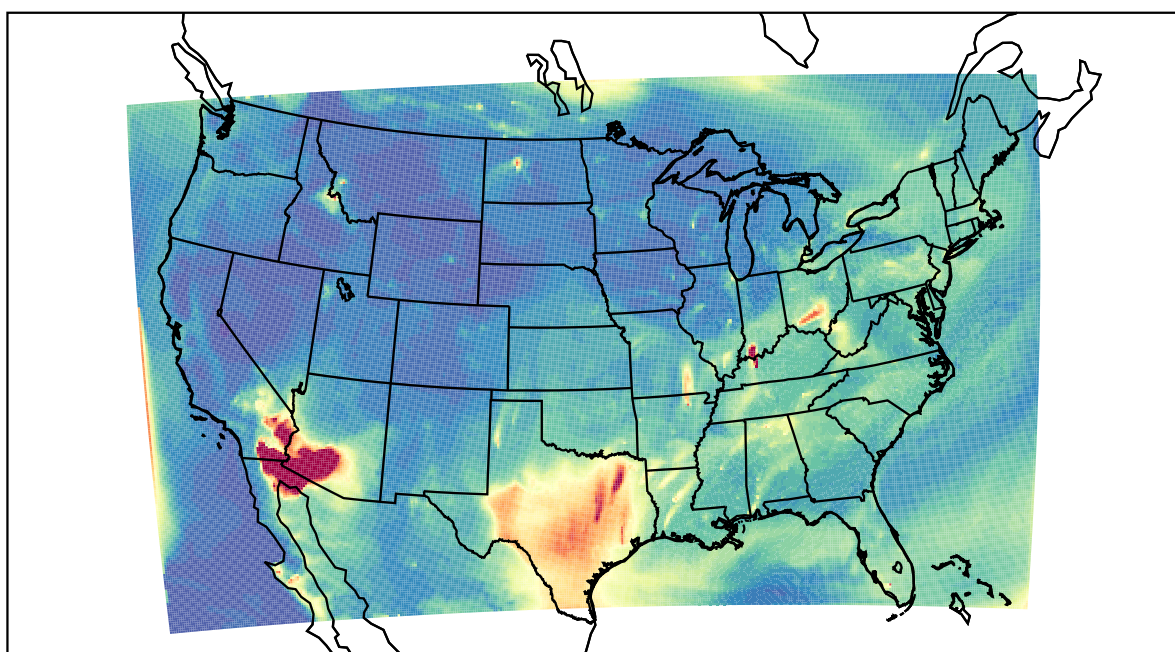
WRF 2022-07-22_10:00:00
