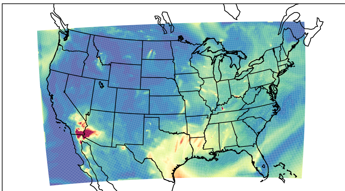
WRF 2022-07-21_08:00:00
