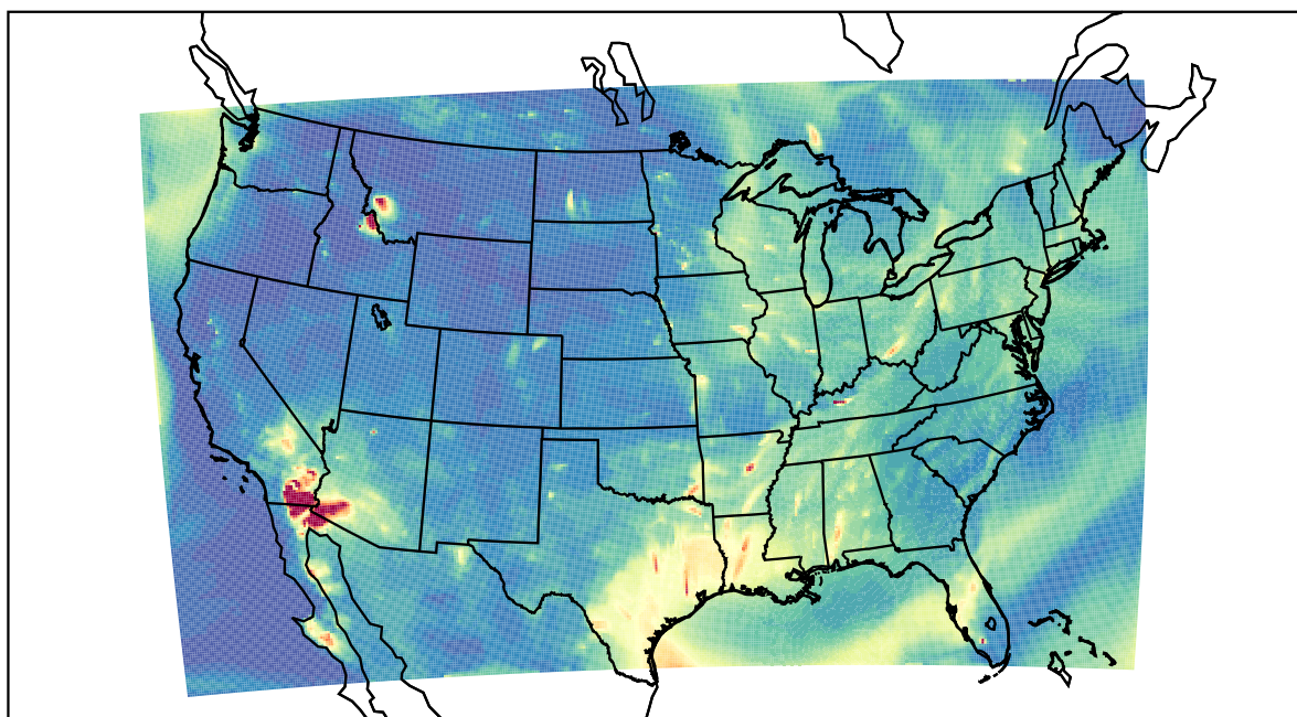
WRF 2022-07-21_04:00:00
