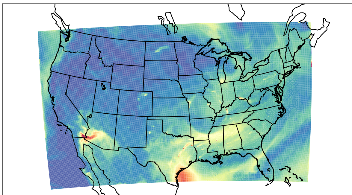
WRF 2022-07-21_17:00:00
