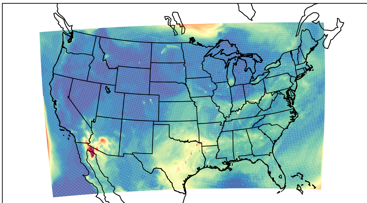
WRF 2022-07-22_17:00:00
