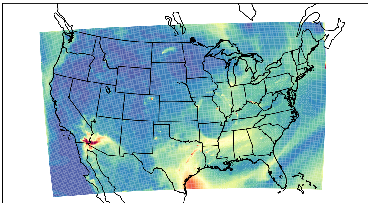
WRF 2022-07-21_16:00:00
