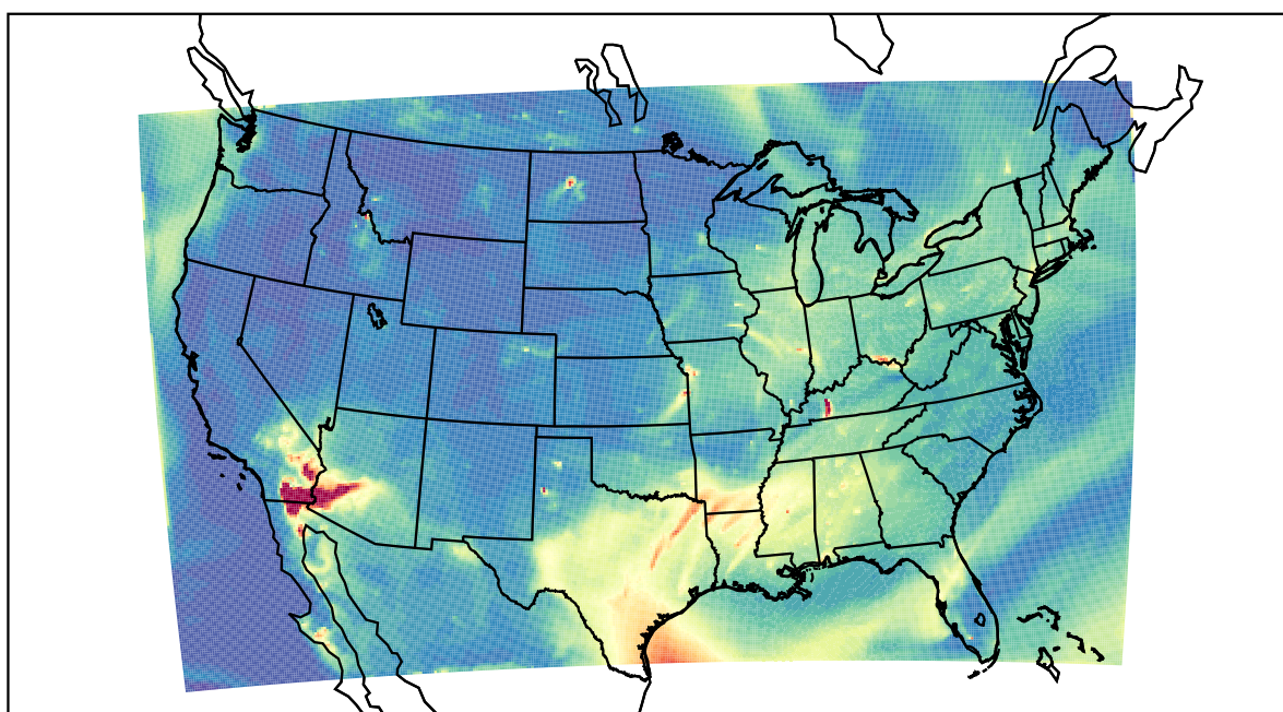
WRF 2022-07-21_11:00:00
