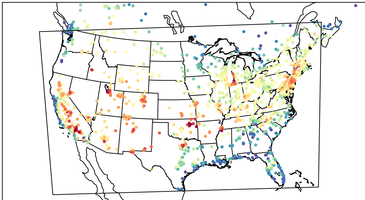
AirNOW (2022-07-21_20:00:00)
