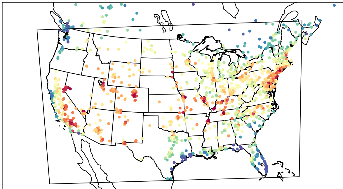
AirNOW (2022-07-22_20:00:00)
