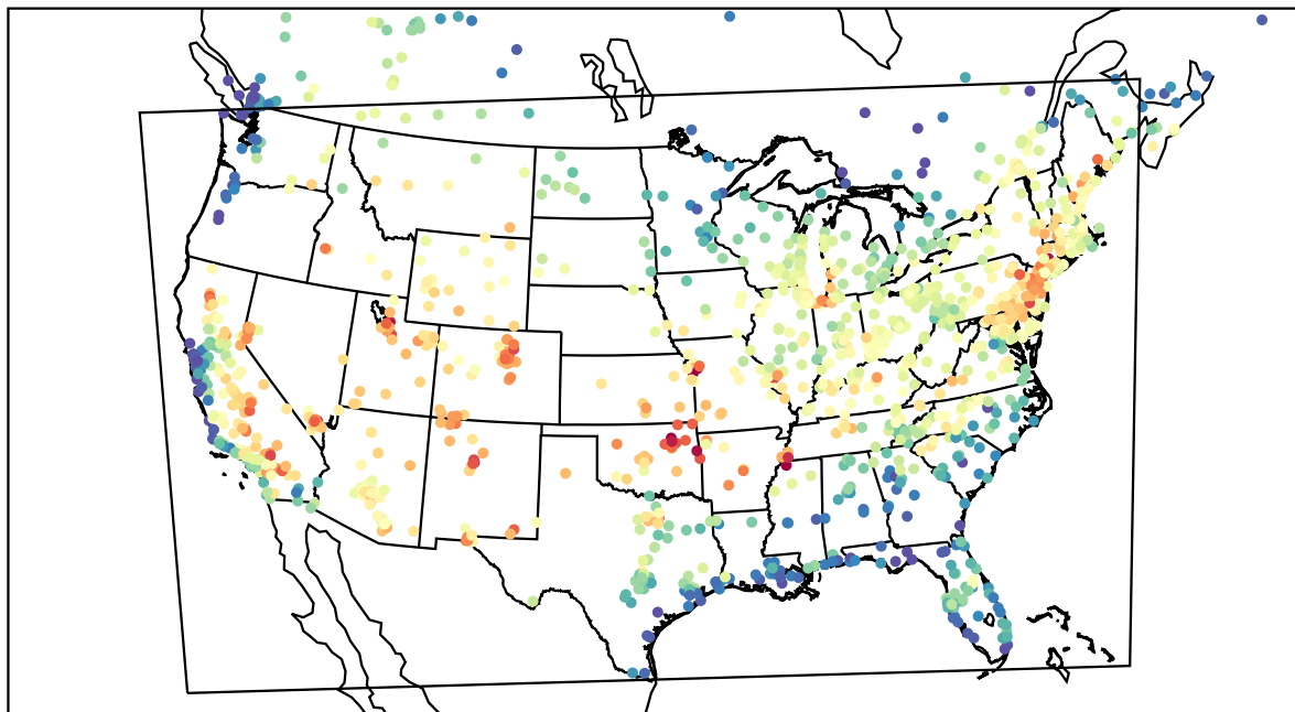
AirNOW (2022-07-21_18:00:00)
