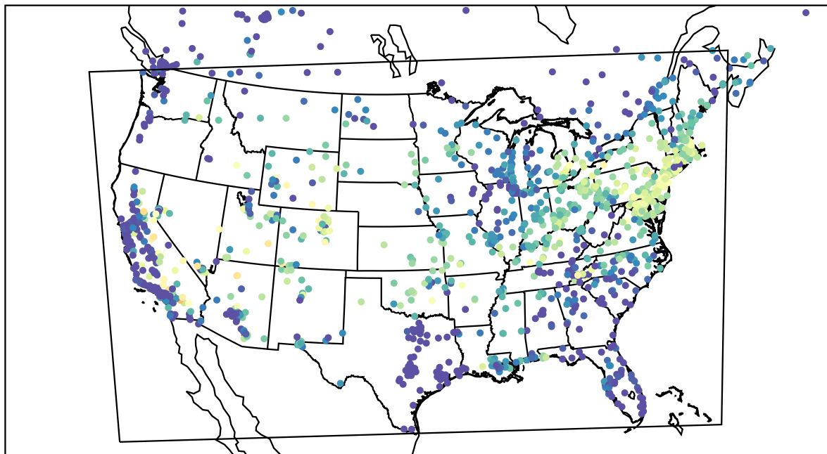
AirNOW (2022-07-22_13:00:00)
