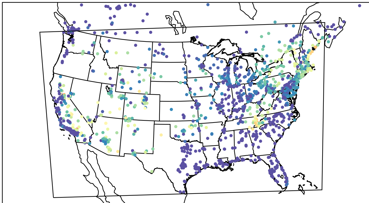
AirNOW (2022-07-21_11:00:00)
