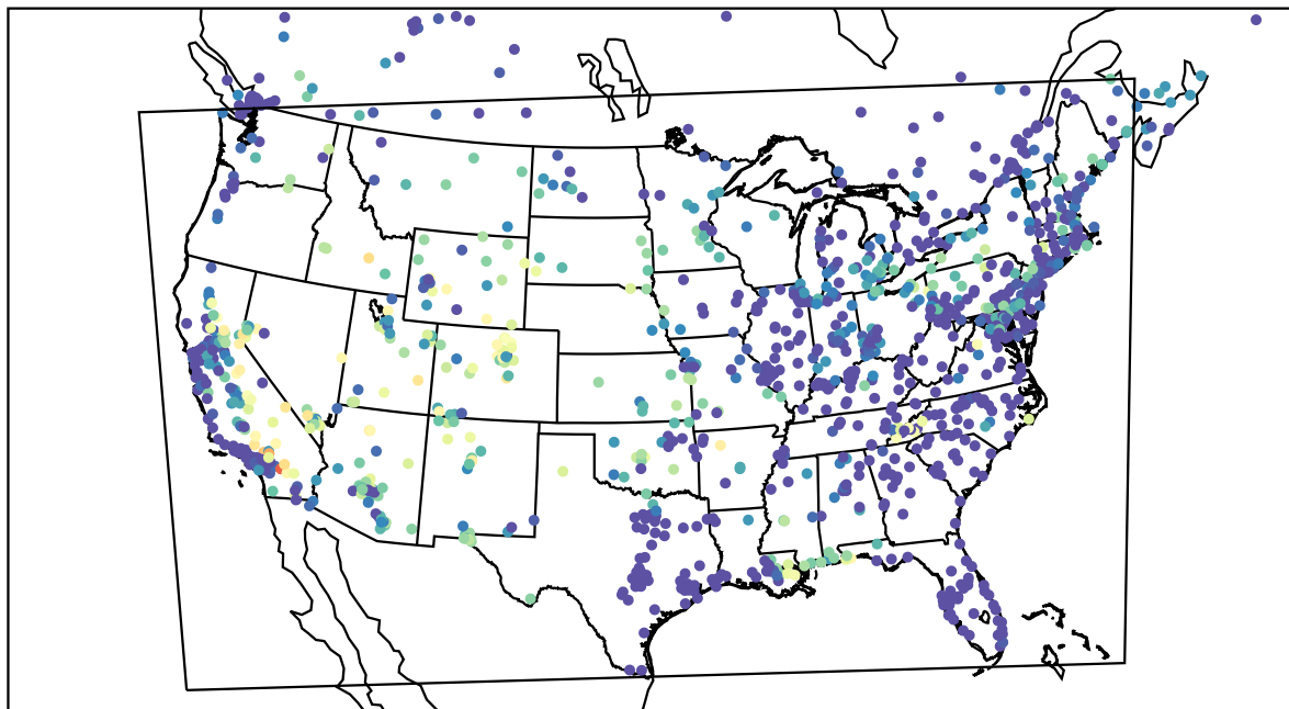
AirNOW (2022-07-22_10:00:00)
