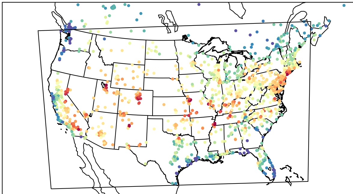
AirNOW (2022-07-22_18:00:00)
