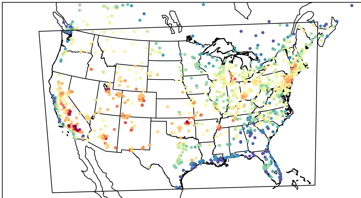
AirNOW (2022-07-21_23:00:00)
