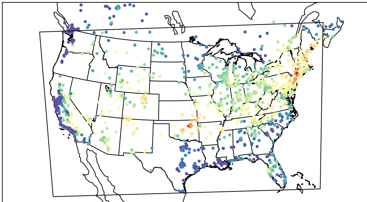
AirNOW (2022-07-21_15:00:00)
