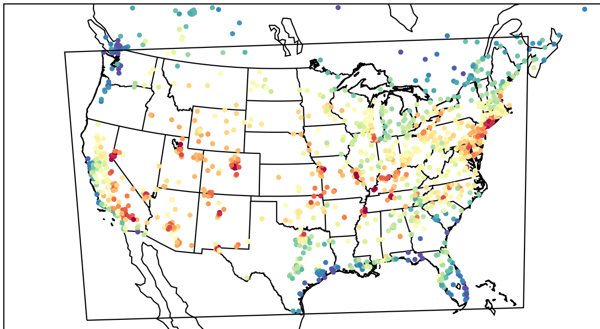
AirNOW (2022-07-22_19:00:00)
