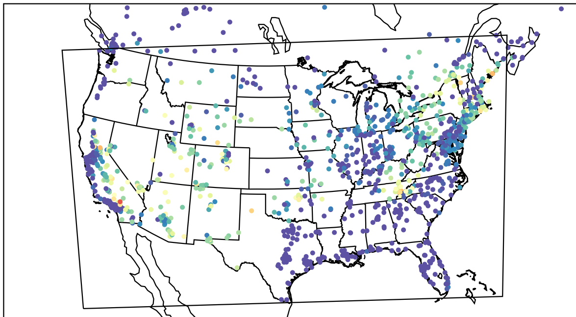
AirNOW (2022-07-21_10:00:00)
