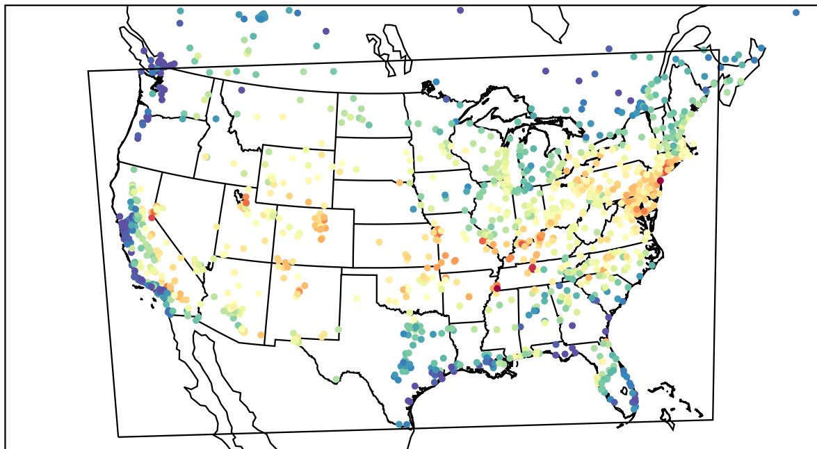
AirNOW (2022-07-22_16:00:00)
