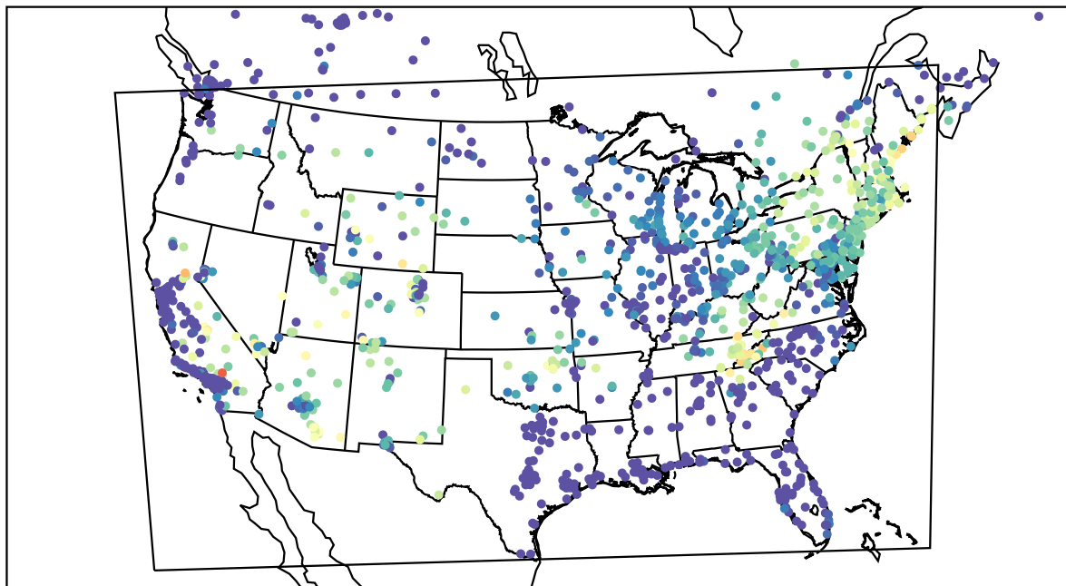
AirNOW (2022-07-21_12:00:00)
