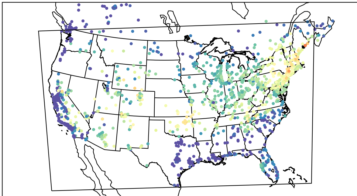
AirNOW (2022-07-21_14:00:00)
