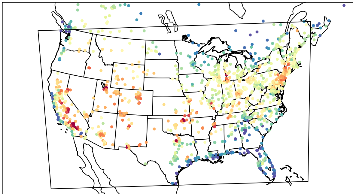
AirNOW (2022-07-21_22:00:00)
