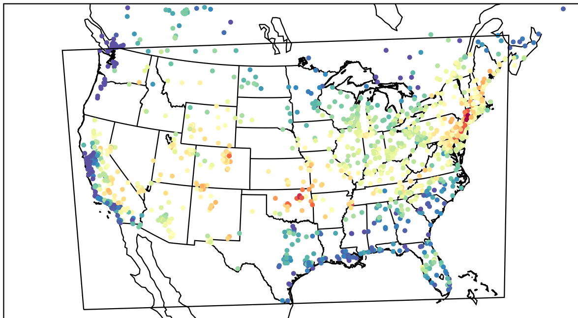
AirNOW (2022-07-21_16:00:00)
