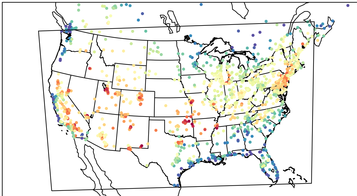
AirNOW (2022-07-21_19:00:00)
