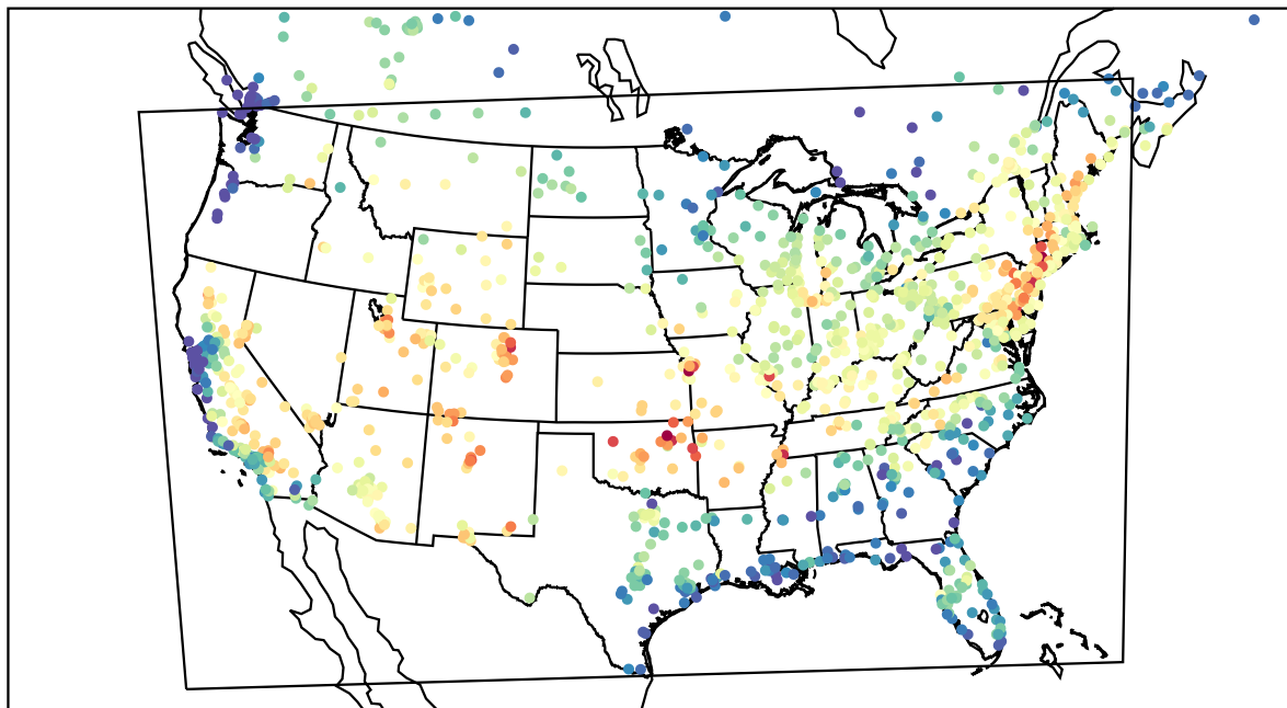
AirNOW (2022-07-21_17:00:00)
