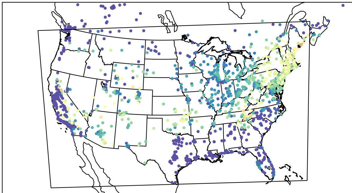
AirNOW (2022-07-21_13:00:00)
