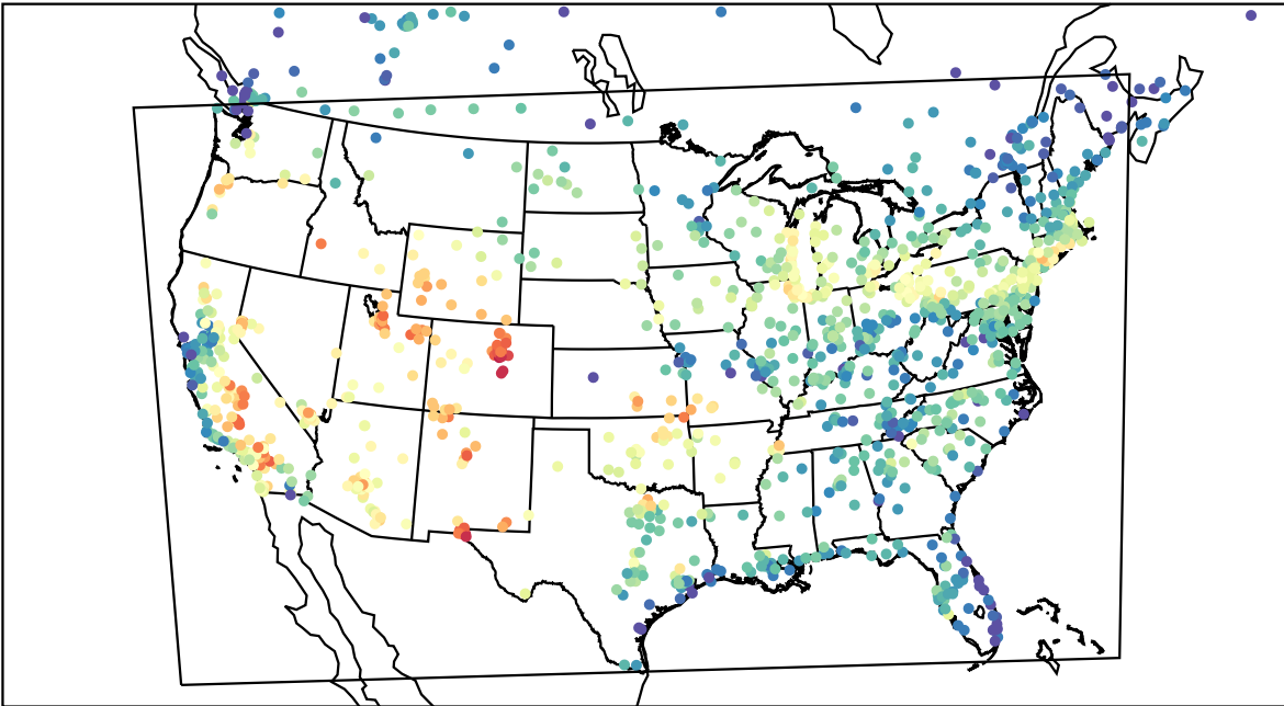
AirNOW (2022-07-26_18:00:00)
