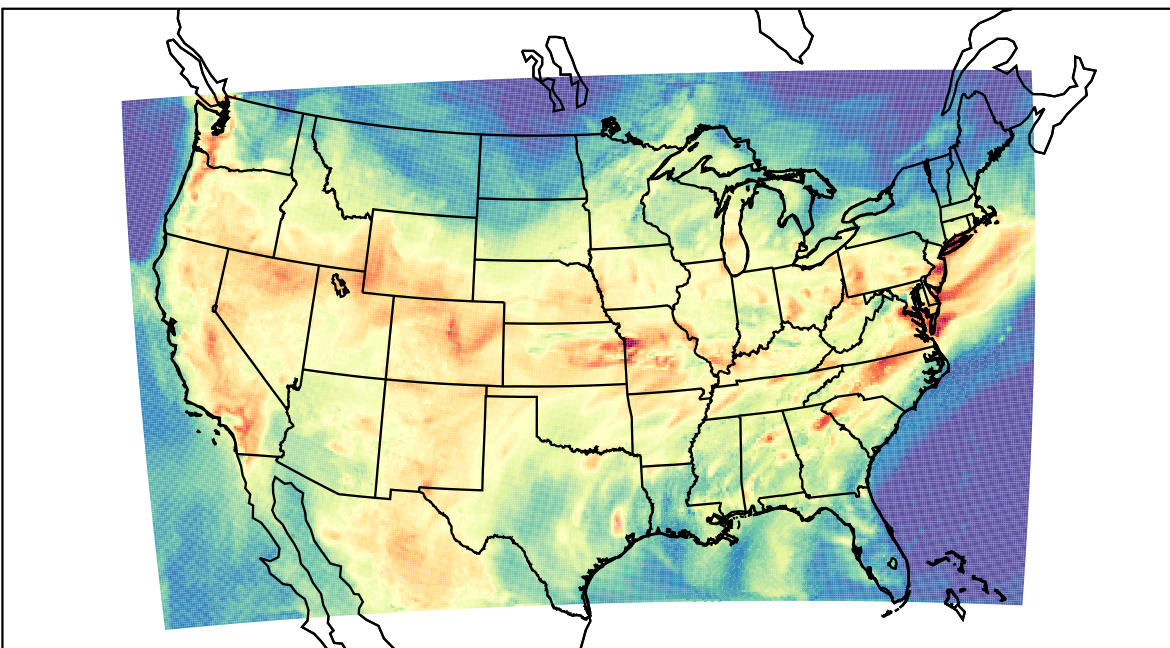
WRF (2022-07-26_19:00:00)
