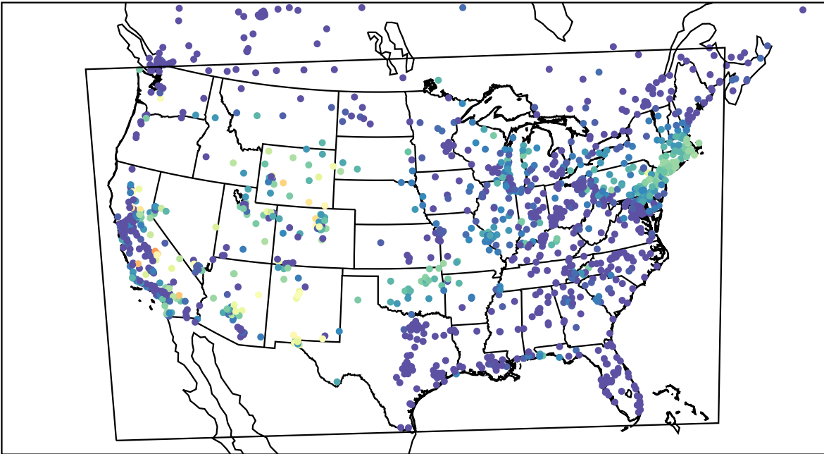
AirNOW (2022-07-26_13:00:00)
