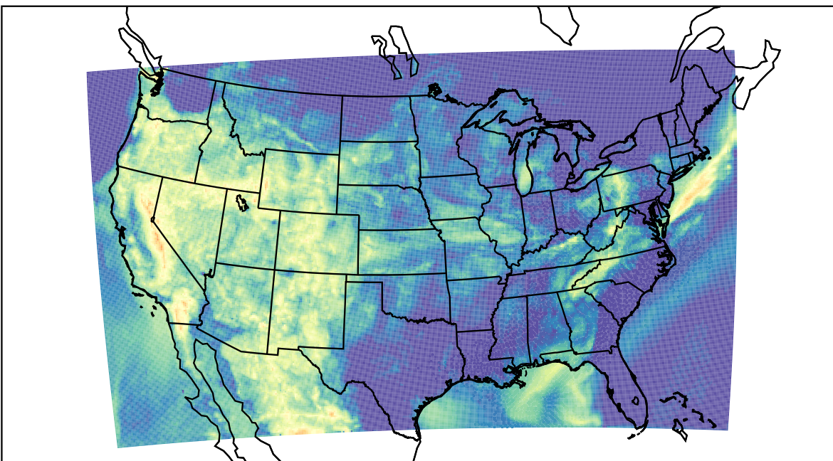
WRF (2022-07-26_10:00:00)
