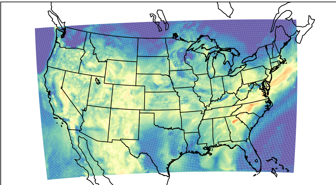
WRF (2022-07-26_15:00:00)
