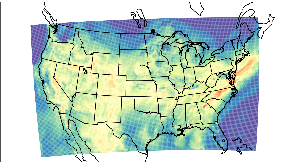
WRF (2022-07-26_16:00:00)
