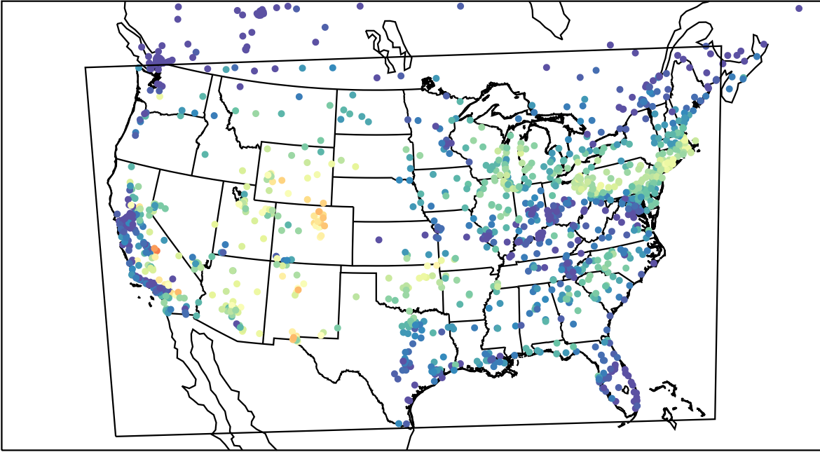
AirNOW (2022-07-26_15:00:00)
