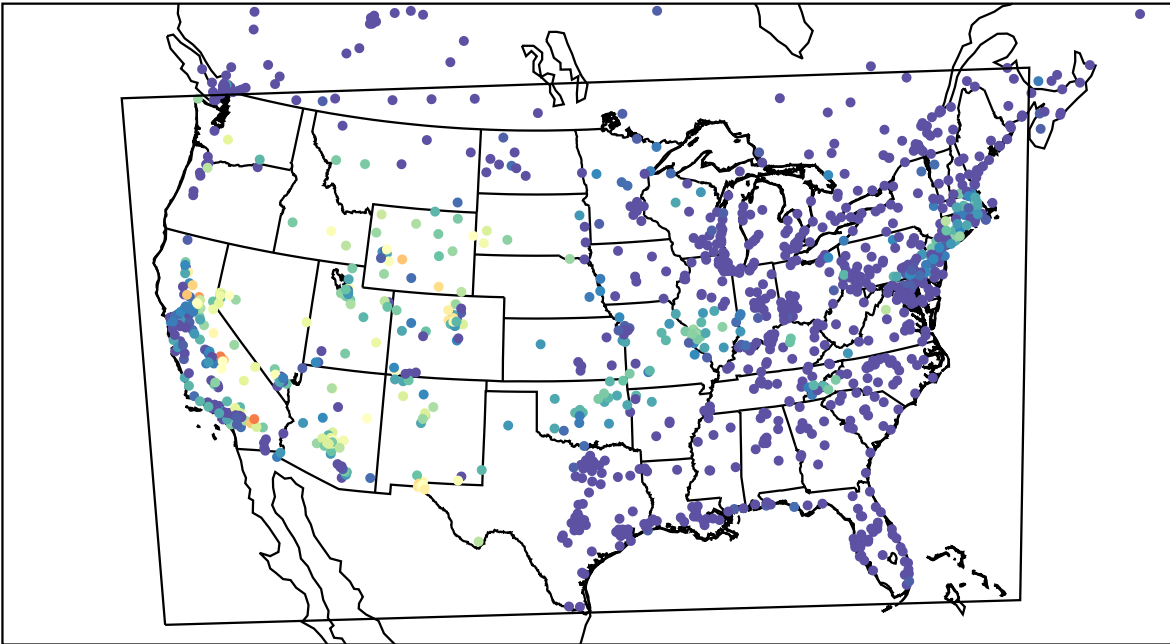
AirNOW (2022-07-26_10:00:00)
