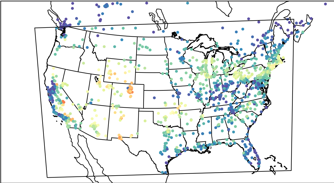
AirNOW (2022-07-26_16:00:00)
