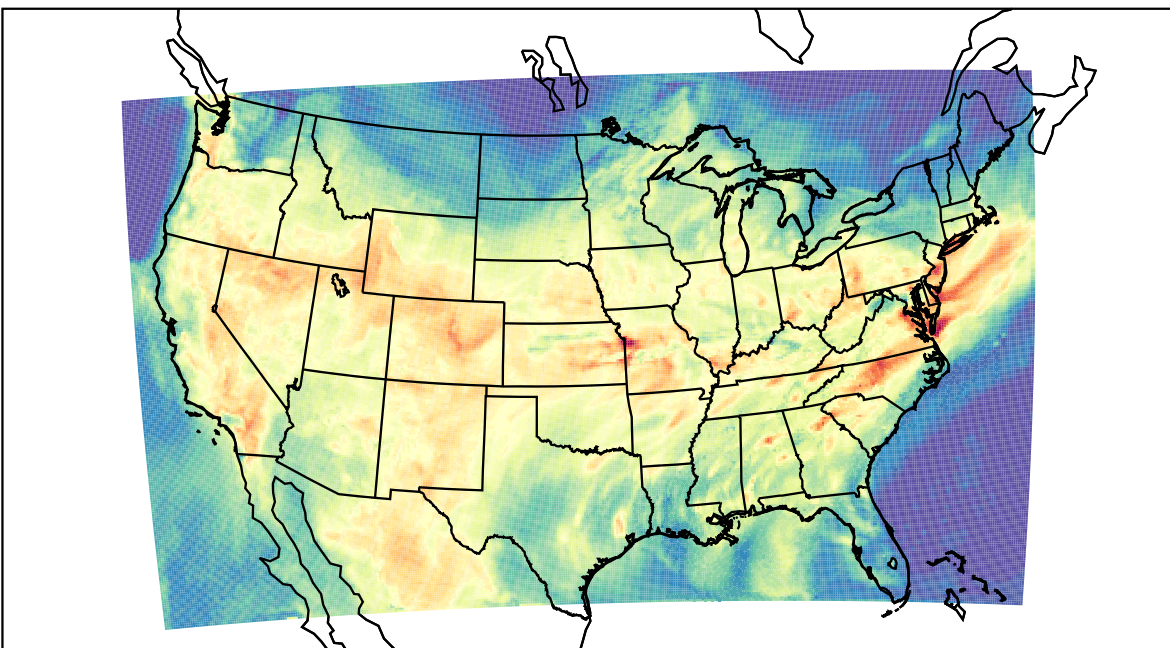
WRF (2022-07-26_18:00:00)
