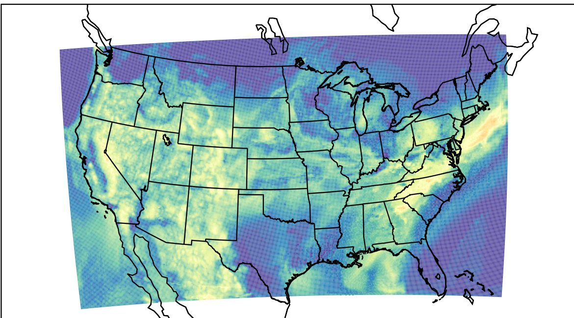
WRF (2022-07-26_14:00:00)
