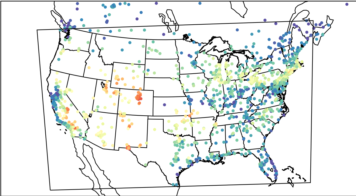
AirNOW (2022-07-26_17:00:00)
