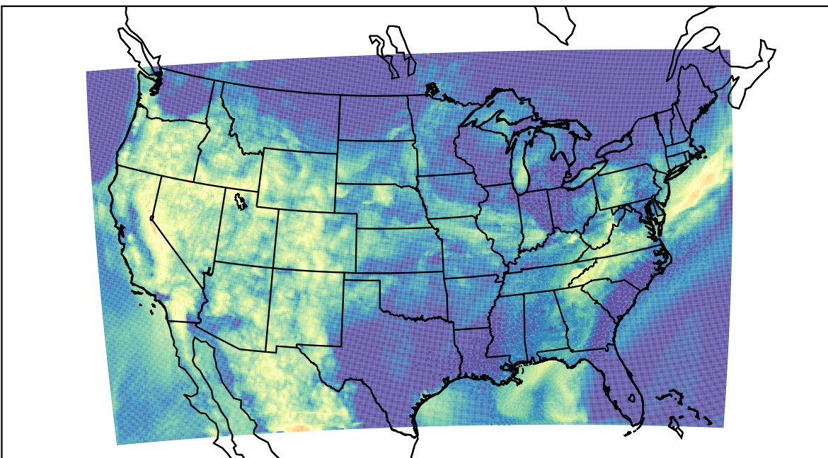
WRF (2022-07-26_13:00:00)
