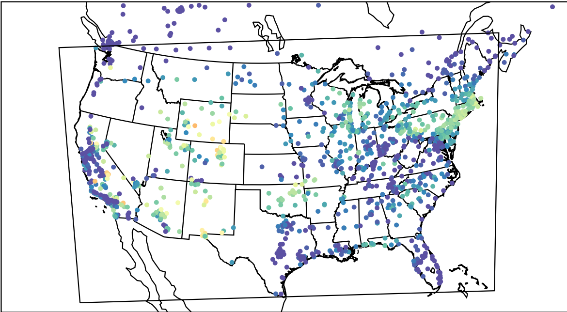
AirNOW (2022-07-26_14:00:00)
